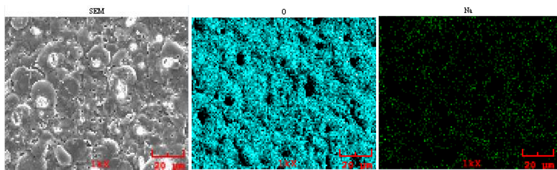
Şekil 7.11. (M-Si-1-Ag)-2 numaralı numunenin mikro ark oksidasyon sonrasındaki SEM fotoğrafı ve EDS analizi
