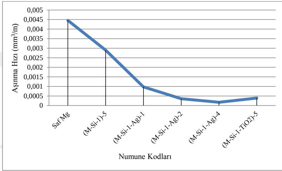
Şekil 7.21. Saf magnezyum ve (M-Si-1)-5, (M-Si-1-Ag)-1, (M-Si-1-Ag)-2, (M-Si-1-Ag)-4, (M-Si-1- \text{TiO}_2 )-5 kodlu numunelerde 3N yük altında aşınma hızında gözlemlenen değişimler
