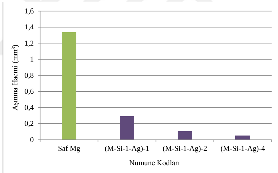
Şekil 7.17. Saf magnezyum ve (M-Si-1-Ag)-1, (M-Si-1-Ag)-2, (M-Si-1-Ag)-4 kodlu numunelerde 3N yük altında aşınma kaybında gözlemlenen değişimler
