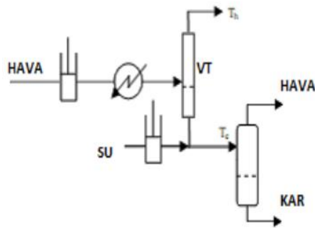
Şekil 3.16. Vorteks tüp ile kar üretme sisteminin şematik gösterimi [55,57].
