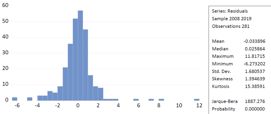
Şekil 5-6 Kalıntılar İçin Normallik Testi Sonuçları
