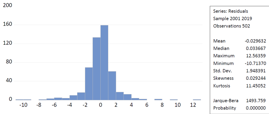
Şekil 5-8 Kalıntılar İçin Normallik Testi Sonuçları
