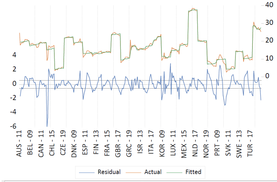
Şekil 5-3 FMOLS Tahmincisi PT-EMP Bağımlı Değişkeni Gerçek, Tahmin ve Kalıntılar Grafiği
