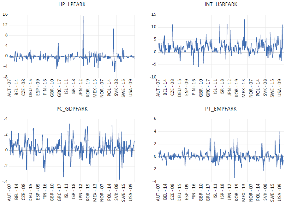
Şekil 5-2 Fark Serilerinin Grafikleri
