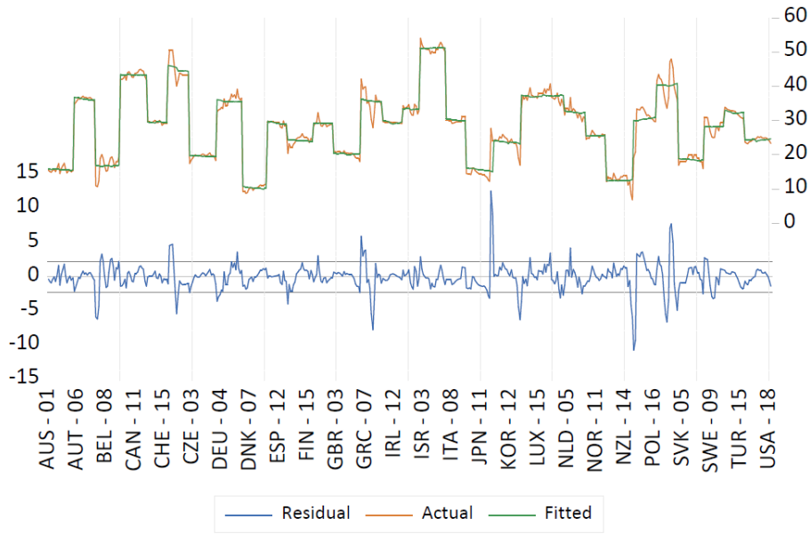
Şekil 5-7 FMOLS Tahmincisi HP+LP Değişkeni Gerçek, Tahmin ve Kalıntılar Grafiği
