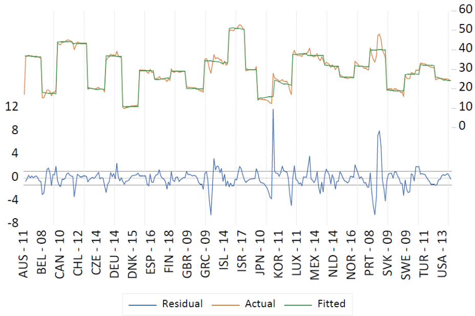
Şekil 5-5 FMOLS tahmincisi HP+LP Değişkeni Gerçek, Tahmin ve Kalıntılar Grafiği
