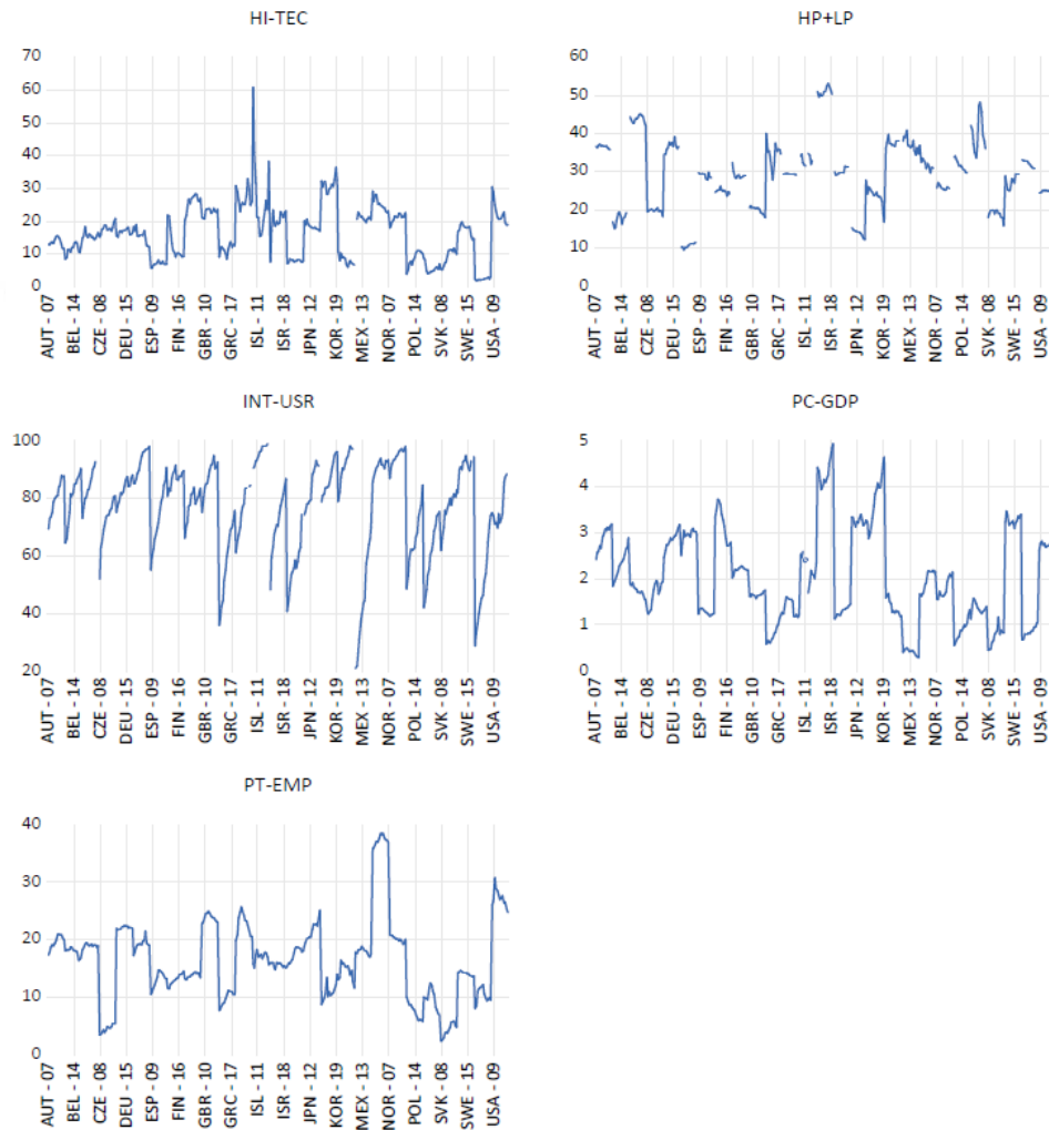
Şekil 5-1 Serilerin Düzey Değerlerinde Grafikleri
