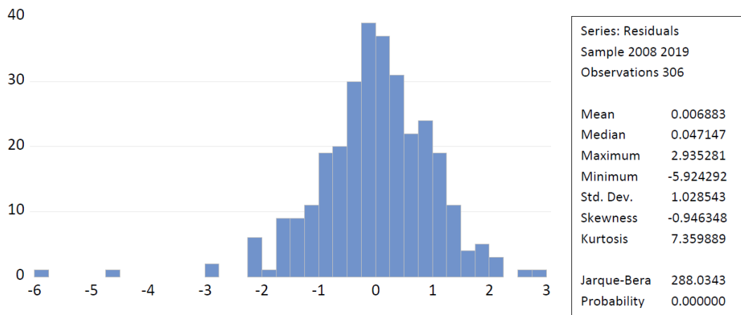
Şekil 5-4 Kalıntılar İçin Normallik Testi Sonuçları
