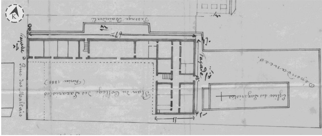
Şekil 5.30: Propaganda Koleji Planı, (Cumhurbaşkanlığı Osmanlı Arşivi, İMMS 82/3522, 1886).
