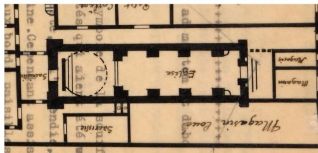
Şekil 5.15: Lazarist Kilisesi Plamı (Droulez, 1945).
