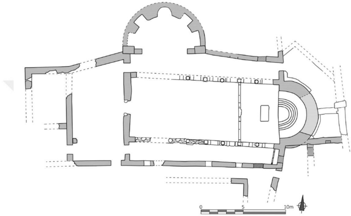
Şekil 10. 3 No'lu Kilise planı (Olympos kazı arşivi)
