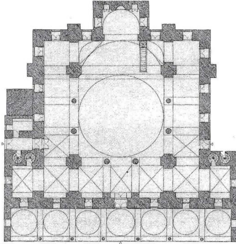
Çizim 3. 2: Şerafeddin Cami Planı (Baş, 1999, s. 237)
