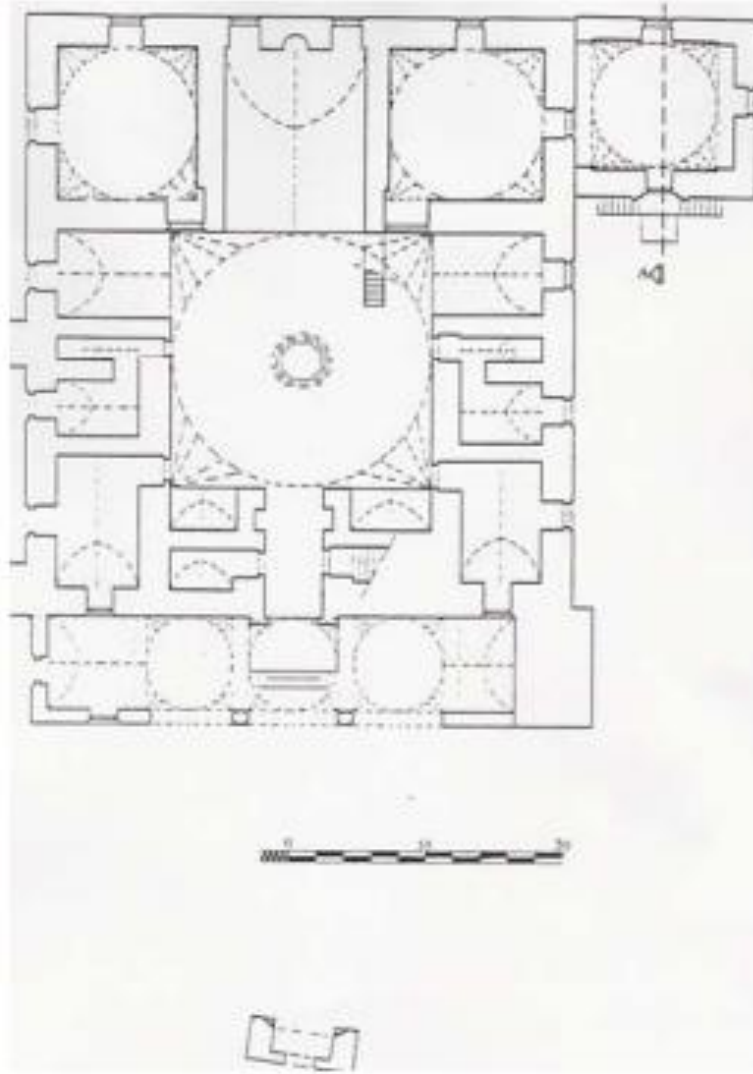
Çizim 3. 4: Karaman İbrahim Bey İmareti Planı (Ksragöz, 2012’den Alınmıştır)
