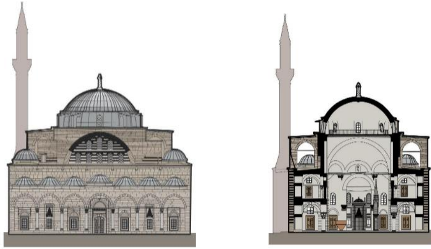
Çizim 3. 3: Şerafeddin Cami Kuzey Cephesi ve B-B Kesiti (Baş, 1999, s. 237)
