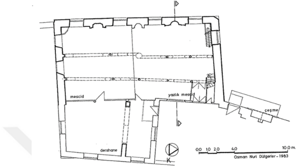
Çizim 3. 5: Hoca Mahmud, Mektep, Cami ve Türbesi Planı (O.N. Dülgerler'den)
