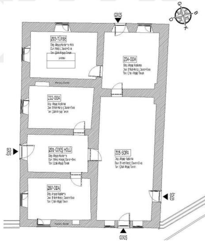
Çizim 3. 1: Ebû İshak Kâzerûnî Zaviyesi Planı (Toydemir, 2022)
