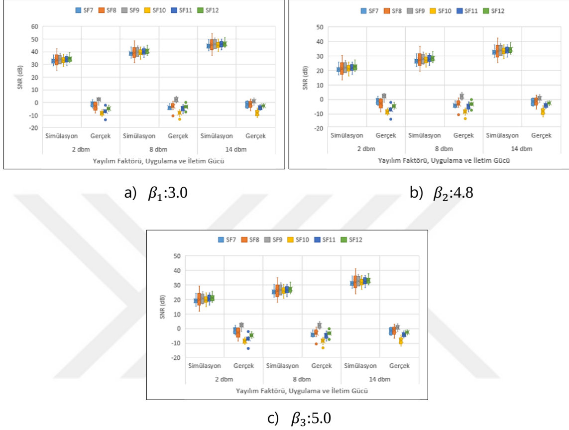
Şekil 5.30. Simülasyon ve gerçek uygulamaya göre 467m deki konum için SNR kıyaslaması
