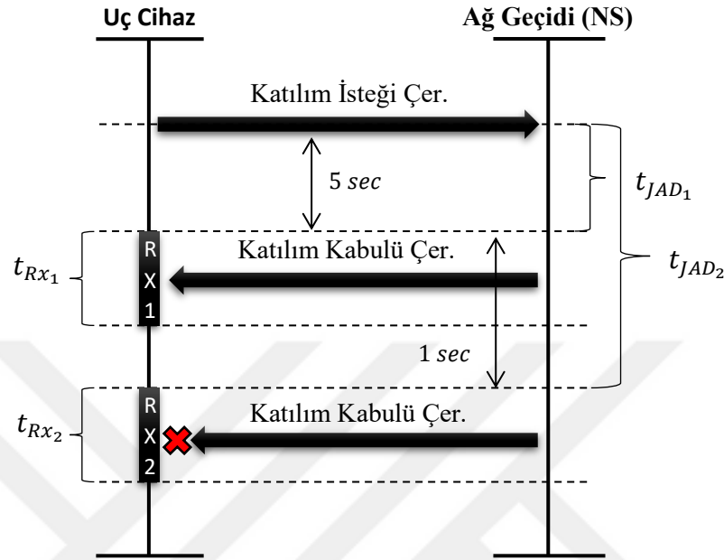
Şekil 4.21. LoRaWAN'da OTA aktivasyon grafiği
