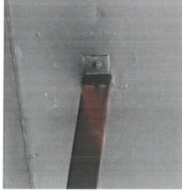
Resim 13. Çelik Dübelle Tavana Monte İşlemi
