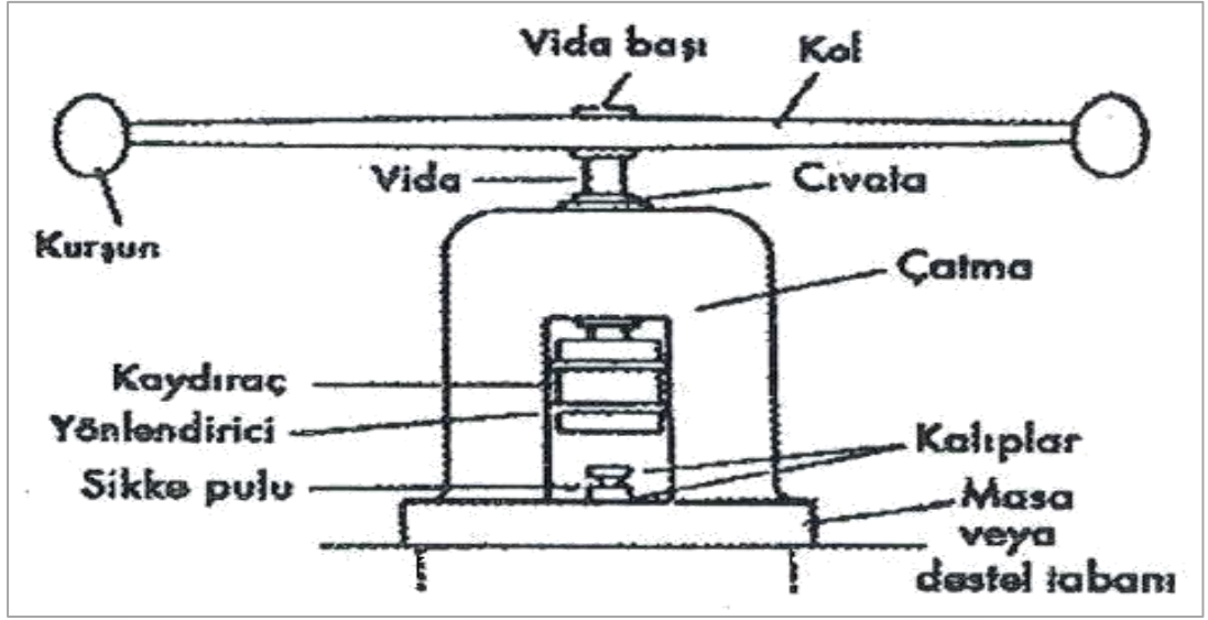
Çizim 4. Mekanik Darp Tekniği Sikke Basma Makinesi (Cecile Morrison'dan, 2002)
