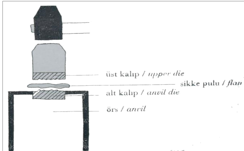
Çizim 3. Sikke (Darp) Basım Düzeneği (Mehmet Özhanlı'dan, 2011)
