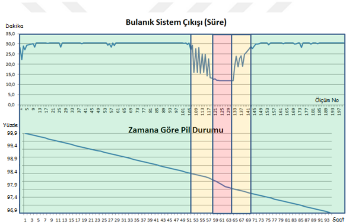
Şekil 4.7. Bulanık sistem çıkışına göre pilin doluluk durumu
