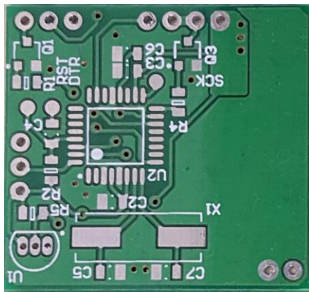
Resim 3.3. Verici sistemin devre kartının görüntüsü
