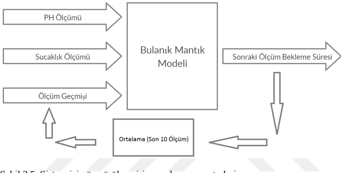
Şekil 3.5. Sistem için ön görülen giriş ve çıkış parametreleri
