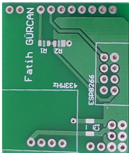
Resim 3.4. Alıcı sistemin devre kartının görüntüsü
