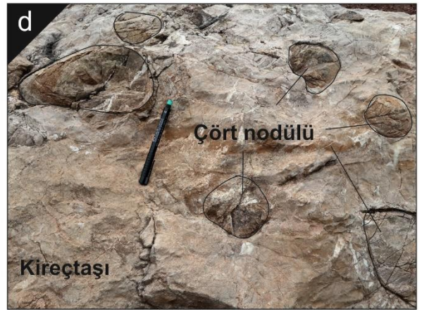
Şekil 5.8: a) Vezirler melanjını oluşturan altere serpentinit, b) Metagranit ve melanj içerisindeki kireçtaşı bloğu arasındaki tektonik kontak ve kireçtaşlarında normal fay, c) Kireçtaşlarının genel görünümü, d) Kireçtaşları içerisinde gözlenen çört nodülleri
