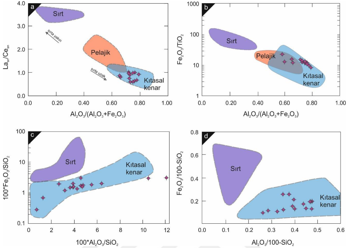
Şekil 6.4: a. La_{SN}/Ce_{SN}-Al_2O_3/(Al_2O_3 + Fe_2O_3) , b. Fe_2O_3/TiO_2- Al_2O_3/(Al_2O_3 + Fe_2O_3) , c. 100*Fe_2O_3/SiO_2-100* Al_2O_3/SiO_2 , d. Fe_2O_3/100*SiO_2-Al_2O_3/100-SiO_2 diagramı. Sirt, pelajik ve kıtasal kenar alanları Murray (1994)'den alınmıştır.
