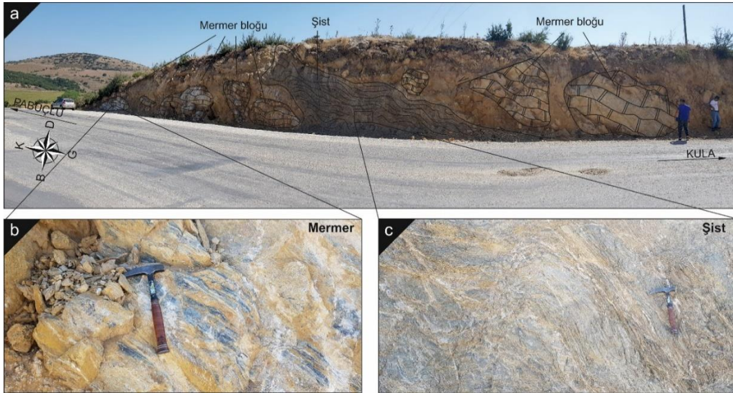
Şekil 5.5: Bölgede gözlenen şistlerin ve içerisinde gözlenen mermer bloklarının uzaktan ve yakından görünümü
