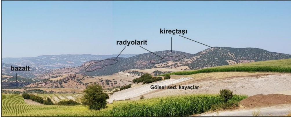
Şekil 5.7: İnceleme alanında Vezirler melanjı içerisinde gözlenen radyolarit-çört, kireçtaşı blokları, hemen üzerinde uyumsuz gölgesel sedimanter kayalar ve bu kayalar üzerinde gözlenen bazaltların görünümü
