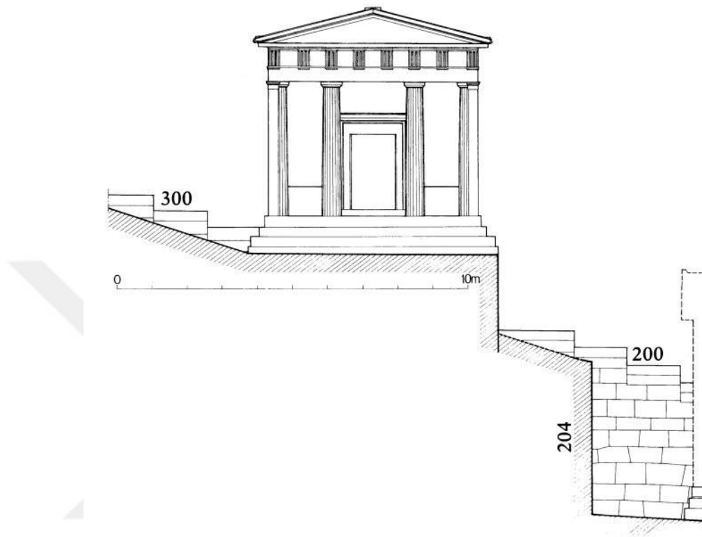
Görsel 77: Kyrene (XIV) thesauros. Bommelaer and Laroche, 1991, s. 156, fig. 62.
