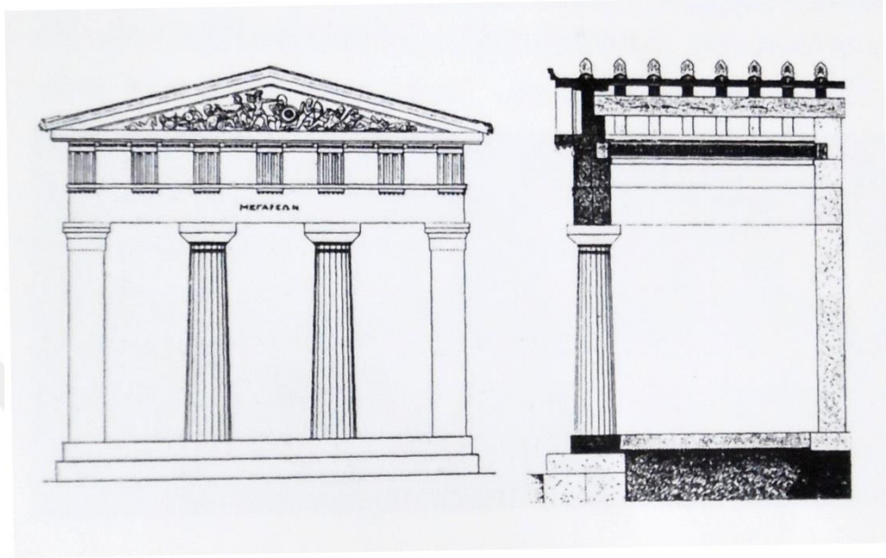
Görsel 42: Megara thesauros önden görünüm ve kesit çizimi.
