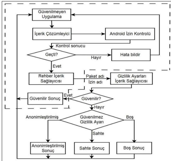
Şekil 3.19. TISSA sisteminin çalışma mantığı [77]
