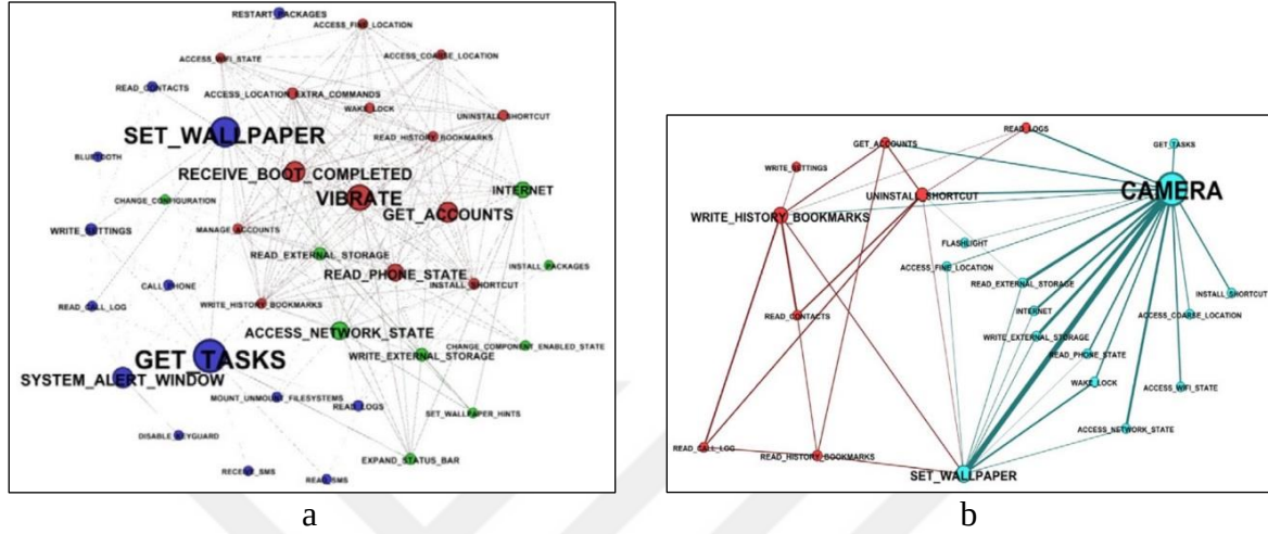
Şekil 3.10. a) Kişiselleştirme kategorisinin izin modeli b) Fotoğrafçılık kategorisinin izin modeli [66]
