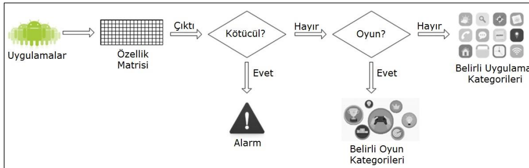
Şekil 3.12. Wang ve diğerlerinin geliştirdiği sistemin akış şeması [68]
