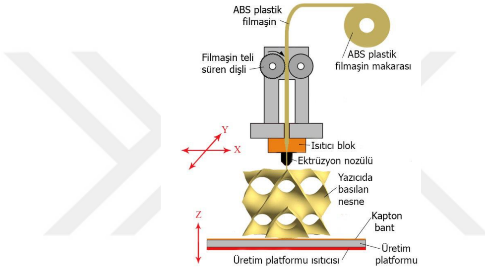
Şekil 2.2: FDM teknolojili üç boyutlu yazıcı (Gür, 2017).
