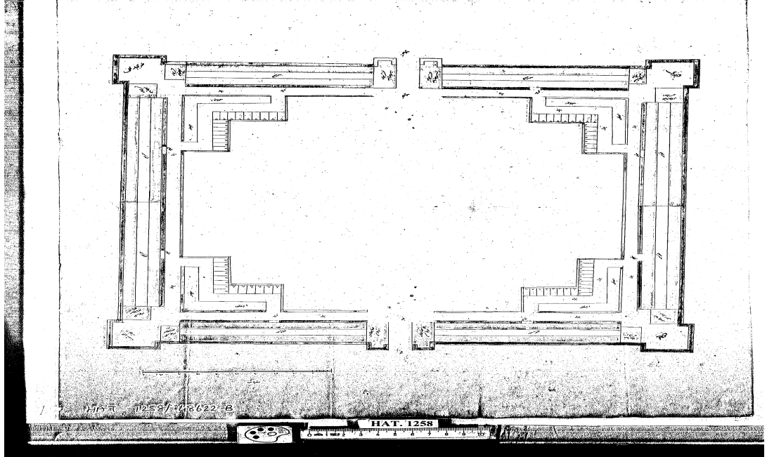
Şekil 2;17 Ankara Redif Kışlası Ana Bina Planı. 250
