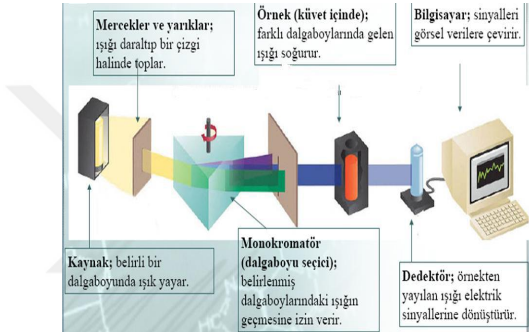
Şekil 2.14. UV-GB spektrofotometresinin şematik gösterimi (Arge ve Kalite [Internet]. 2014 [04.02.2020]. Erişim adresi: http://kalitece1.blogspot.com/2014/10/kromotografik-ve-spektroskopik_30.html ).
