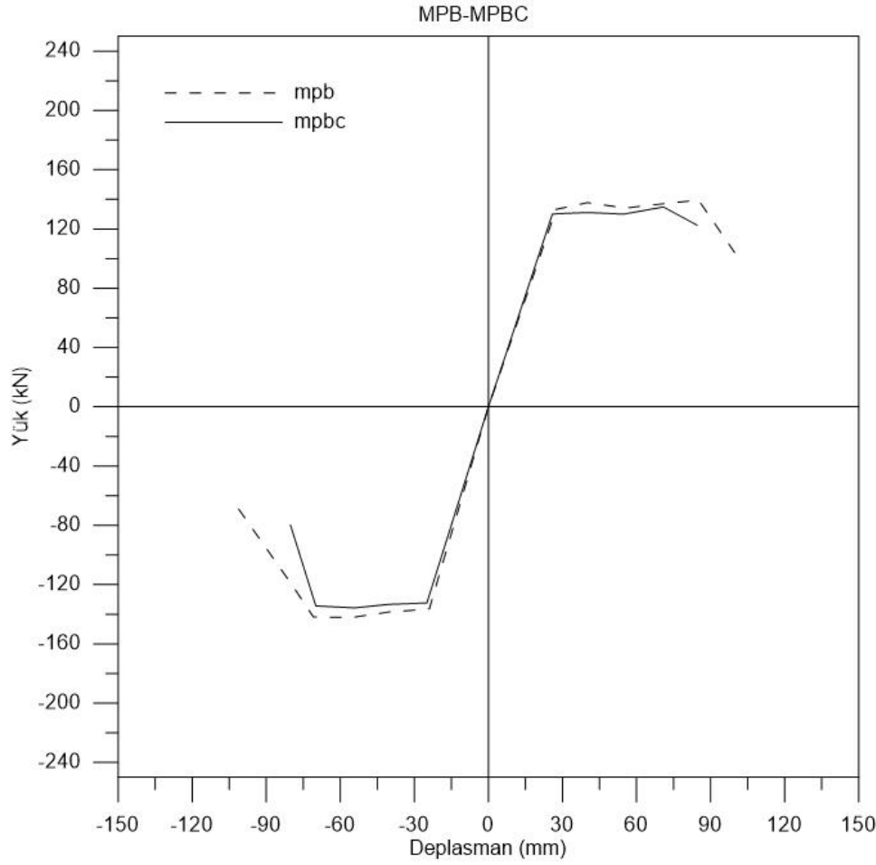
Şekil 5.10. MPB-MPBC zarf eğrileri karşılaştırması
