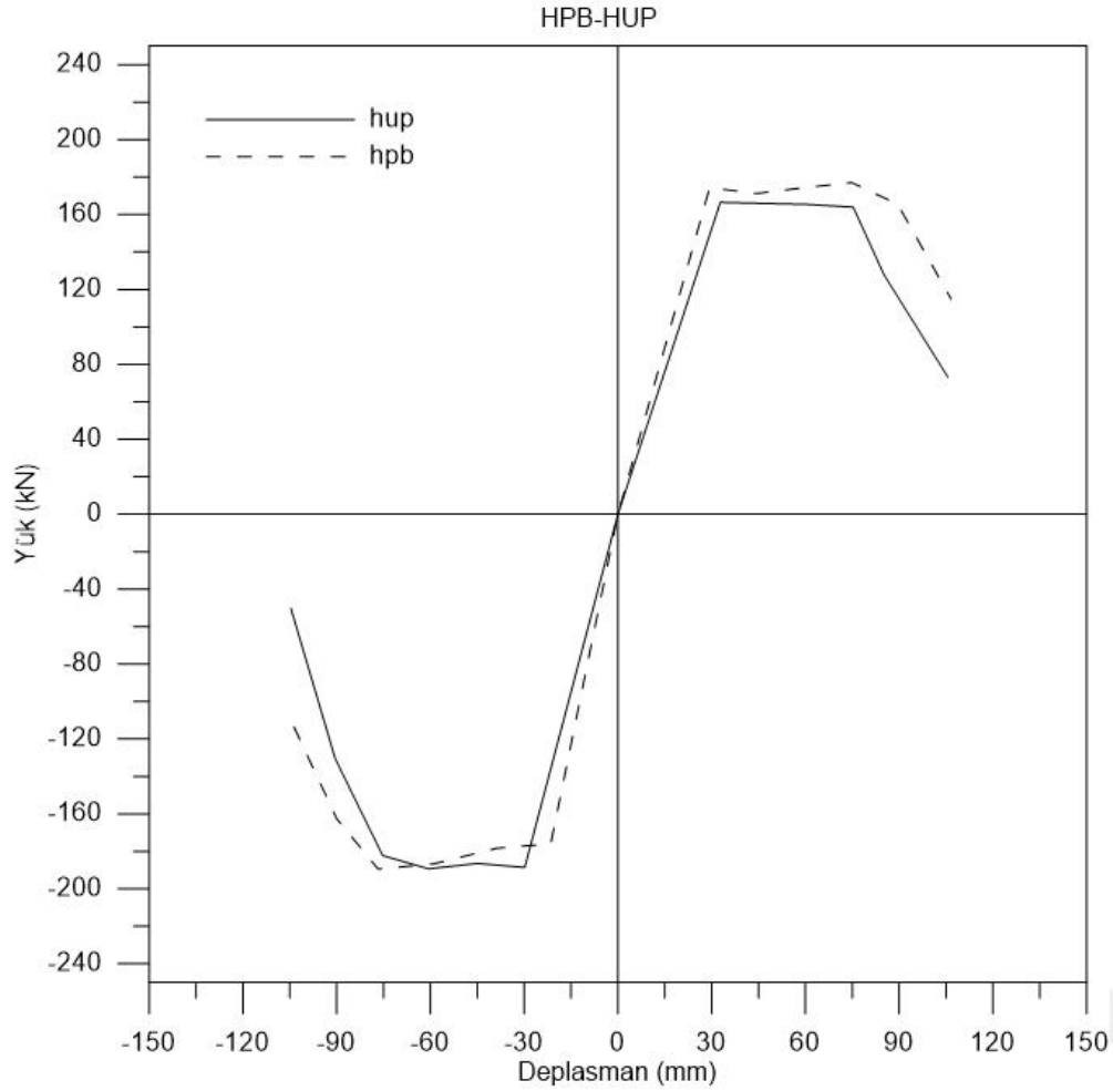
Şekil 5.24. HUP-HPB zarf eğrileri karşılaştırması
