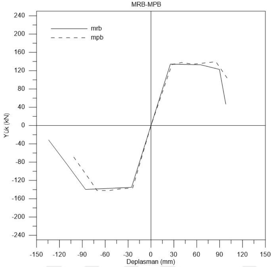
Şekil 5.3. MRB-MPB zarf eğrileri karşılaştırması
