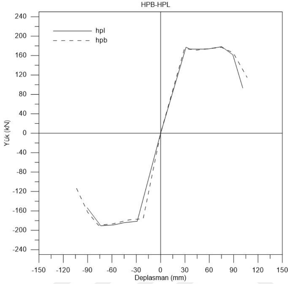
Şekil 5.20. HPB-HPL zarf eğrileri karşılaştırması
