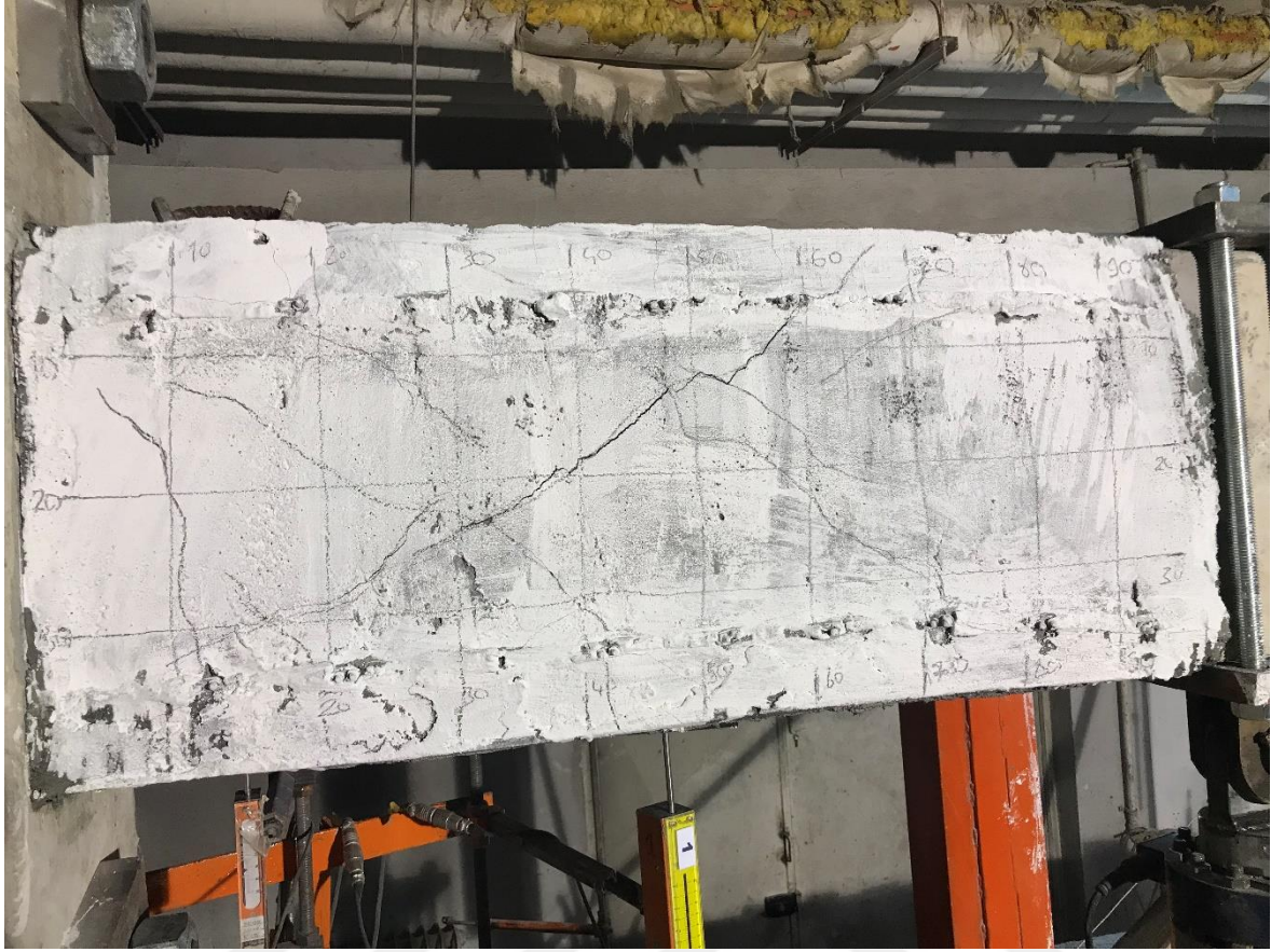
Resim 4.18. HPL numunesi 1. çevrim sonu çatlak görüntüsü
