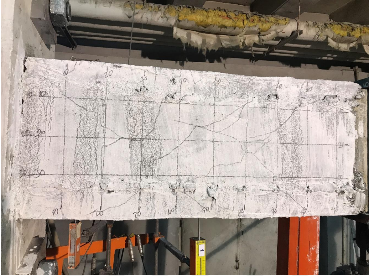
Resim 4.11. MPLC numunesi 1. çevrim sonu çatlak düzeni
