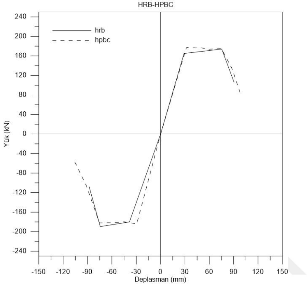
Şekil 5.17. HRB-HPBC zarf eğrileri karşılaştırması
