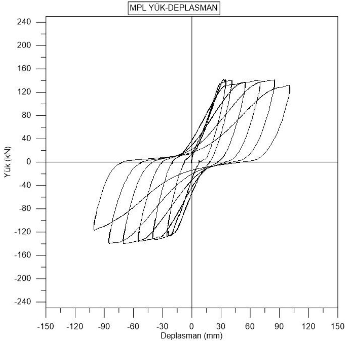
Şekil 4.11. MPL numunesi yük-deplasman grafiğı
