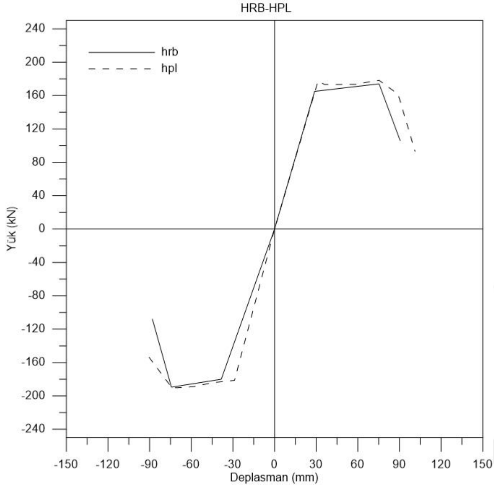
Şekil 5.16. HRB-HPL zarf eğrileri karşılaştırması
