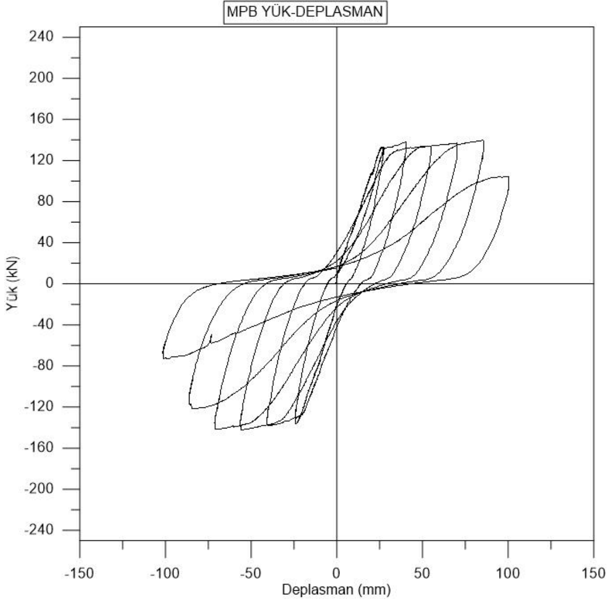
Şekil 4.10. MPB numunesi yük-deplasman grafiği
