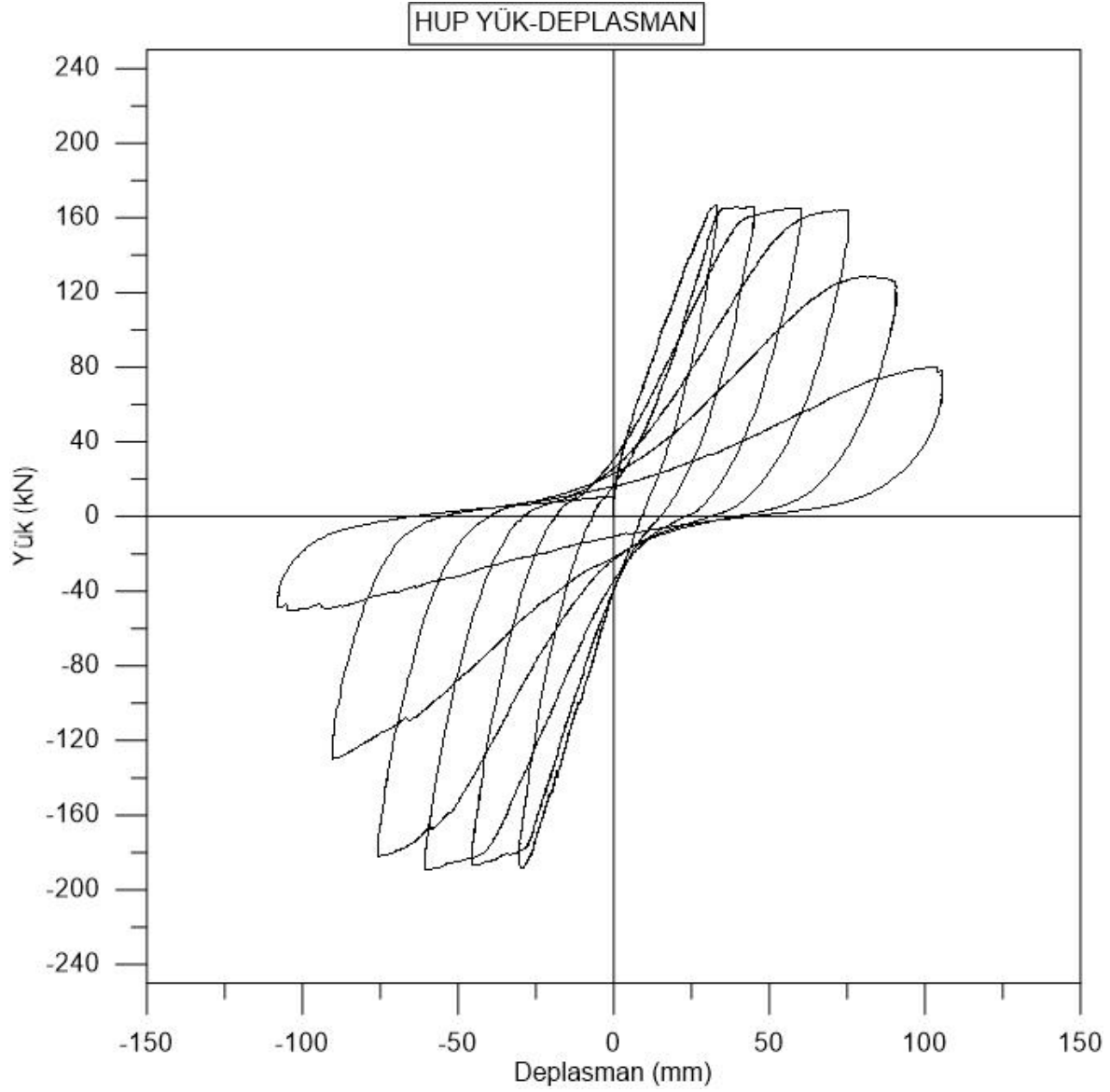
Şekil 4.15. HUP numunesi yük-deplasman grafiği
