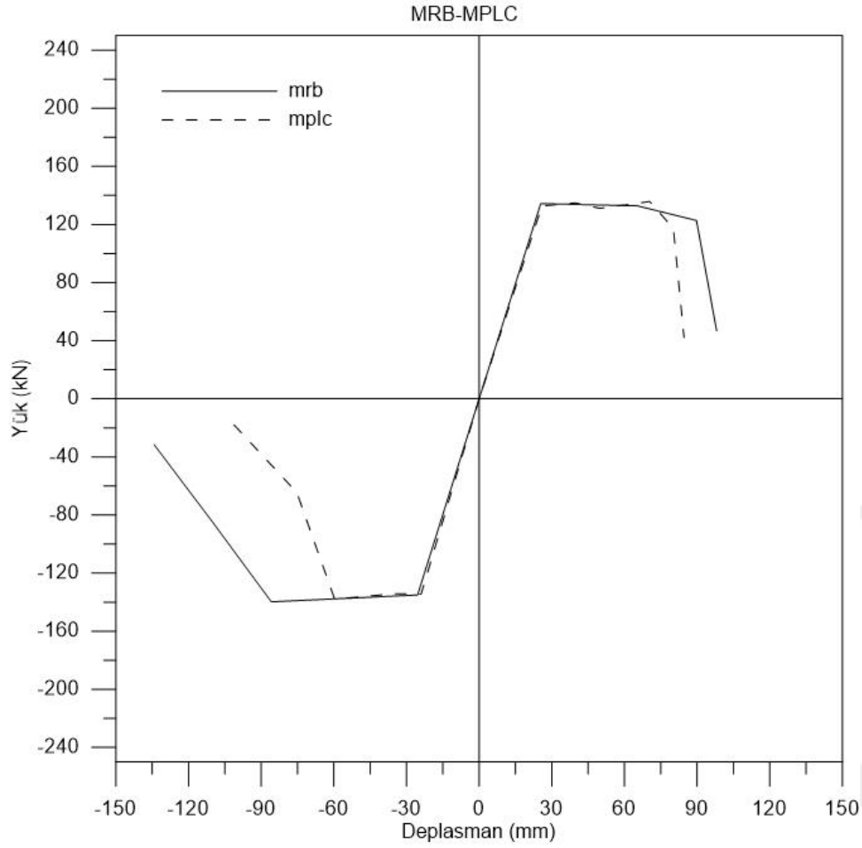
Şekil 5.6. MRB-MPLC zarf eğrileri karşılaştırması
