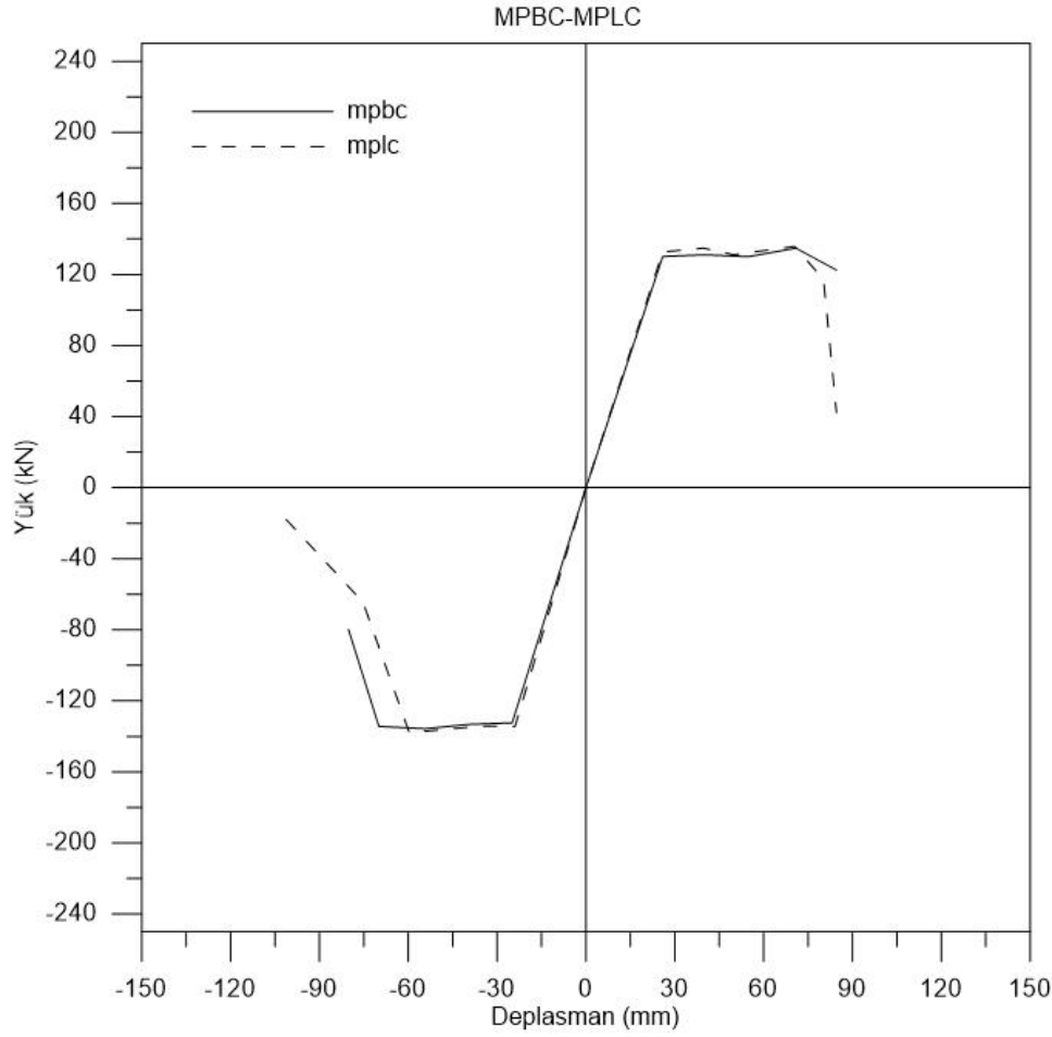
Şekil 5.9. MPBC-MPLC zarf eğrileri karşılaştırması
