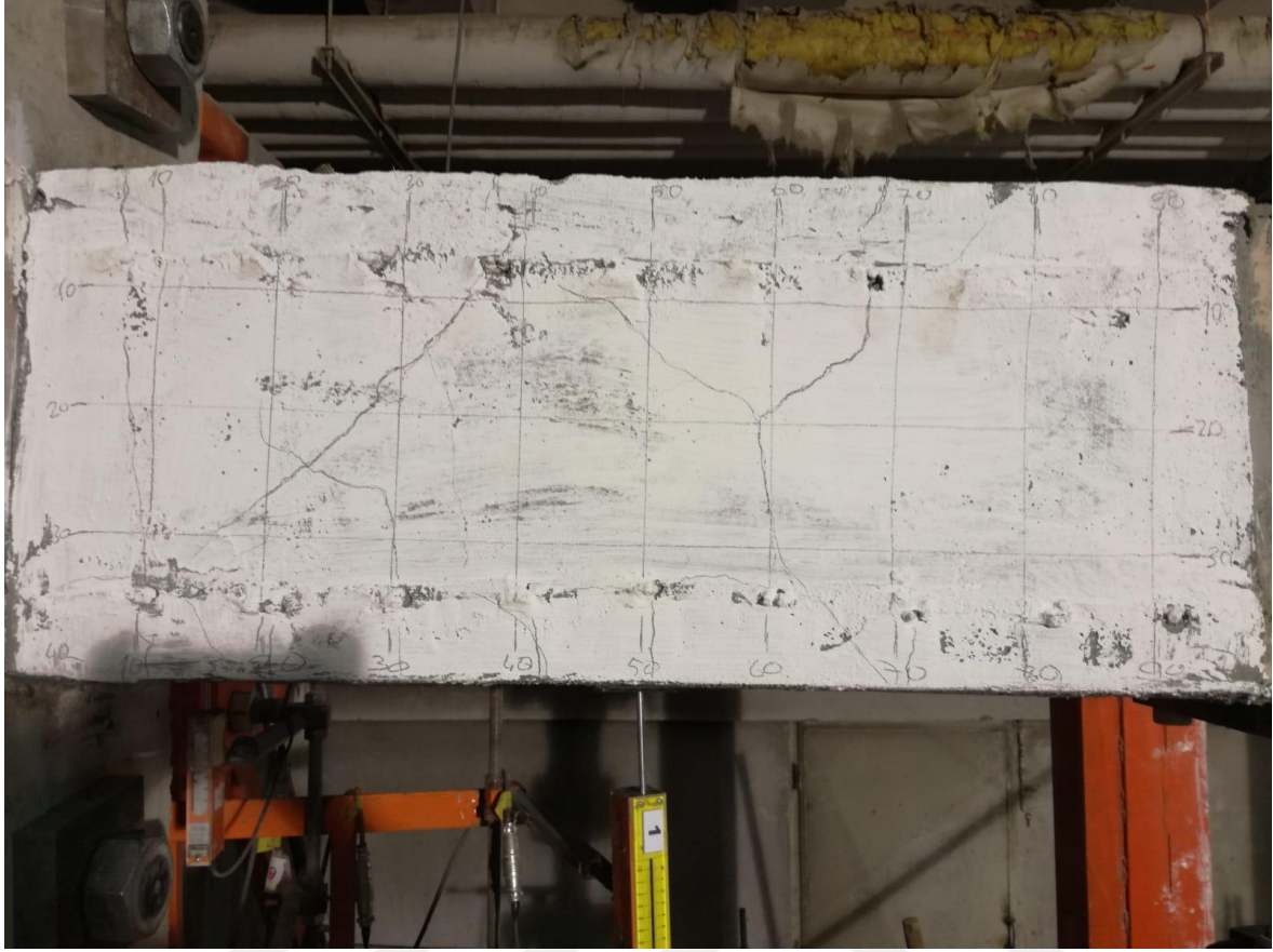
Resim 4.7. Kelepçe hizası boyunca uzanan çatlaklar
