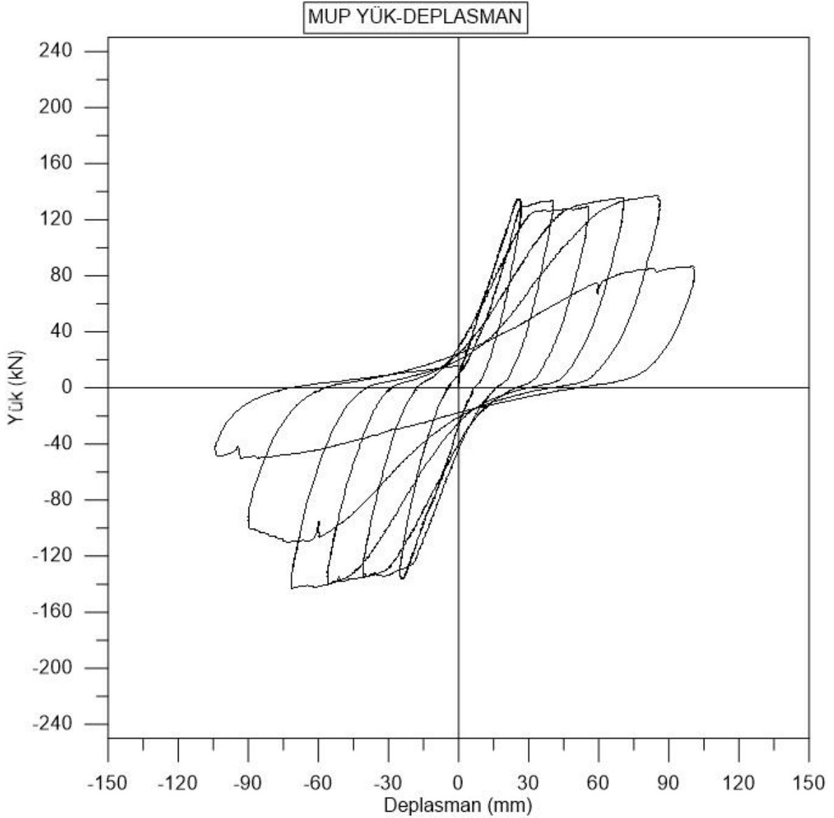
Şekil 4.9. MUP numunesi yük deplasman grafiği
