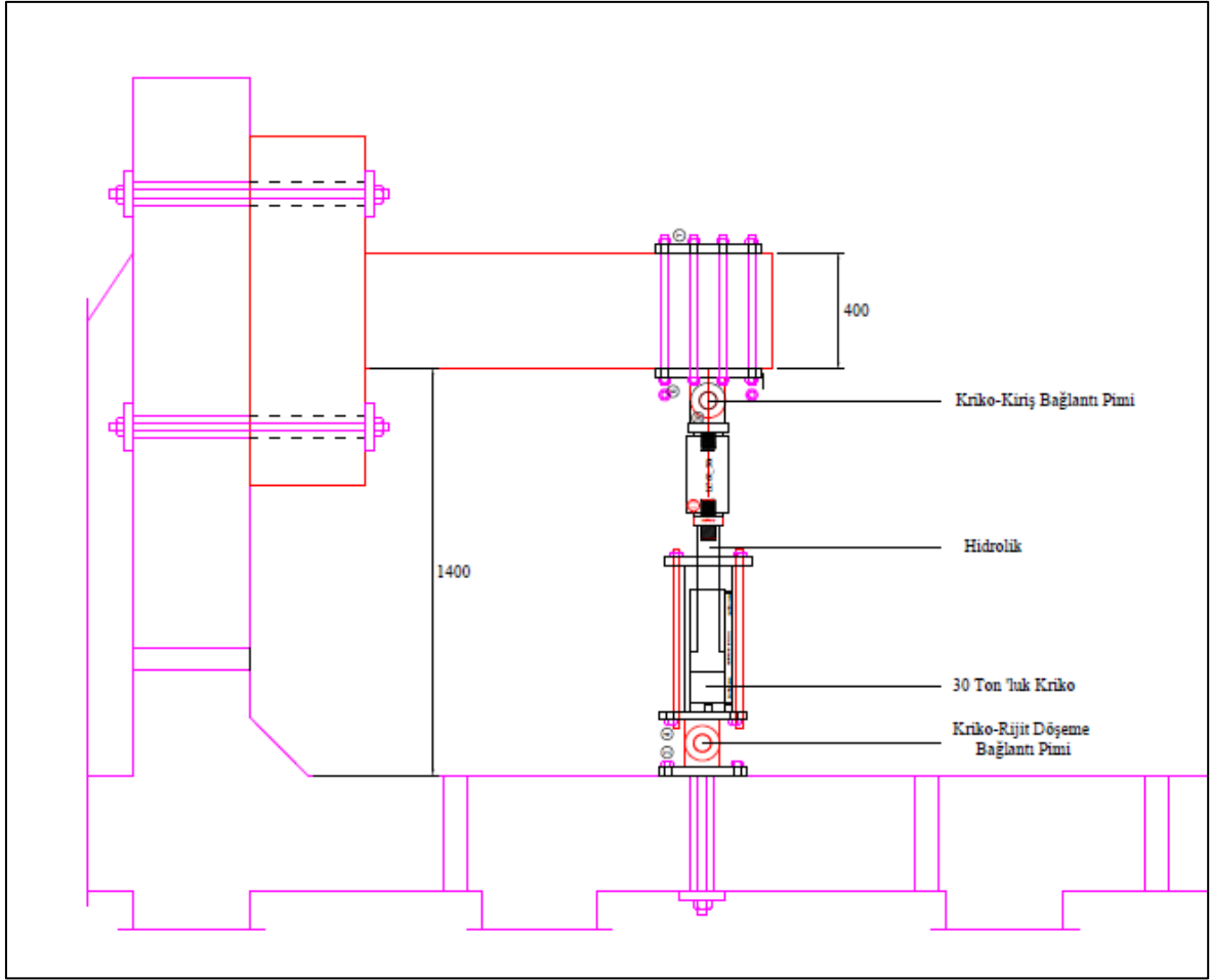
Şekil 4.6. Yükleme düzeni
