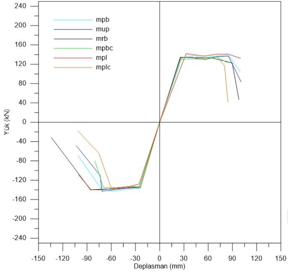
Şekil 5.1. MRB-MUP-MPB-MPBC-MPL-MPLC zarf eğrileri karşılaştırması
