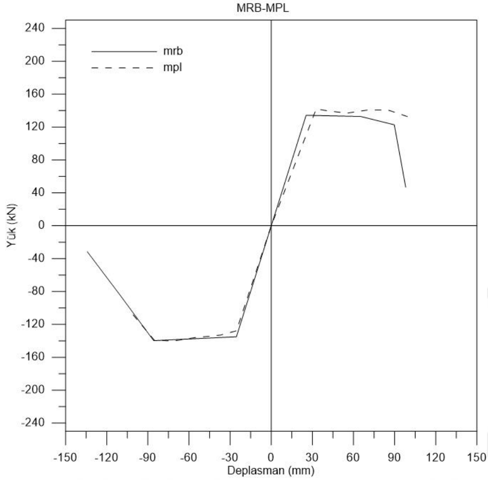
Şekil 5.4. MRB-MPL zarf eğrileri karşılaştırması
