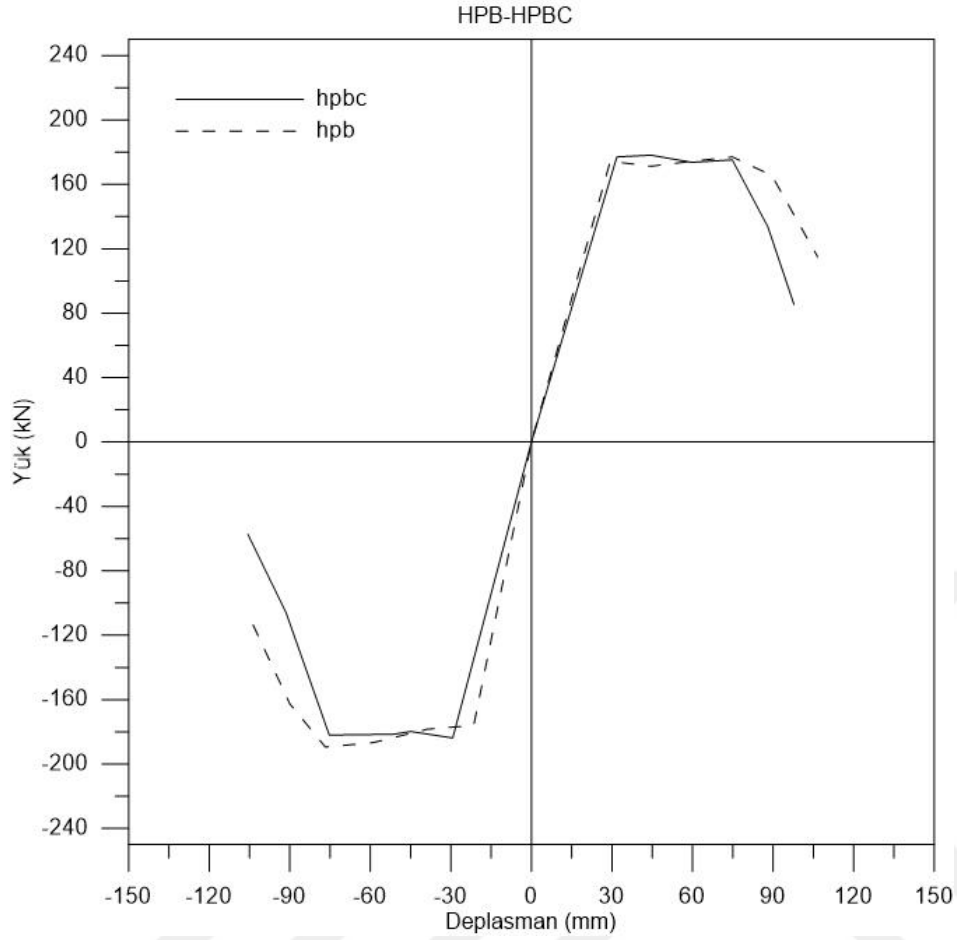
Şekil 5.22. HPB-HPBC zarf eğrileri karşılaştırması
