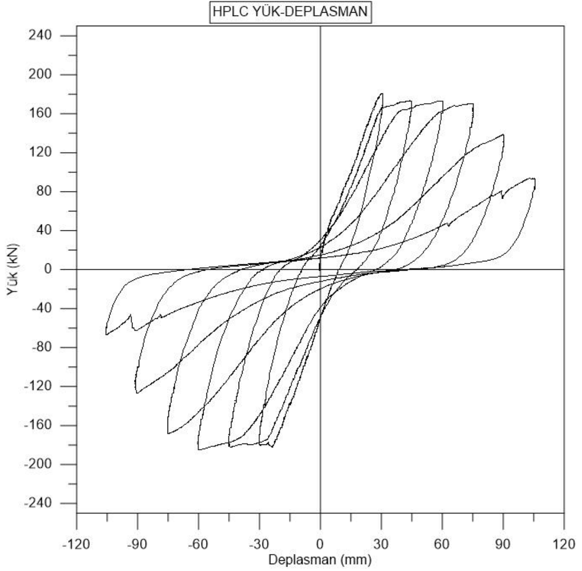
Şekil 4.19. HPLC numunesi yük-deplasman grafiği
