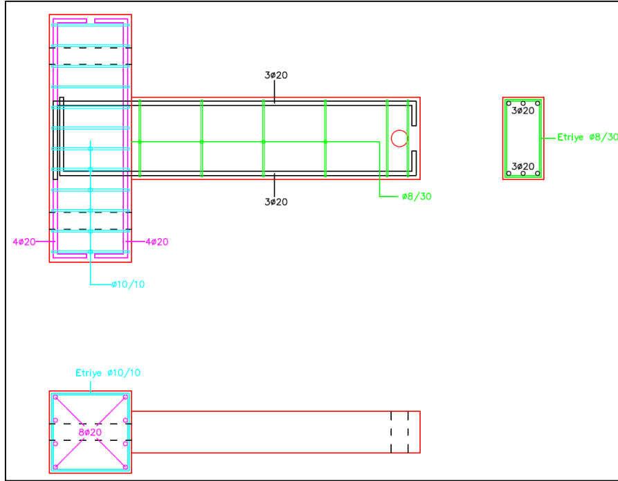
Şekil 4.3. Az donatılı güçlendirilecek deney elemanları
