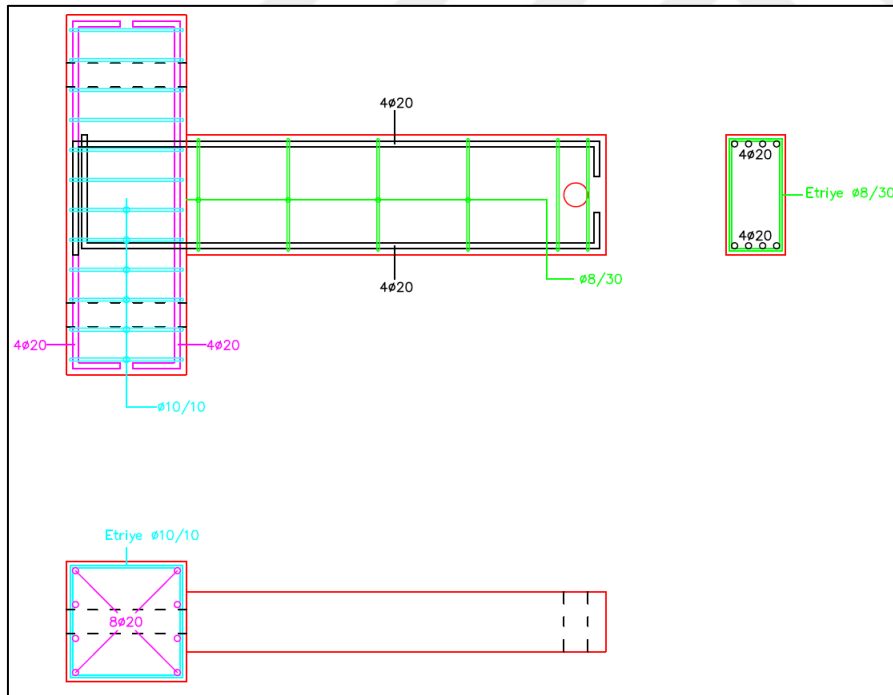
Şekil 4.4. Çok donatılı güçlendirilecek deney elemanları
