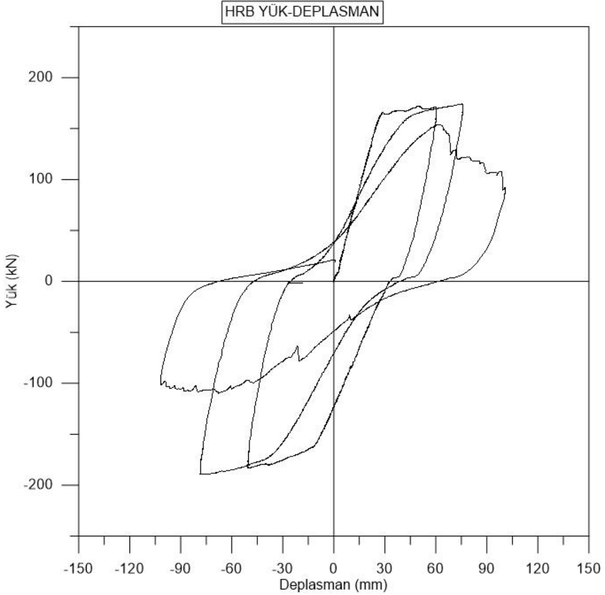
Şekil 4.14. HRB numunesi yük-deplasman grafiği
