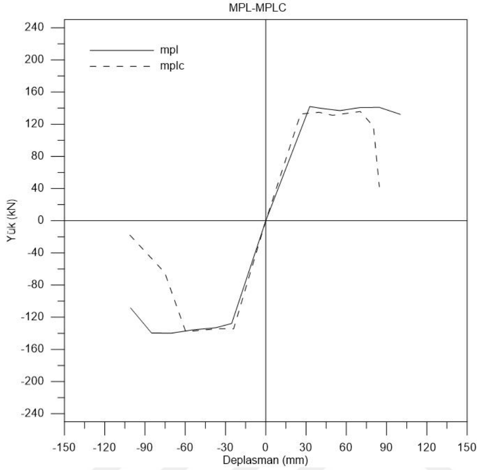
Şekil 5.11. MPL-MPLC zarf eğrileri karşılaştırması
