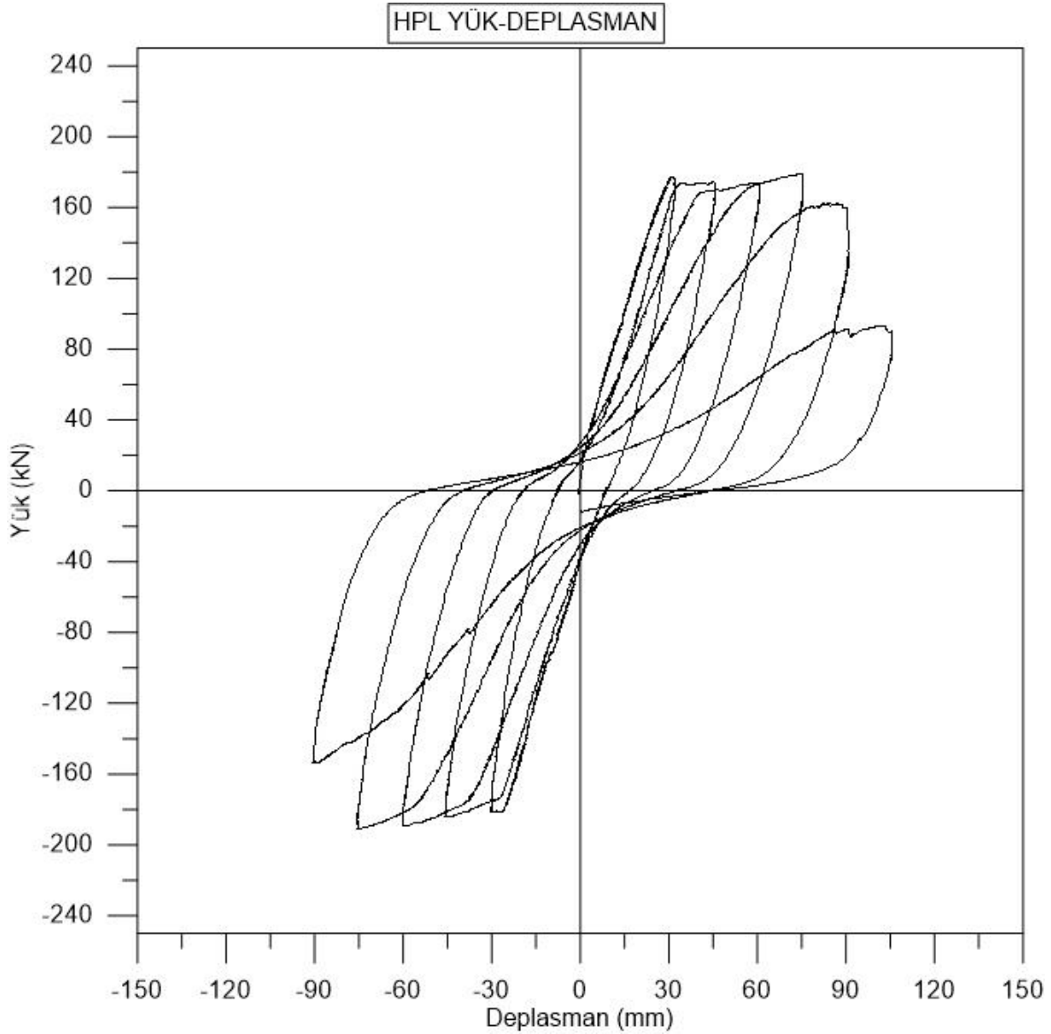
Şekil 4.17. HPL numunesi yük-deplasman ilişkisi
