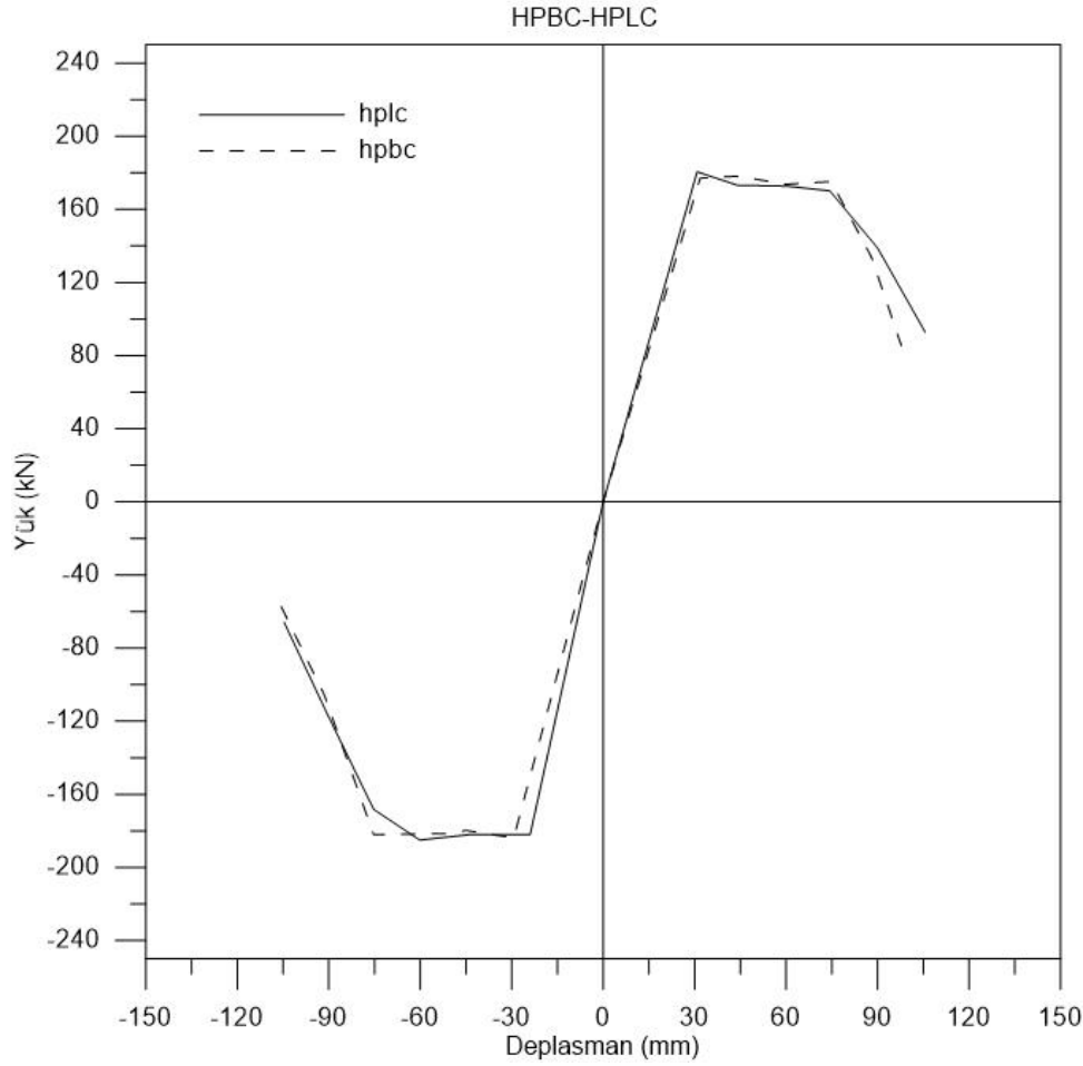
Şekil 5.21. HPBC-HPLC zarf eğrileri karşılaştırması
