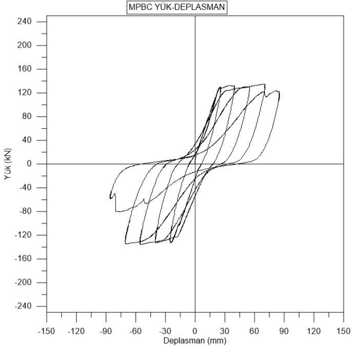
Şekil 4.12. MPBC numunesi yük-deplasman grafiği
