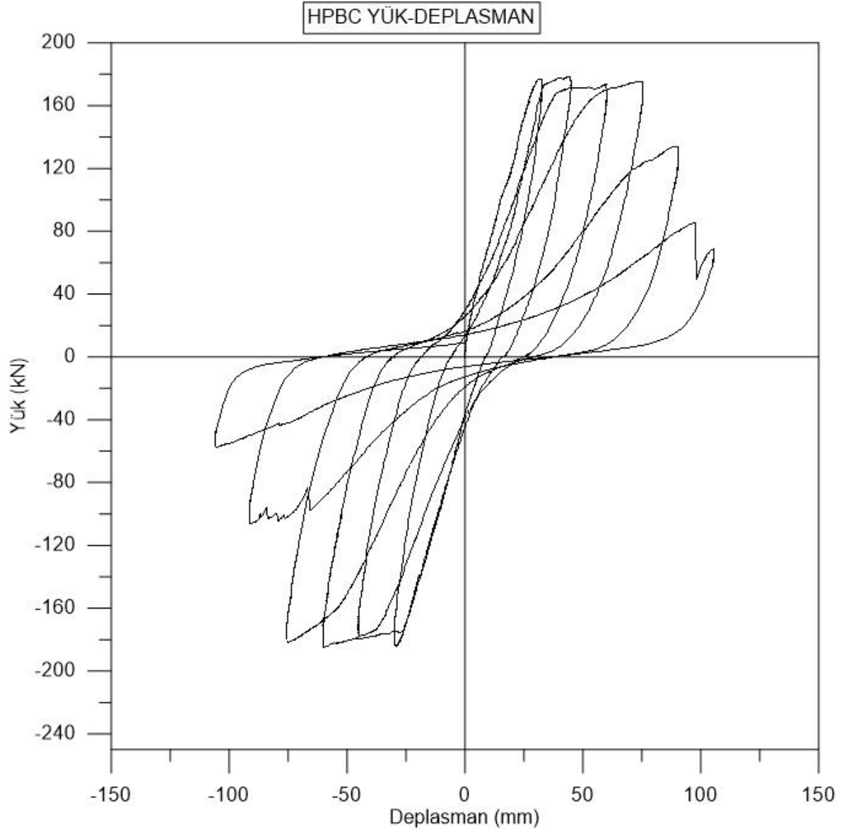
Şekil 4.18. HPBC numune yük-deplasman grafiği
