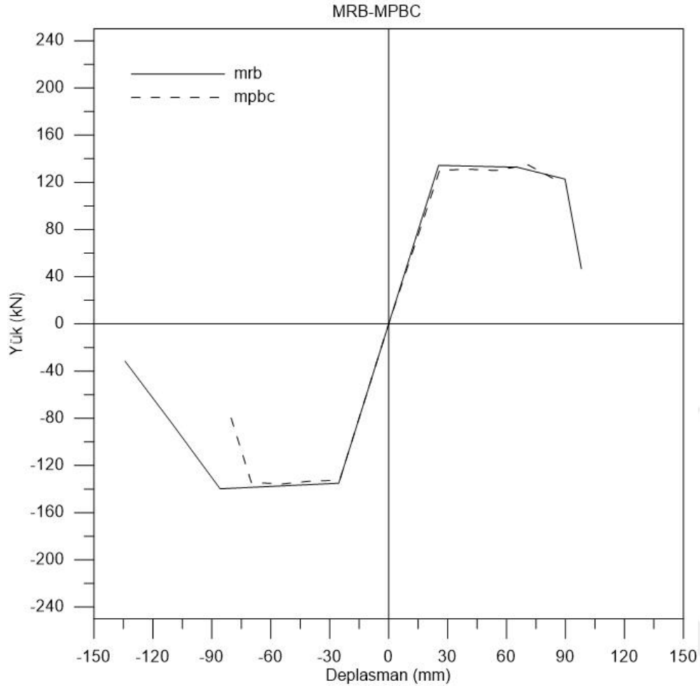
Şekil 5.5. MRB-MPBC zarf eğrileri karşılaştırması
