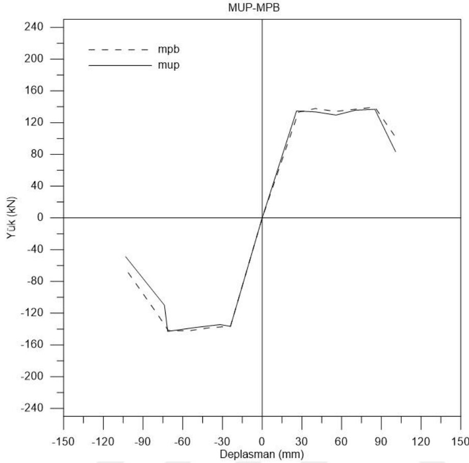
Şekil 5.12. MUP-MPB zarf eğrileri karşılaştırması
