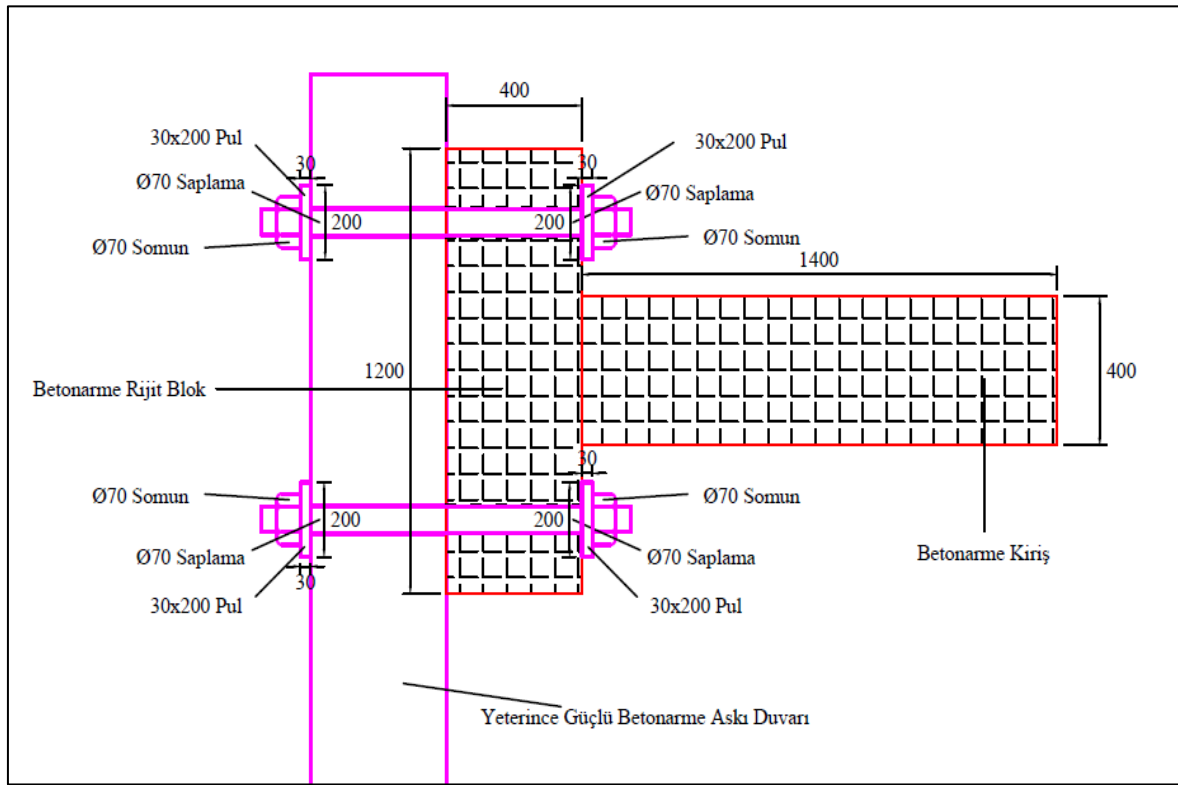
Şekil 4.5. Betonarme kirişin güçlü duvara tutturulduğu sistem
