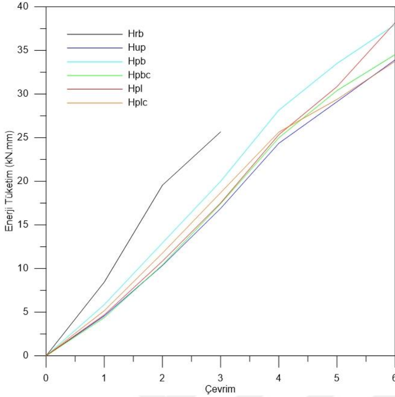
Şekil 5.26. Çok donatılı numunelerin enerji tüketimleri
