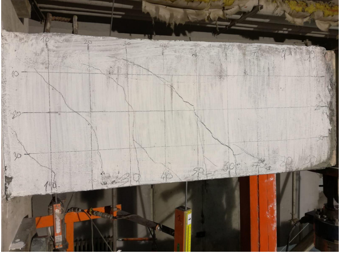
Resim 4.8. MPBC numunesi akma yüklemesi
