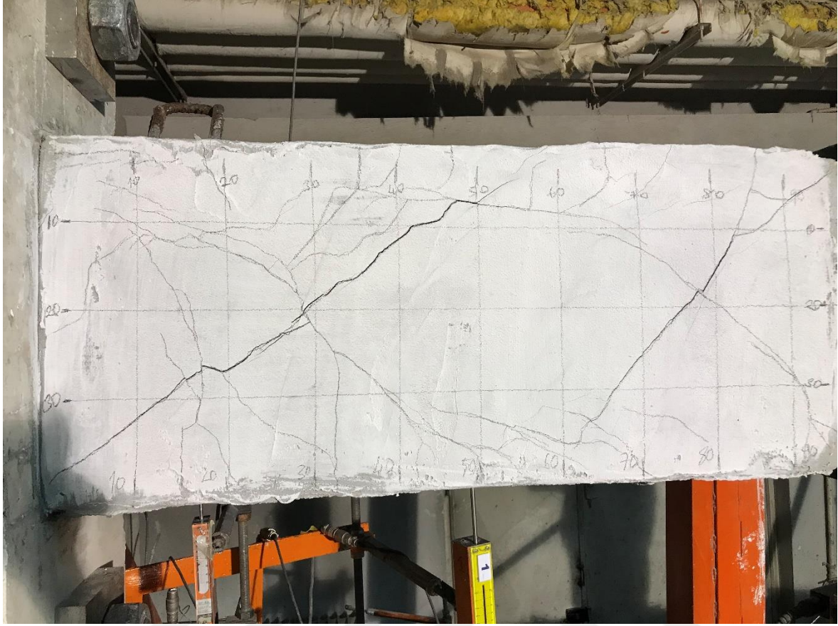
Resim 4.14. HUP numunesi 1. çevrim sonu çatlak düzeni
