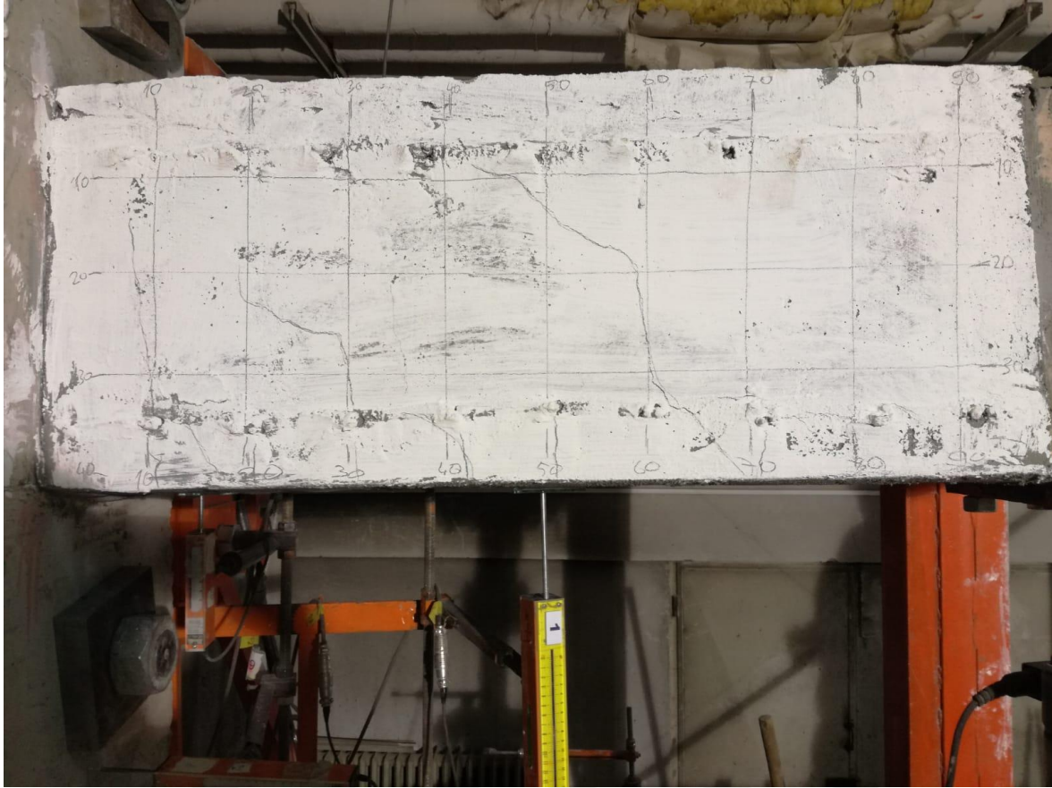
Resim 4.6. MPL numunesi akma yüklemesi
