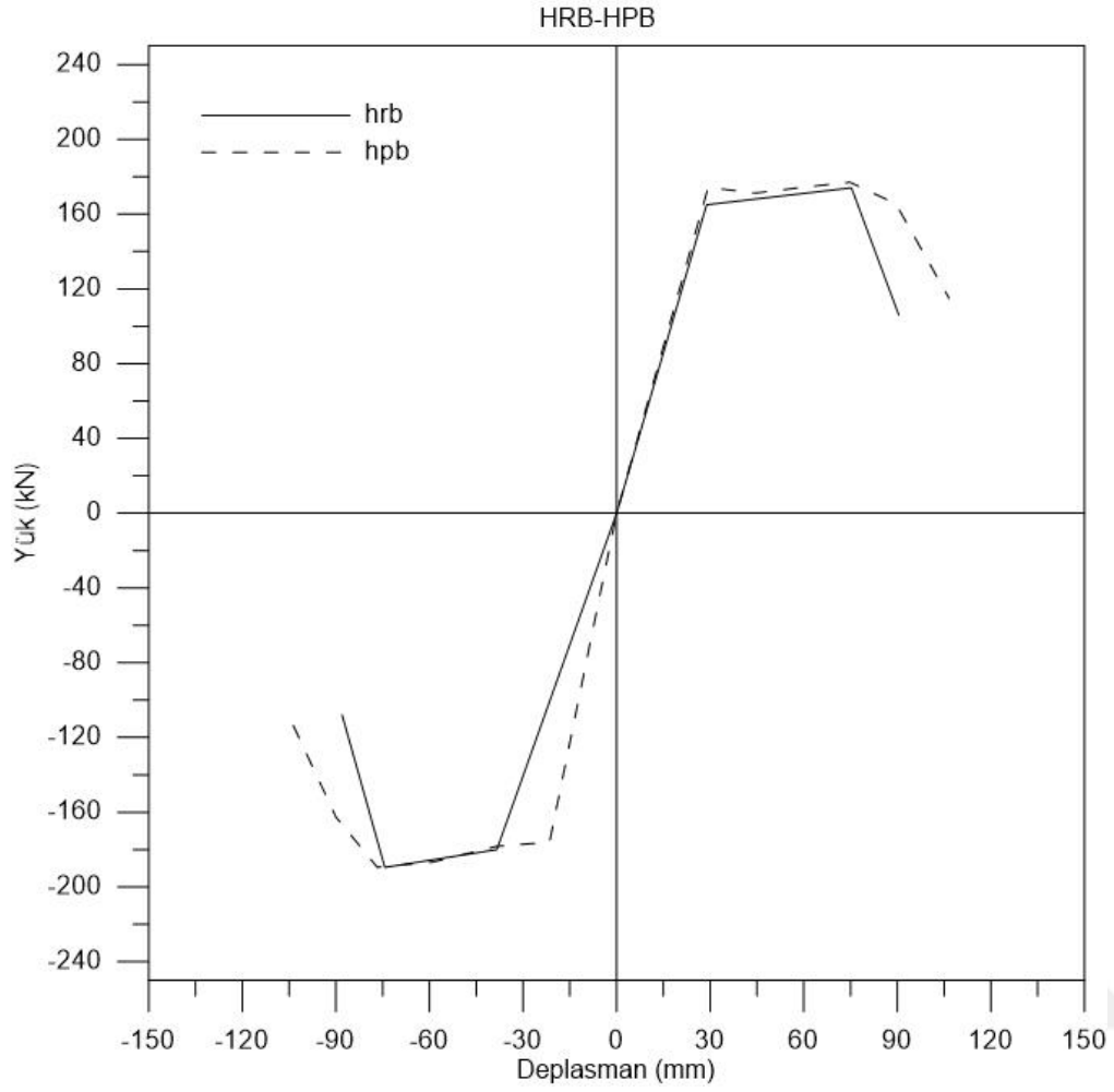
Şekil 5.15. HRB-HPB zarf eğrileri karşılaştırması
