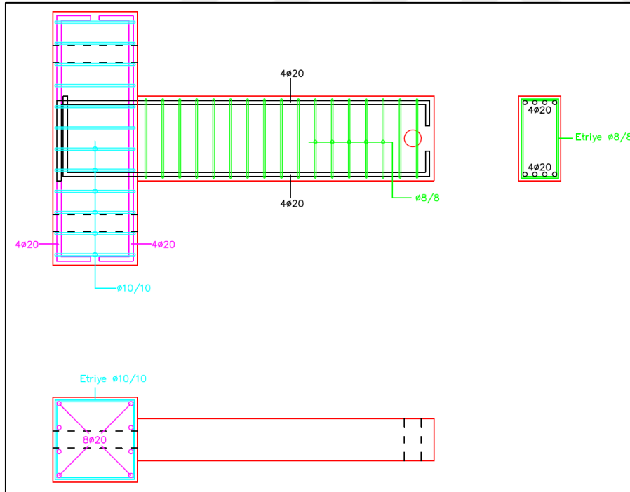
Şekil 4.2. HRB deney elemanı
