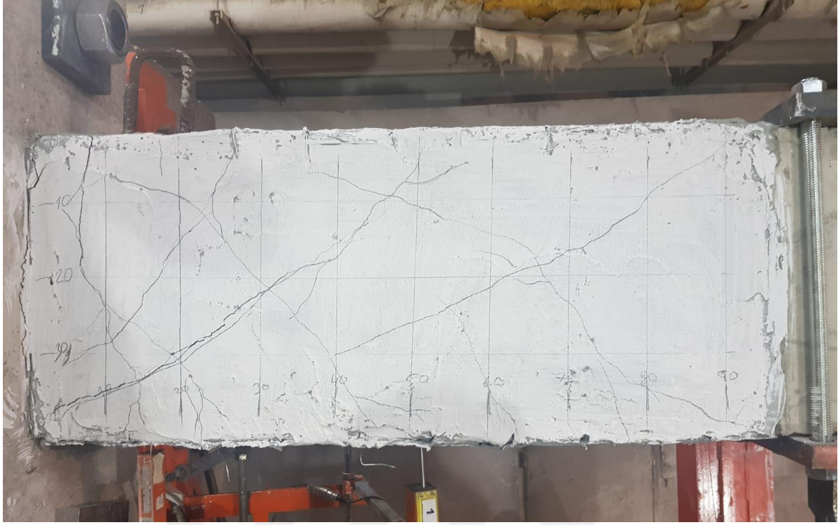
Resim 4.3. MUP numunesi 1. çevrim sonu çatlak görünümü
