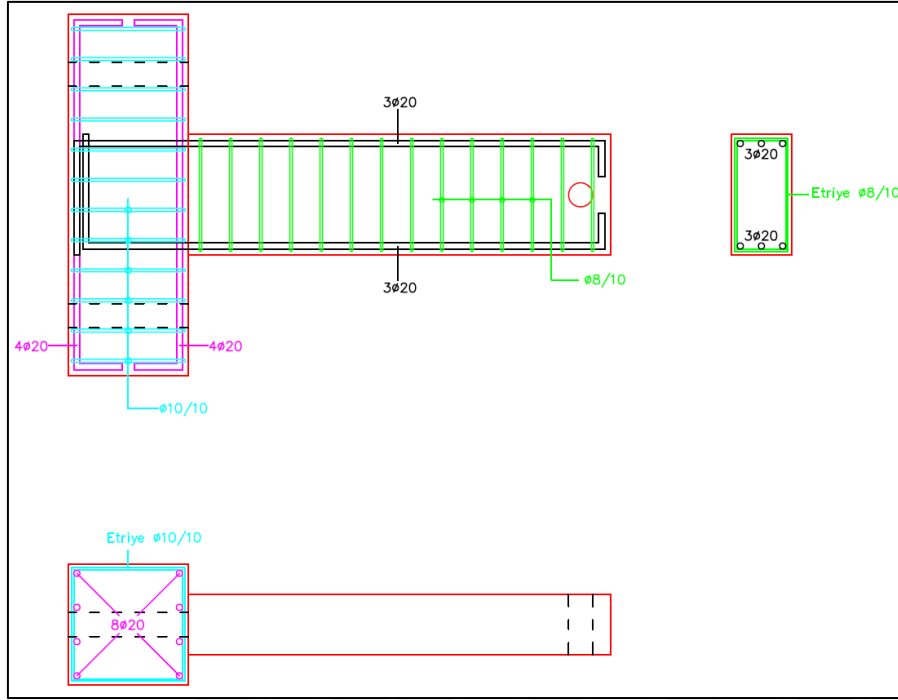
Şekil 4.1. MRB deney elemanı
