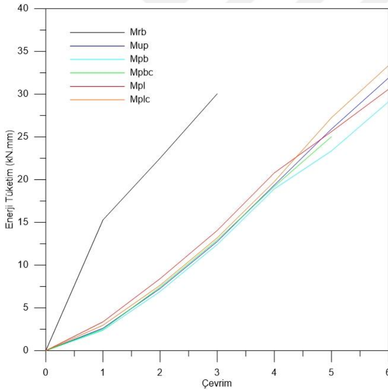
Şekil 5.25. Az donatılı numunelerin enerji tüketimleri
