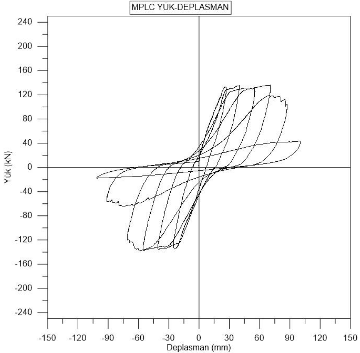
Şekil 4.13. MPLC numunesi yük-deplasman grafiği
