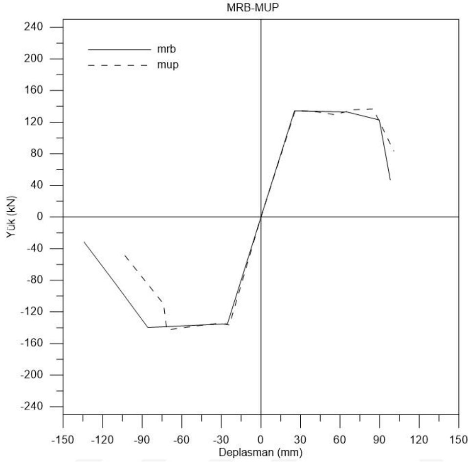
Şekil 5.2. MRB-MUP zarf eğrileri karşılaştırması
