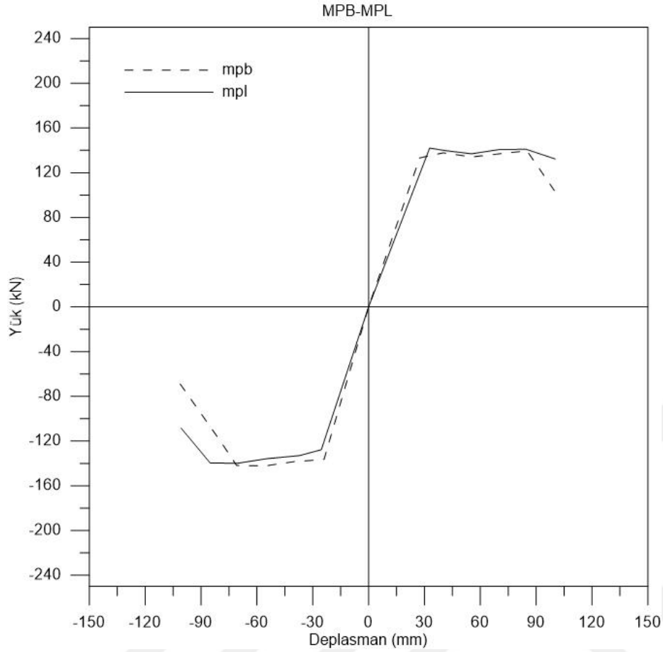
Şekil 5.8. MPB-MPL zarf eğrileri karşılaştırması
