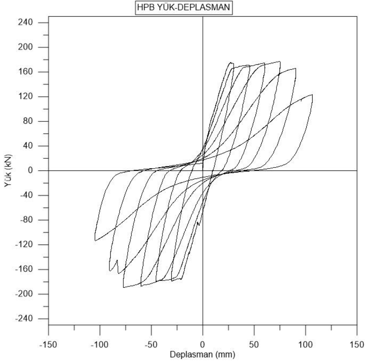
Şekil 4.16. HPB numunesi yük-deplasman grafiği
