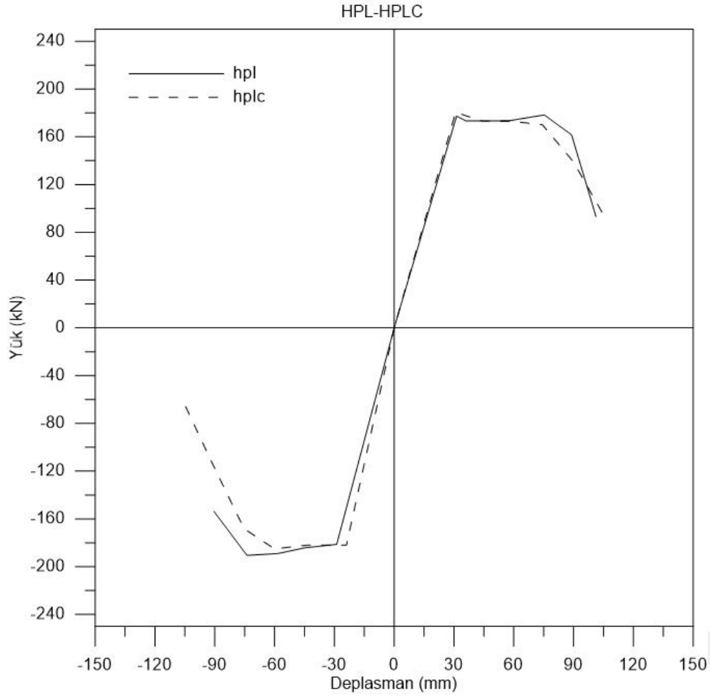
Şekil 5.23. HPL-HPLC zarf eğrileri karşılaştırması
