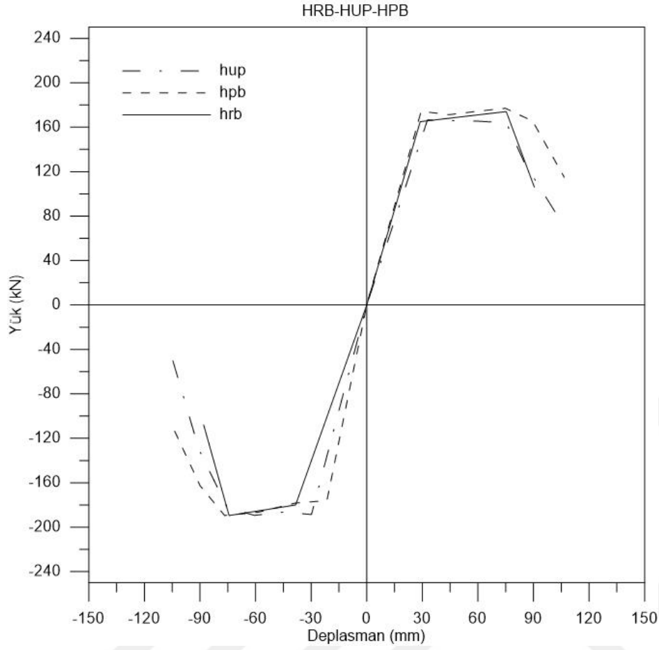
Şekil 5.19. HRB-HUP-HPB zarf eğrileri karşılaştırması
