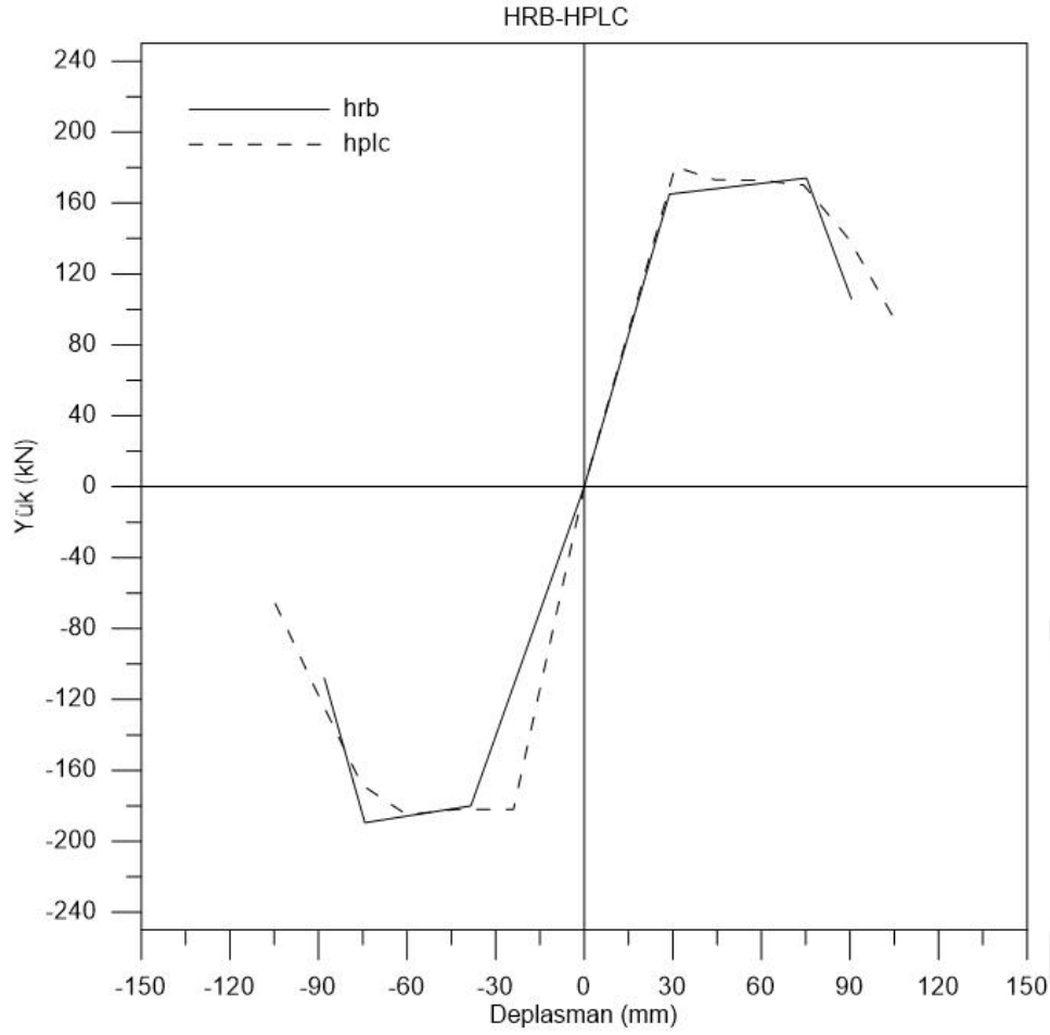
Şekil 5.18. HRB-HPLC zarf eğrileri karşılaştırması
