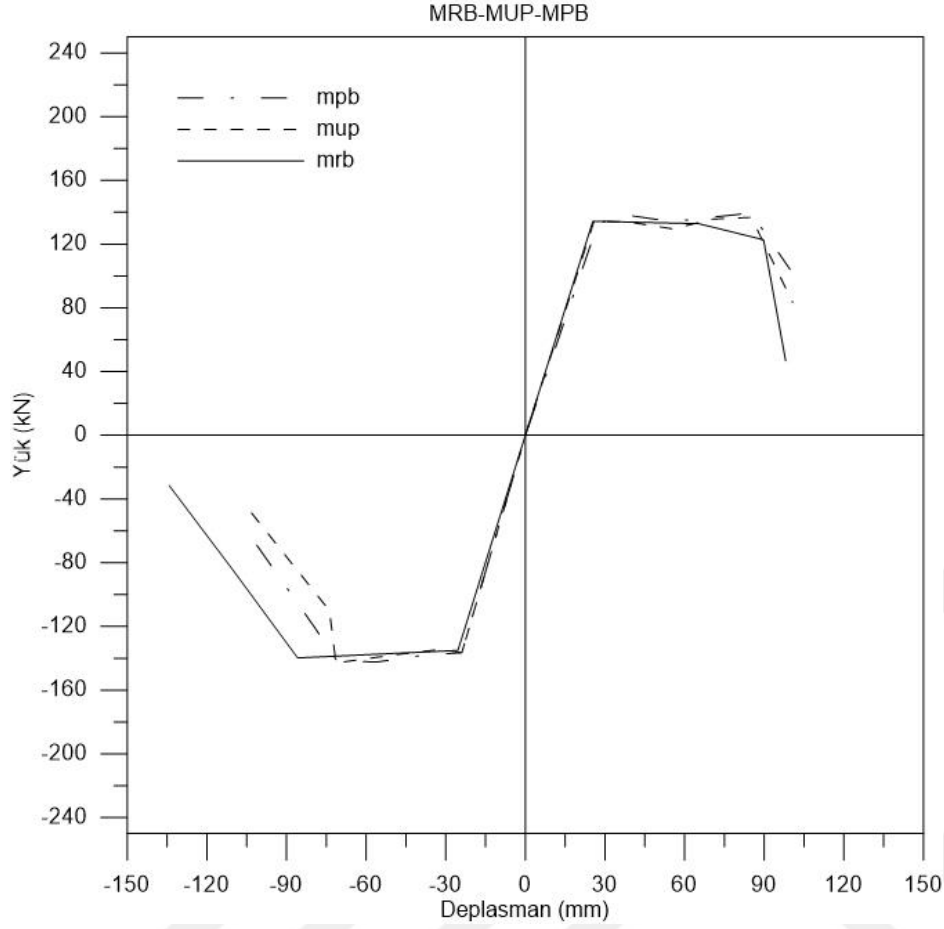
Şekil 5.7. MRB-MPB-MUP zarf eğrileri karşılaştırması
