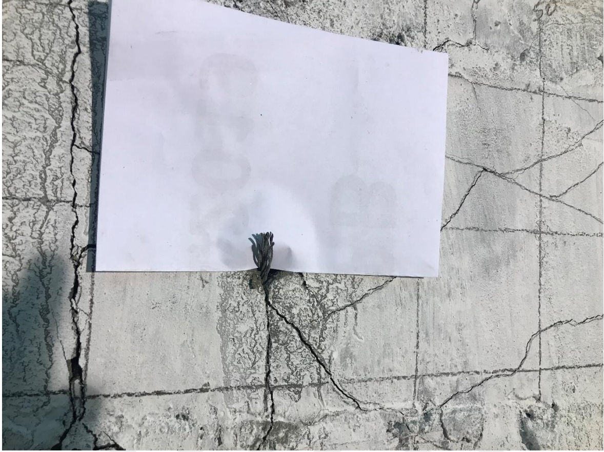
Resim 4.12. MPLC numunesi kablo kesimi
