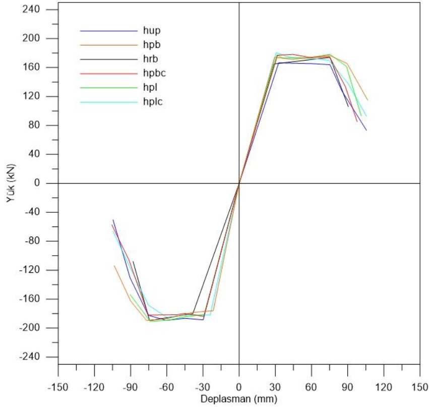
Şekil 5.13. HRB-HUP-HPB-HPBC-HPL-HPLC zarf eğrileri karşılaştırması
