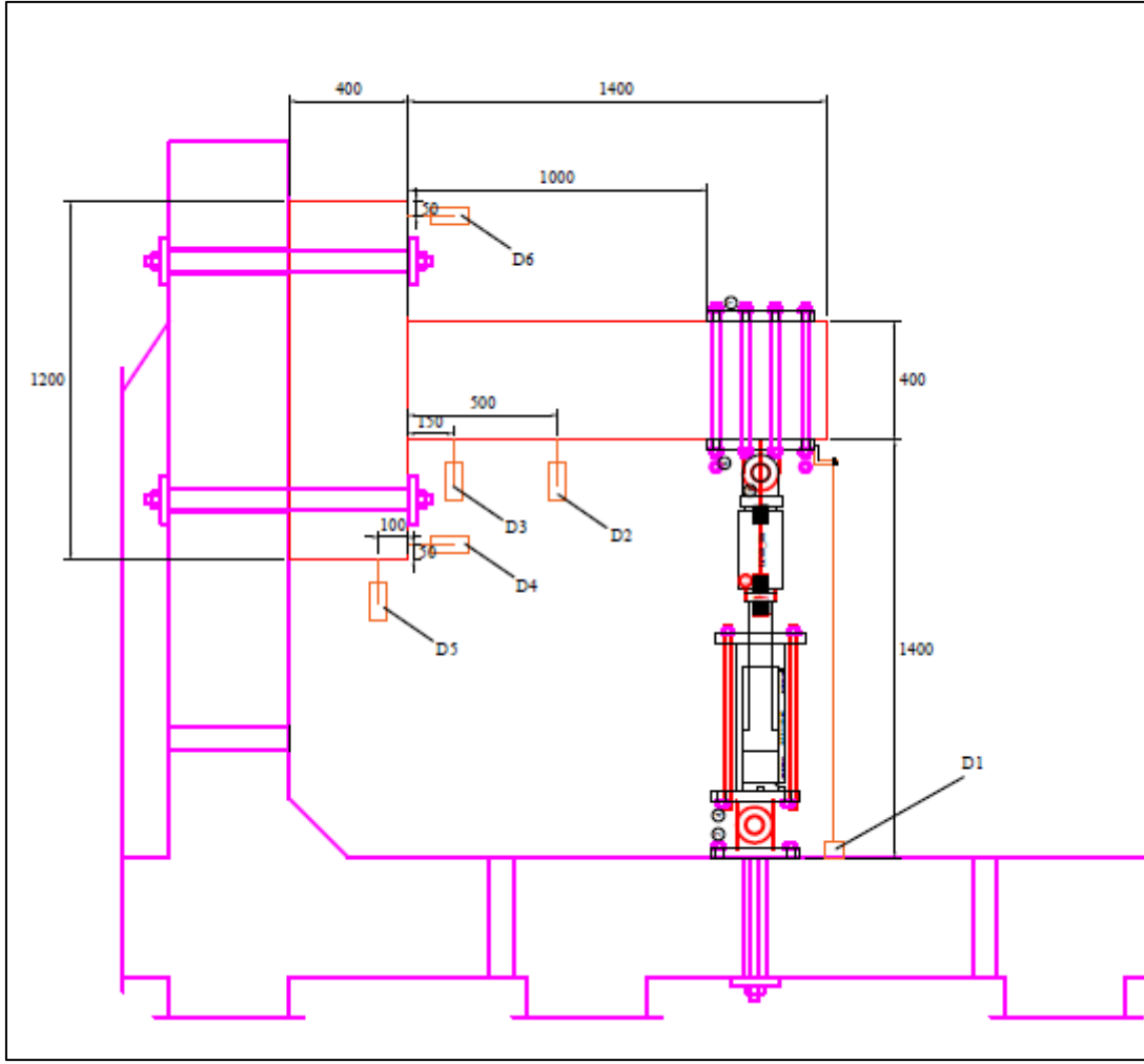
Şekil 4.7. Ölçüm düzeni
