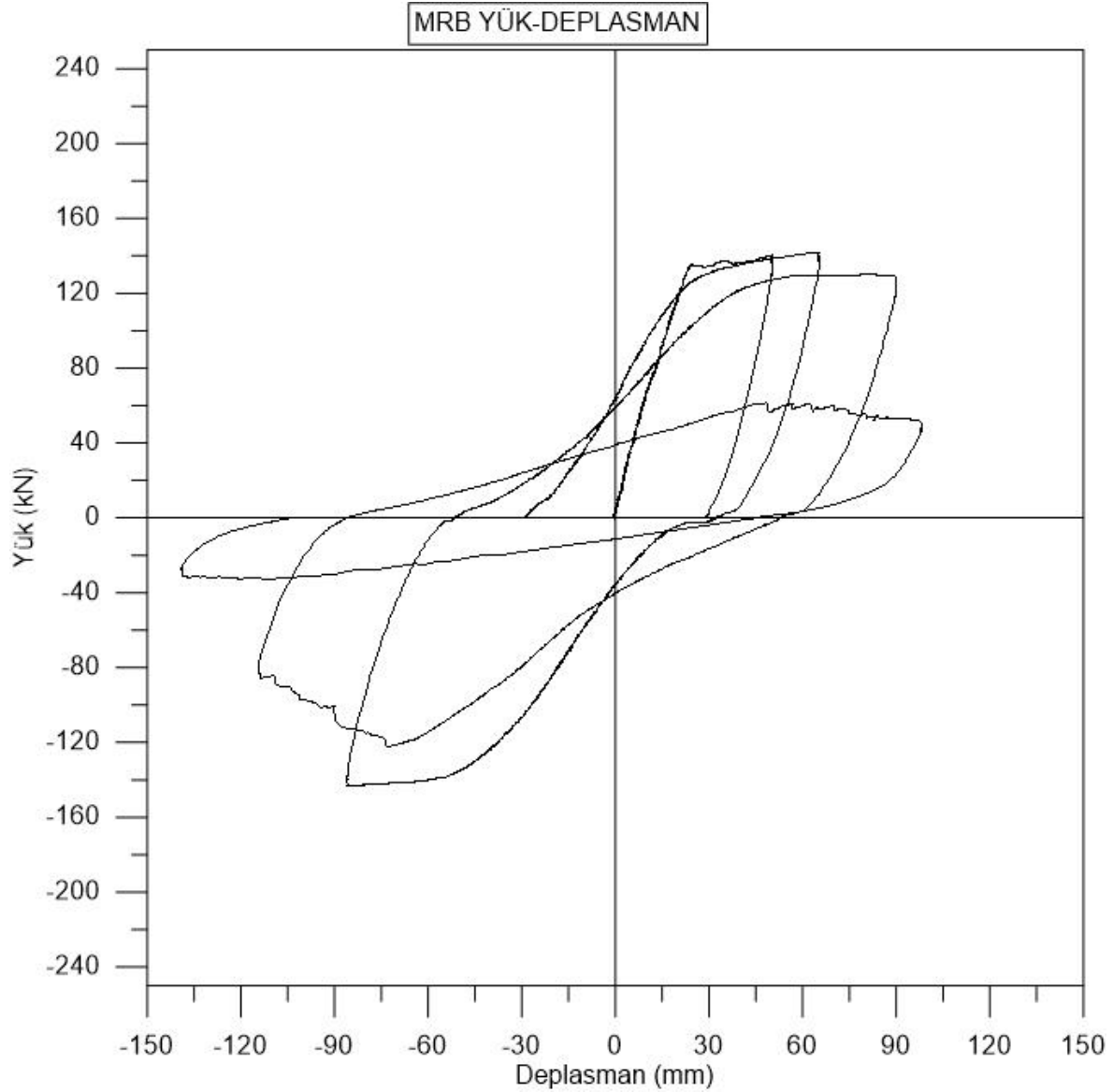
Şekil 4.8. MRB numunesi yük-deplasman grafiği
