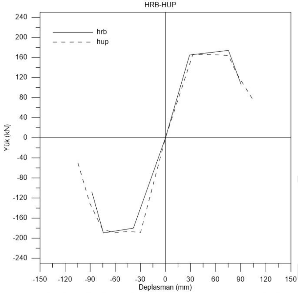
Şekil 5.14. HRB-HUP zarf eğrileri karşılaştırması
