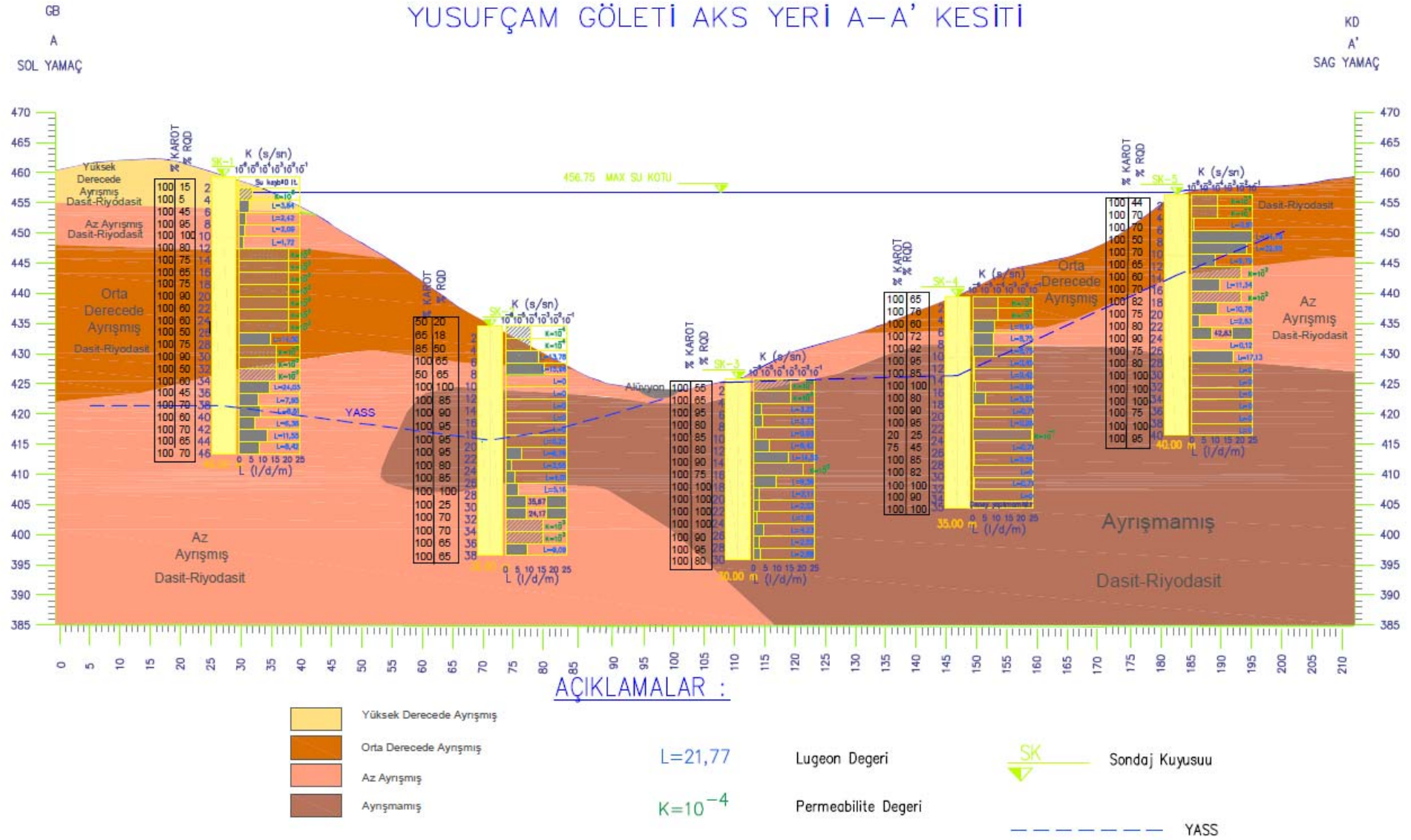
Şekil 3.13: Gölet aks yeri (SK-1,2,3,4,5) kaya kütle özellikleri A-A' kesiti.
