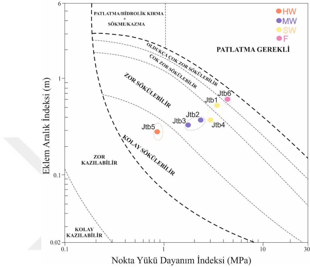
Şekil 3.16: Gölet yerinde tanımlanan jeoteknik birimlerin ve gölet yeri ve göl alanındaki farklı derecede ayrılmış kaya kütlelerinin kazılabilirliğinin Pettifer ve Fookes, (1994) 'e göre değerlendirilmesi.
