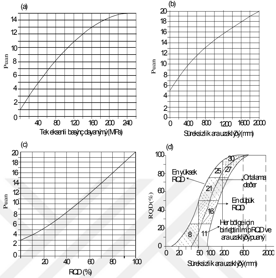
Şekil 3.12: Tek eksenli basınç dayanımı (a), süreksizlik ara uzaklığı (b) ve RQD parametrelerine (c) ait puanları bulmak için kullanılan grafikler (Bieniawski, 1989).
