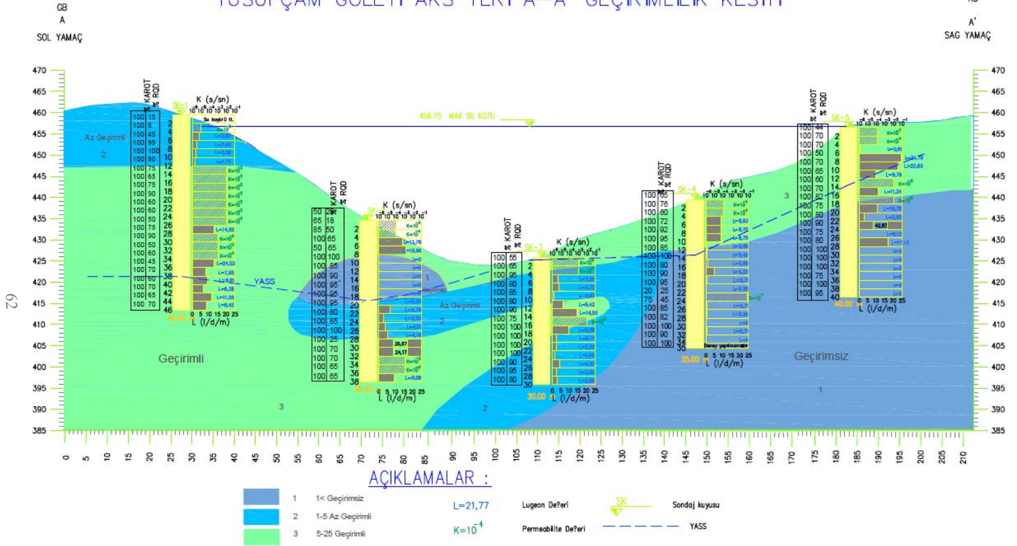
Şekil 3.18: Gölet aks yeri A-A' (SK-1,2,3,4,5) geçirimsizlik kesiti.
