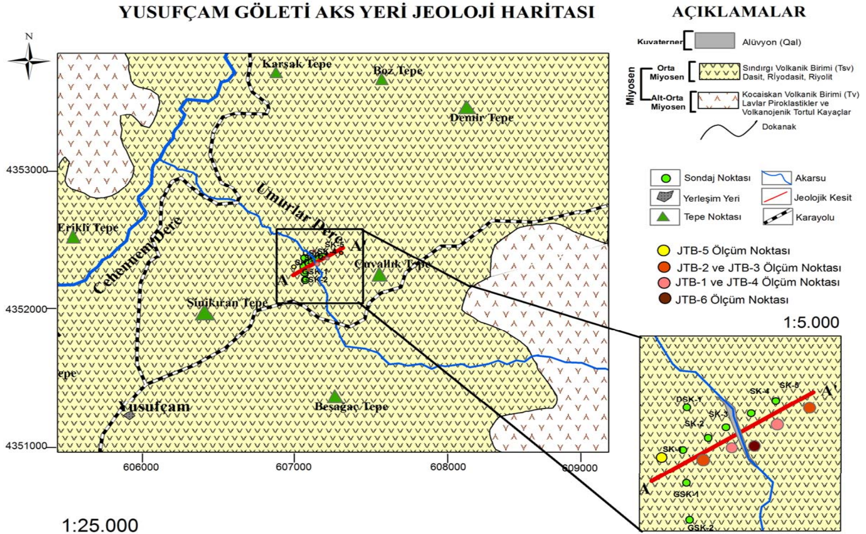
Şekil 3.1: Yusufçam Göleti Aks Yeri Jeoloji Haritası ( http://yerbilimleri.mta.gov.tr ).
