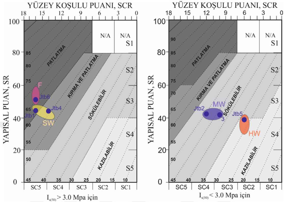
Şekil 3.17: Gölet yerinde tanımlanan jeoteknik birimlerin ve gölet yeri ve göl alanındaki farklı derecede ayrıışmış kaya kütlelerinin kazılabilirliğinin Tsiambaos ve Saroglou (2010)'a göre değerlendirilmesi.
