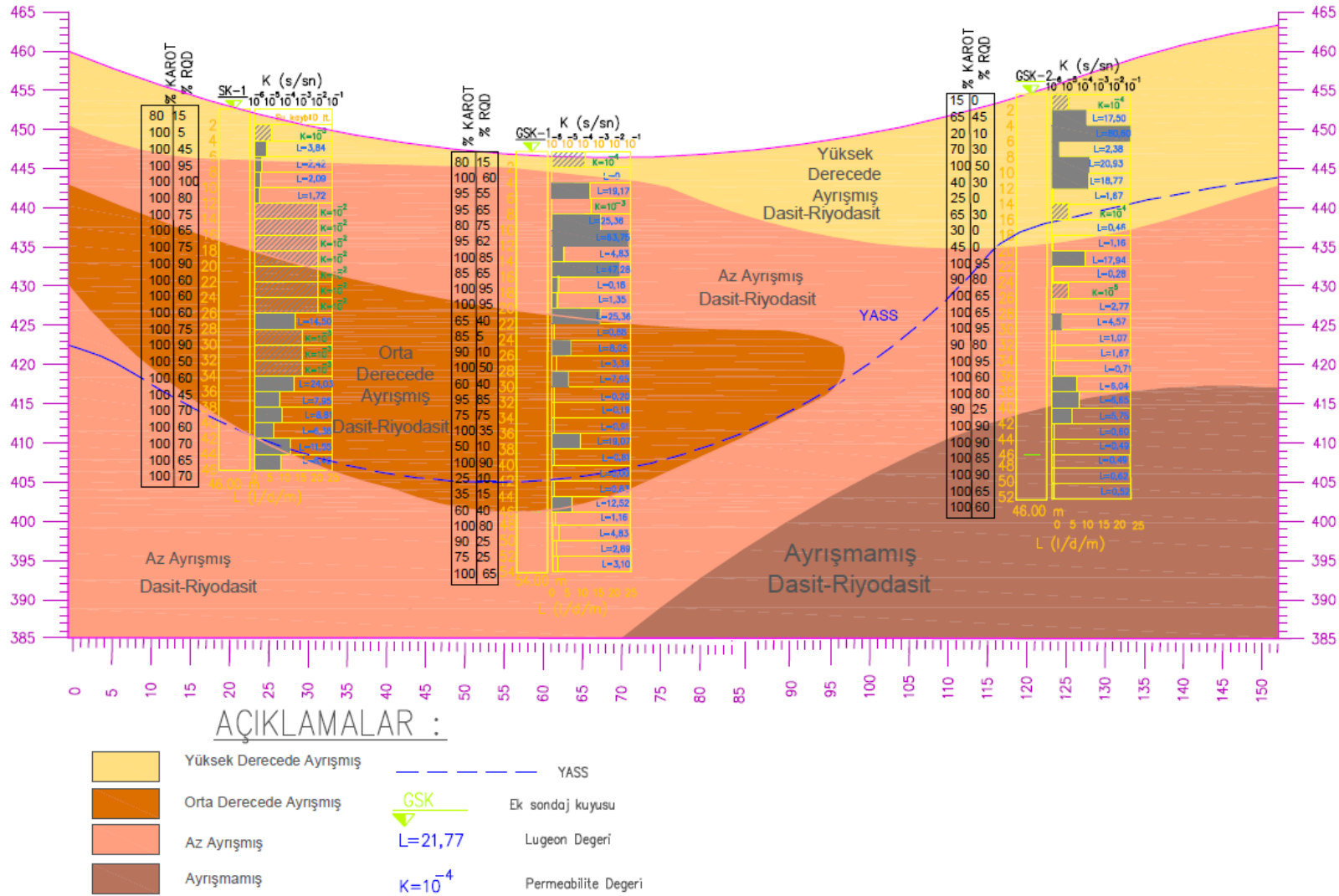
Şekil 3.14: Gölet rezervuar alanı (SK-1, GSK-1 ve GSK-2) kütle özellikleri kesiti.
