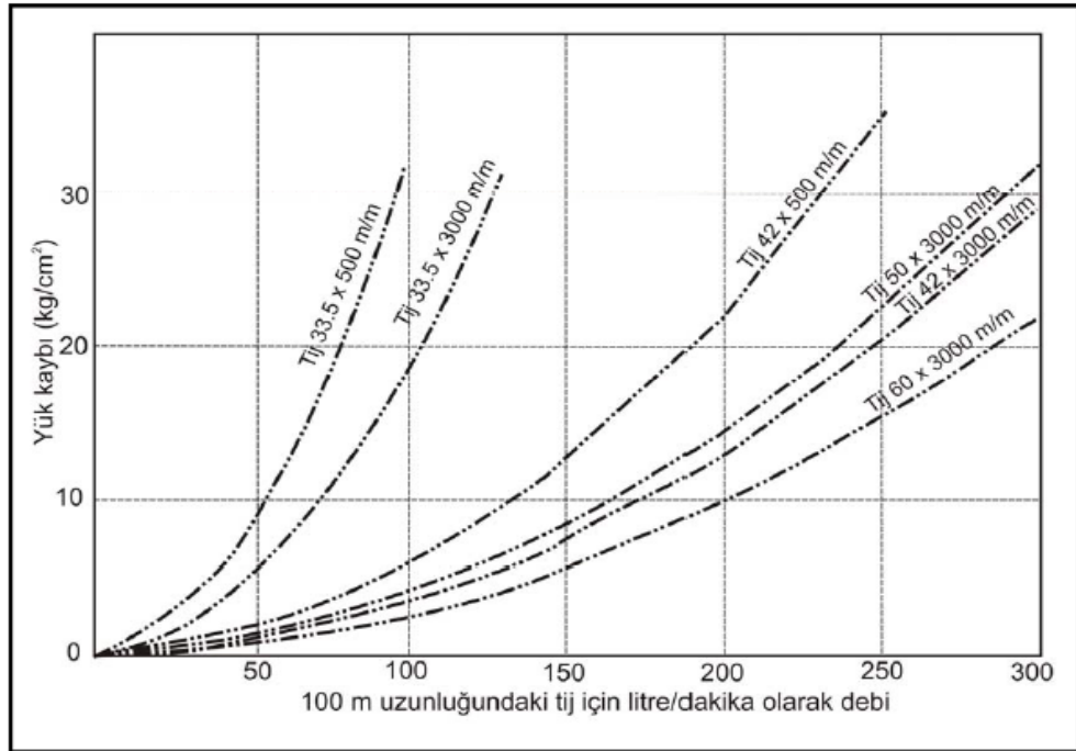
Şekil 2.12: Tij ve manşonlardaki yük kaybını gösterir abak (Şekercioğlu, 2007).
