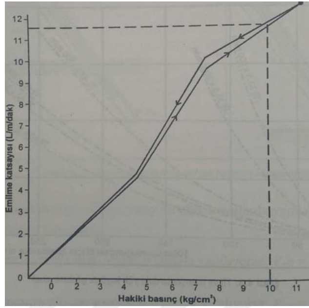
Şekil 2.13: Lugeon deneyi ile geçirimliliğin hesaplanması (Şekercioğlu, 2007).
