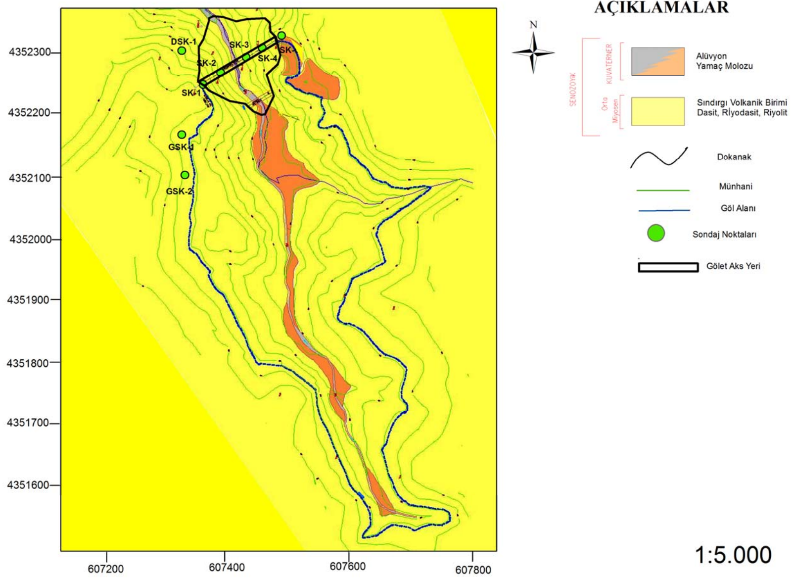
Şekil 3.10: Yusufçam Göletinin Göl Alanı Jeoloji Haritası (DSİ ve Sepa Müh. Müş. İnş. Tic. Ltd. Şti, 2015).
