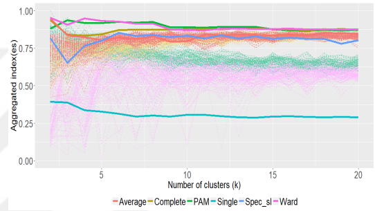
(d) Range: AW+(0.5)AB+Ent+PG+NSB K \sim [2 : 20]
