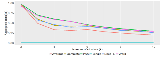
(b) CH Index K \sim [2 : 10]
