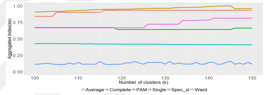
(f) Dunn Index K \sim [100 : 150]
