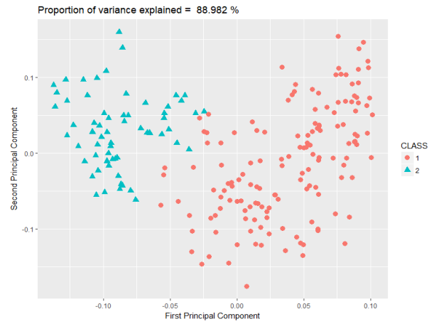
(d) Ward's method ( K = 2 )
