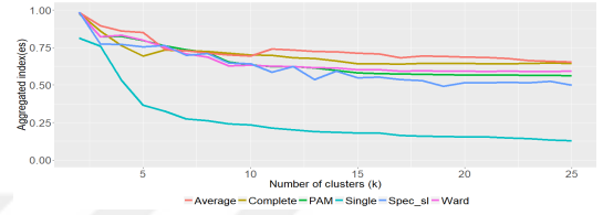
(d) ASW Index K \sim [2 : 25]
