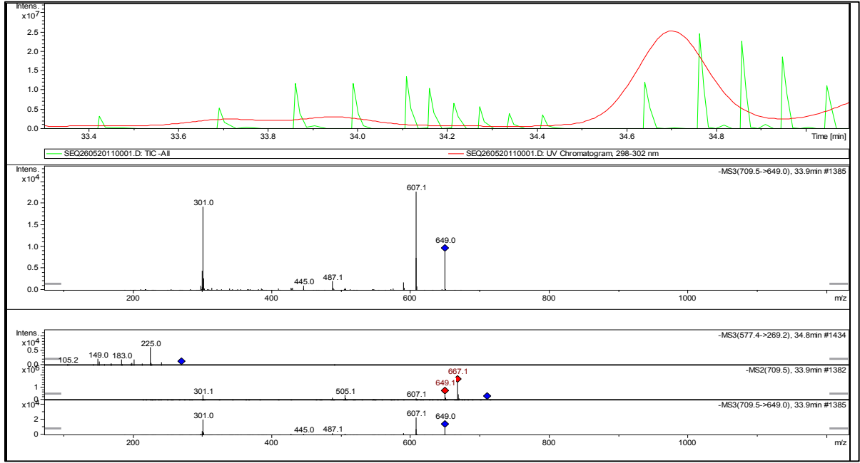
Şekil 70: Hipoletin 7-O-[6'''-O-asetil]-allosil-(1→2)-[6''-O-asetil]-glukozit için UV spektrumu, MS, MS 2 ve MS 3 kütleleri
