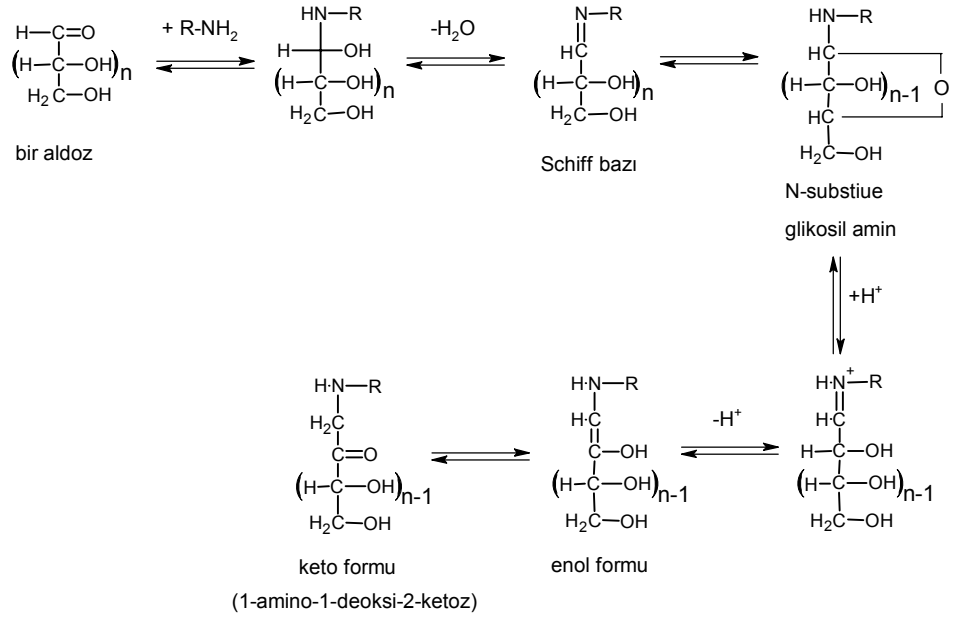
Şekil 1.2. Maillard tepkimesinin ilk basamakları
