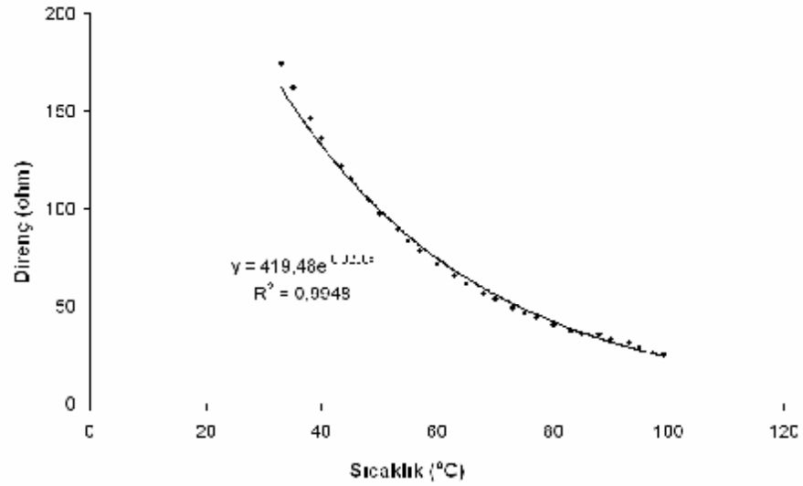
Şekil 2.4. Termistörün sıcaklık-direnç değişimi grafiği
