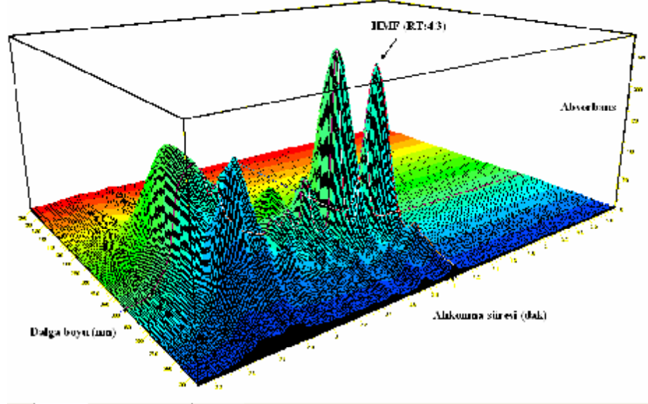
Şekil 3.24. Glyglygly' nin glukoz ile tepkimesinden (pH 5.5, 110°C), 4 saat sonra alınan numuneye ait spektro-kromatogram
