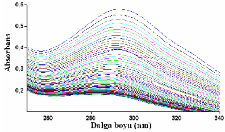
Şekil 3.11. Lisin/glukoz (pH 7) sisteminin 45°C’ de 22 saatlik ısıtma süresi boyunca 20 dakikada bir kaydedilen spektrumları
