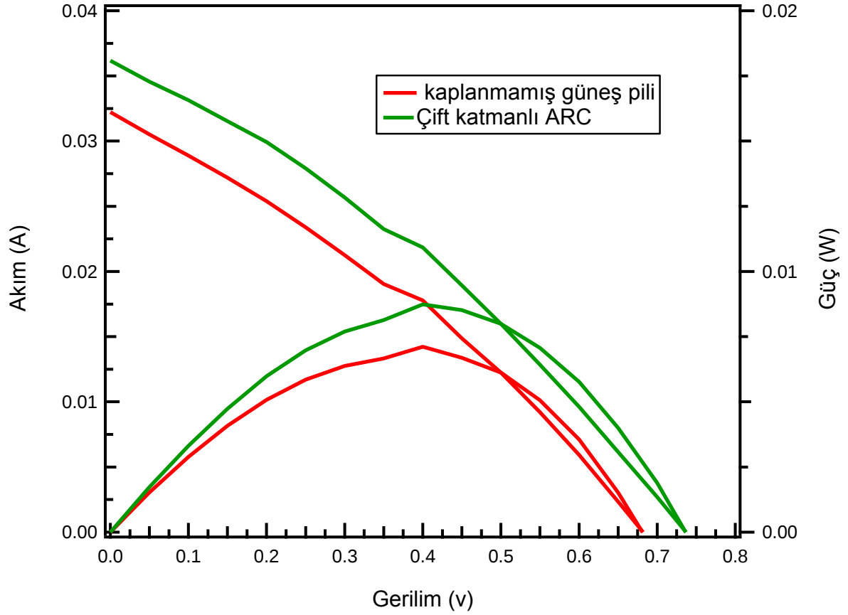
Şekil 5.9. a\text{-SiO}_x\text{:H}/a\text{-SiN}_x\text{:H} yapısındaki yansıtma kaplama yapılmış güneş gözesi için, kaplama öncesi ve sonrası için akım-gerilim ve güç gerilim eğrileri
