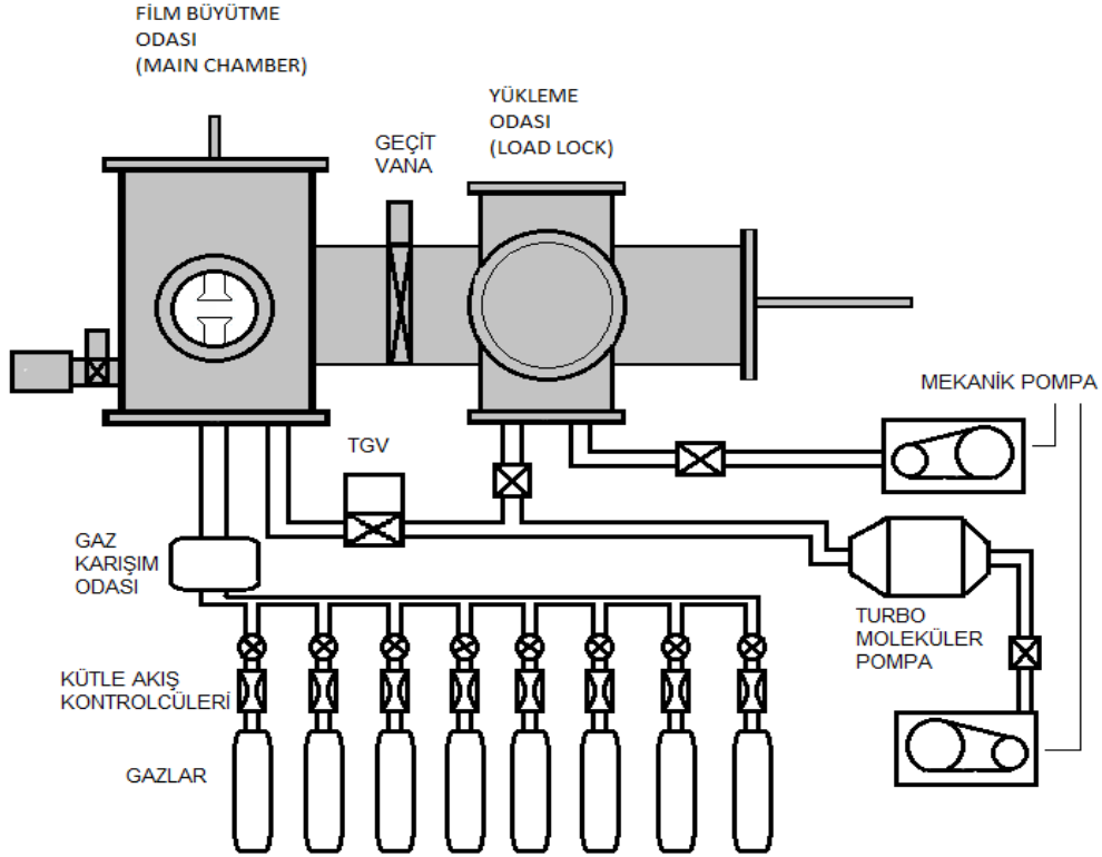
Şekil 3.1. PECVD sistemi
