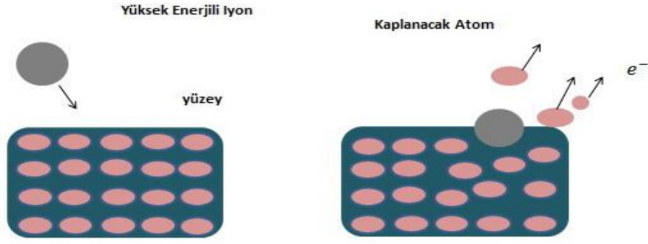
Şekil 2.8. Saçtırma mekanizması [45]
