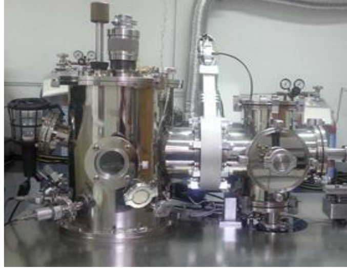
Şekil 2.9. Çift odacıklı PECVD sistemi
