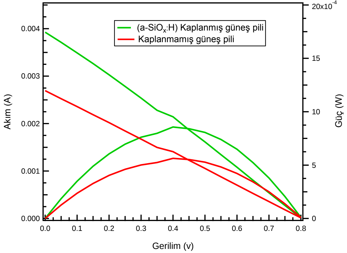
Şekil 5.3. Tek katman a\text{-SiO}_x\text{:H} yansıtma kaplama yapılmış güneş gözesi için, kaplama öncesi ve sonrası için akım-gerilim ve güç gerilim eğrileri.
