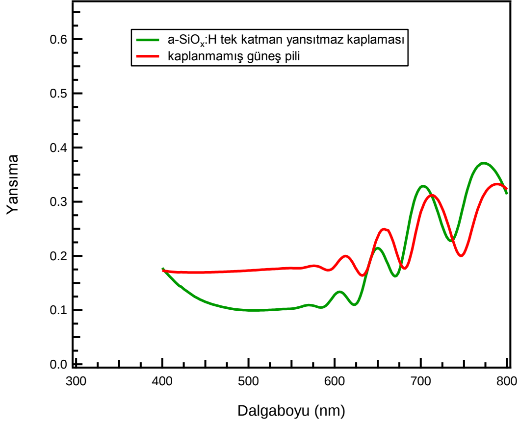
Şekil 5.2. Tek katman a-SiO x :H yansıtma verimliliği yapılmış güneş gözesi için, kaplama öncesi ve sonrası için yansıtmanın dalgaboyuna bağlı değişimi.
