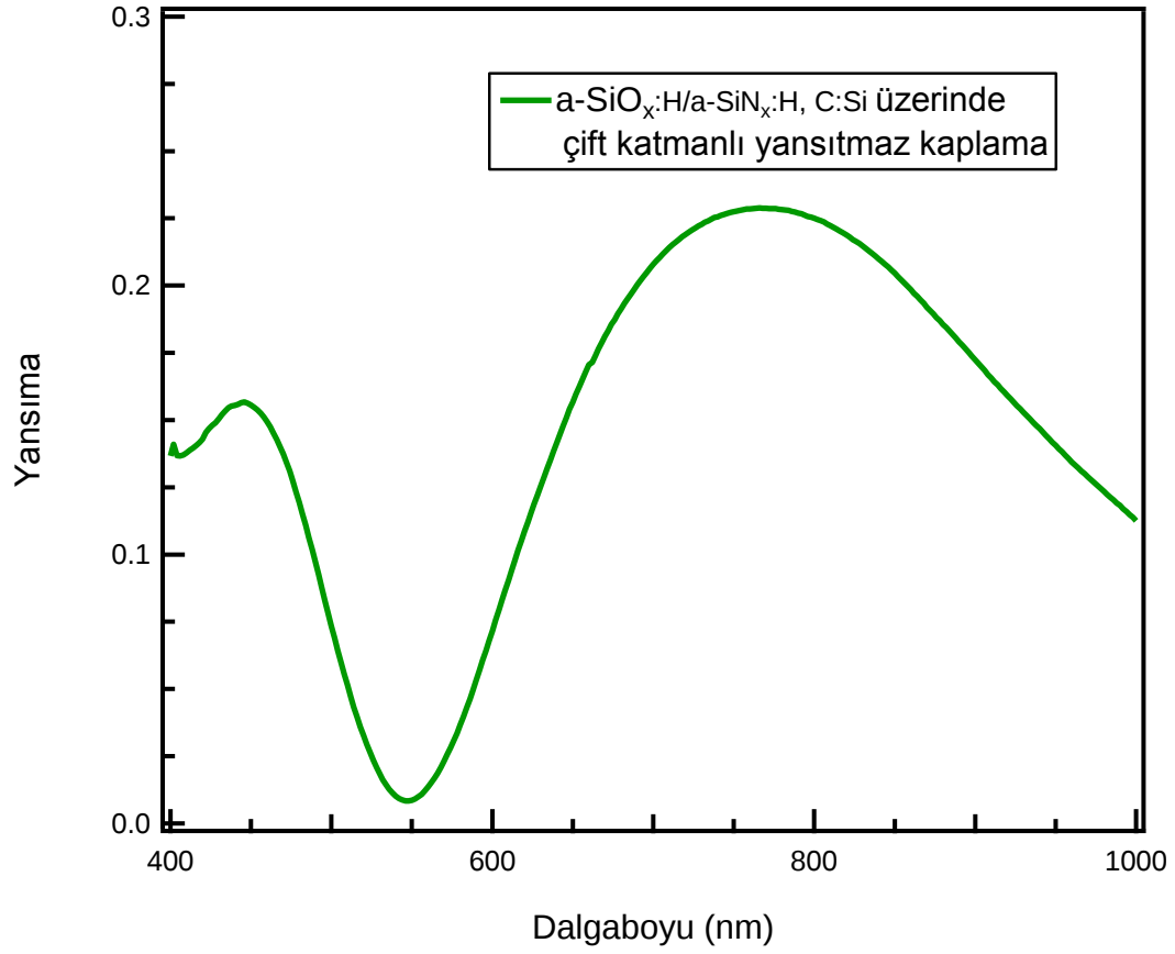
Şekil 4.14. Kristal silisyum üzerinde çift katmanlı yansıma önleyici kaplama
