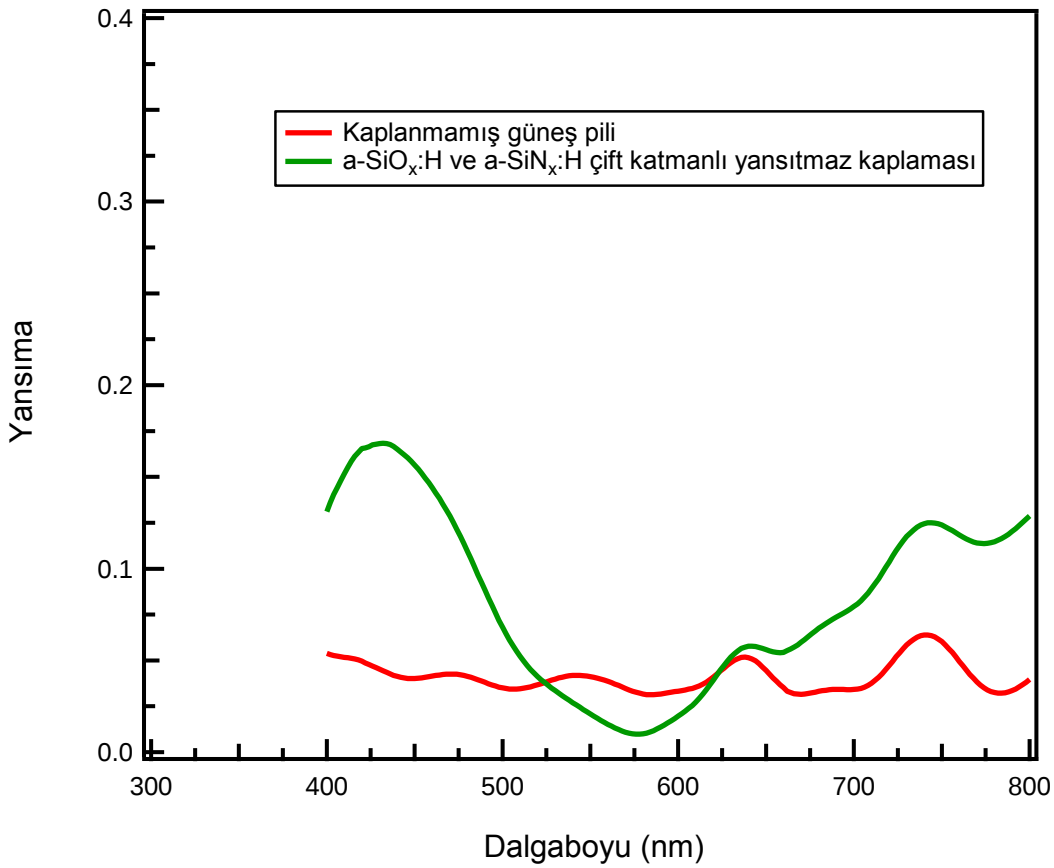
Şekil 5.7. a-SiO x :H/a-SiN x :H yapısındaki yansıtma kaplama yapılmış güneş gözesi için, kaplama öncesi ve sonrası yansıtma spektrumları.
