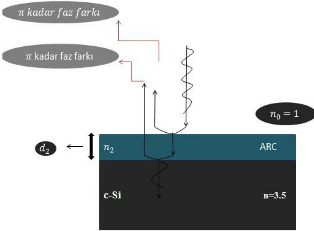
Şekil 4.6. Kristal silisyum üzerinde tek katmanlı yansıma önleyici kaplama
