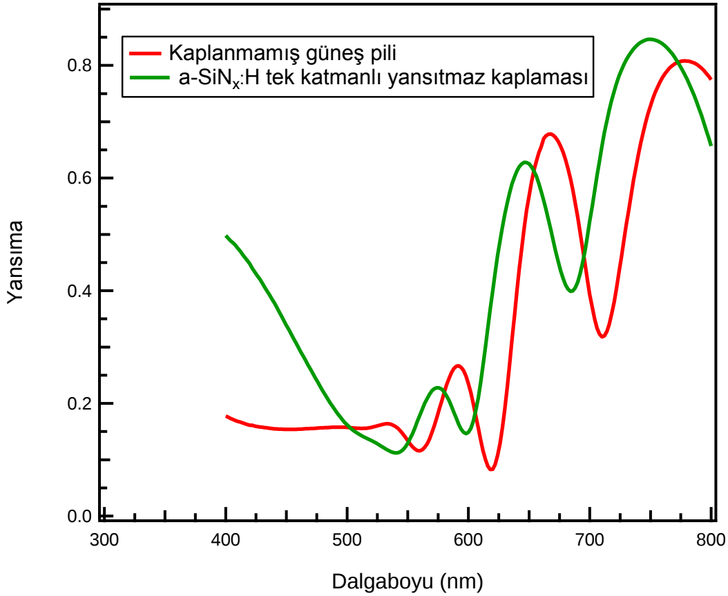
Şekil 5.4. Tek katman a-SiN x :H yansıtmaaz kaplama yapılmış güneş gözesi için, kaplama öncesi ve sonrası için yansıtmanın dalgaboyuna bağlı değişimi.
