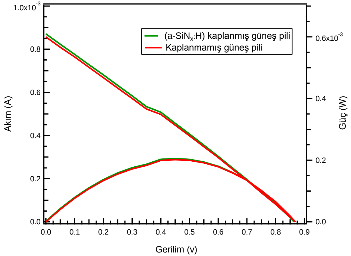
Şekil 5.6. Tek katman a\text{-SiN}_x\text{:H} yansıtma kaplama yapılmış güneş gözesi için, kaplama öncesi ve sonrası için akım-gerilim ve güç gerilim eğrileri.
