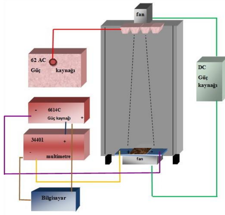
Şekil 3.5. I-V ölçüm düzeneğinin şematik gösterimi.
