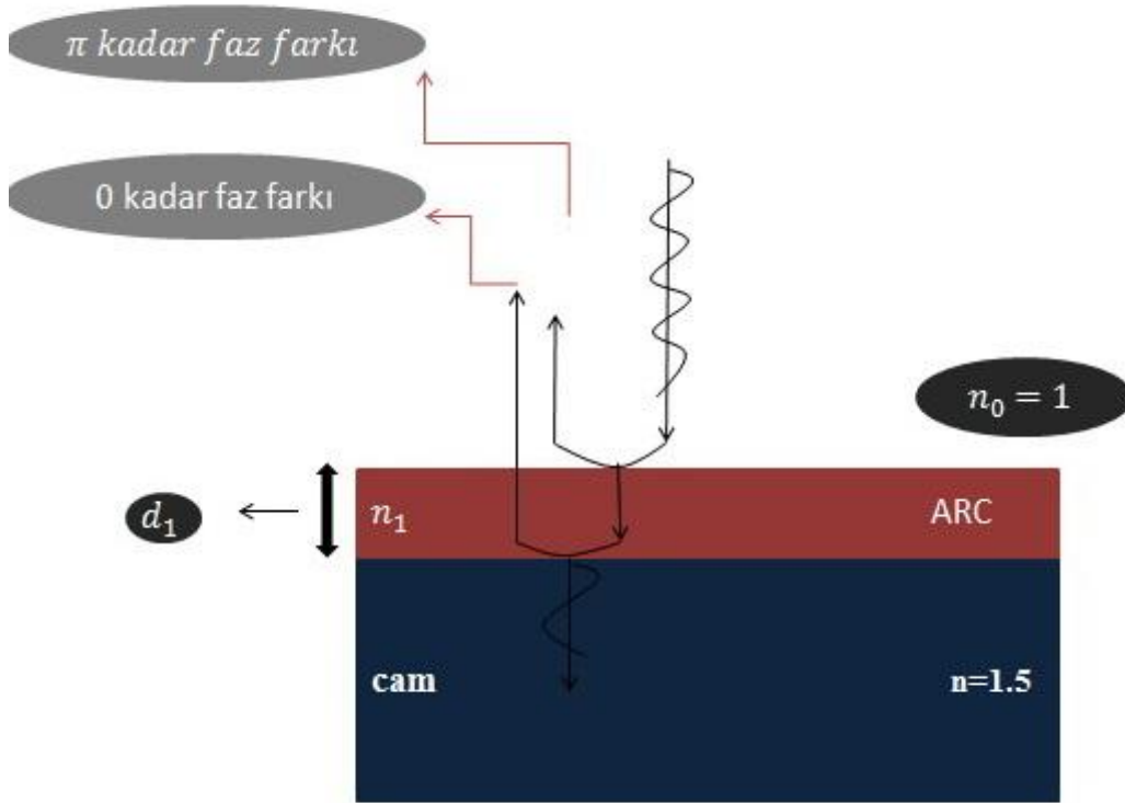
Şekil 4.5. Cam üzerinde tek katmanlı yansıma önleyici kaplama
