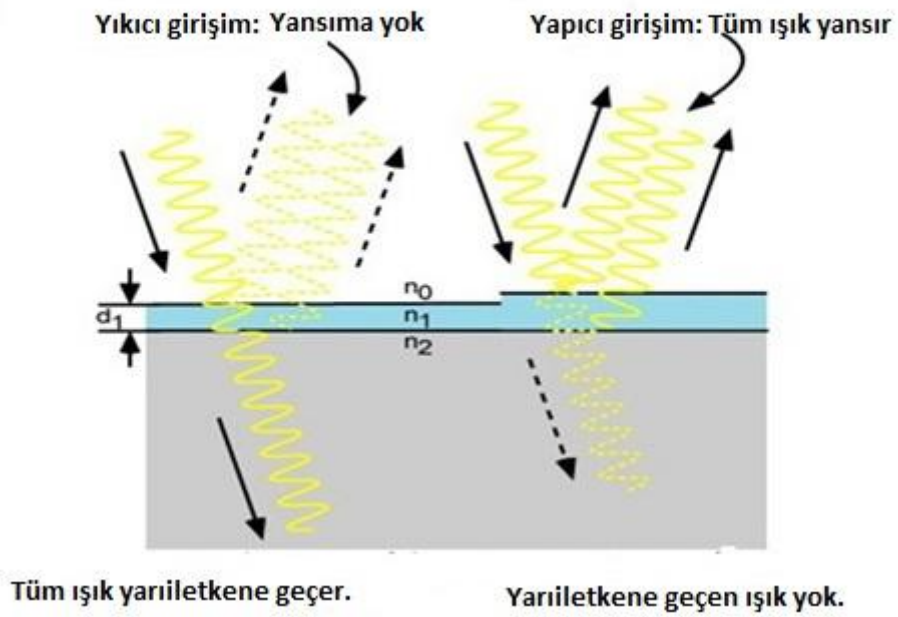
Şekil 2.4. Bir güneş gözesinin yüzeyine, kırma indisi n_1 ve kalınlığı d_1 olan yansıma önleyici kaplama yapılması
