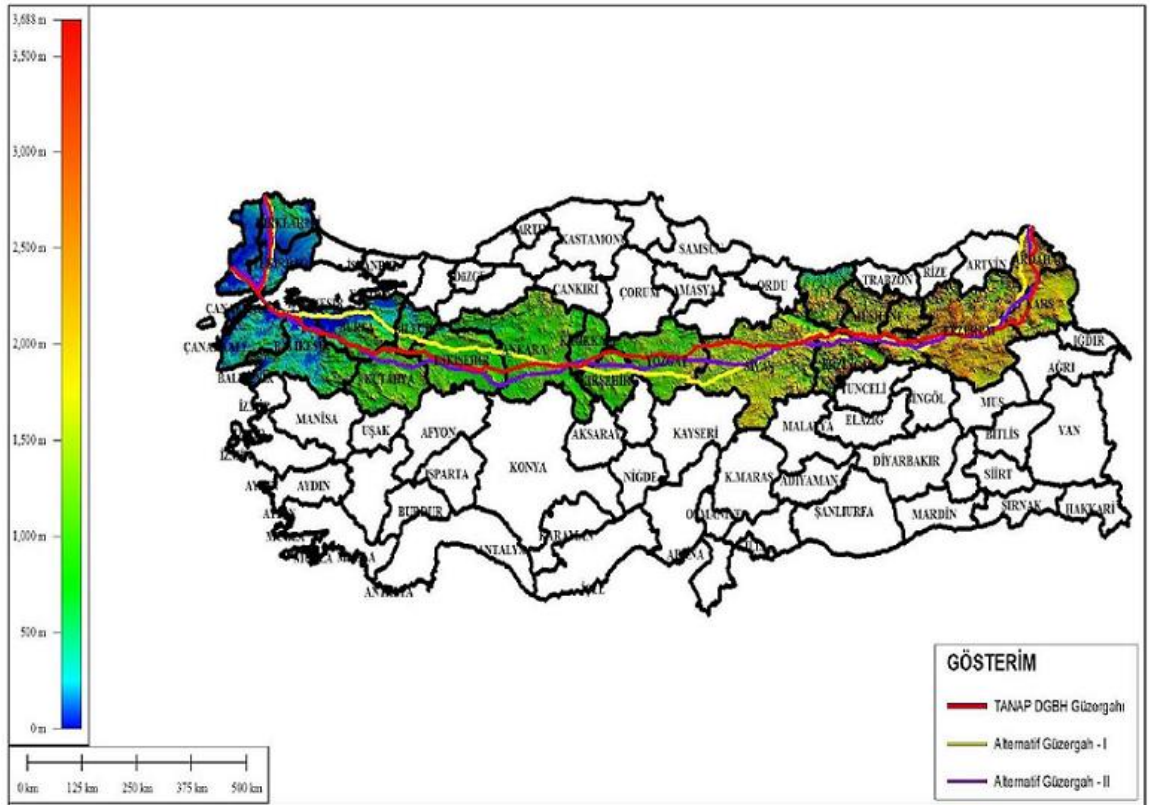
Harita 6: TANAP Proje Güzergâhlarının Sayısal Yükseklik Modeli Üzerinde Gösterimi
