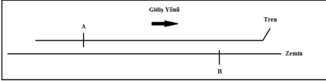
Şekil 7: Referans Cisme Göre Göreceli Hareket
