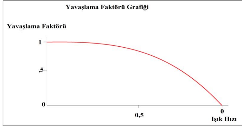
Şekil 9: Zaman ve Işık Hızı İlişkisi
