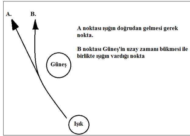
Şekil 13: Uzay Zamanın Bükülmesi ve Işığın Sapması
