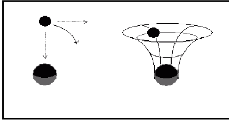
Şekil 10: Kütle ve Uzay Yapısı İlişkisi
