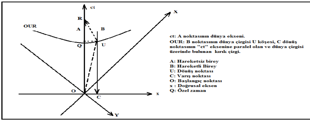
Şekil 8: Saat Paradoksunun Gösterilişi
