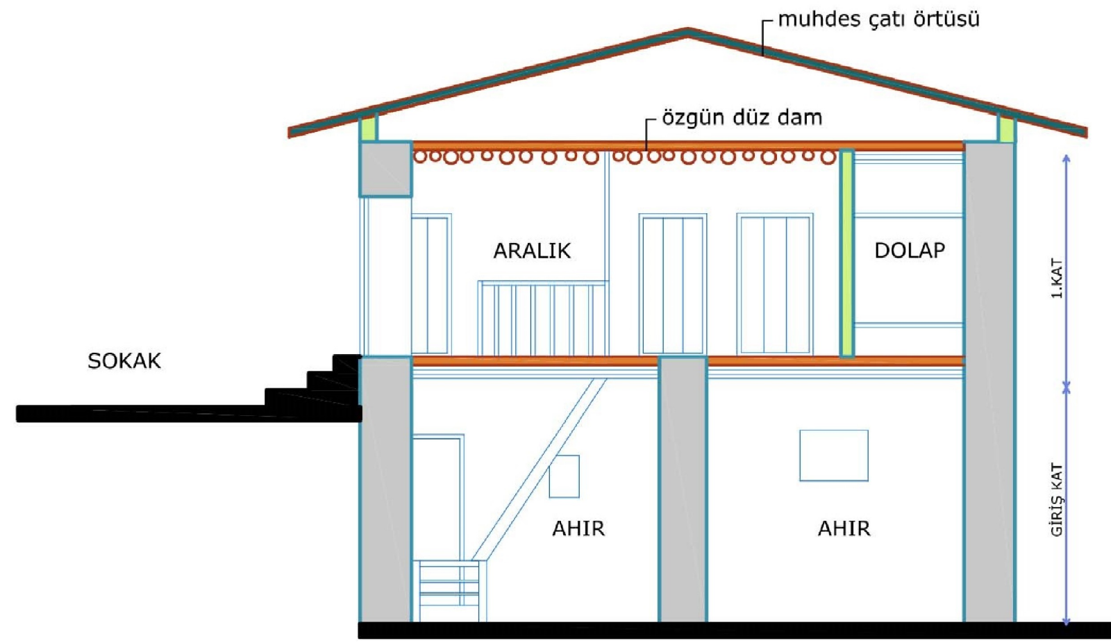
B - B' KESİTİ
