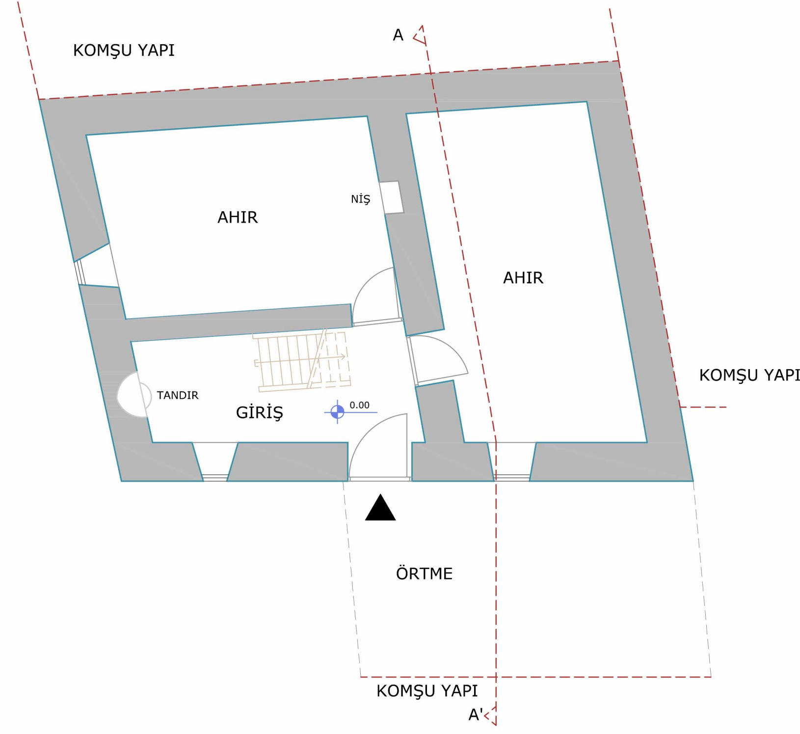
ZEMİN KAT PLANI
