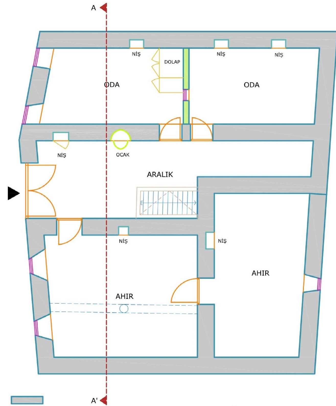
ZEMİN KAT PLANI
