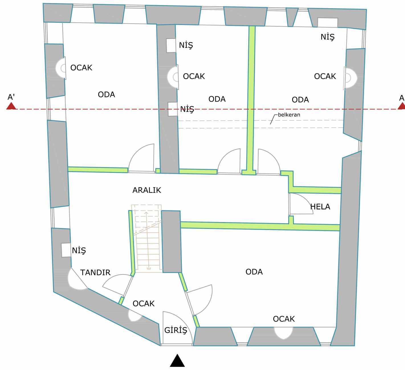
1. KAT PLANI
