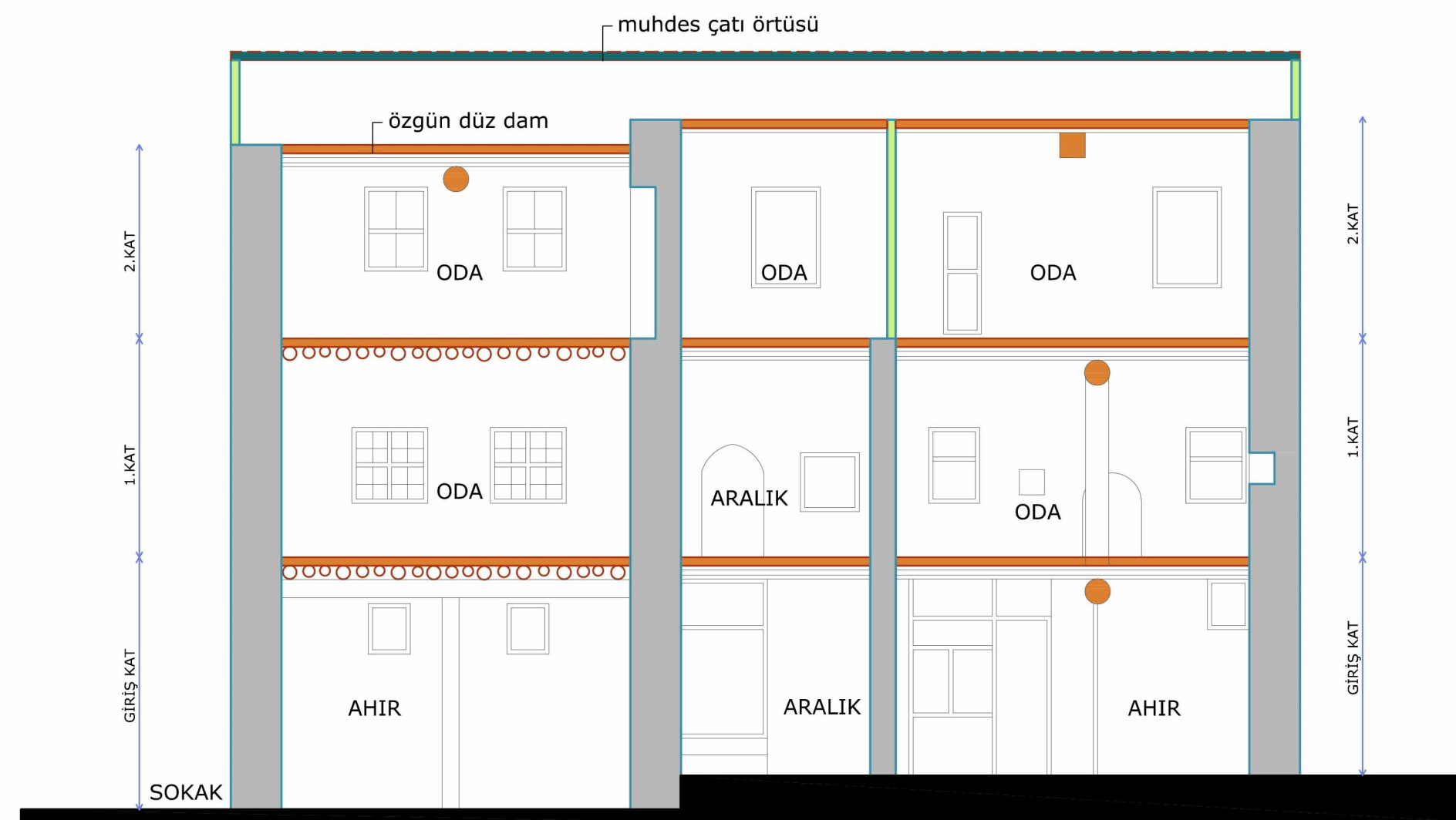
A - A' KESİTİ
