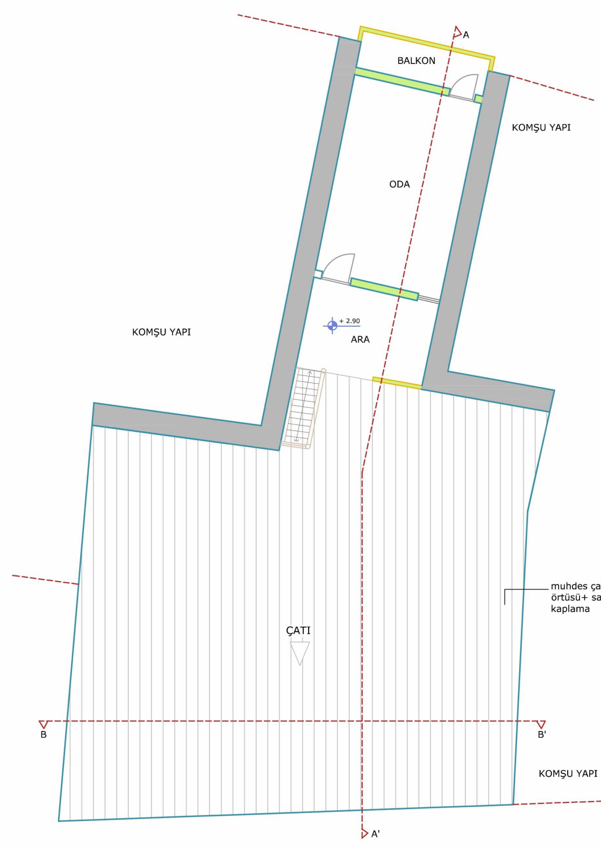
3. KAT PLANI
