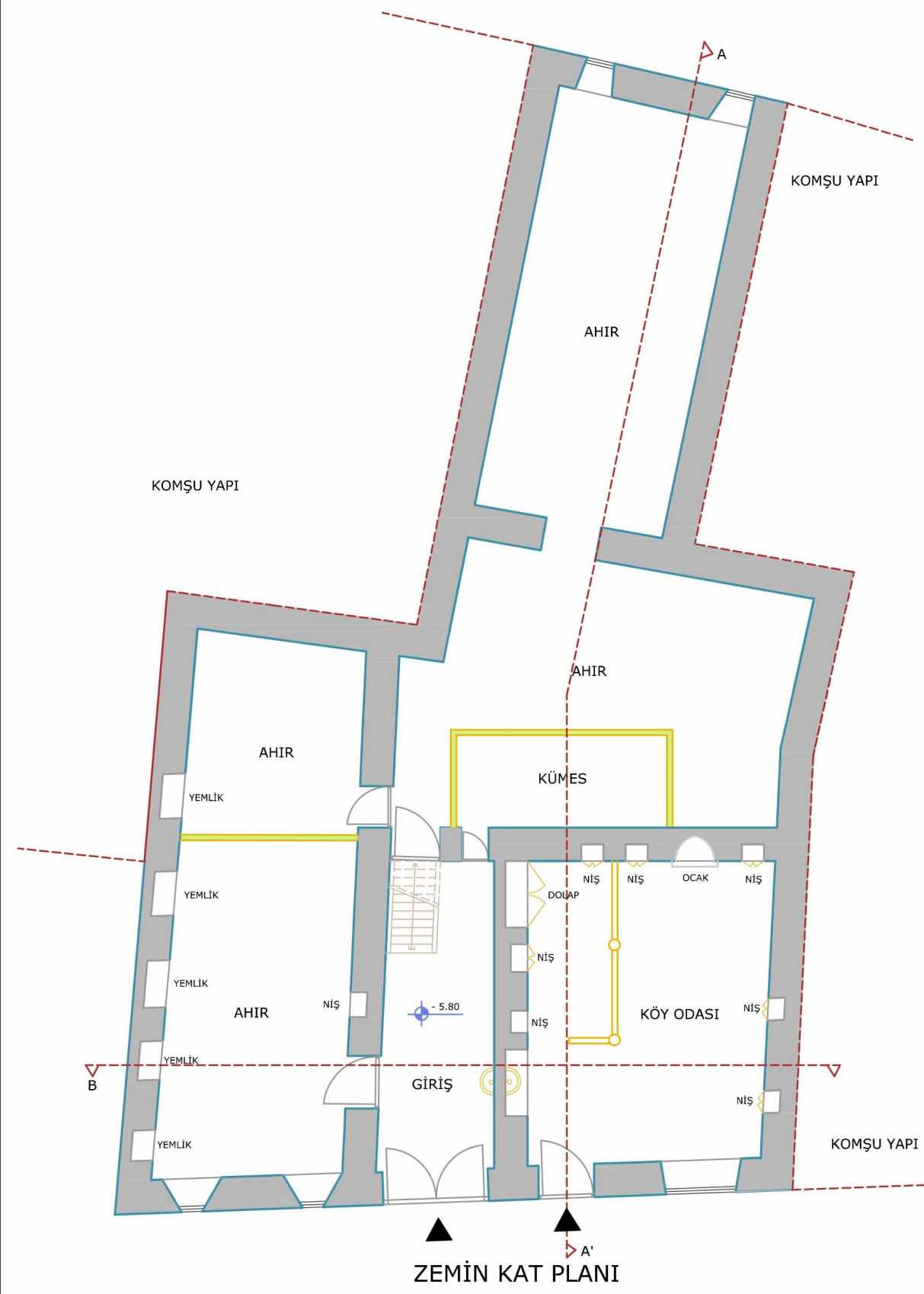
ZEMİN KAT PLANI
