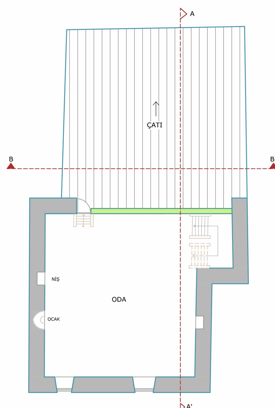
3. KAT PLANI
