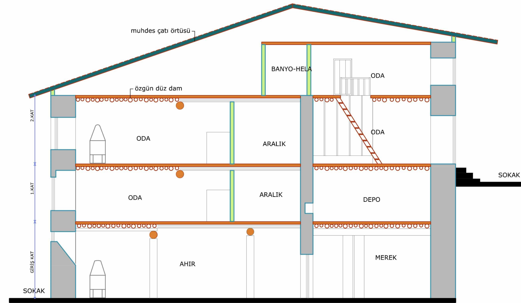
A-A' KESİTİ
