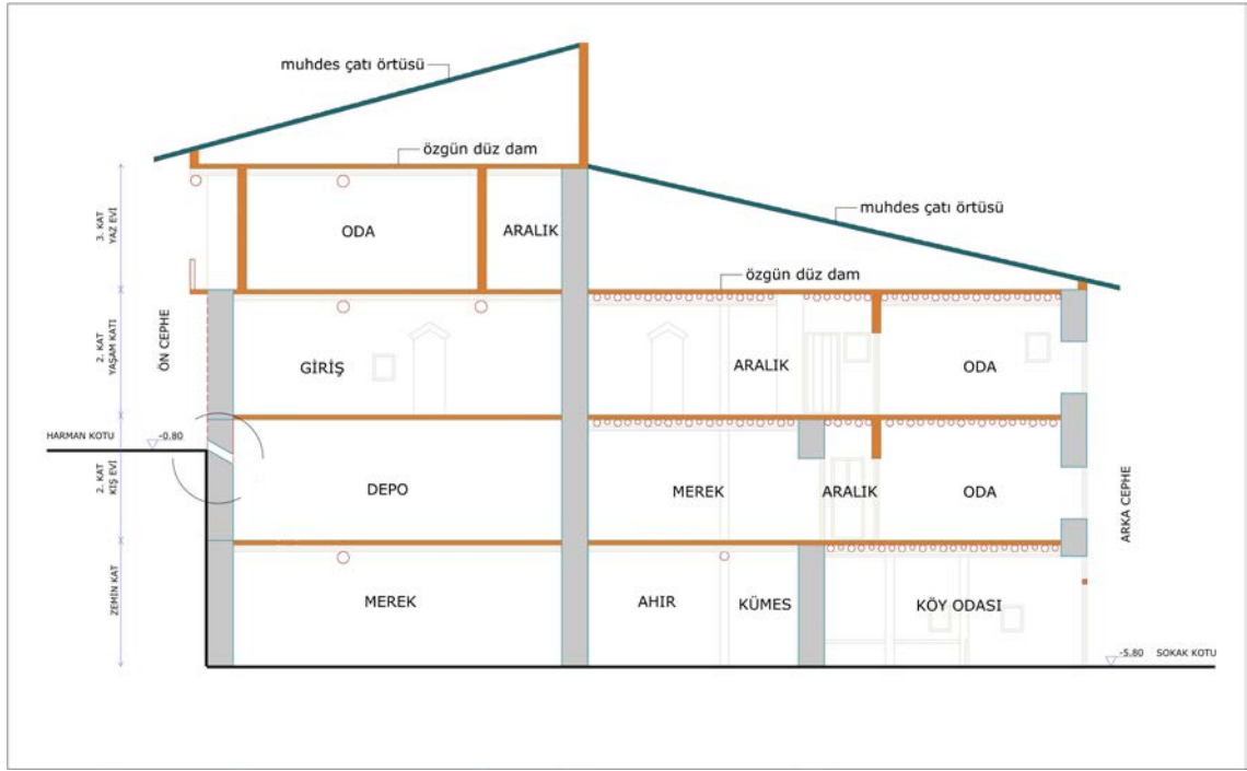
Şekil 5. 10 Harman kotunun altında iki kat olan konut (Envanter no: 264-13)
