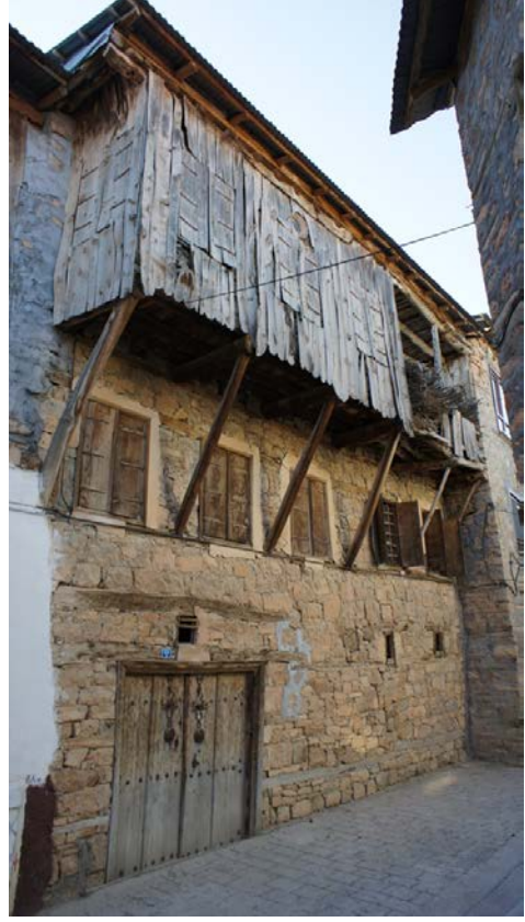
Şekil 5. 34 Çıkmalı cephe örnekleri, 261-43 ve 264-13 yapıları
