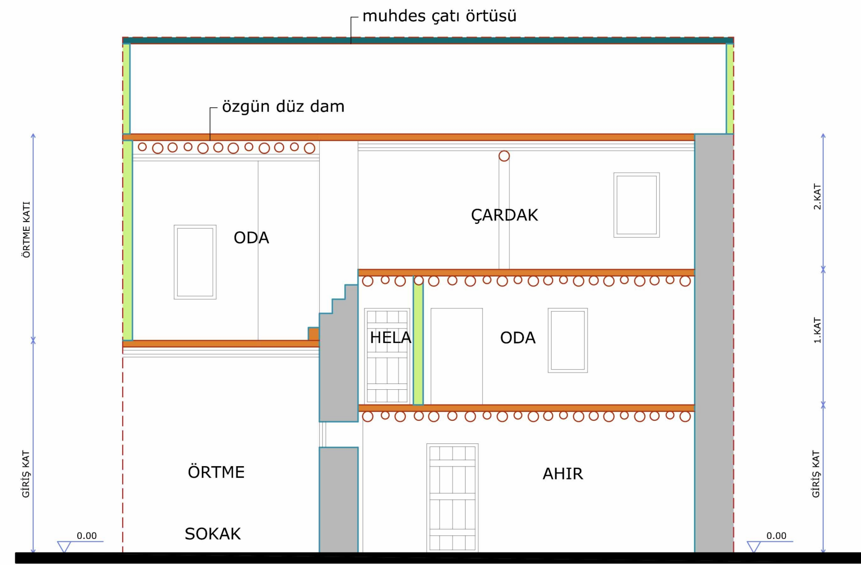
A - A' KESİTİ
