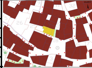
VAZİYET PLANI
