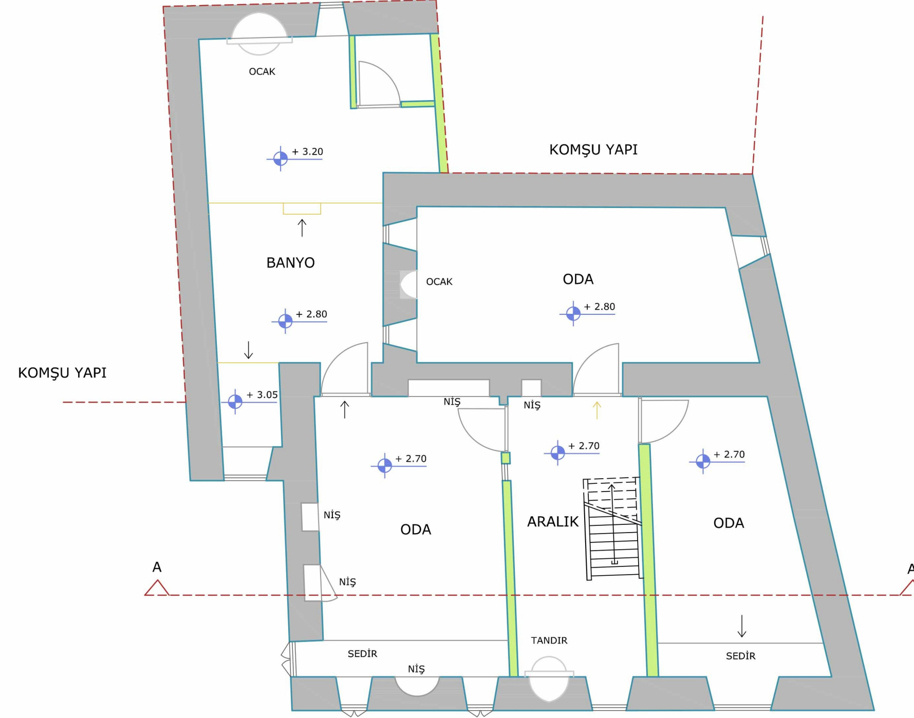
1. KAT PLANI
