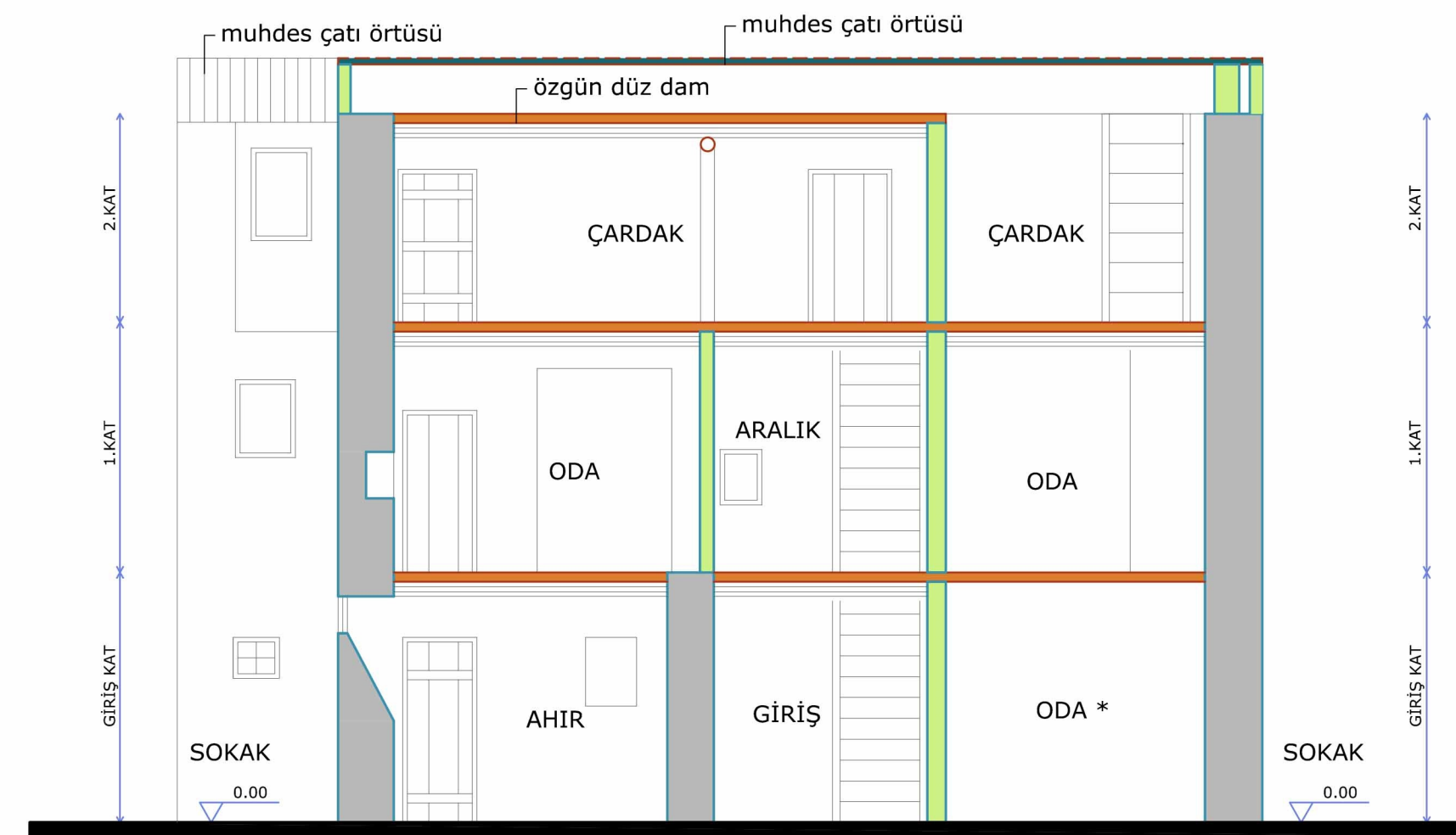
A - A' KESİTİ
