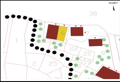
VAZİYET PLANI
