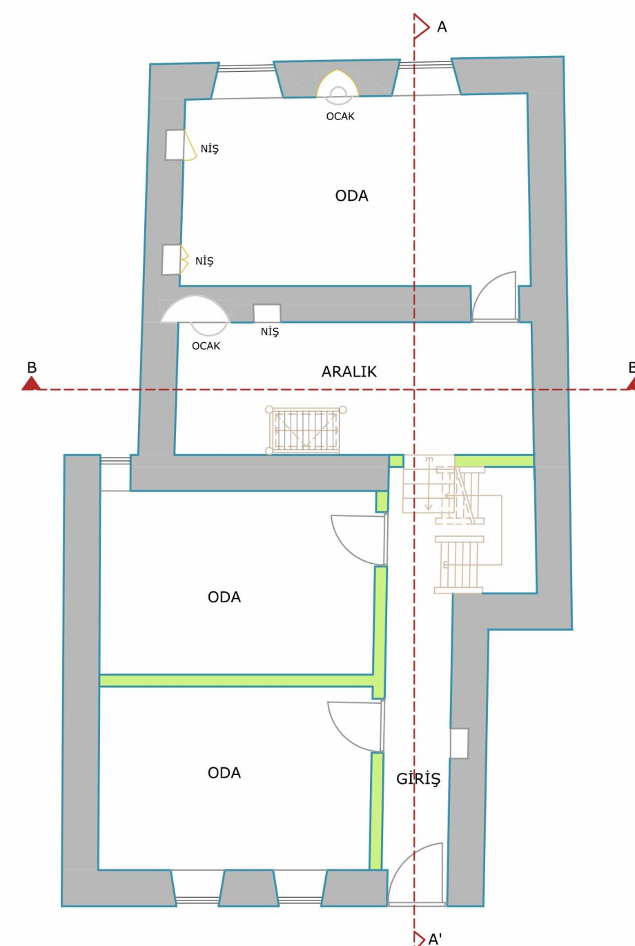
1. KAT PLANI
