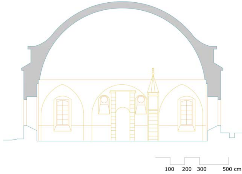
Şekil 3.18 Selim Ağa Cami'sinin kesiti
