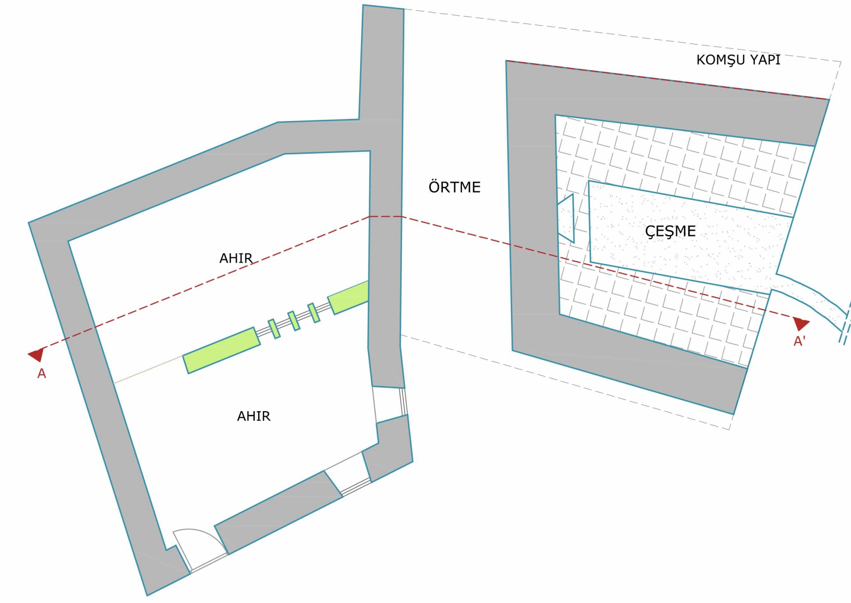
ZEMİN KAT PLANI
