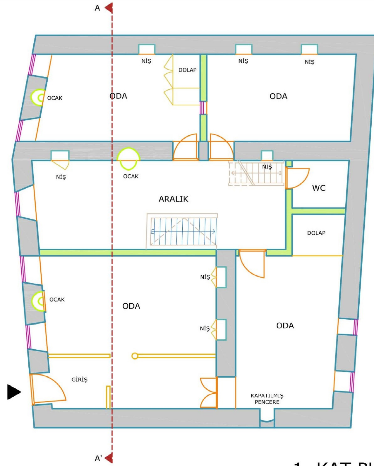
1. KAT PLANI
