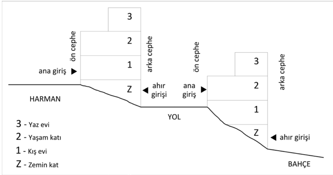
Şekil 5. 4 Konutların eğim ve yol ile olan ilişkileri
