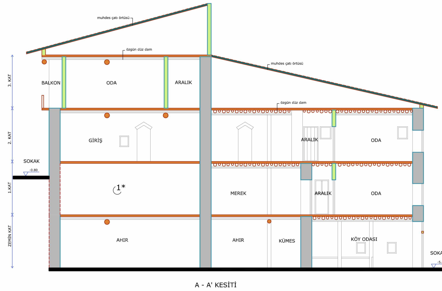
A - A' KESİTİ
