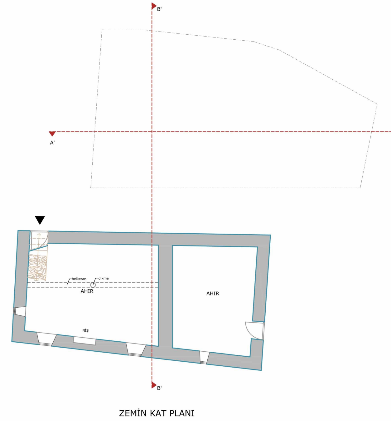
ZEMİN KAT PLANI
