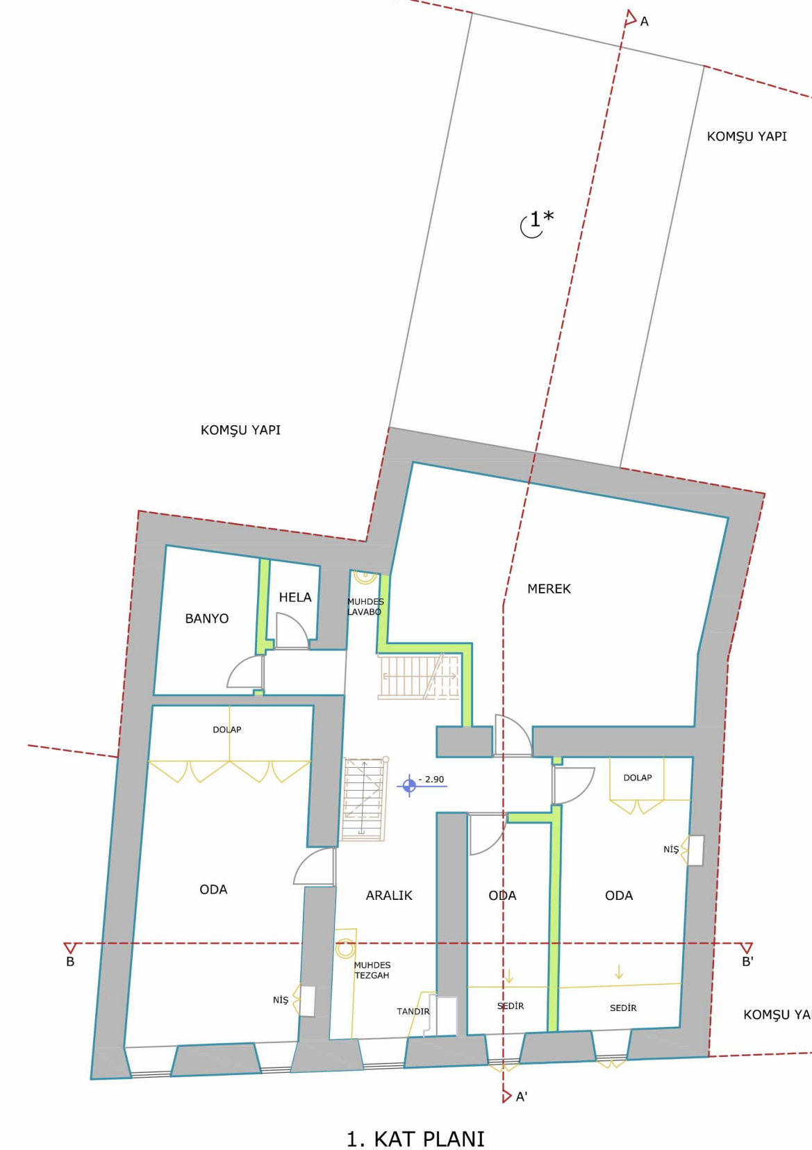
1. KAT PLANI
