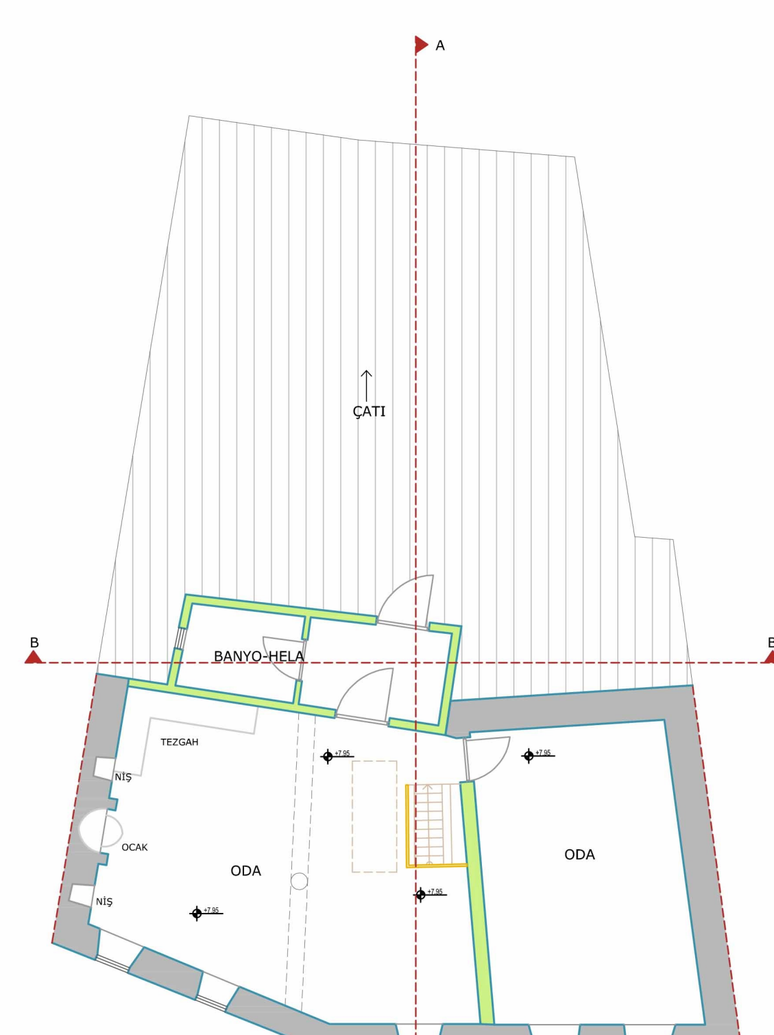
3. KAT PLANI
