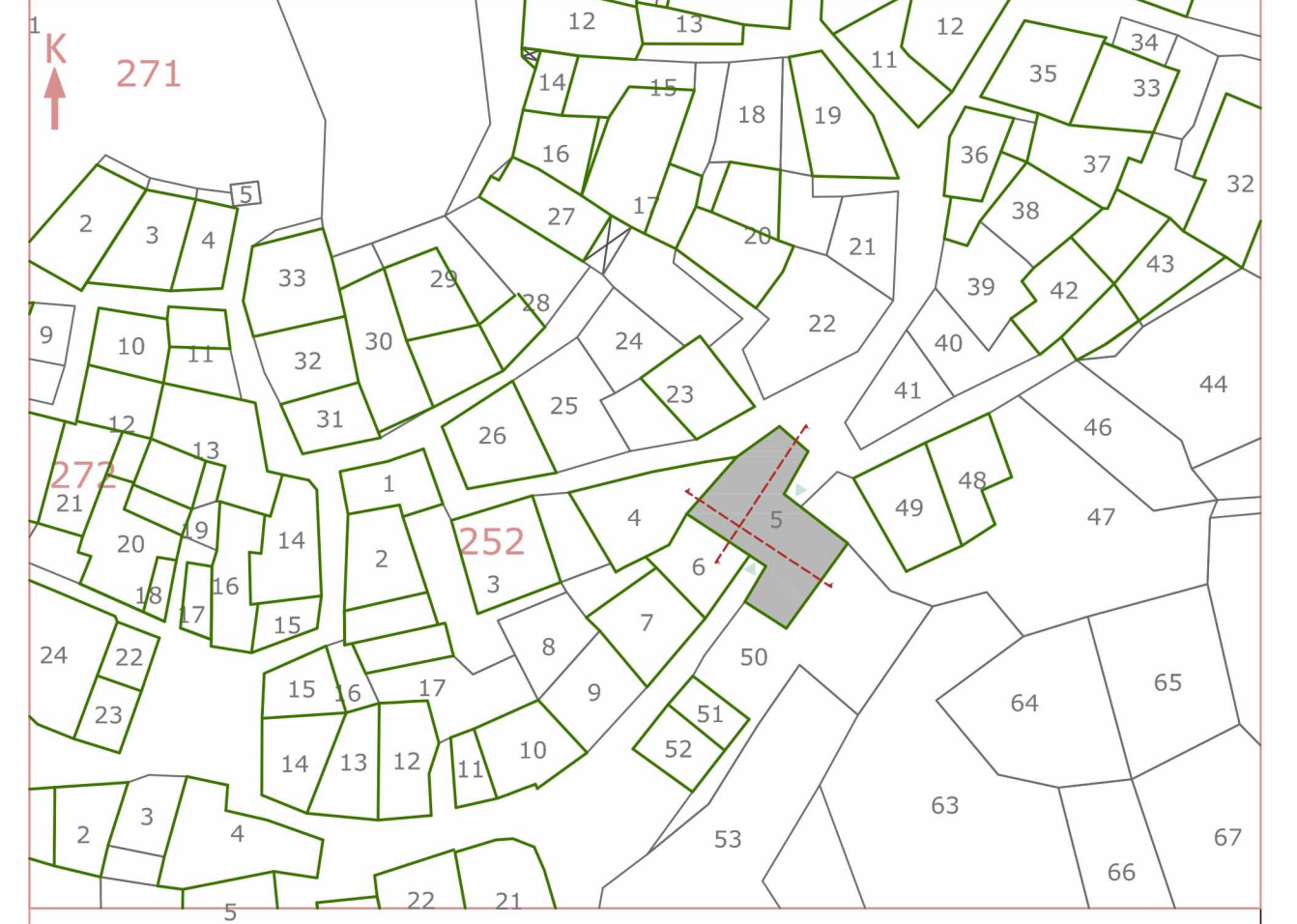
VAZİYET PLANI
