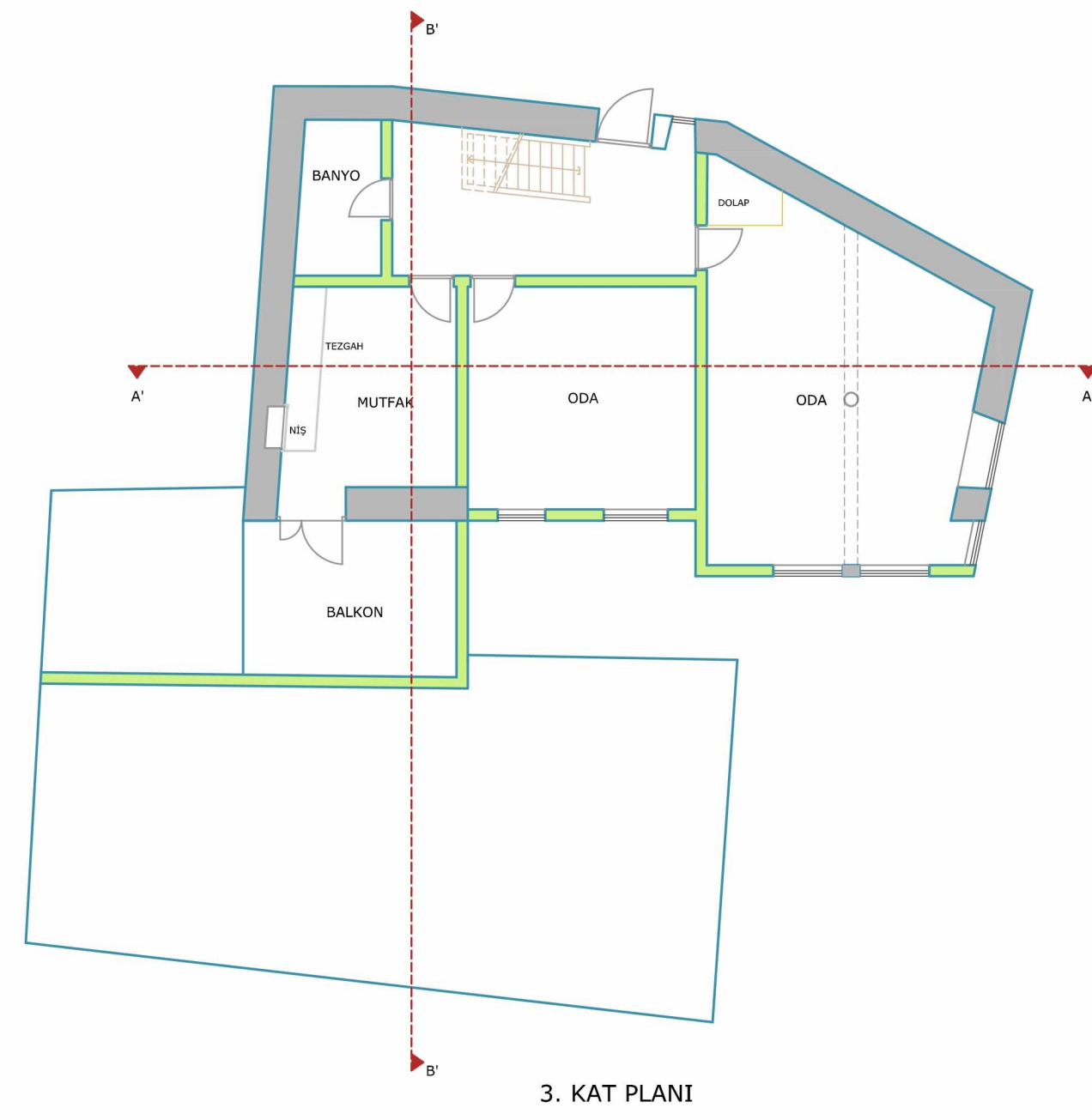
3. KAT PLANI
