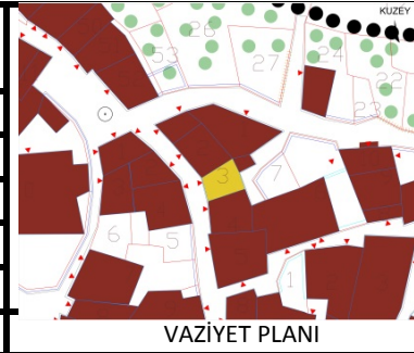
VAZİYET PLANI
