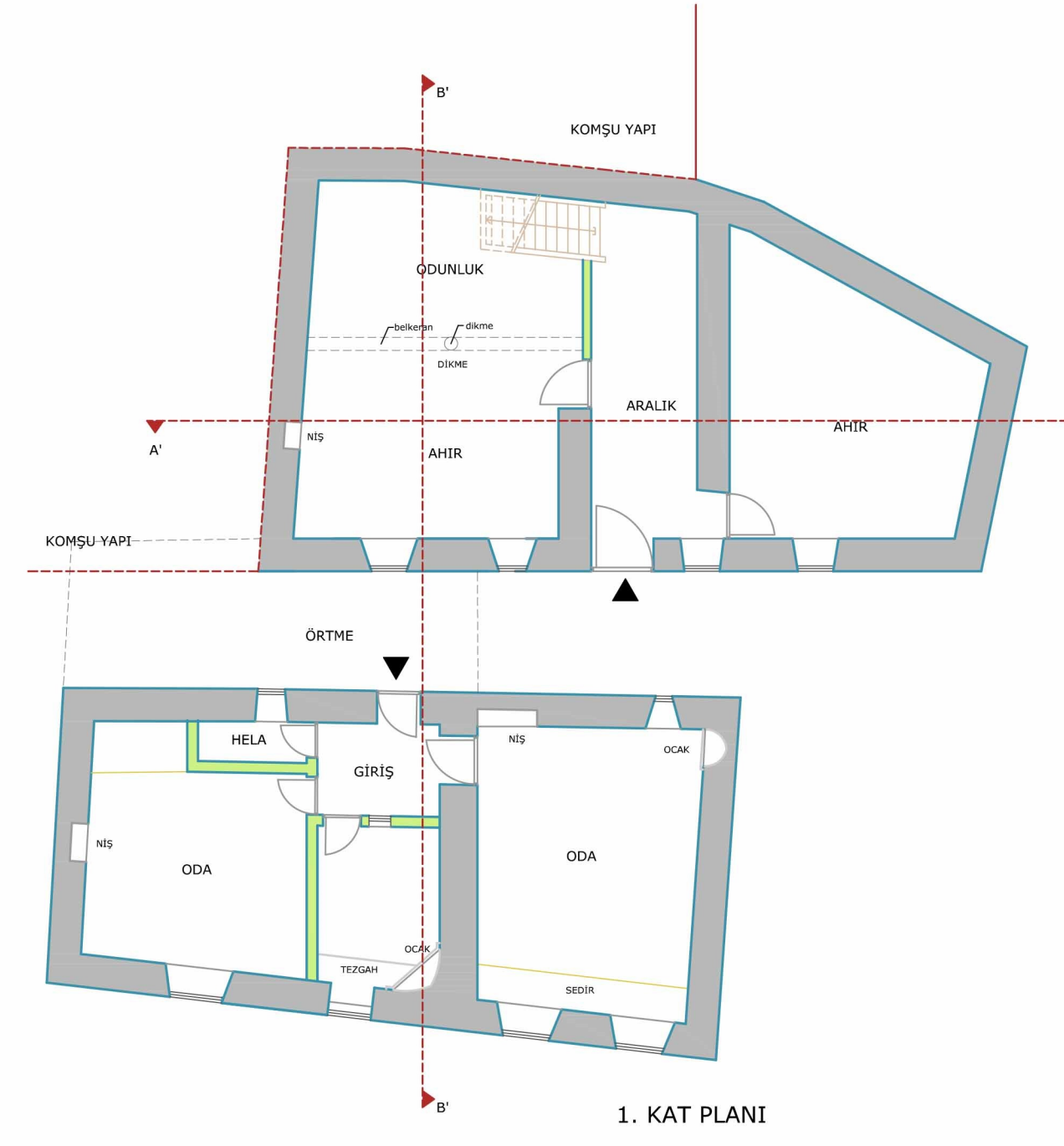
1. KAT PLANI
