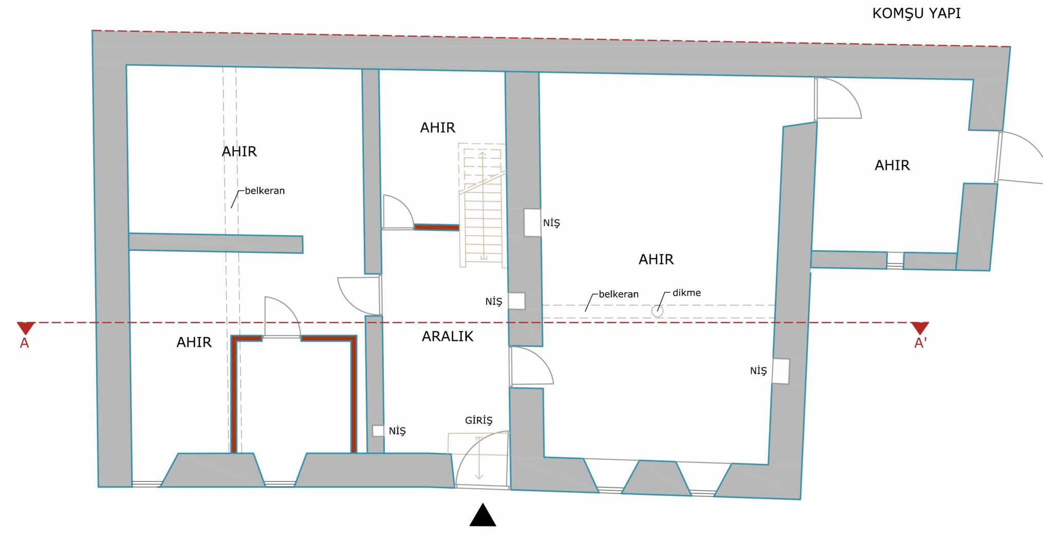
ZEMİN KAT PLANI
