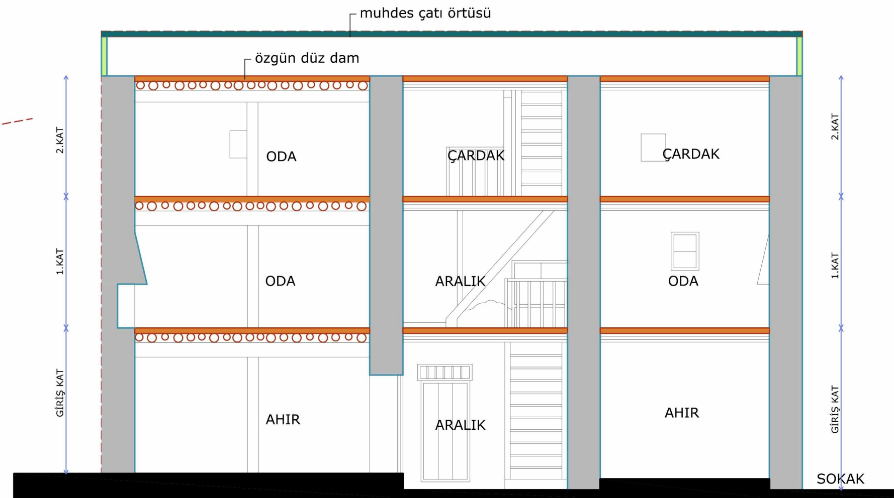
A - A' KESİTİ
