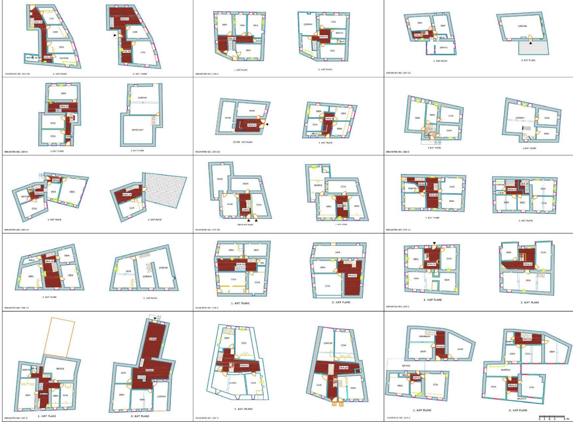
Şekil 5.16 Başpınar yerleşimindeki 15 konutun birinci ve ikinci katlarının çizimleri
