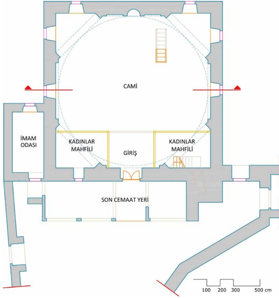
Şekil 3.17 Selim Ağa Cami'sinin planı
