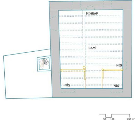
Şekil 3. 33 Cami'nin galeri katı planı
