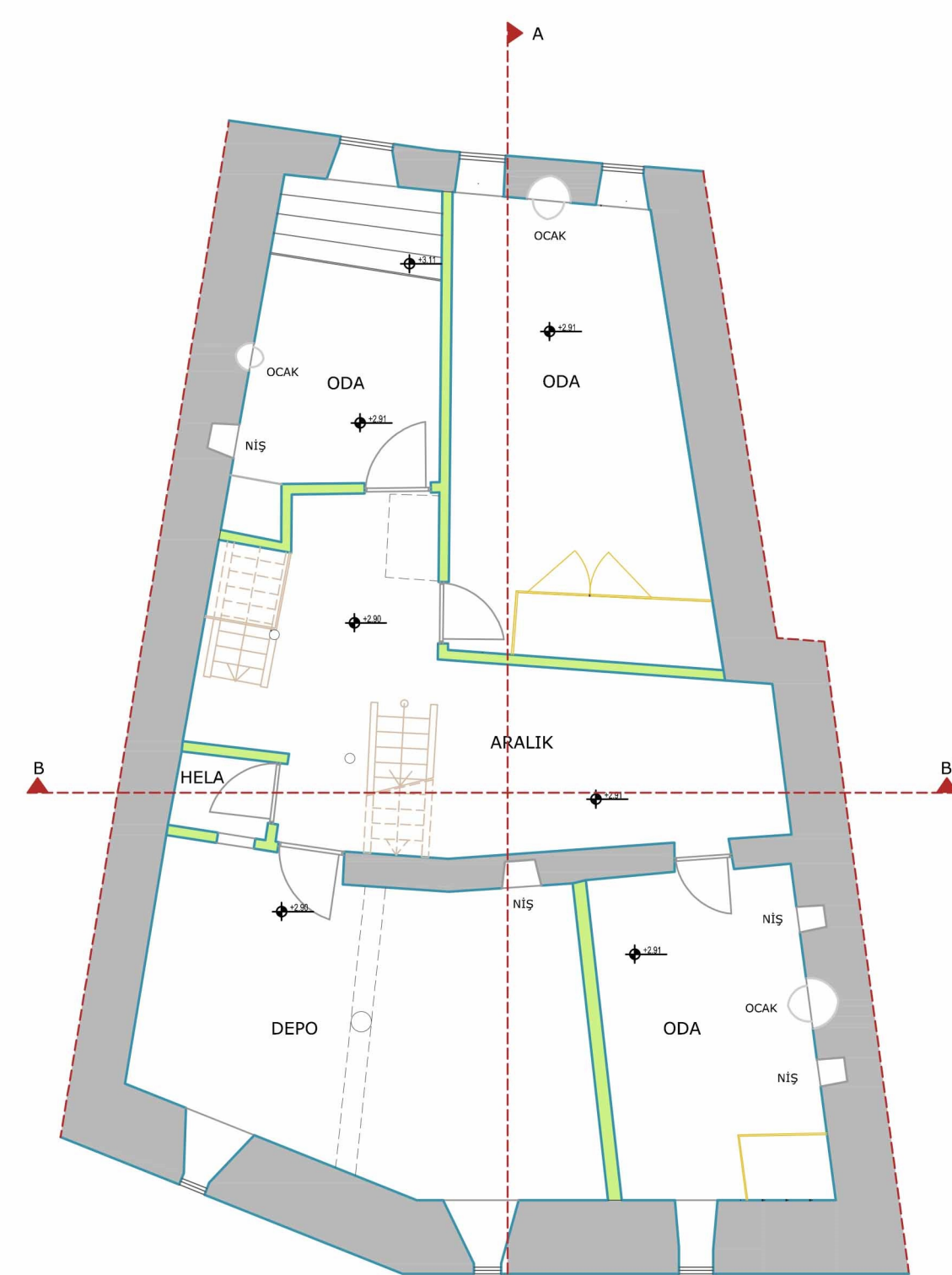
1. KAT PLANI
