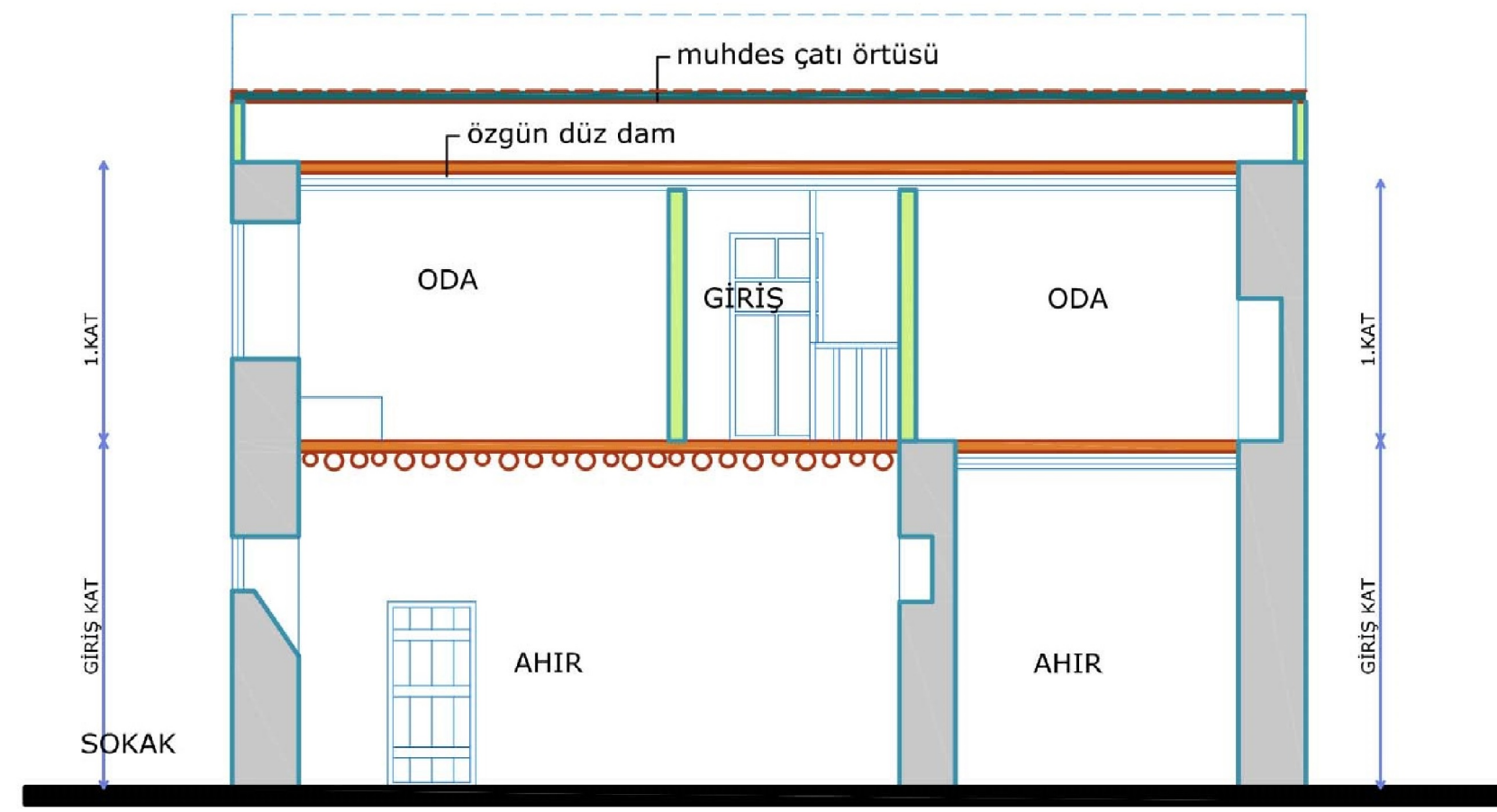
A - A' KESİTİ
