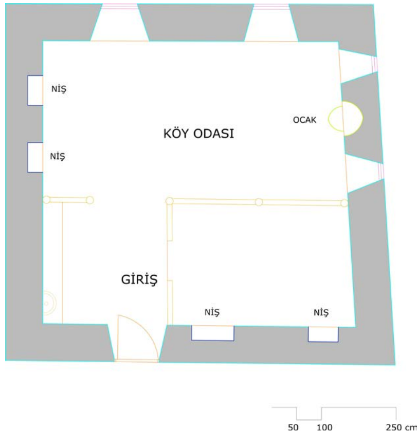
Şekil 3. 57 Aşağı Oda'nın planı
