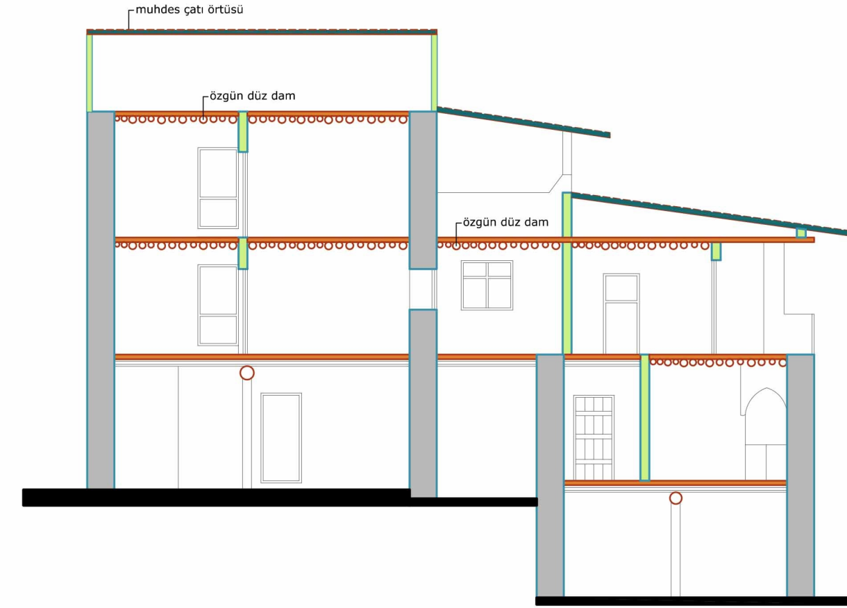
B - B' KESİTİ
