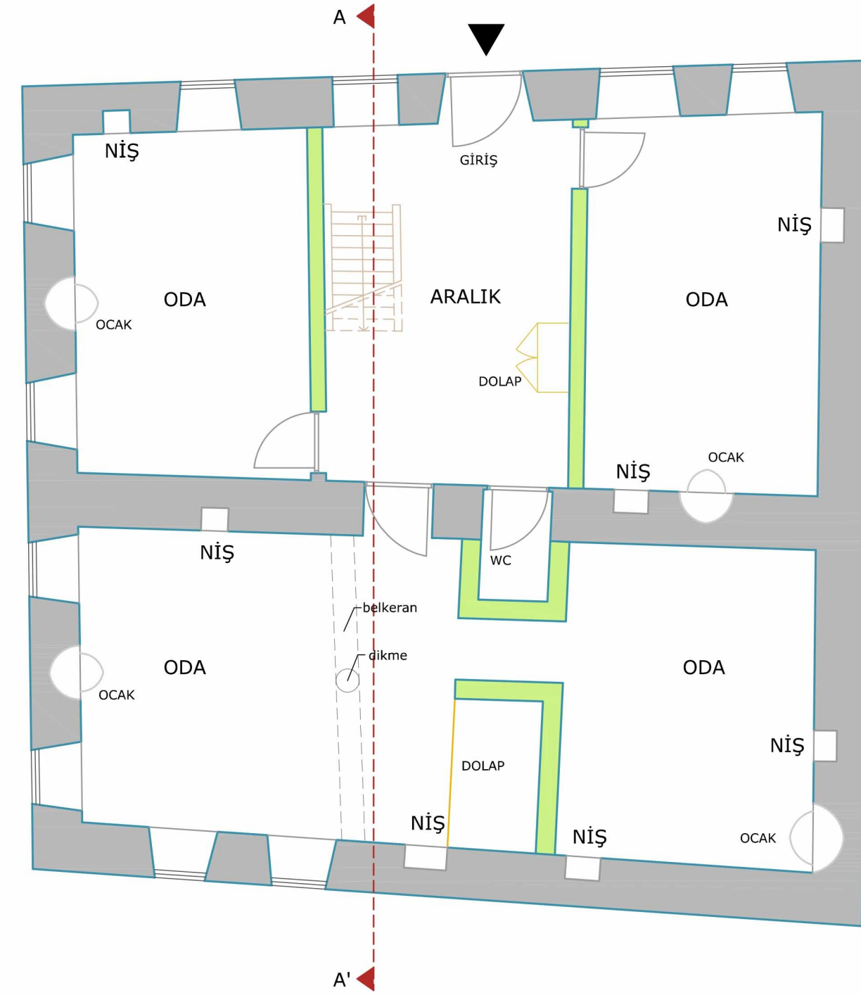
1. KAT PLANI
