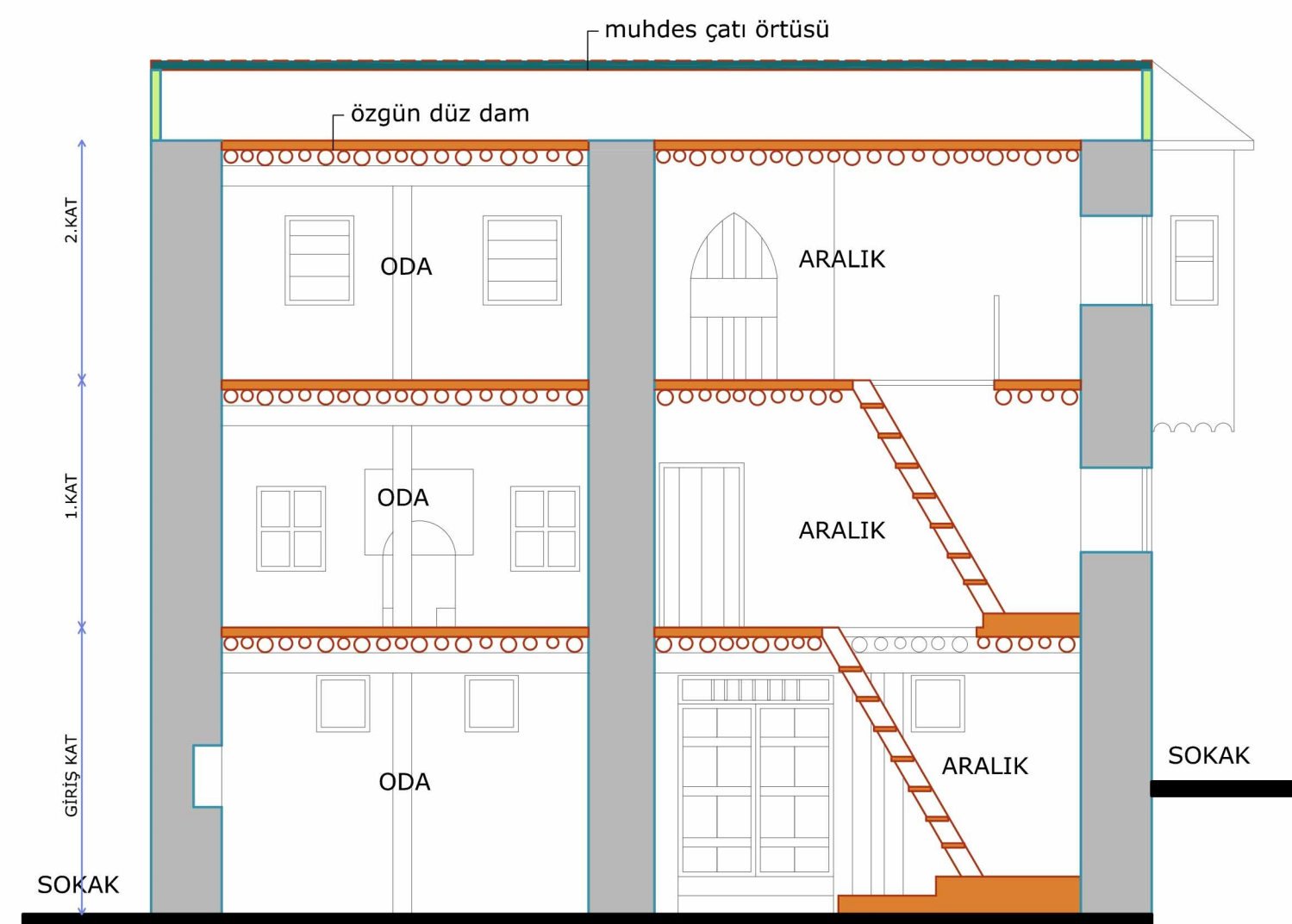
A - A' KESİTİ
