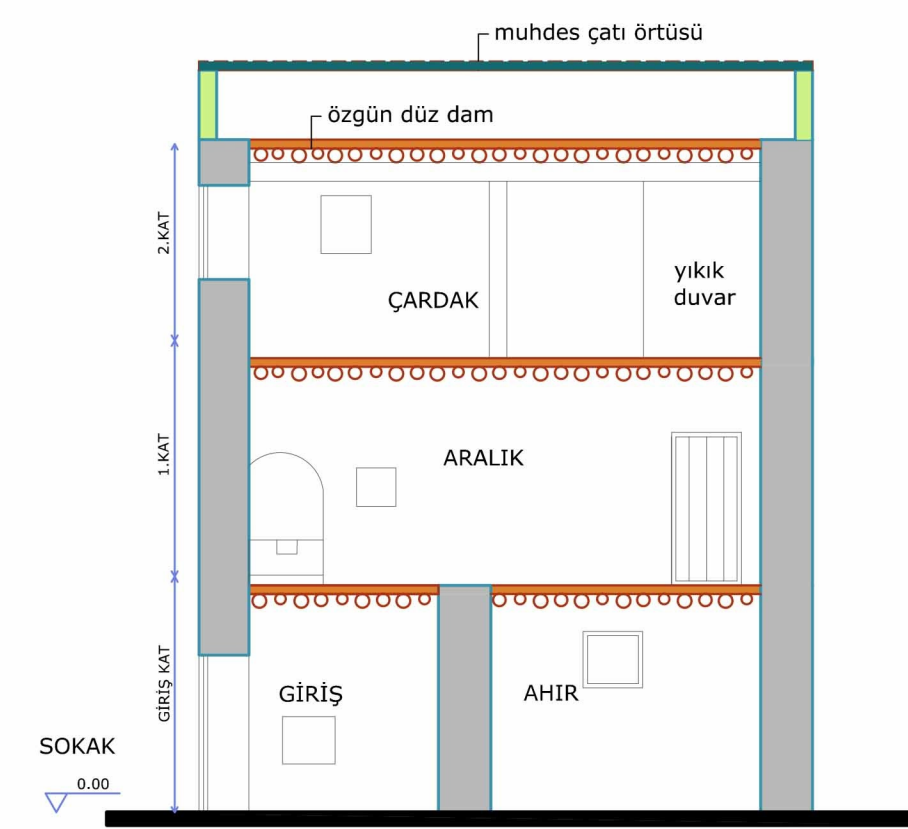
B - B' KESİTİ
