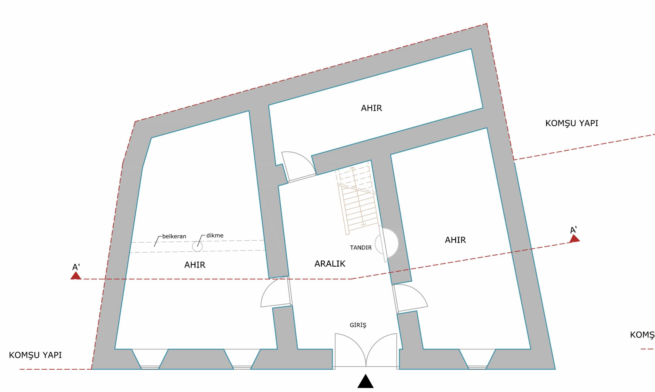
ZEMİN KAT PLANI
