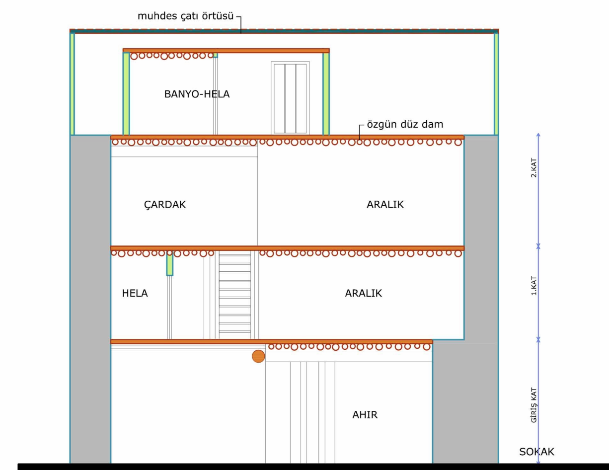
B-B' KESİTİ
