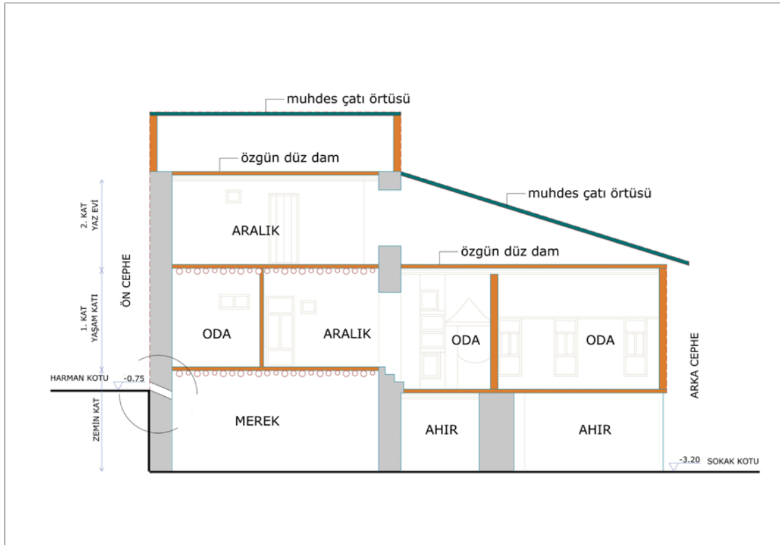
Şekil 5. 9 Harman kotunun altında tek kat olan konut (Envanter no: 262-8)
