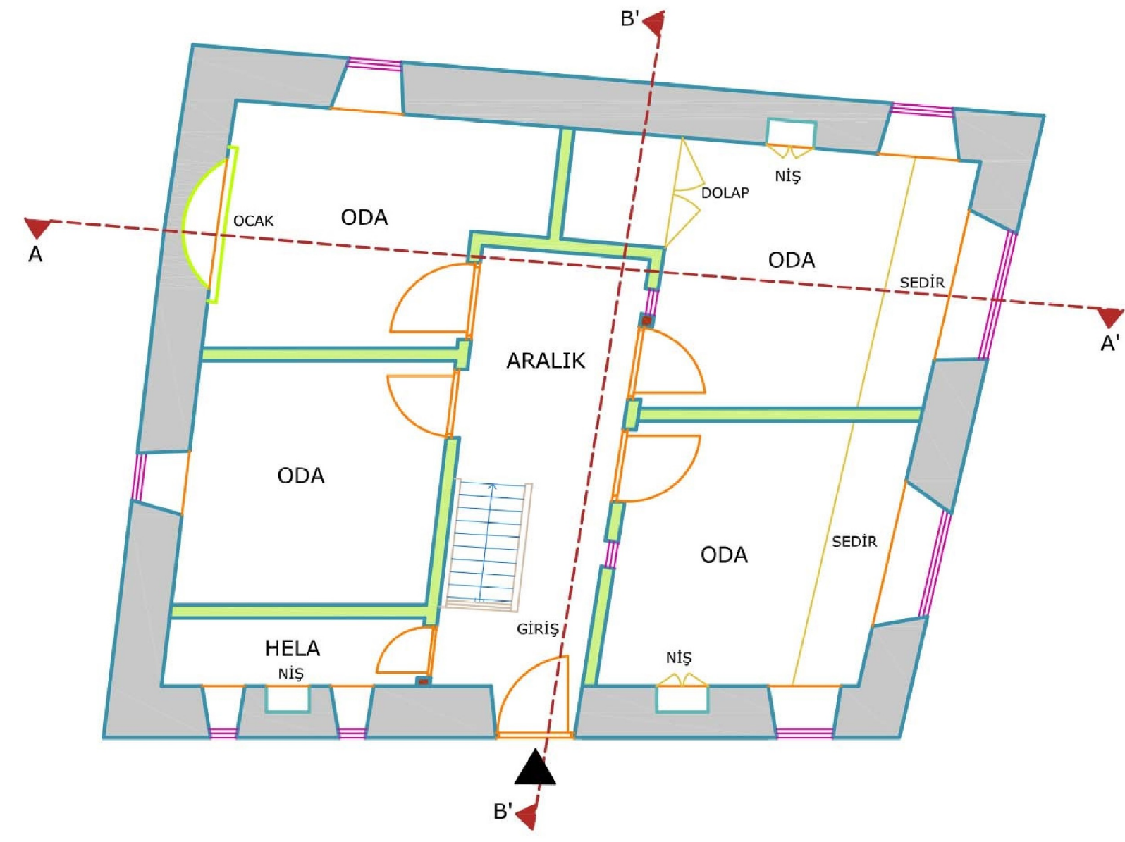
1. KAT PLANI
