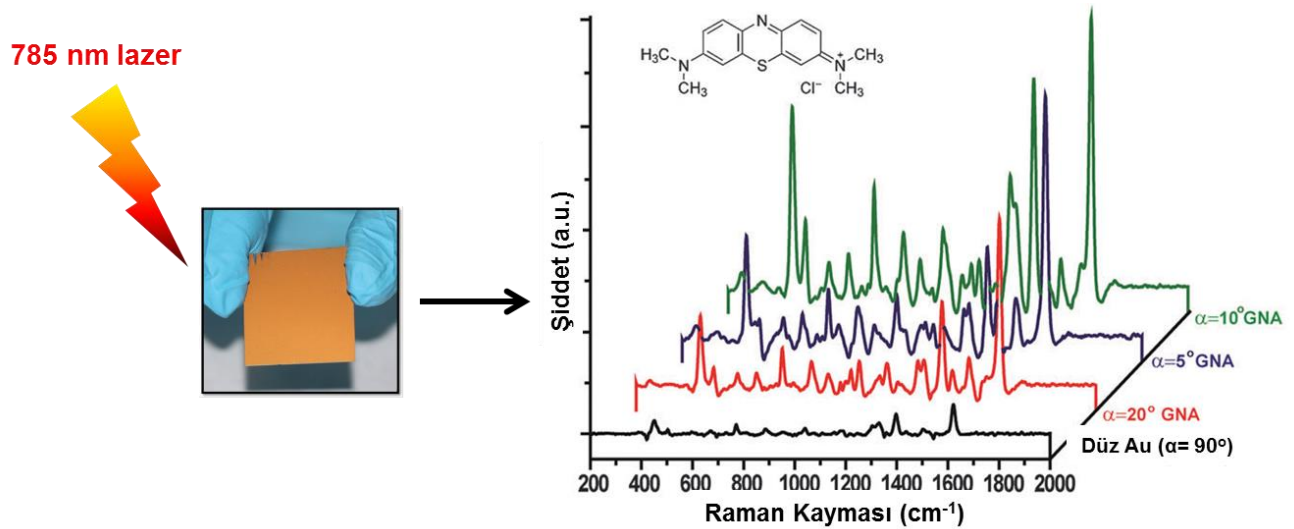
Şekil 4.35. 10 μM MB için elde edilen SERS spektraları: GNA nanoyapılar için buhar akısı açısının (α) elde edilen SERS spektrası üzerine etkisi.
