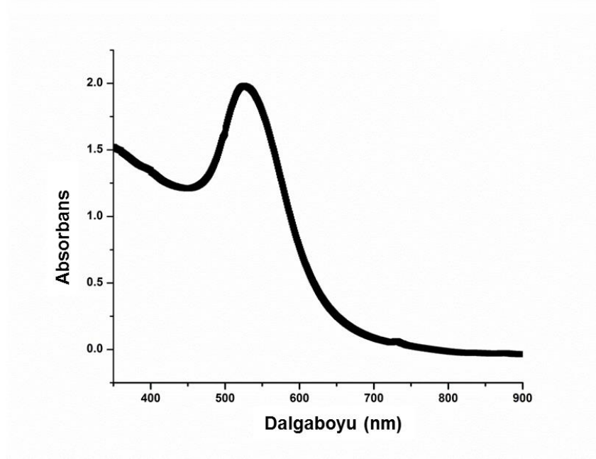
Şekil 4.7. Sitrat indirgeme yöntemiyle elde edilen AuNP örneğinin UV-vis spektrumu AuNR sentezinde ayrıntıları Dr. El-Sayed tarafından geliştirilen iki aşamalı sentez protokolü temel alınmıştır [149]. Bu kapsamda sentezlenen AuNR örneklerinin farklı büyütme ölçeklerindeki TEM görüntüleri ve çapa ve boya göre partikül boyut dağılım grafikleri
