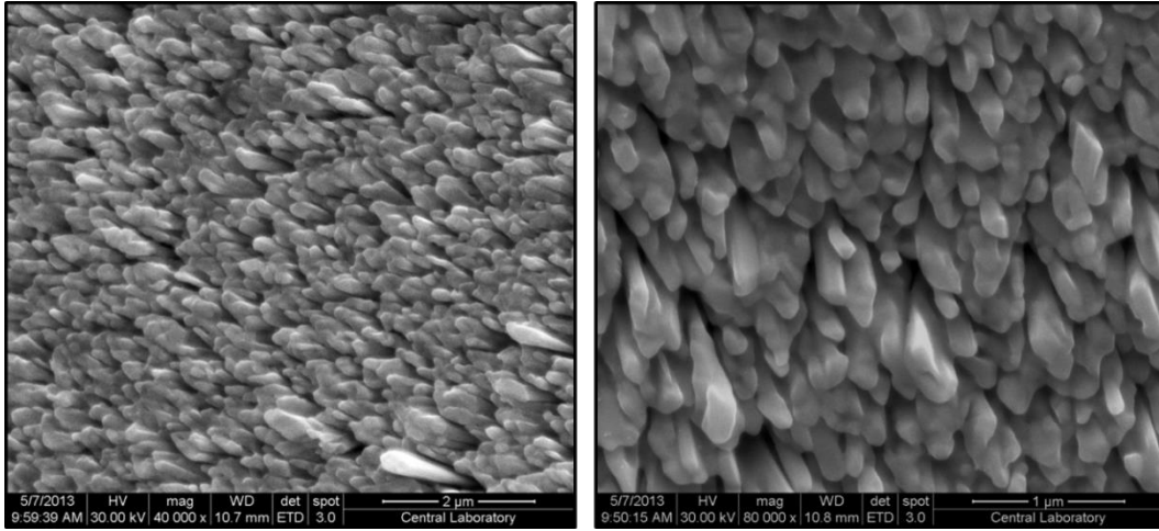
Şekil 4.23. 10° buhar akısı açısında ( \alpha ) üretilen anizotropik GNA nanoçubuk yapıların farklı büyütme ölçeklerinde üstten çekilmiş SEM görüntüleri.
