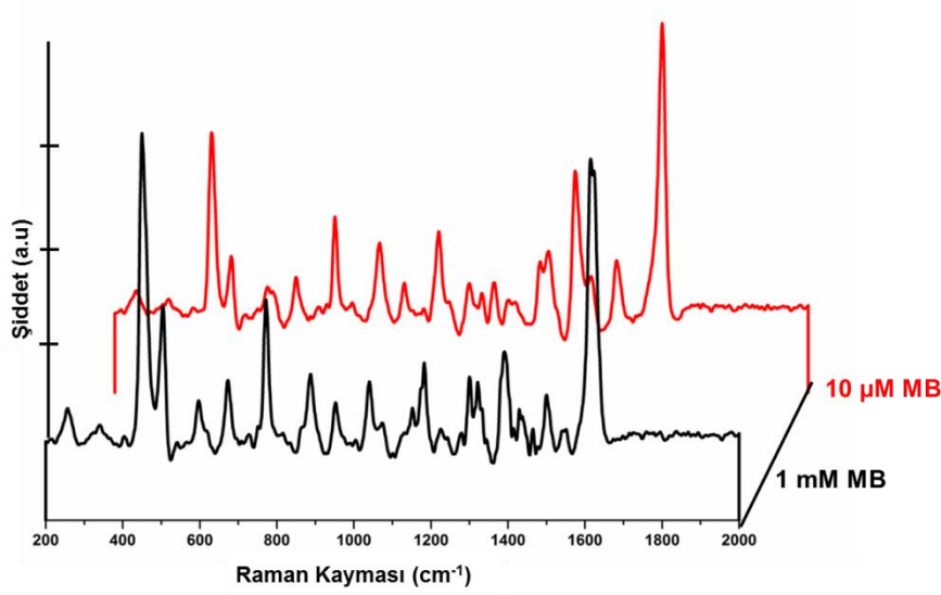
Şekil 4.34. Farklı derişimlerdeki MB için elde edilen SERS spektraları (GNA, \alpha = 10^\circ ).
