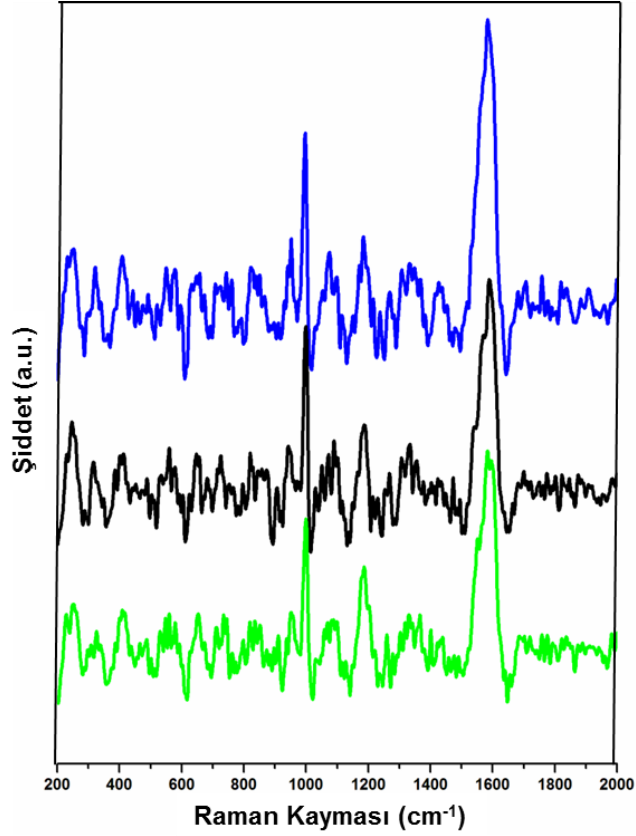
Şekil 4.48. Altın kaplandıktan sonra (32 nm) tek tabaka PS mikrokürelerden (~5 \mu\text{m} ) elde edilen 10 \mu\text{M} MB SERS spektralleri.
