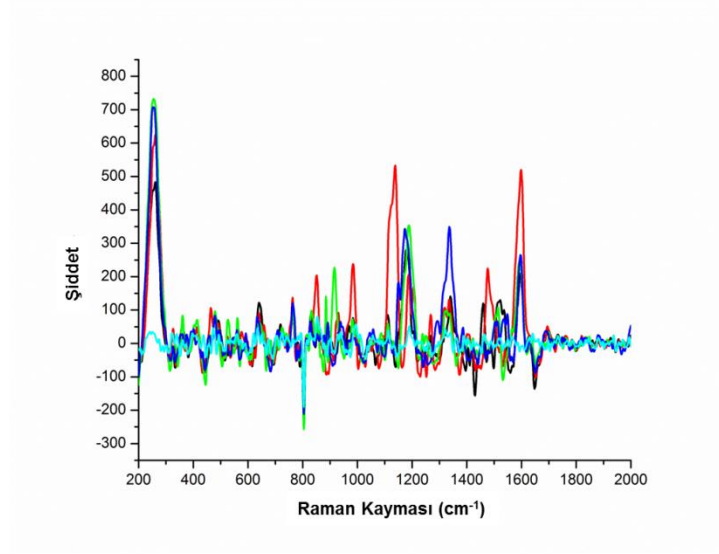
Şekil 4.58. FITC boyalı albumin (1 \mu\text{M} ) ile modifiye edilmiş GNAs nanoçubuk yüzeyden elde edilen SERS spektraları ( \alpha = 10^\circ ).
