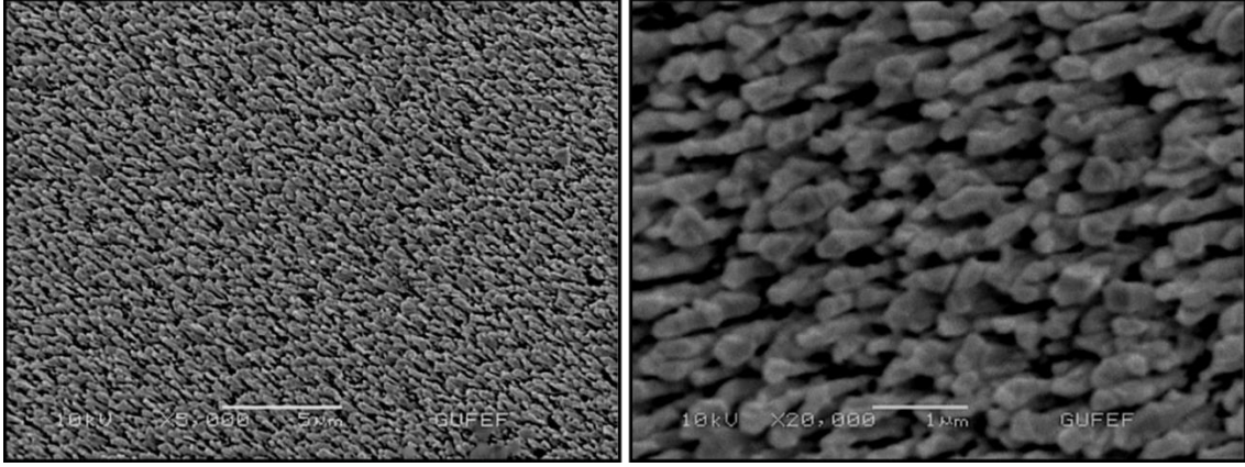
Şekil 4.22. 5° buhar akısı açısında ( \alpha ) üretilen anizotropik GNA nanoçubuk yapıların farklı büyütme ölçeklerinde üstten çekilmiş SEM görüntüleri.
