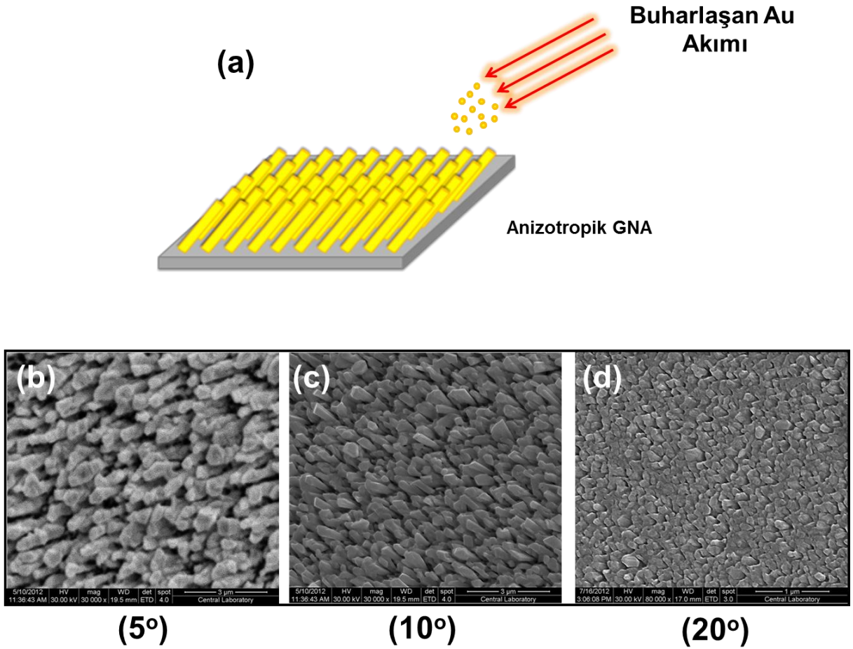
Şekil 4.21. Eğik açı vakum biriktirme tekniği ile anizotropik GNA ya da SNA nanotel yapıların oluşum mekanizması (a). ve (b, c ve d) farklı buhar akısının açısı ( \alpha ) degerleri için elde edilen GNA nanoyapıların üstten SEM görüntüleri.
