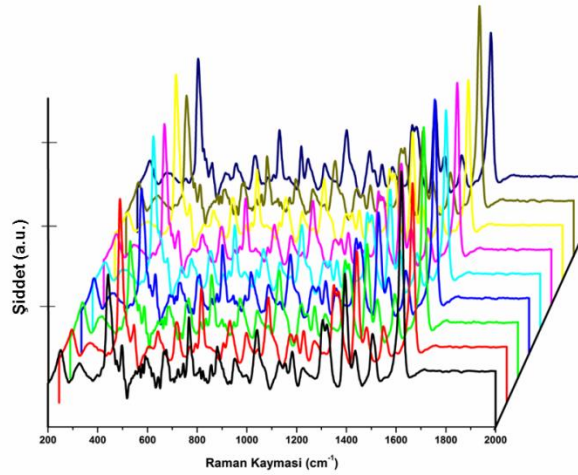
Şekil 4.55. 10 \mu M MB için elde edilen tekrarlanabilir SERS spektraları ( \alpha=10^0 ve 20 ppm AgNR).
