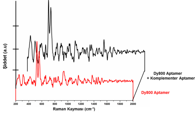
Şekil 4.63. Komplementer aptamerinin Dy800-aptamer ile modifiye edilmiş GNA nanoçubukların ( \alpha = 10^0 ) SERS spektrası üzerine etkisi.
