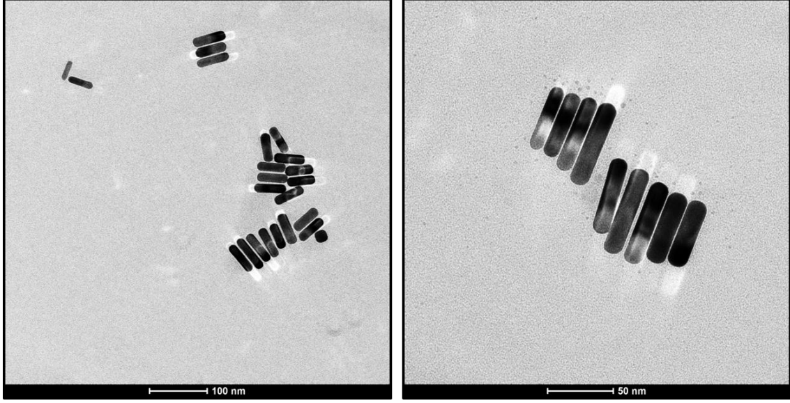
Şekil 4.8. Elde edilen AuNR örneğinin farklı büyütmelelerdeki TEM görüntüleri
