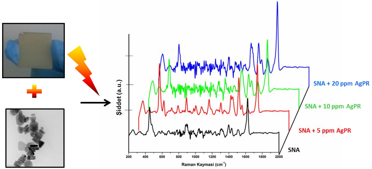
Şekil 4.51. 10 \mu\text{M} MB için elde edilen SERS spektraları: AgPR ile kombine/dekore edilmiş SNA nanoçubuklar ( \alpha = 10^0 ) ve elde edilen SERS spektrası üzerine nanopartikül derişiminin etkisi.
