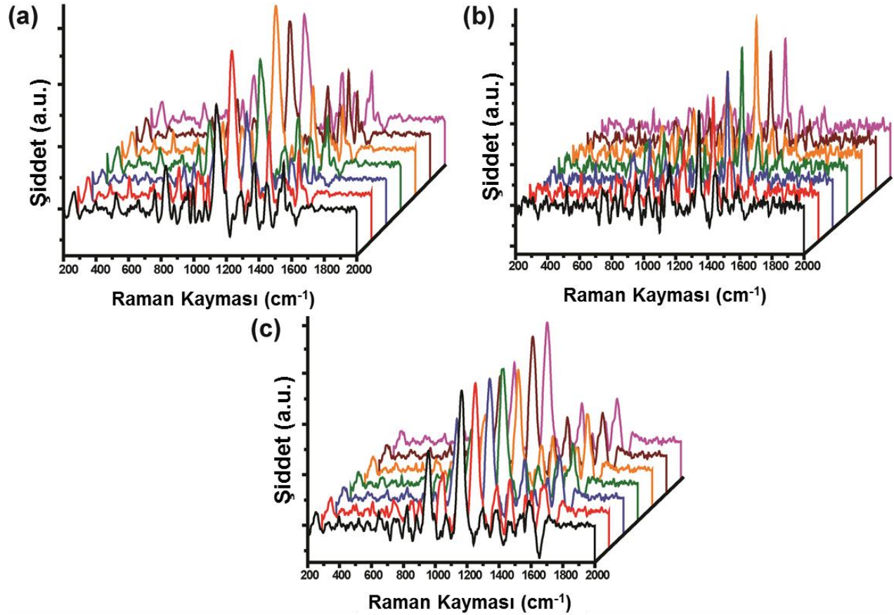
Şekil 4.45. 5 ppm DIP (a), MP (b) ve DP (c) için tekrarlanabilir SERS spektraları ( \alpha = 10^\circ ve 20 ppm AuNR).
