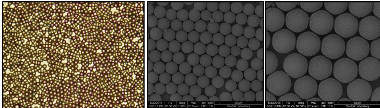
Şekil 4.47. PVD yöntemi ile altın kaplandıktan sonra (32 nm) tek tabaka PS mikrokürelerin (~5 \mu\text{m} ) optik mikroskop ve farklı büyütme ölçeklerindeki SEM görüntüleri.
