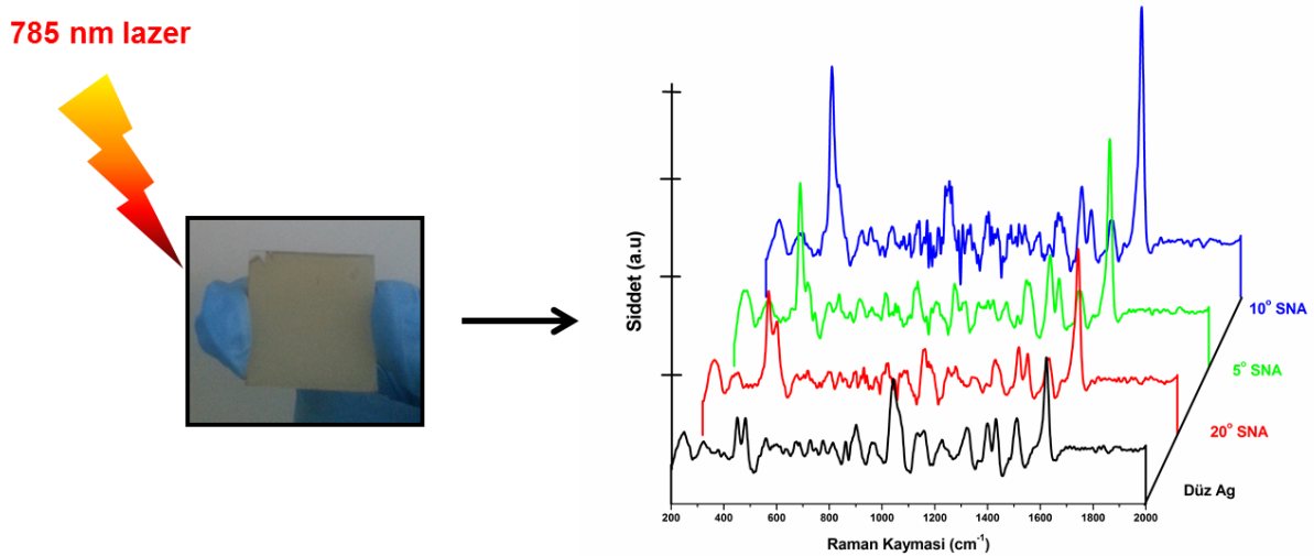
Şekil 4.49. 10 µM MB için elde edilen SERS spektraları: SNA nanoyapılar için buhar akısı açısının ( \alpha ) elde edilen SERS spektrası üzerine etkisi.
