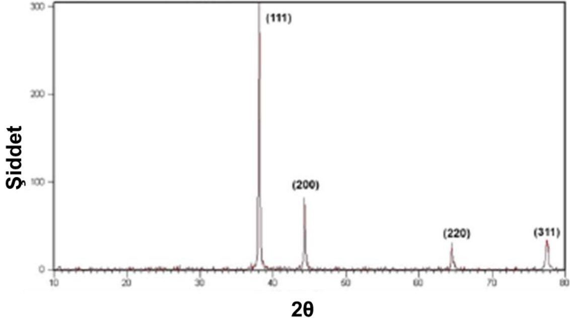
Şekil 4.26. 10^\circ buhar akısı açısında ( \alpha ) üretilen anizotropik GNA nanoçubuk yapıların XRD desenleri.
