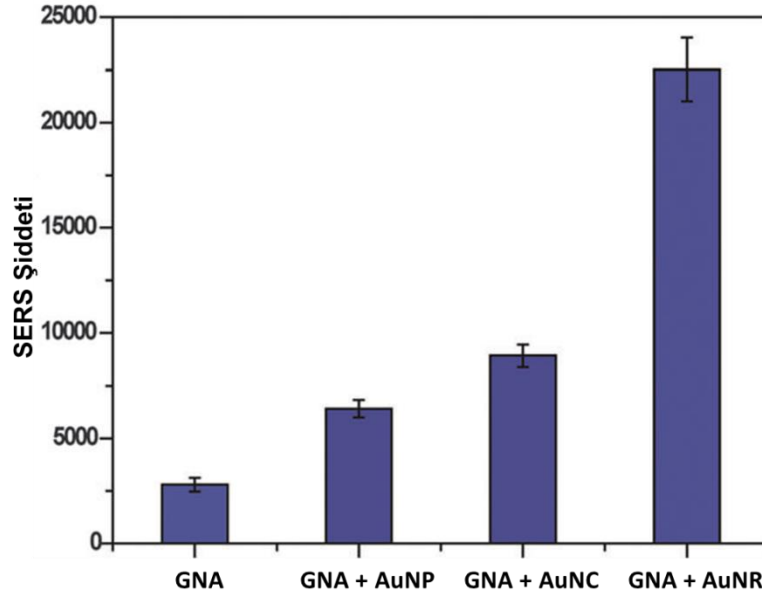
Şekil 4.39. Farklı nanopartiküller ile kombine/dekore edilmiş GNA nanoçubukların ( \alpha=10^0 ) 10 \mu M MB ve 20 ppm nanopartikül derişimi için SERS şiddetlerinin karşılaştırılması.
