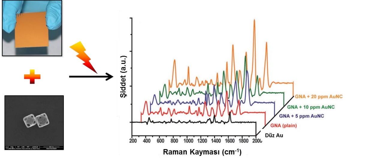
Şekil 4.37. 10 \mu\text{M} MB için elde edilen SERS spektraları: AuNC ile kombine/dekore edilmiş GNA nanoçubuklar ( \alpha = 10^0 ) ve elde edilen SERS spektrası üzerine nanopartikül derişiminin etkisi.
