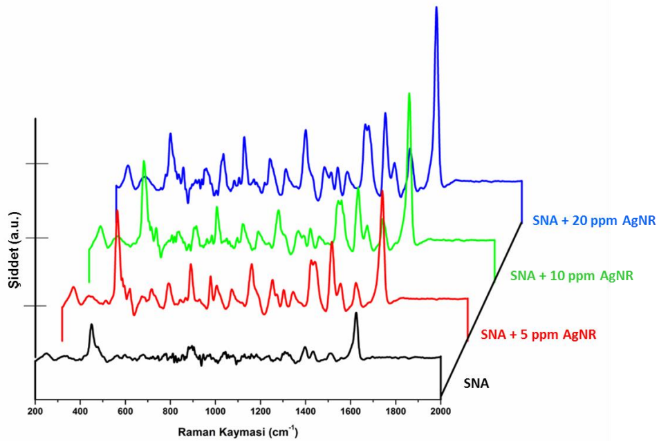
Şekil 4.52. 10 \mu\text{M} MB için elde edilen SERS spektraları: AgNR ile kombine/dekore edilmiş SNA nanoçubuklar ( \alpha = 10^0 ) ve elde edilen SERS spektrası üzerine nanopartikül derişiminin etkisi.
