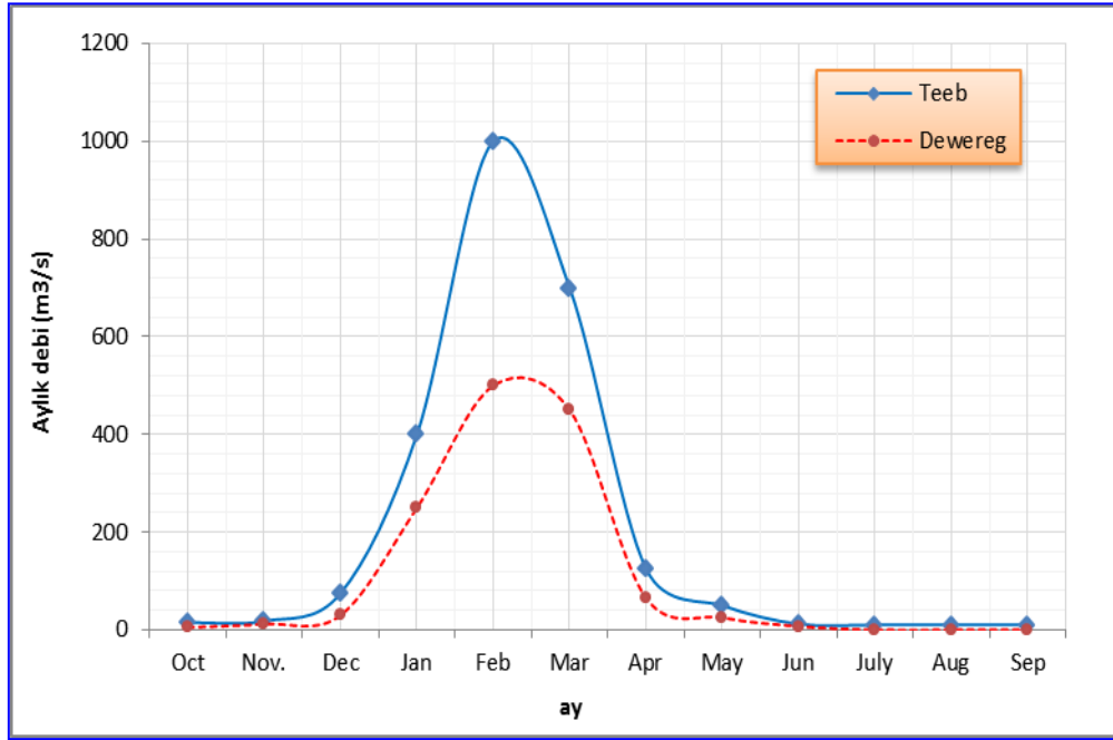
Şekil 4.8. Çalışma alanındaki Teeb ve Dewereg aylık ortalama debi hidrografı.
