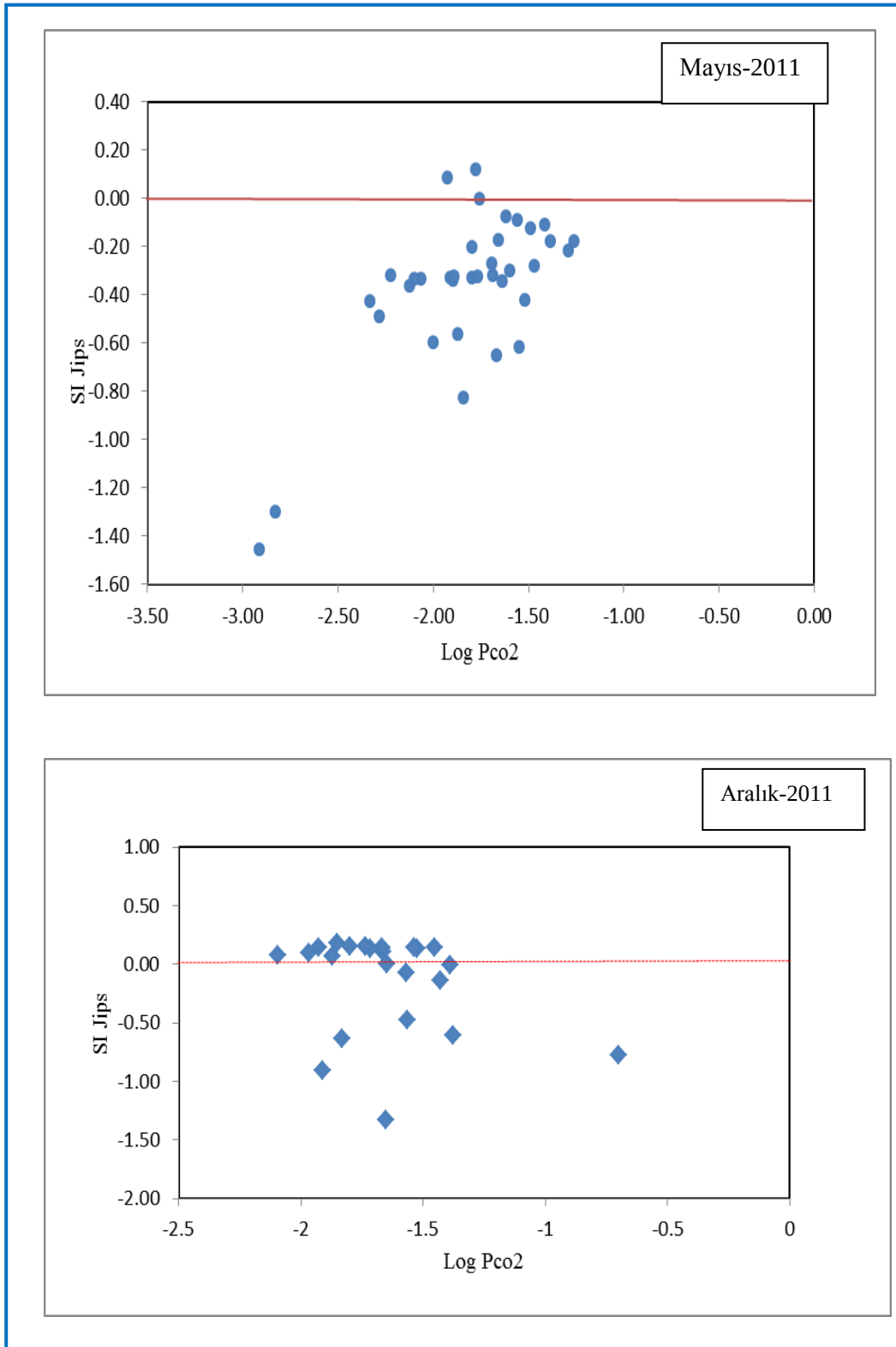
Şekil 4.42. Çalışma alanındaki yeraltı sularının LogPco 2 - SI Jips ilişkisi ve doygunluk bölgeleri diyagramı
