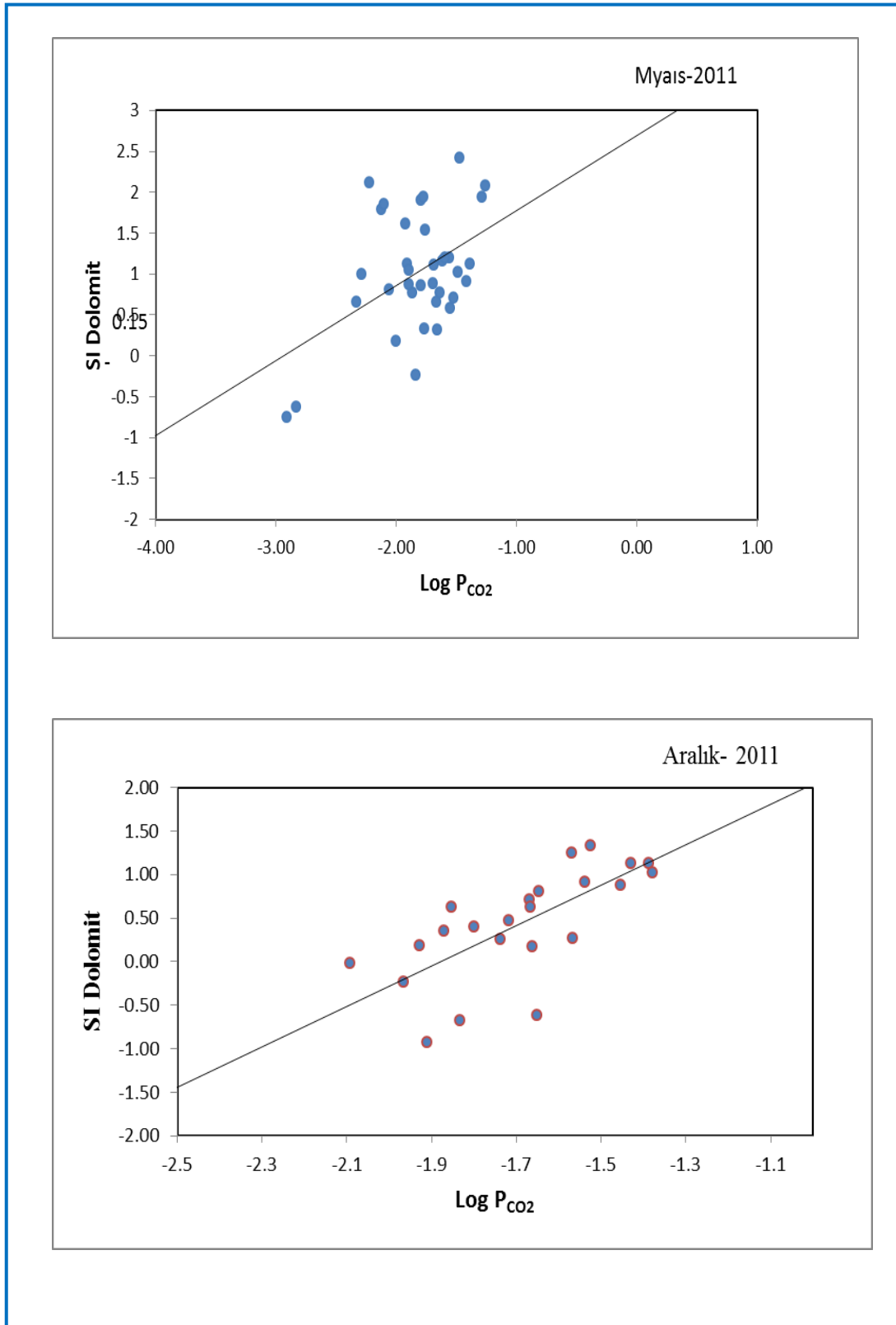
Şekil 4.47. Çalışma alanındaki yeraltı sularının \text{Log } P_{\text{CO}_2} -SI Dolomit ilişkisi diyagramı
