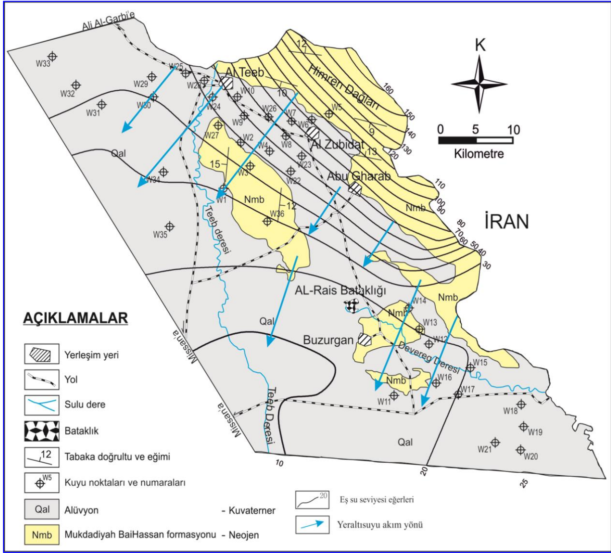
Şekil 4.17. Yeraltı suları seviyesi ve ana akifere göre yönleri
