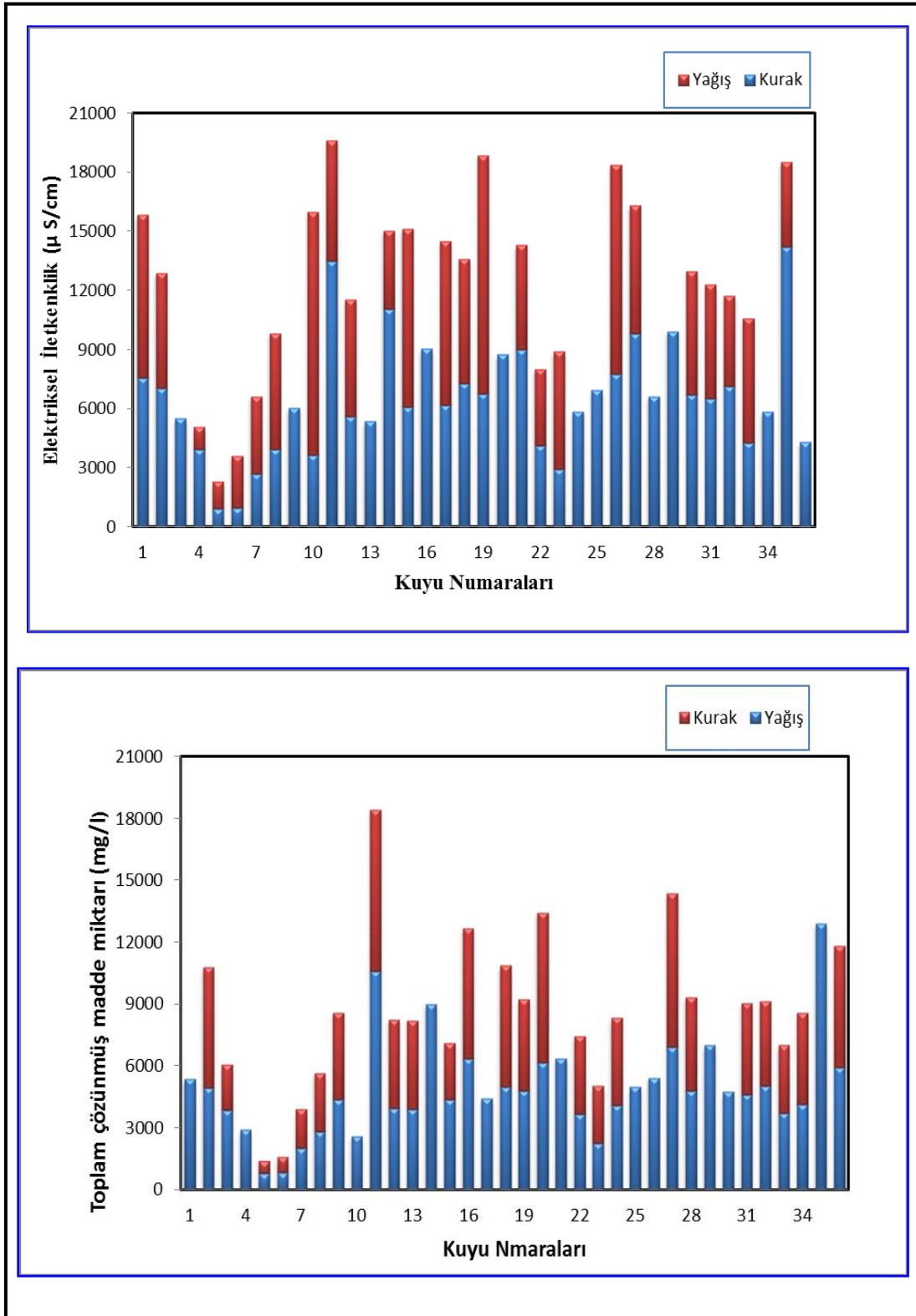
Şekil 4.21. Çalışma alanındaki yeraltı sularının EC ve TDS konsantrasyonları
