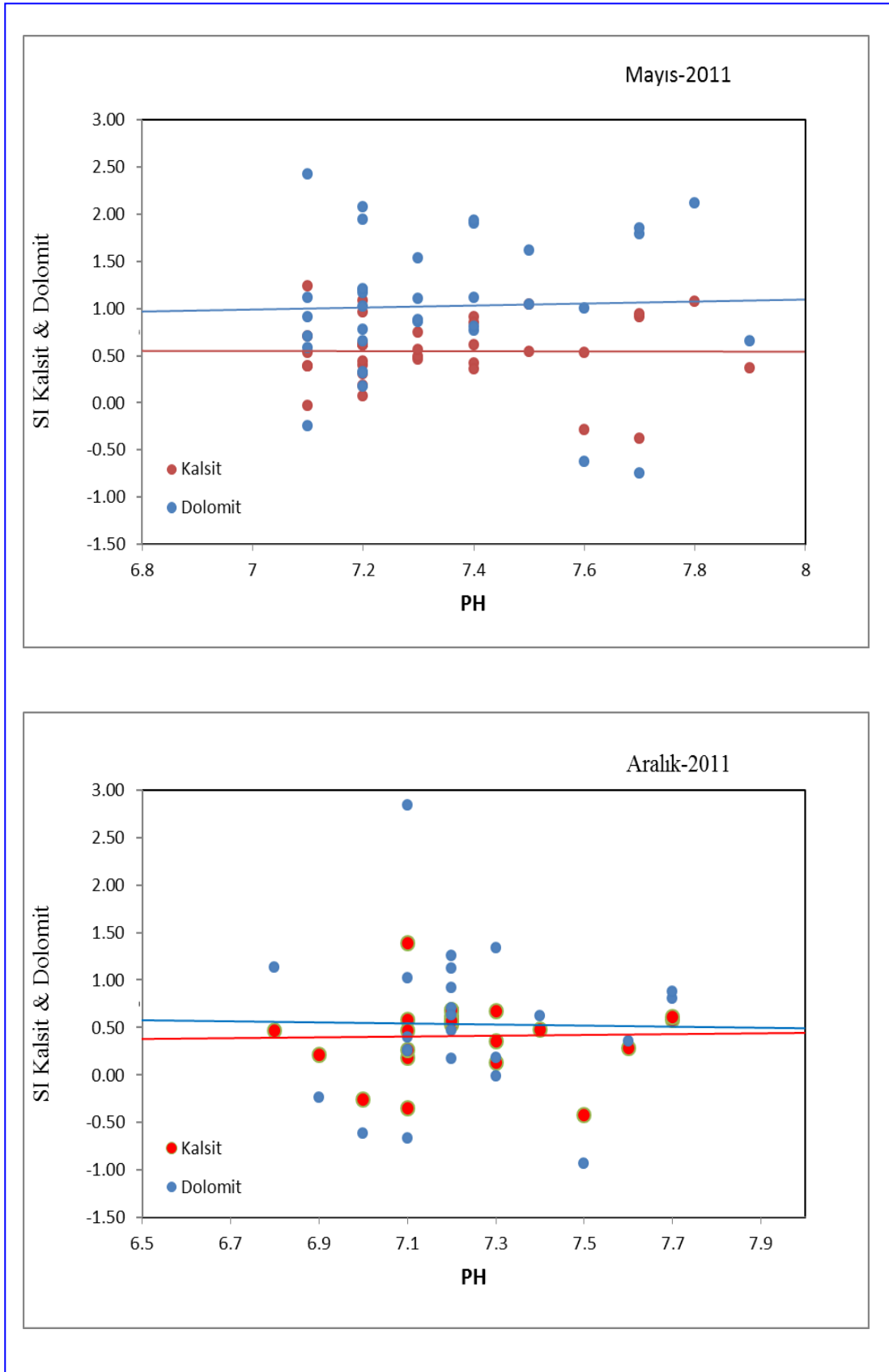
Şekil 4.55. Çalışma alanındaki yeraltı sularının pH - SI Kalsit & Dolomit ilişkisi diyagramı
