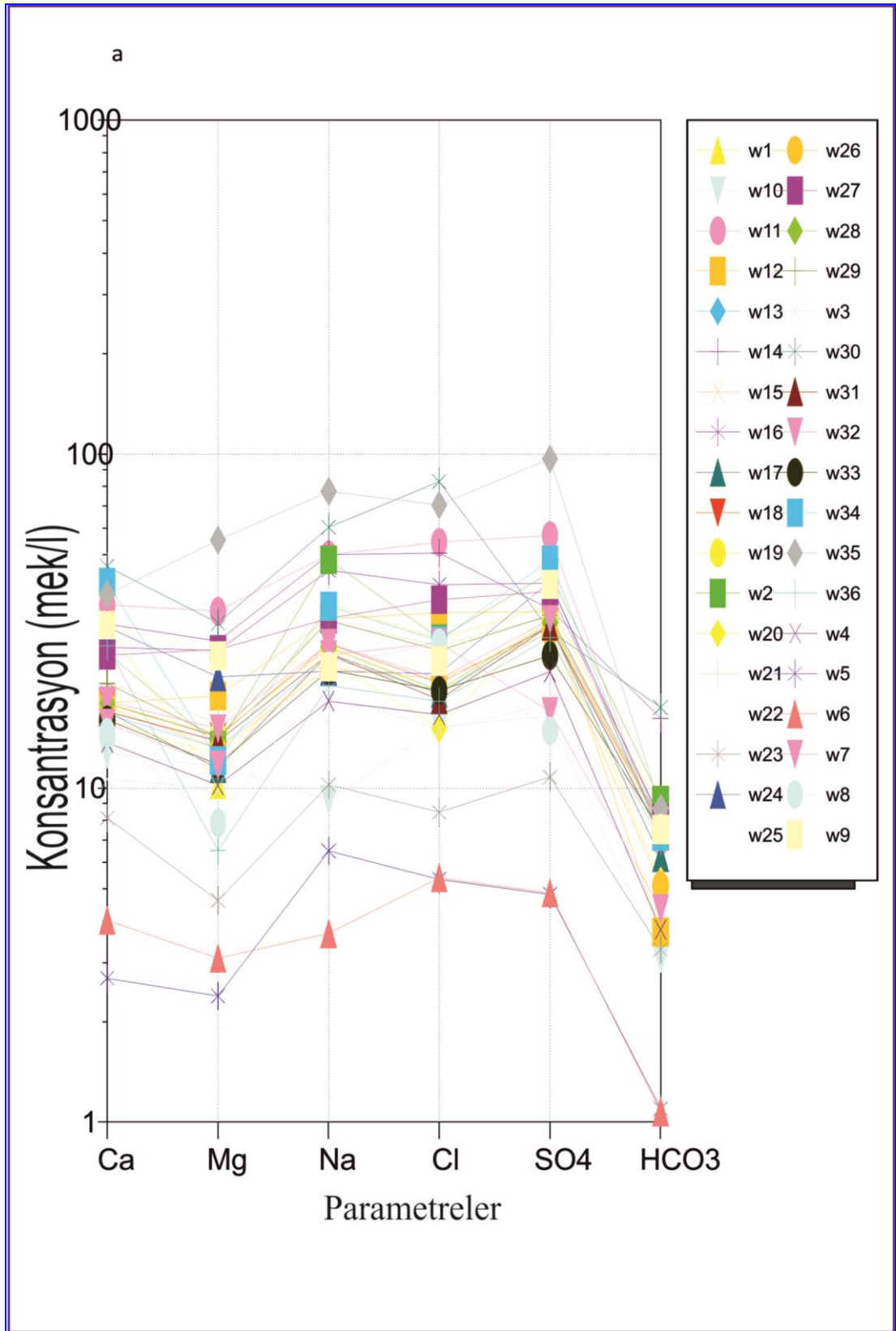
Şekil 4.33 a. Çalışma alanında yer alan yüzey ve yeraltı su örneklerinin Schoeller diyagramındaki konumları a: Kurak dönem (Mayıs 2011)
