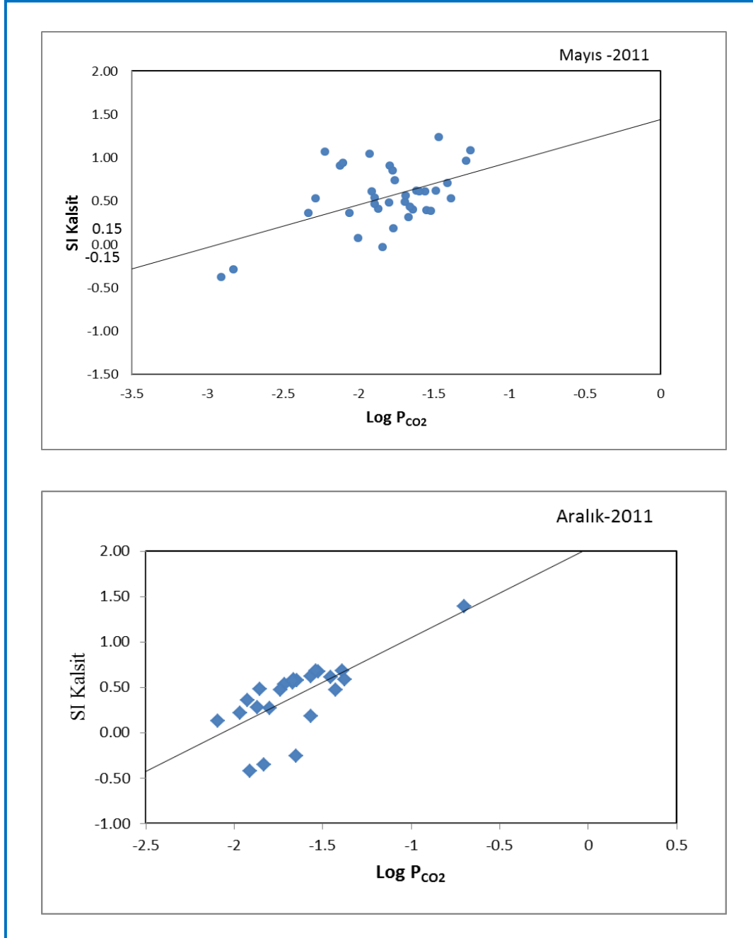
Şekil 4.46. Çalışma alanındaki yeraltı sularının \text{Log } P_{CO_2} - SI Kalsit ilişkisi diyagramı
