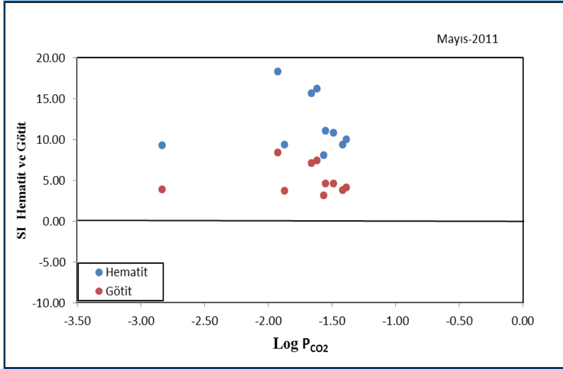
Şekil 4.45. Çalışma alanındaki yeraltı sularının LogPco 2 - SI (Hematit ve Götüt) ilişkisi ve doygunluk bölgeleri diyagramı
