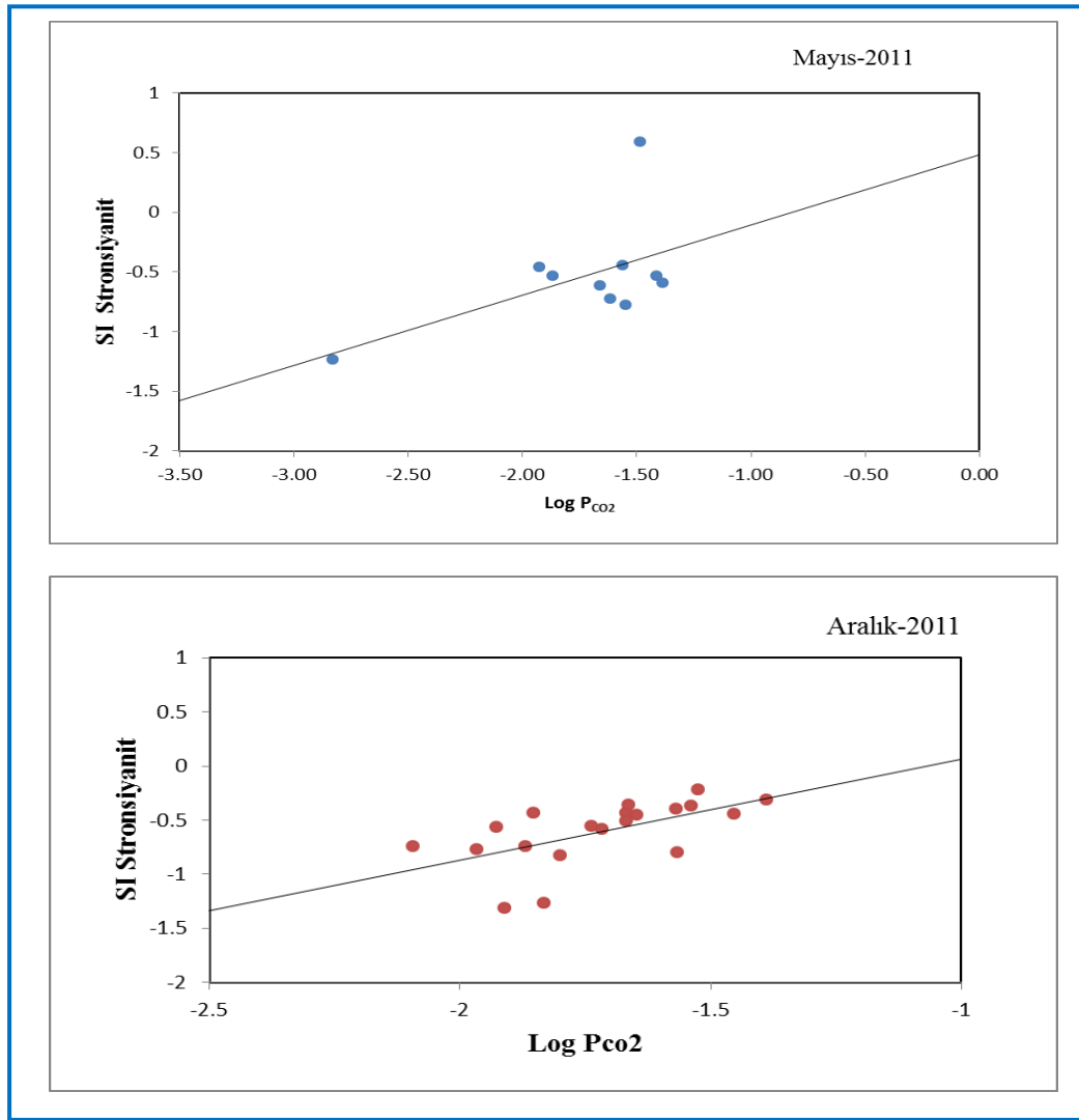
Şekil 4.49. Çalışma alanındaki yeraltı sularının \text{Log P}_{\text{CO}_2} -SI Stronsiyanit ilişkisi diyagramı
