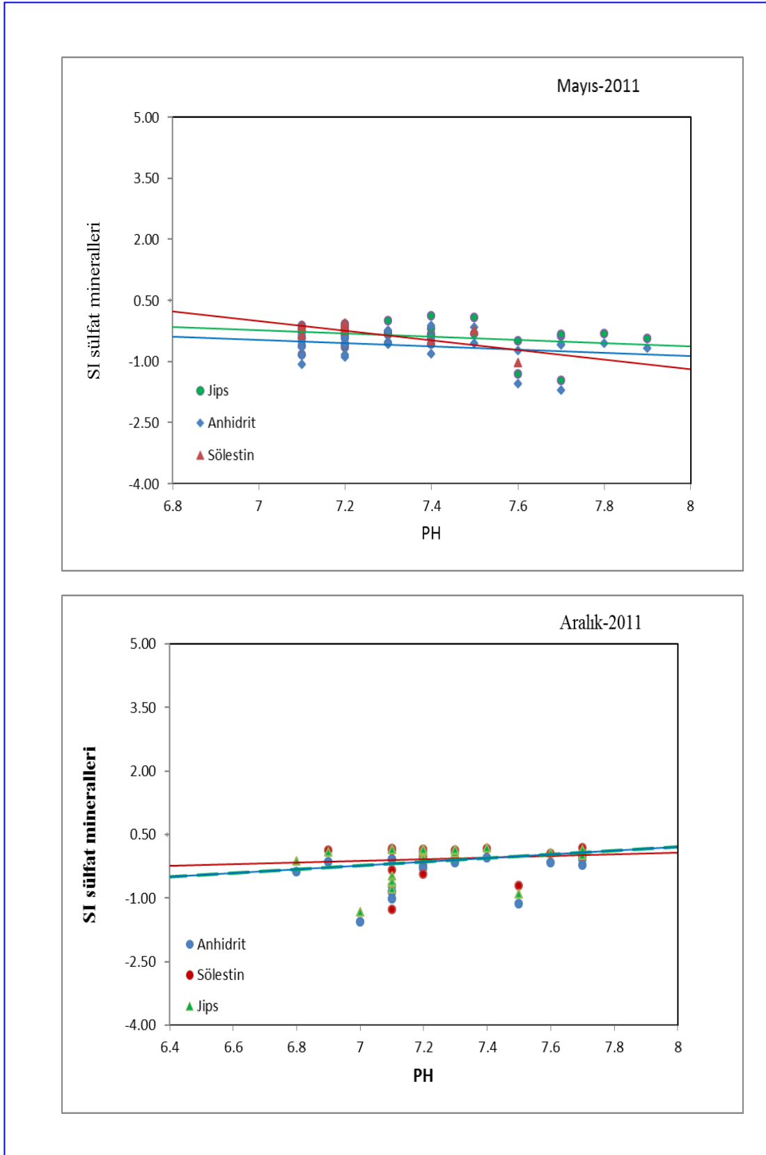
Şekil 4.57. Çalışma alanındaki yeraltı sularının pH-Sülfat mineral ilişkisi diyagramı
