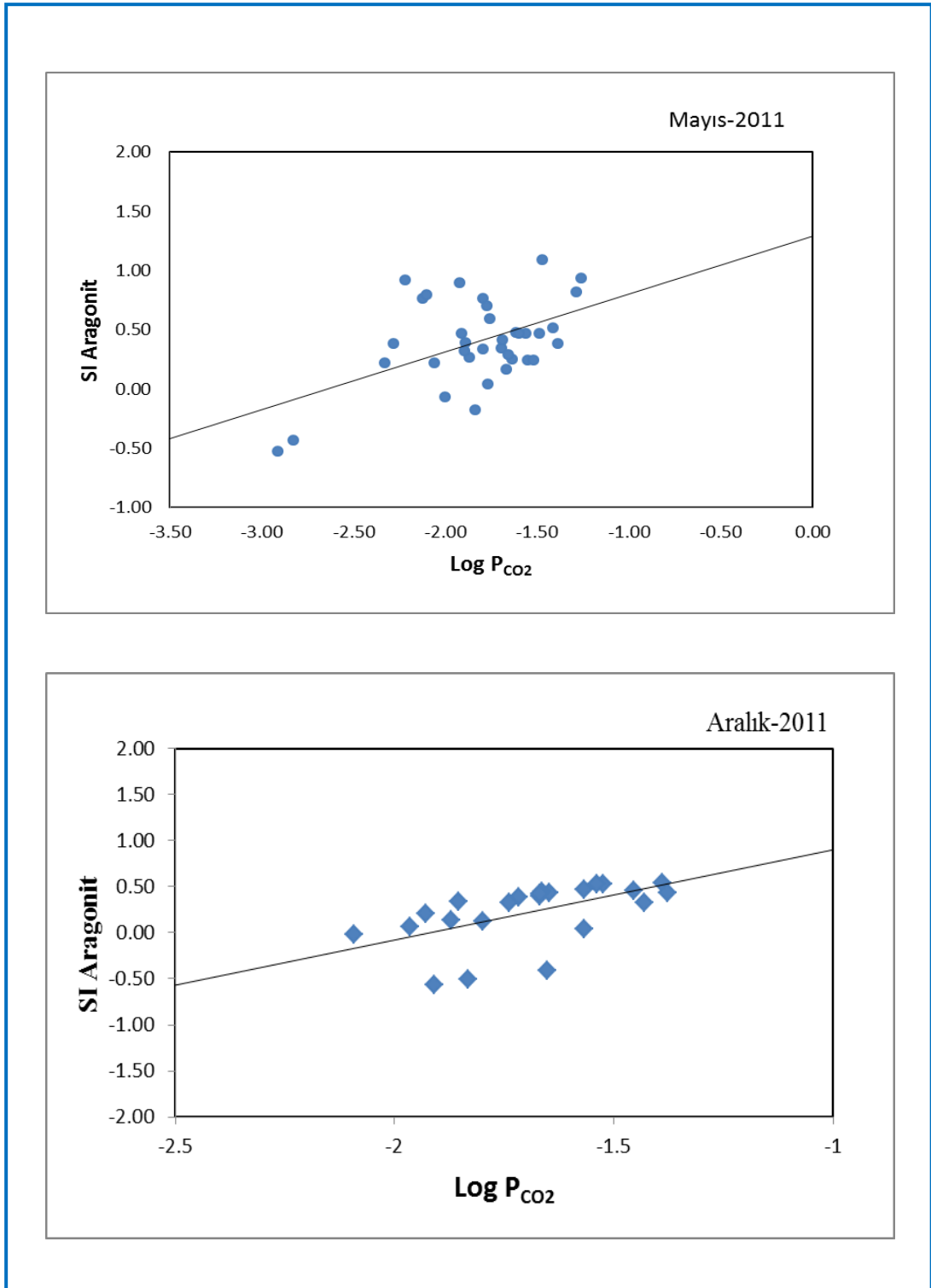
Şekil 4.48. Çalışma alanındaki yeraltı sularının \text{Log } P_{\text{CO}_2} -SI Aragonit ilişkisi diyagramı
