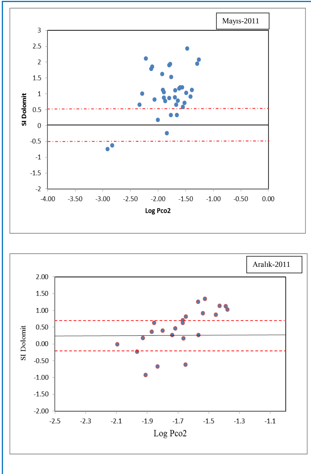
Şekil 4.39. Çalışma alanındaki yeraltı sularının LogPco 2 ve SI Dolomit ilişkisi ve doygunluk bölgeleri diyagramı
