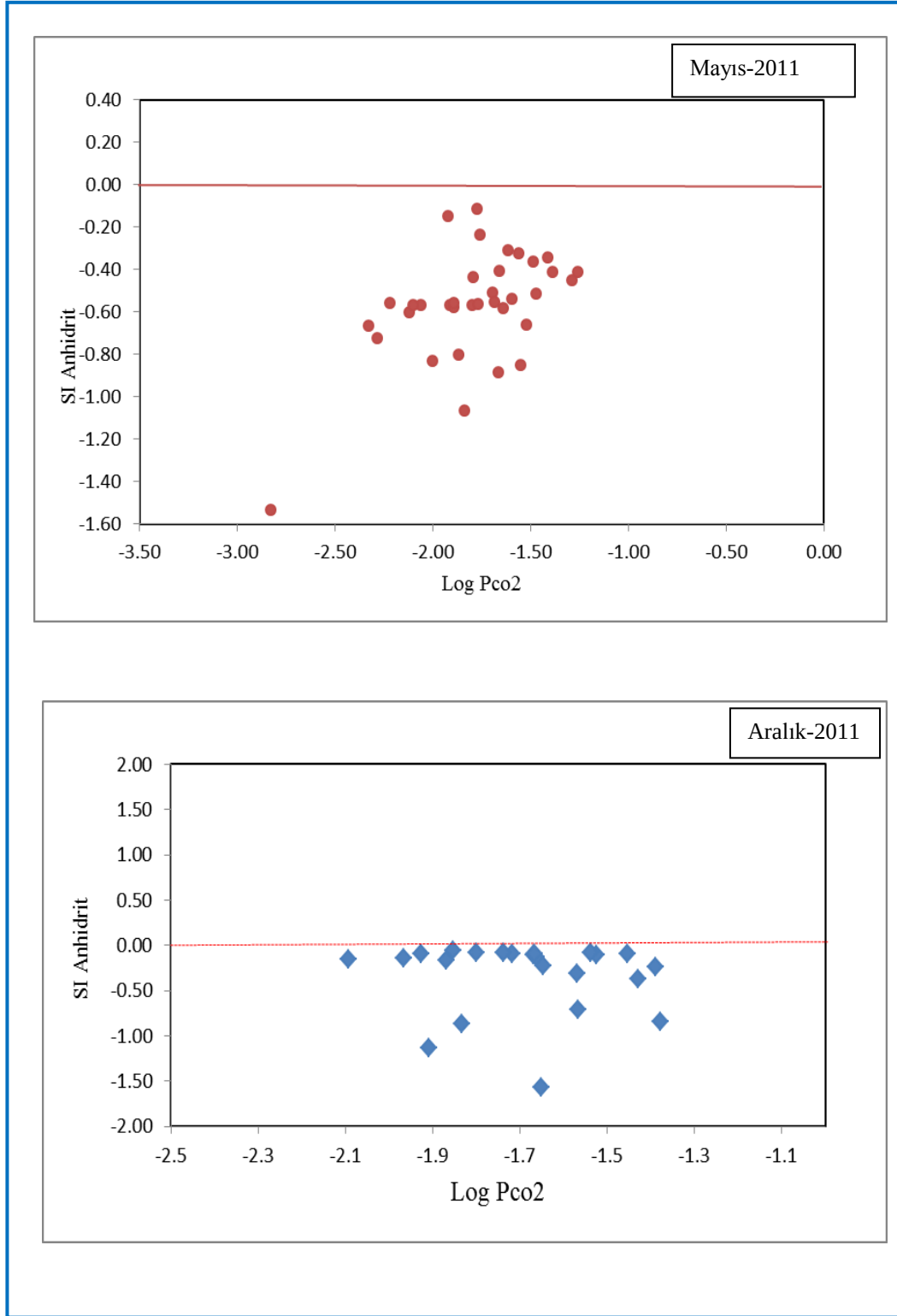
Şekil 4.43. Çalışma alanındaki yeraltı sularının LogPco 2 - SI Anhidrit ilişkisi ve doygunluk bölgeleri diyagramı
