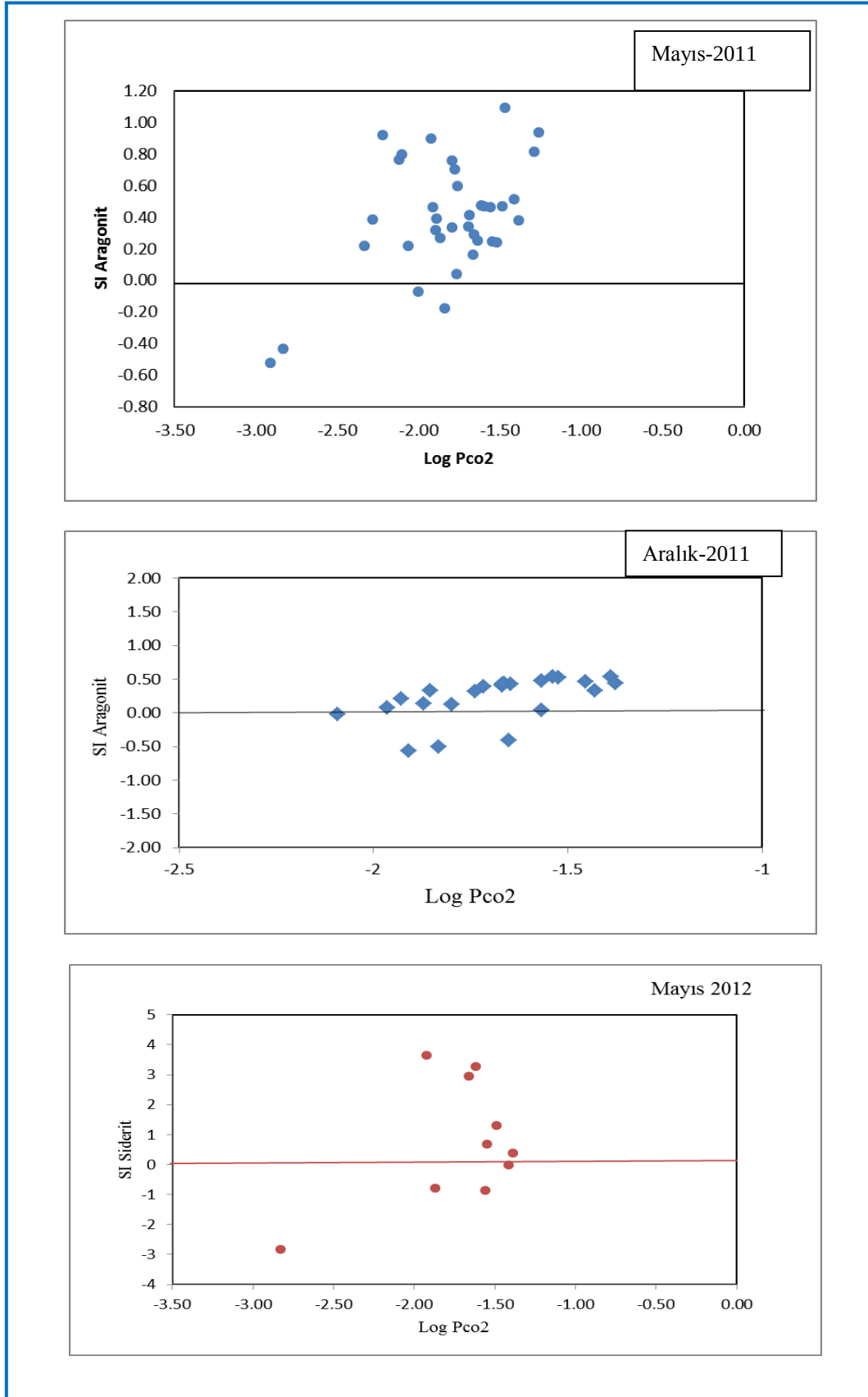
Şekil 4.40. Çalışma alanındaki yeraltı sularının \text{LogP}_{\text{CO}_2} -SI Aragonit ile Siderit ilişkisi ve doygunluk bölgeleri diyagramı
