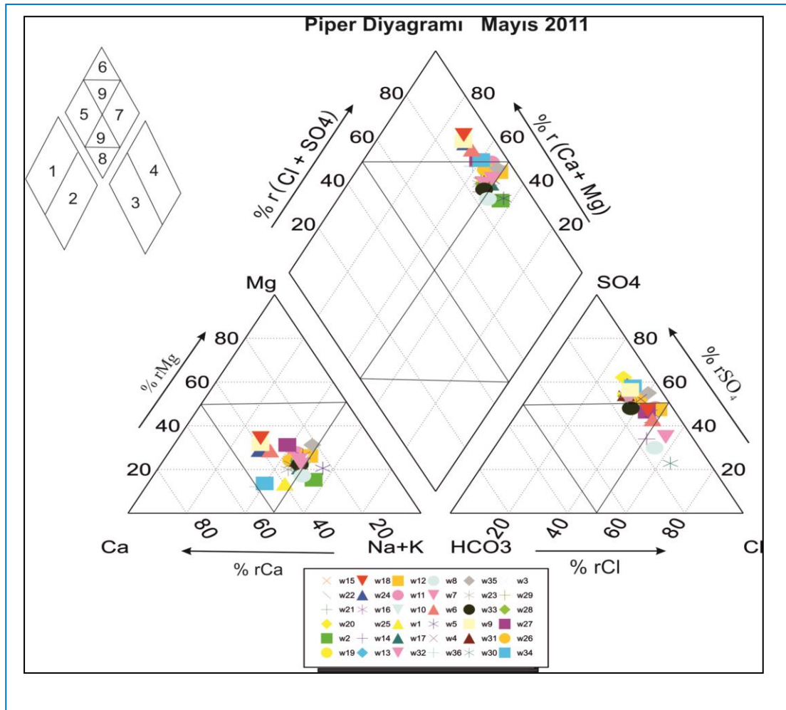
Şekil 4.34. Çalışma alanındaki su örneklerine ait Piper diyagram Mayıs 2011
