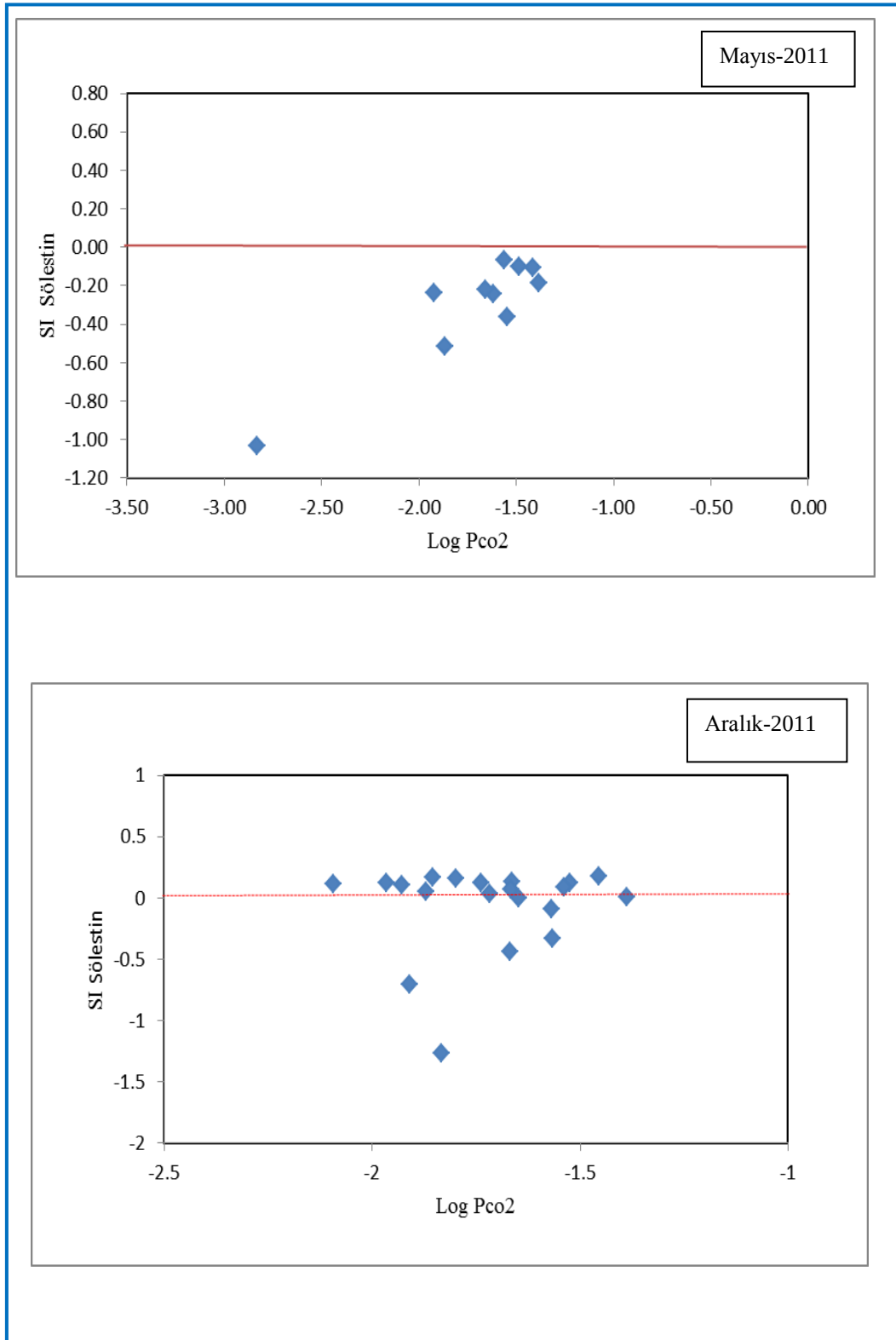
Şekil 4.44. Çalışma alanındaki yeraltı sularının LogPco 2 - SI Sölestin ilişkisi doygunluk bölgeleri diyagramı: Aralık
