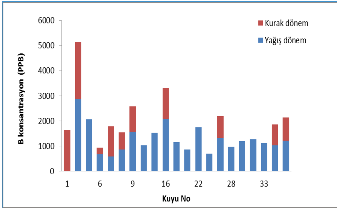
Şekil 4.31. Çalışma alanındaki yeraltı sularının bor konsantrasyonu
