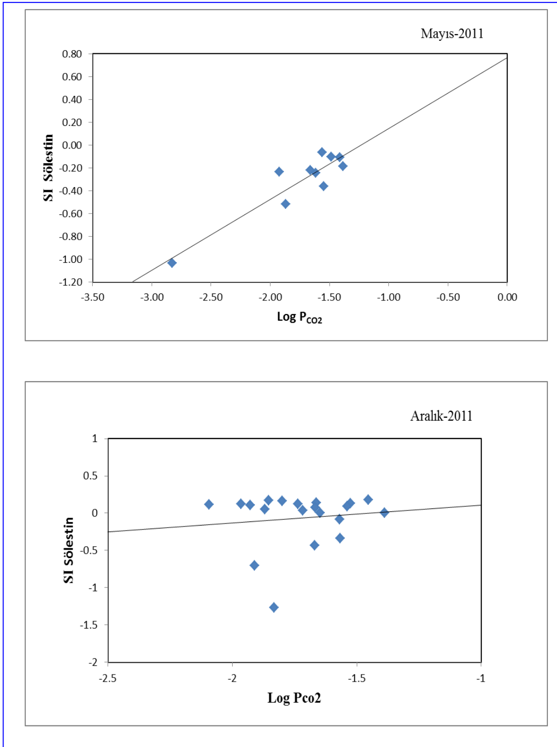
Şekil 4.53. Çalışma alanındaki yeraltı sularının \text{Log P}_{\text{CO}_2} -SI Sölestin ilişkisi diyagramı
