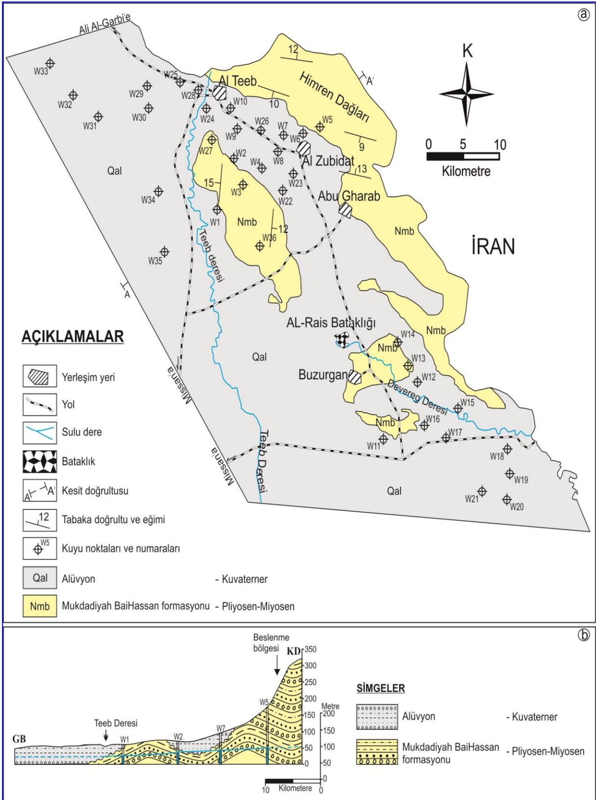
Şekil 4.9. Çalışma alanında seçilen hidrojeolojik kesitler
