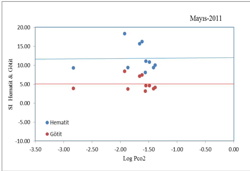
Şekil 4.54. Çalışma alanındaki yeraltı sularının \text{LogP}_{\text{CO}_2} -SI Hematit ve Götite ilişkileri diyagramı
