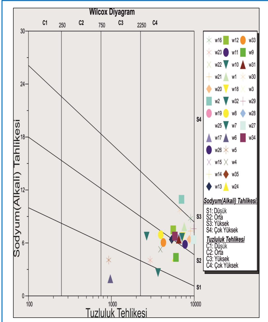
Şekil 4.36 a. Çalışma alanındaki su örneklerine ait Wilcox diyagramı a: Mayıs 20012
