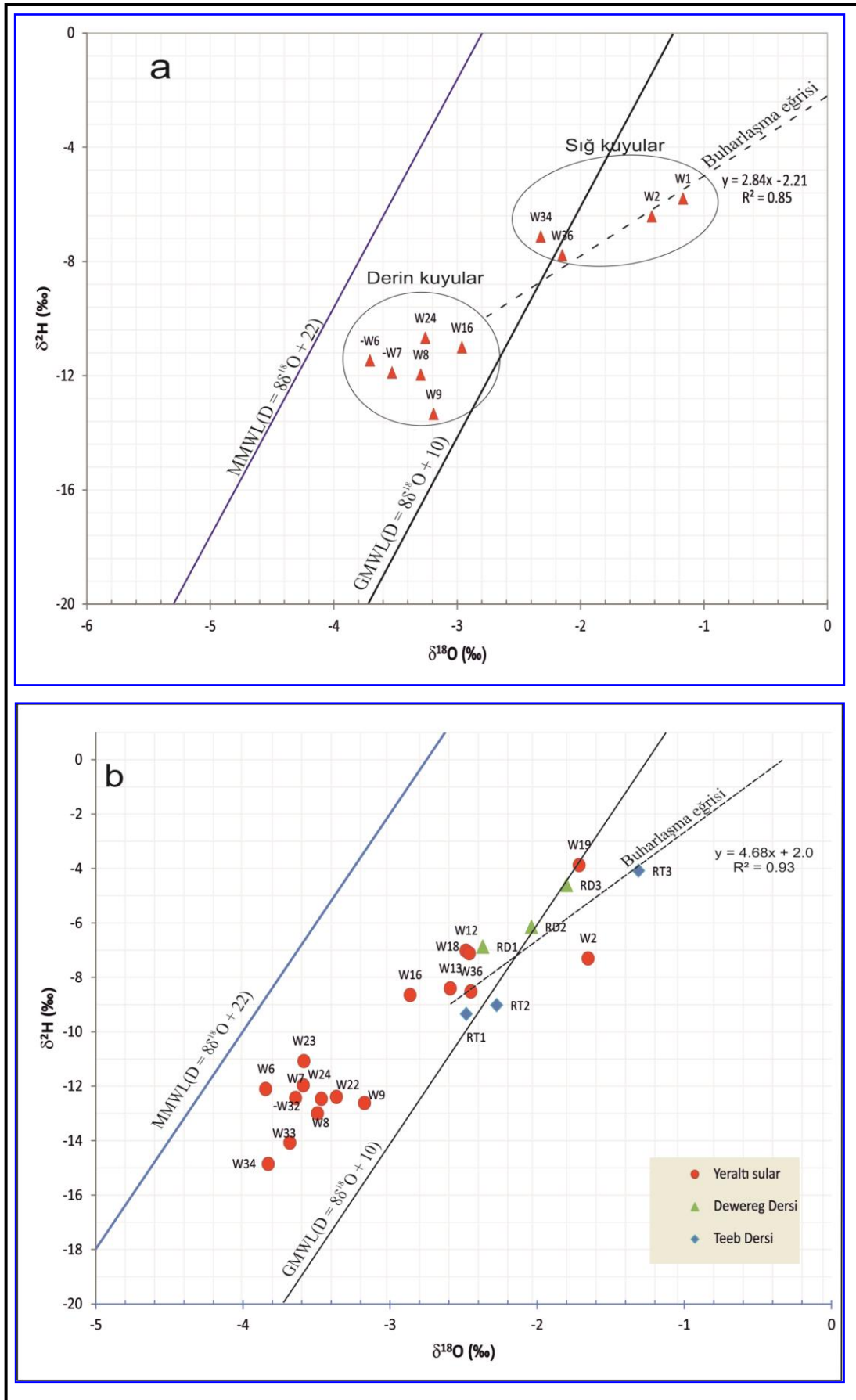
Şekil 4.59. Çalışma alanındaki suların \delta^{18}O - \delta D grafiği, a: Mayıs 2011, b: Aralık 2011
