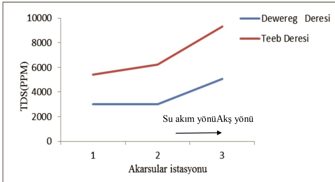
Şekil 4.19. İnceleme alanındaki akarsularda bulunan TDS değerlerinin istasyonlara göre değişimi; Teeb deresi ve Dewereg deresi
