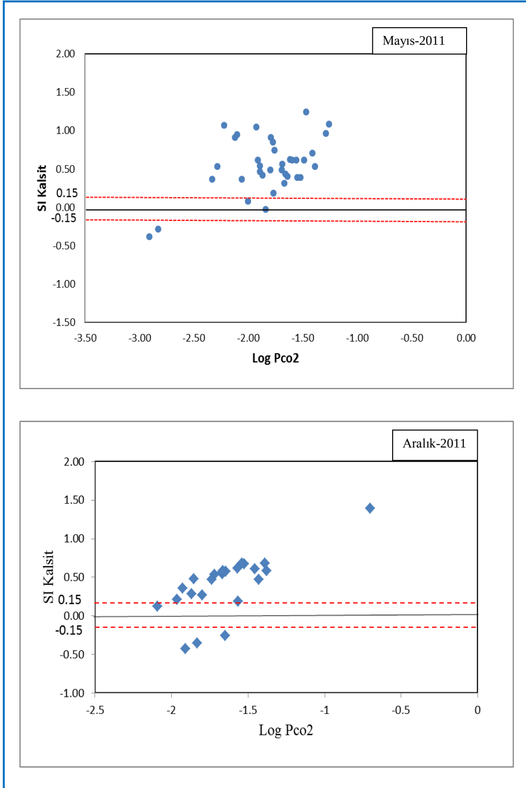
Şekil 4.38. Çalışma alanındaki yeraltı sularının LogPco 2 ve SI Kalsit ilişkisi ve doygunluk bölgeleri diyagramı
