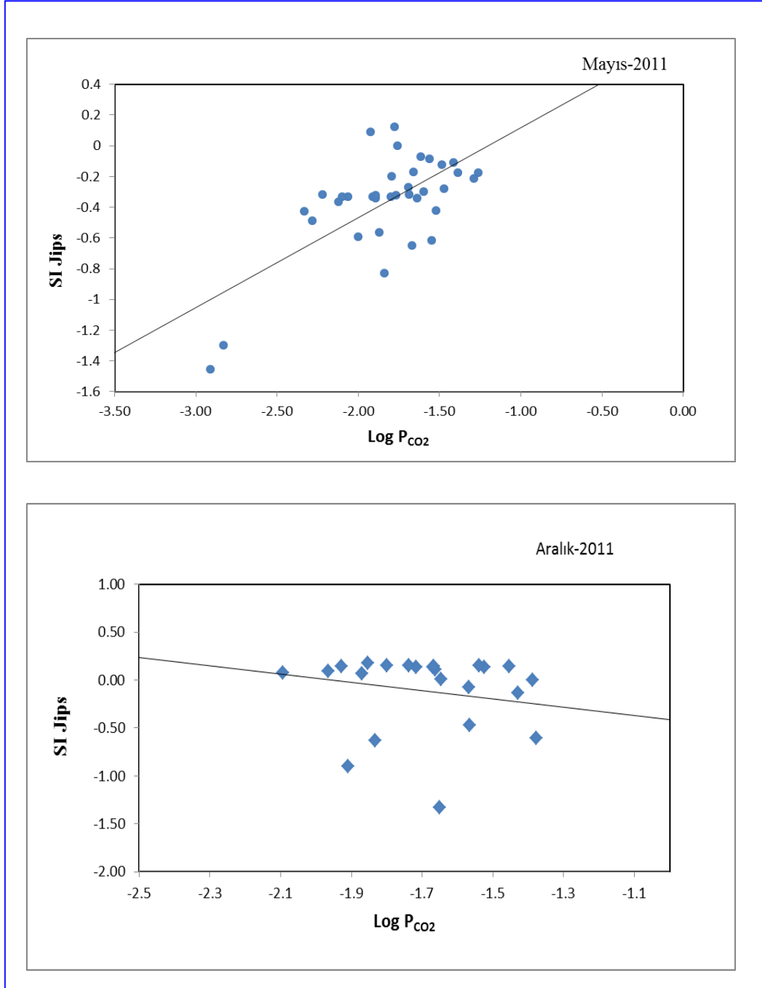
Şekil 4.51. Çalışma alanındaki yeraltı sularının \text{Log } P_{CO_2} - SI Jips ilişkisi diyagramı
