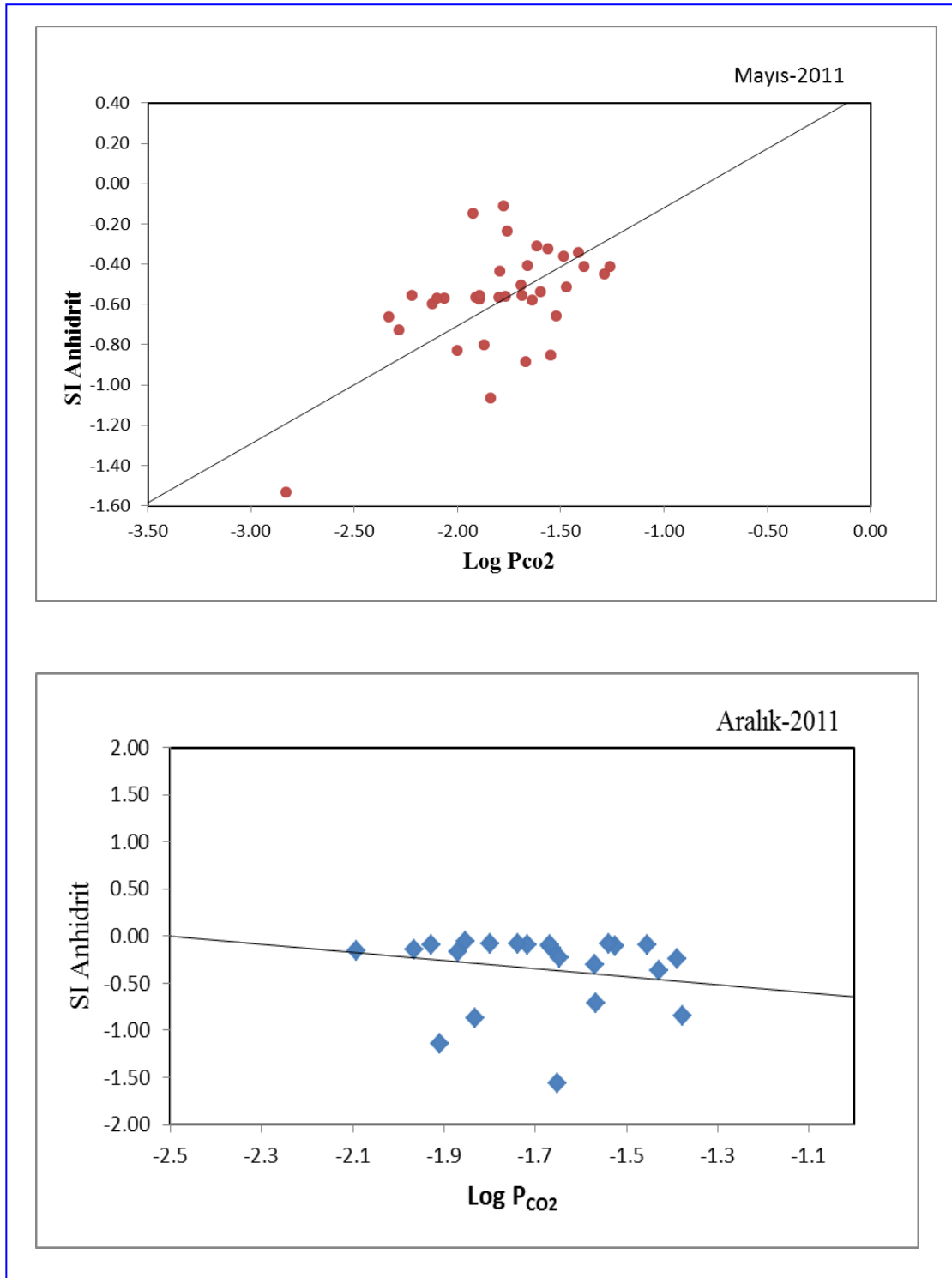
Şekil 4.52. Çalışma alanındaki yeraltı sularının \text{Log P}_{\text{CO}_2} -SI Anhidrit ilişkisi diyagramı
