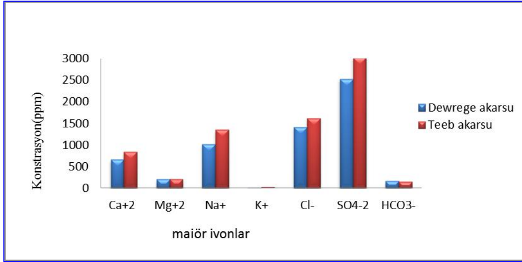
Şekil 4.20. Dewereg ve Teeb akarsularının önemli iyonlarının konsantrasyonu (mg/l).
