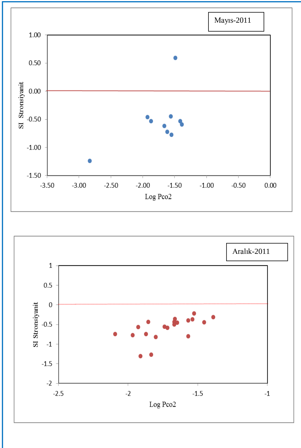
Şekil 4.41. Çalışma alanındaki yeraltı sularının LogPco 2 - SI Stronsiyanit ilişkisi doygunluk bölgeleri diyagramı
