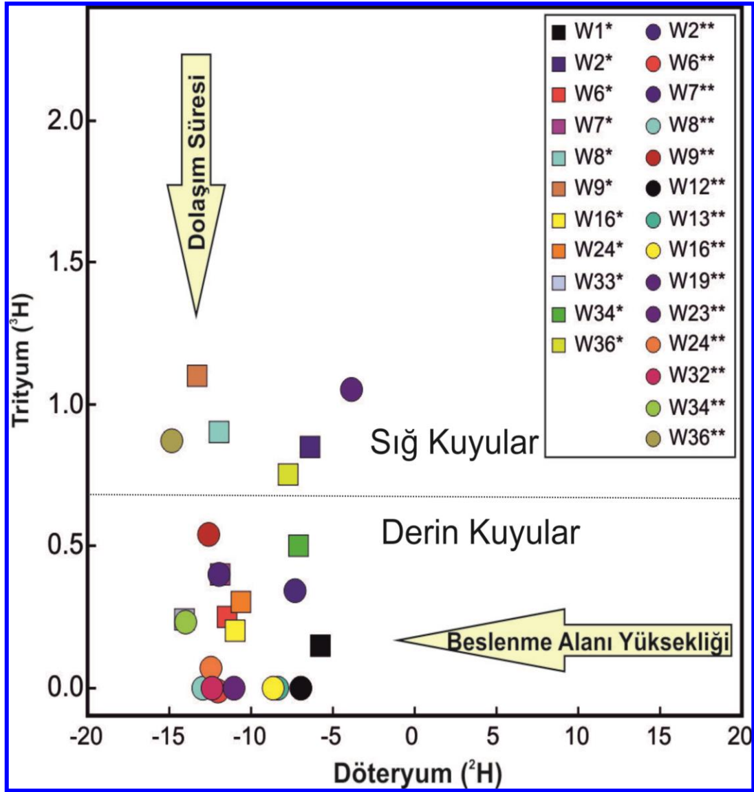
Şekil 4.62 Çalışma alanındaki yeraltı sularının \delta^3\text{H} – \delta\text{D} grafiği (*:Mayıs ve **:Aralık 2011)
