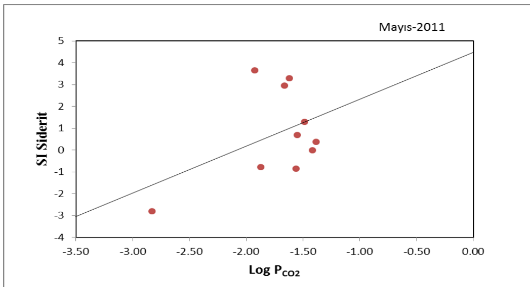
Şekil 4.50. Çalışma alanındaki yeraltı sularının \text{Log P}_{\text{CO}_2} -SI Siderit ilişkisi diyagramı
