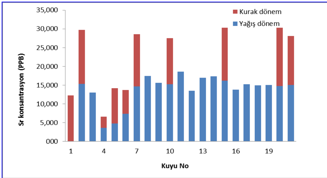
Şekil 4.32. Çalışma alanındaki yeraltı suların Sr konsantrasyonu
