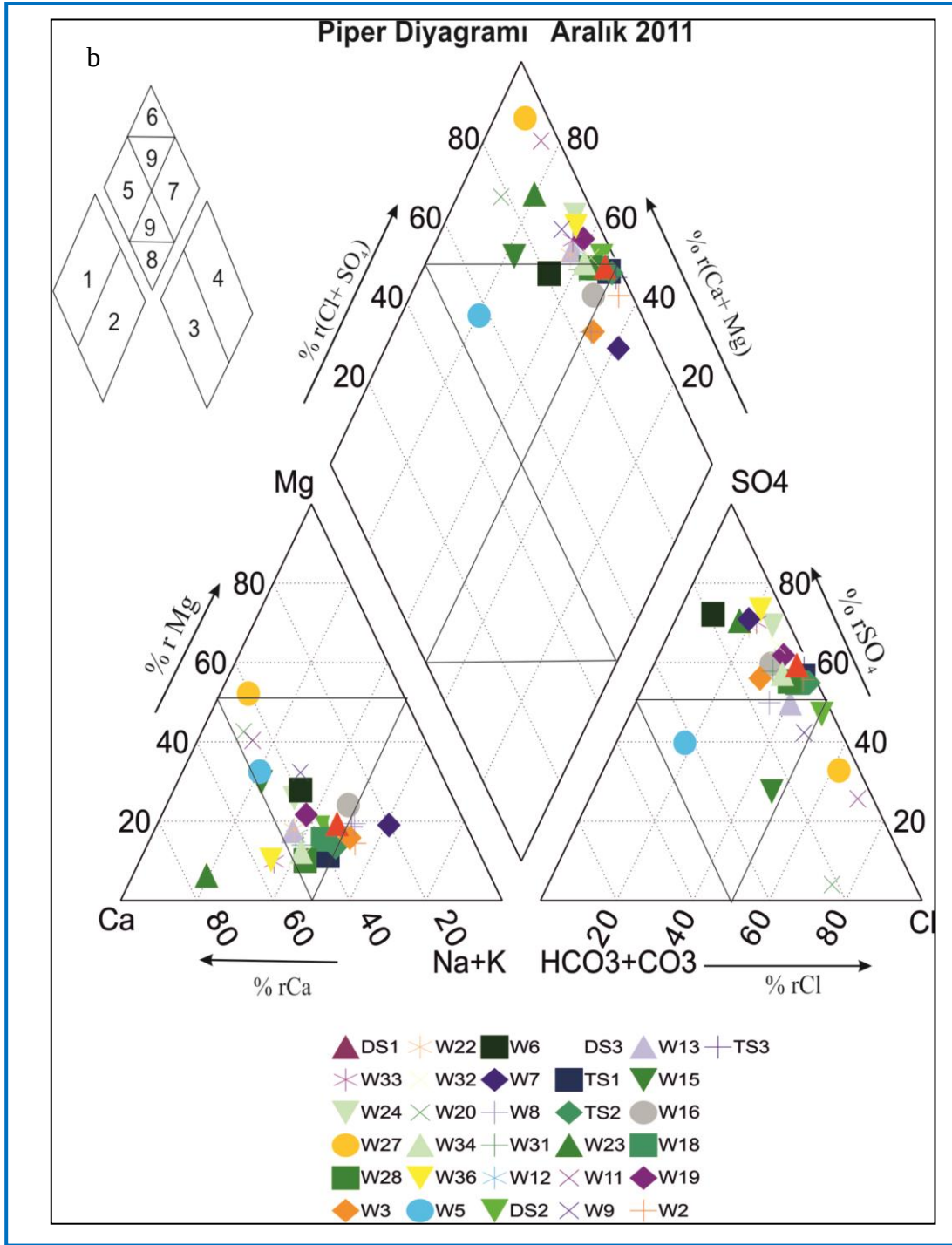
Şekil 4.35. Çalışma alanındaki su örneklerine ait Piper diyagramı, Aralık 2011
