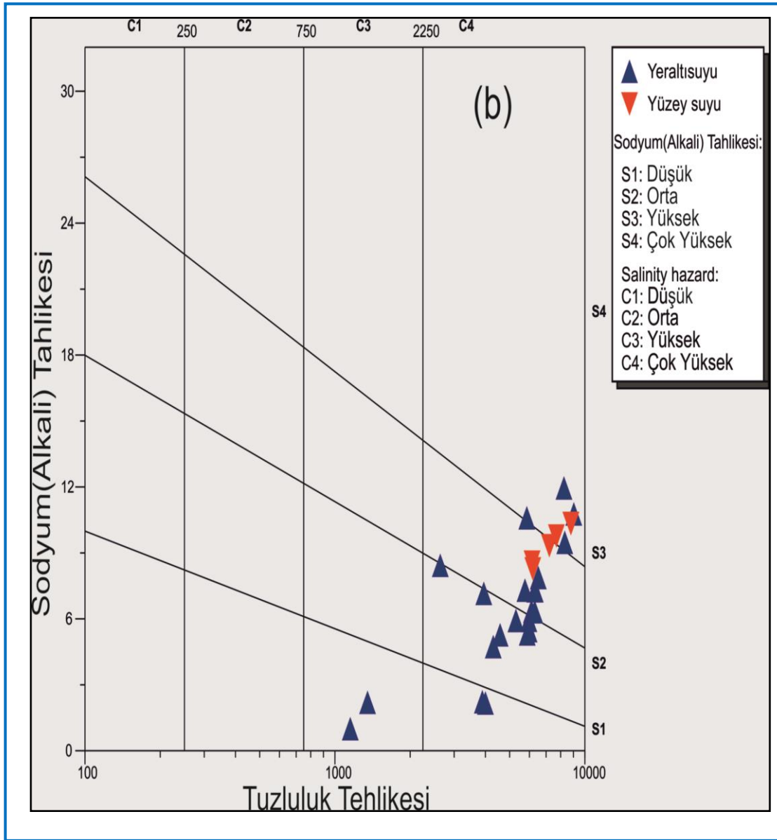
Şekil 4.36 b. Çalışma alanındaki su örneklerine ait Wilcox diyagramı b: Aralık 2011
