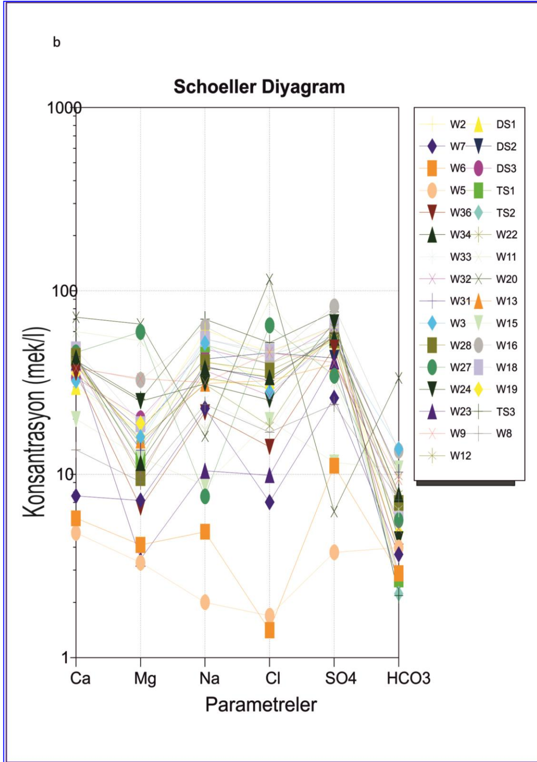
Şekil 4.33 b. Çalışma alanında yer alan yüzey ve yeraltı su örneklerinin Schoeller diyagramındaki konumları b: Yağışlı dönem (Aralık 2011)
