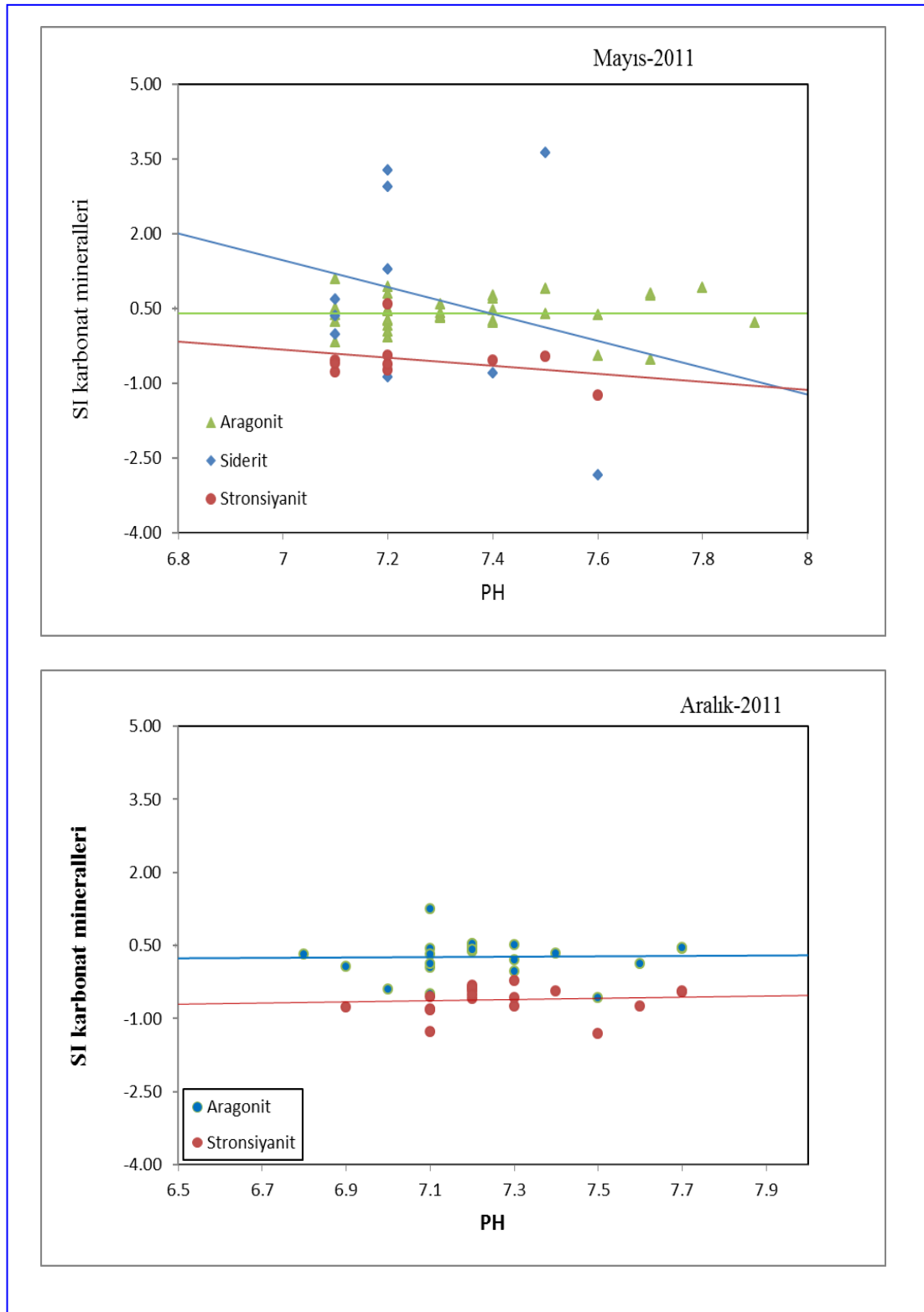
Şekil 4.56. Çalışma alanındaki yeraltı sularının pH – Karbonat mineral ilişkisi diyagramı
