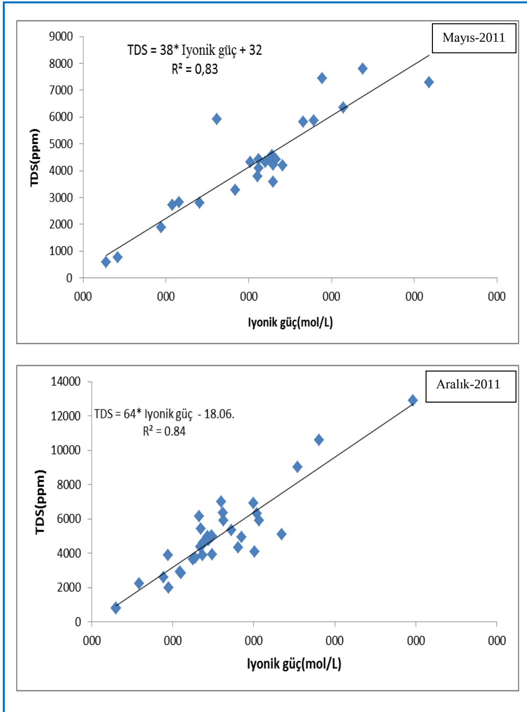
Şekil 4.37. TDS ve iyonik güç ilişkisi
