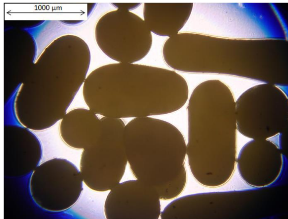
Şekil 3.15. Dibütil Maleat ile kaplanan küresel barutların görünümü
