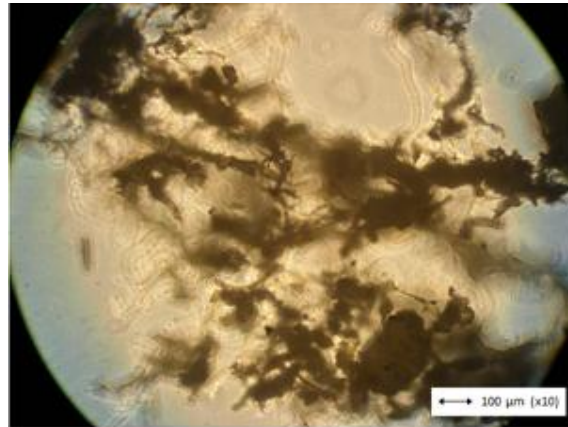
Şekil 3.5. Deney 3.sonucunda optik mikroskopta görüntülenenen nitroselüloz malzeme
