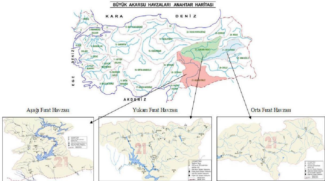
Şekil 4.1: Fırat havzası ve 3 alt havzanın konumu.
