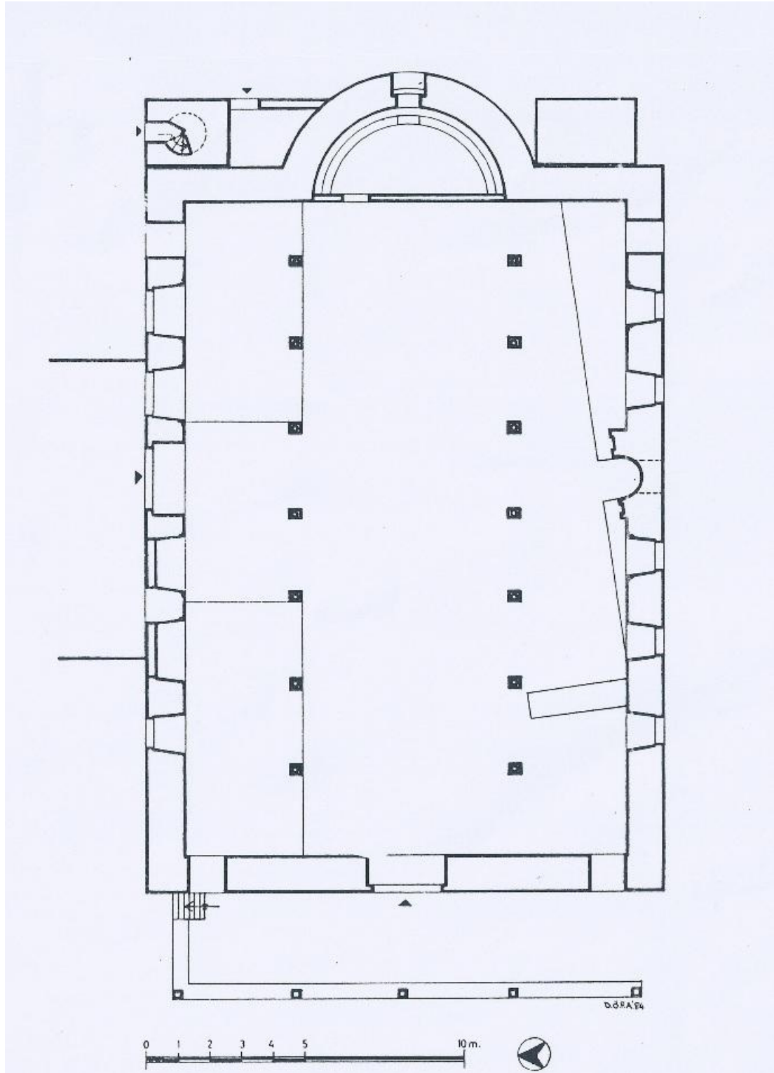
Çiz. 2: Koimesis Tes Theotokos Kilisesi (Bursa-Merkez-Demirtaş Köyü) Kilisesi Planı (DÖPA, 84).
