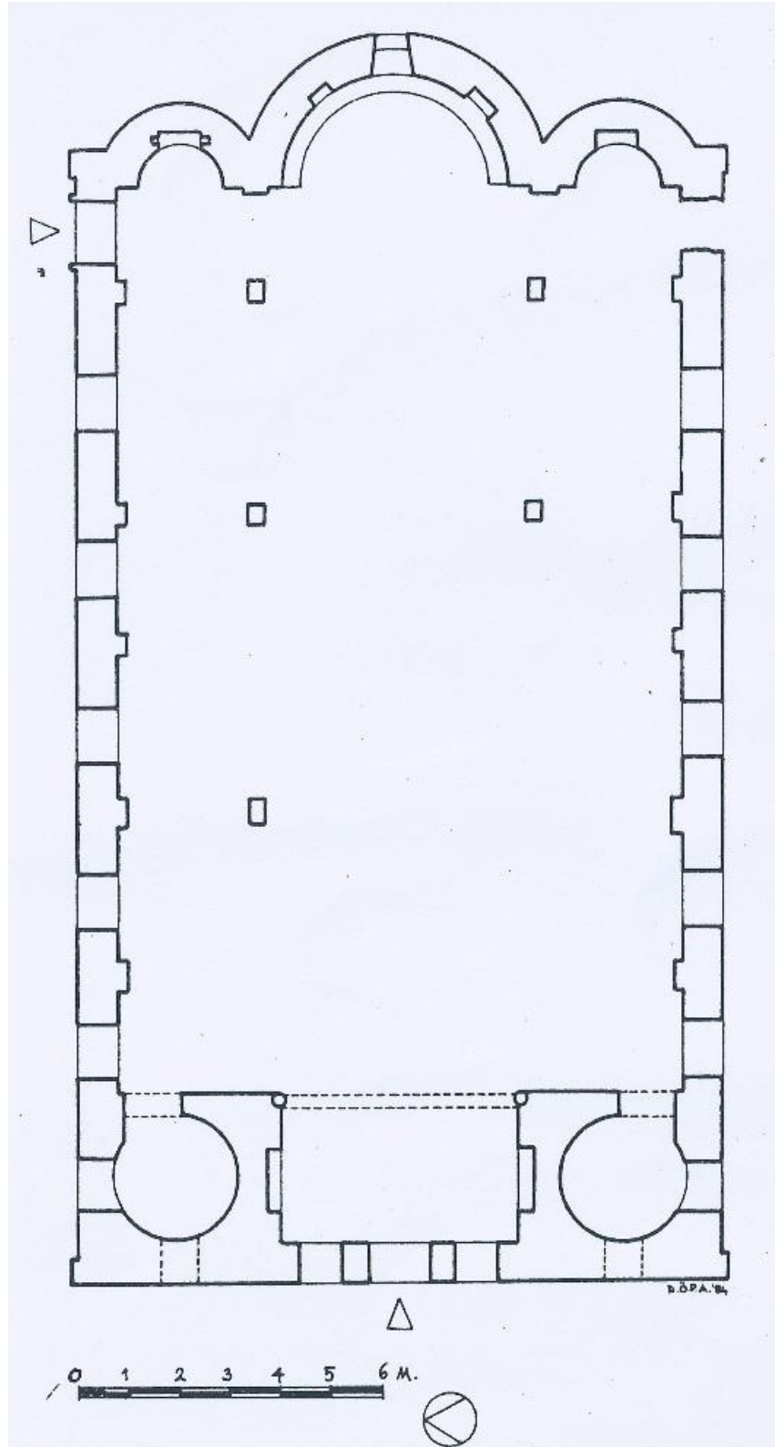
Çiz. 9: Hagios Georgios Kilisesi (Nilüfer-Gölyazı Köyü) Planı (DÖPA, 84).
