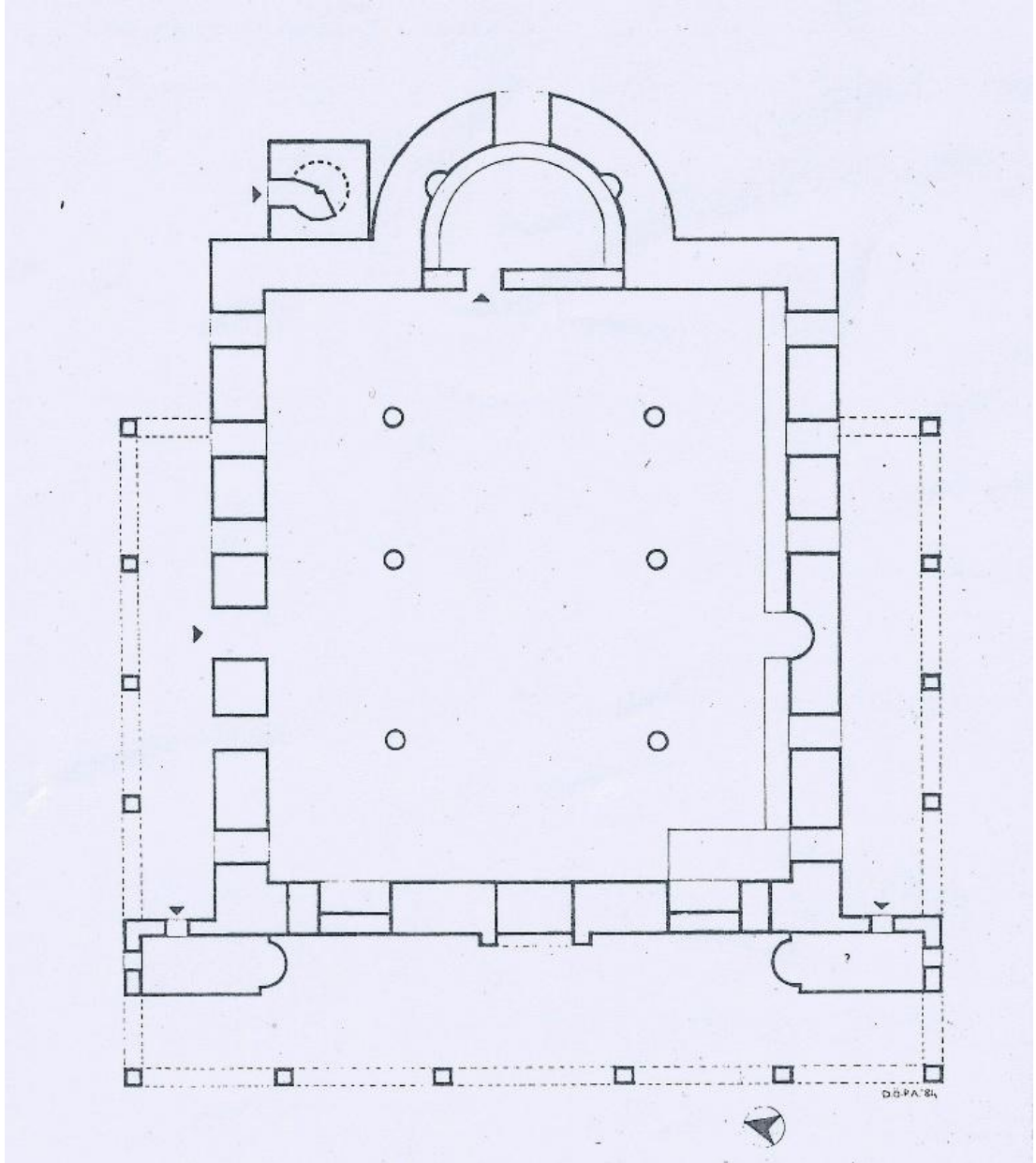
Çiz. 10: Agios Georgios Kilisesi (Nilüfer-Özlüce Köyü) Planı (DÖPA, 84).
