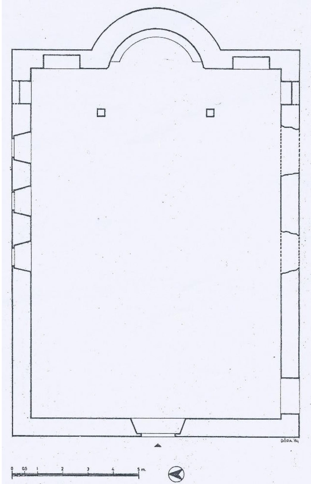
Çiz. 3: Hagios Georgios Kilisesi (Karacabey-Çamlıca Köyü) Planı (DÖPA, 84).
