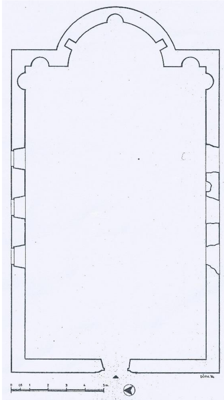
Çiz. 6: Zoodochos Pege Kilisesi (Karacabey-Karakoca Köyü) Planı (DÖPA, 84).
