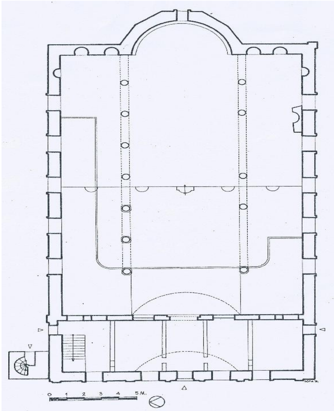
Çiz. 7: Agion Apostolon Kilisesi (Mudanya-Aydınpınar Köyü) Planı (DÖPA, 84).
