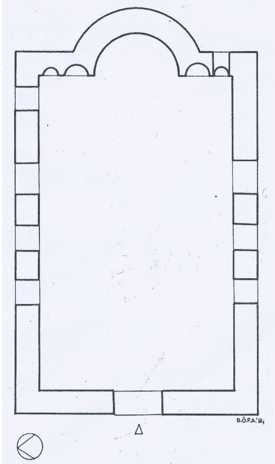
Çiz. 5: Mikhael Archangelos Kilisesi (Karacabey-Eskikaraağaç Köyü) (DÖPA, 84).
