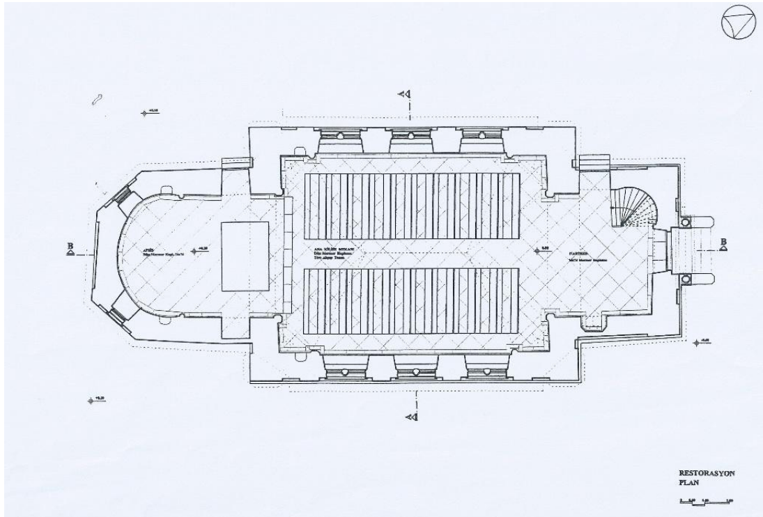
Çiz. 1: Fransız Katolik Kilisesi (Bursa-Merkez) Restorasyon Planı (Esin Şebin).
