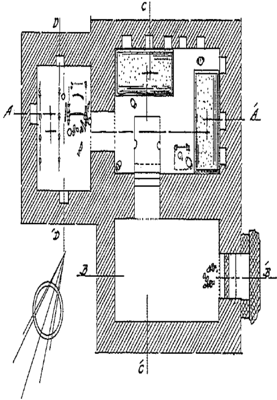
Çizim 5. Altıntepe Yer Altı Örne Mezarı-III
