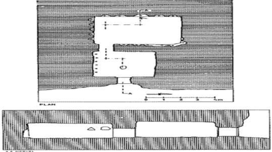
Çizim 1. Şirinlikale Kaya Mezarı-I Plan ve Kesiti
