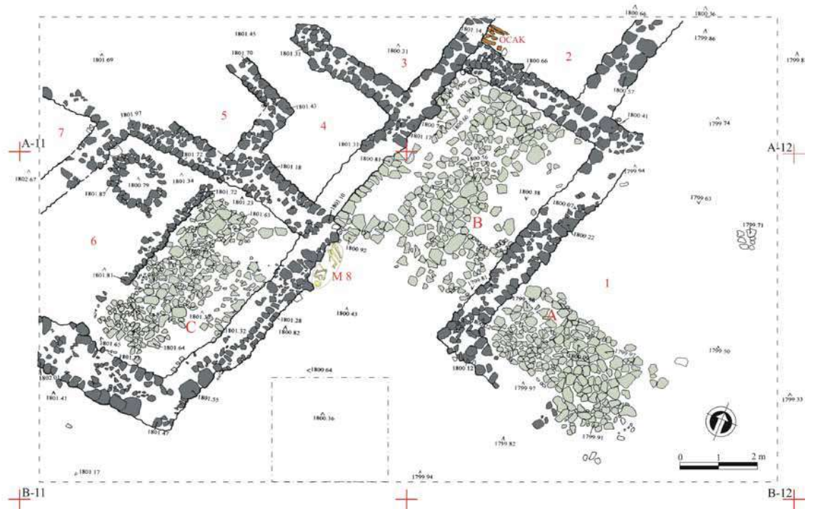
Çizim 9. Güllüdere Geç Demir Çağ Mimarisi
