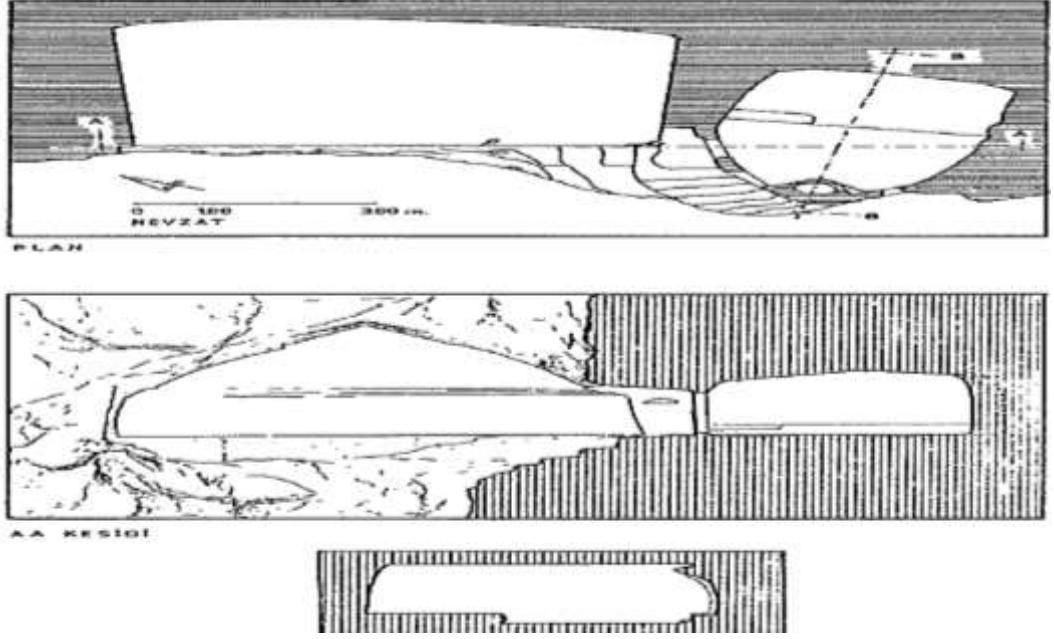
Çizim 6. Umudum Kaya Mezar Planı ve Kesiti
