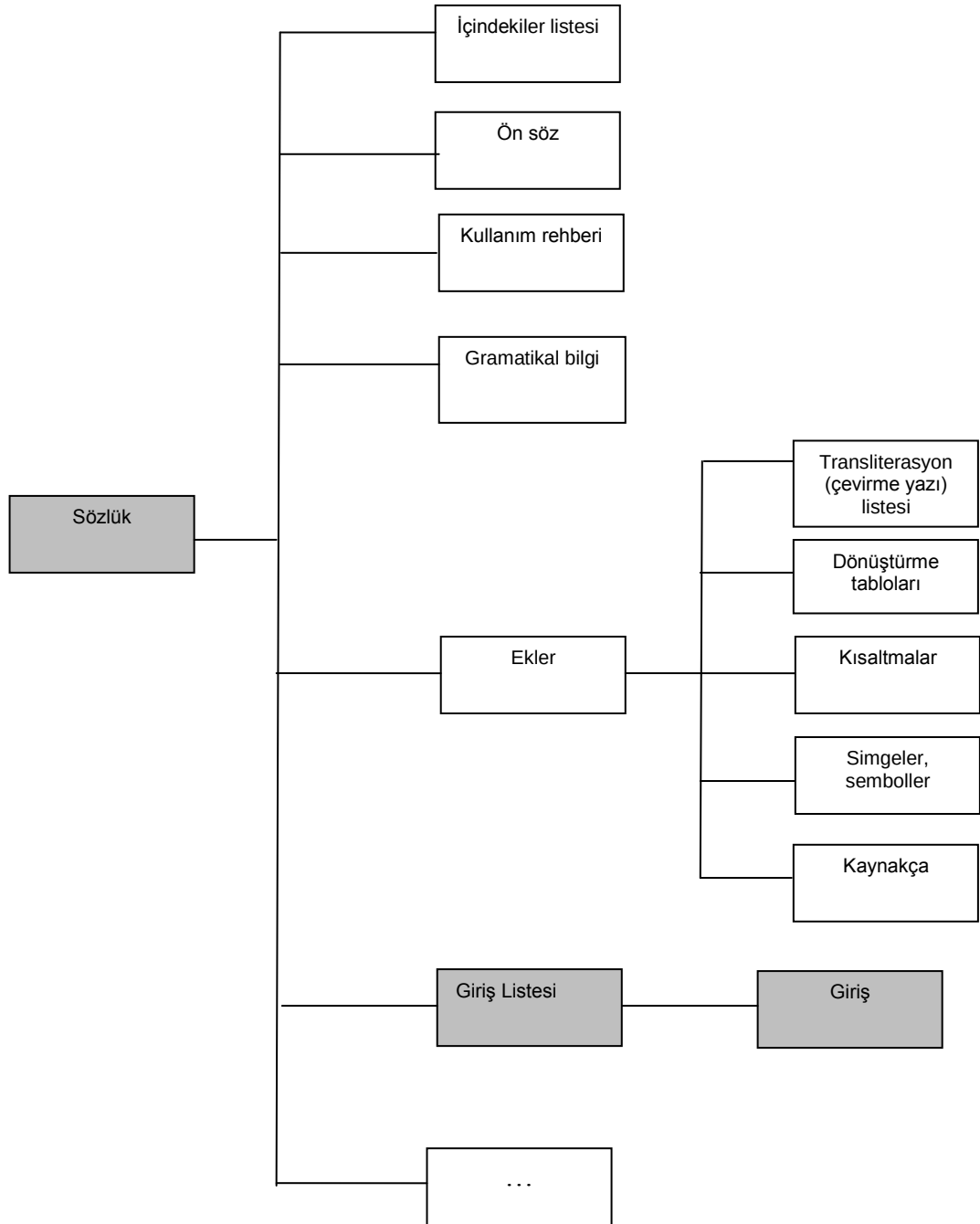
Şekil 2: Sözlüğün Yapısı
