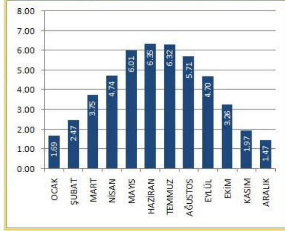
ANKARA Global Radyasyon Değerleri (KWh/m 2 -gün)
