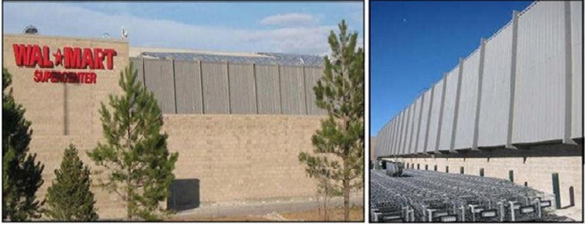
Şekil 4.2. Supercenter'in güney duvarındaki güneş duvarı [10]
