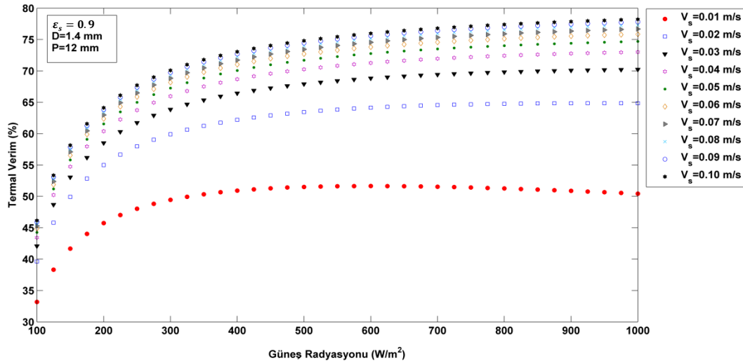
Şekil 3.6. Güneş duvarın üzerine düşen güneş radyasyonuna göre verimin değişimi
