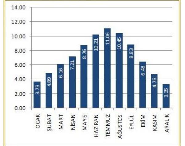
ANKARA Güneşlenme Süreleri (Saat)
