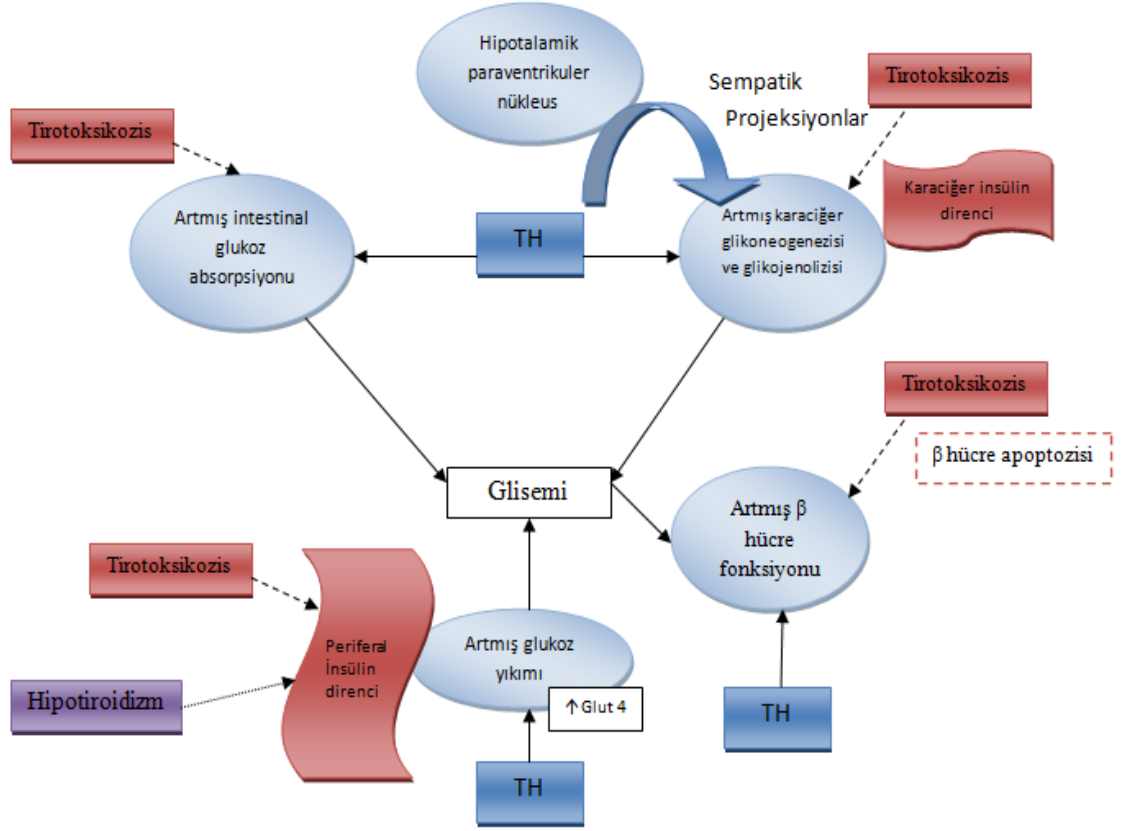
Şekil 6. Tiroid hormonlarının glukoz metabolizmasına etkileri; ötiroidide (kesintisiz çizgi), hipertroidide (kesikli çizgi), hipotroidide (ince kesikli çizgi), TH: tiroid hormonu[158]
