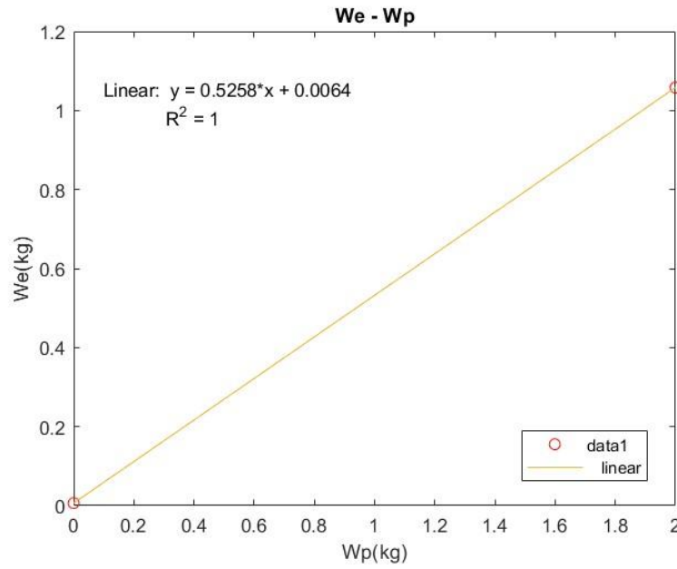
Şekil 3.22. W_e - W_p
