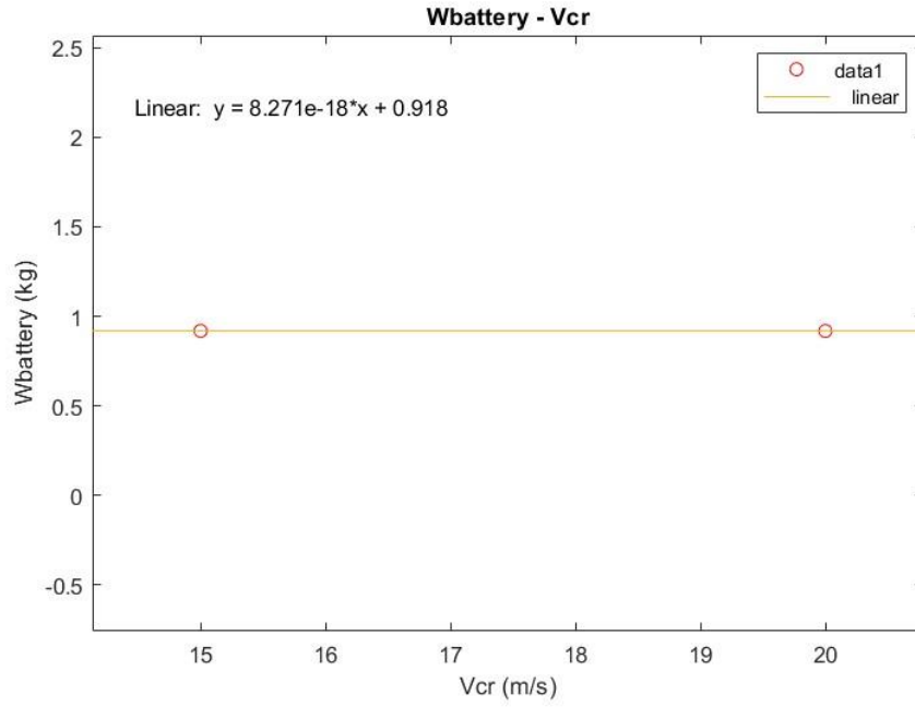
Şekil 3.33. W_f - V_{seyir}
