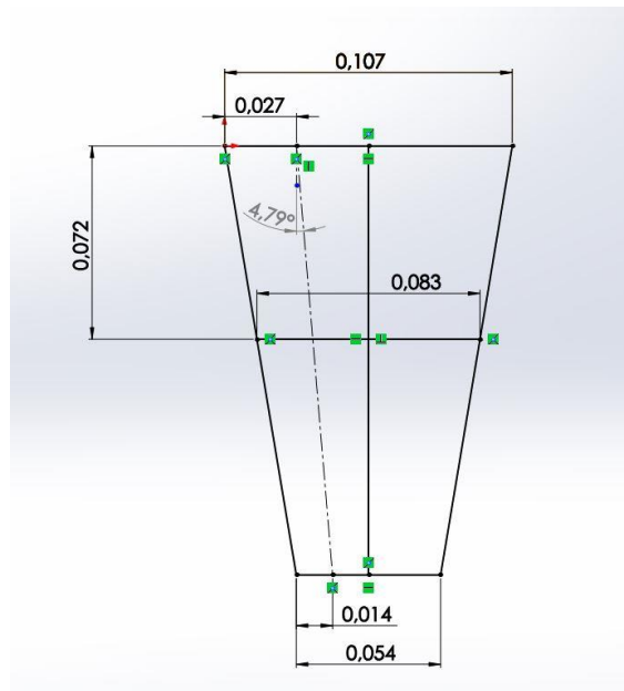
Şekil 3.58. Yatay kuyruğun üstten görünüşü (m)
