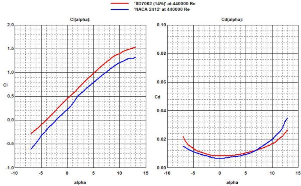
Şekil 3.38. C_l(\alpha) ve C_d(\alpha) – Alfa grafikleri (Airfoil Tools, 2024)
