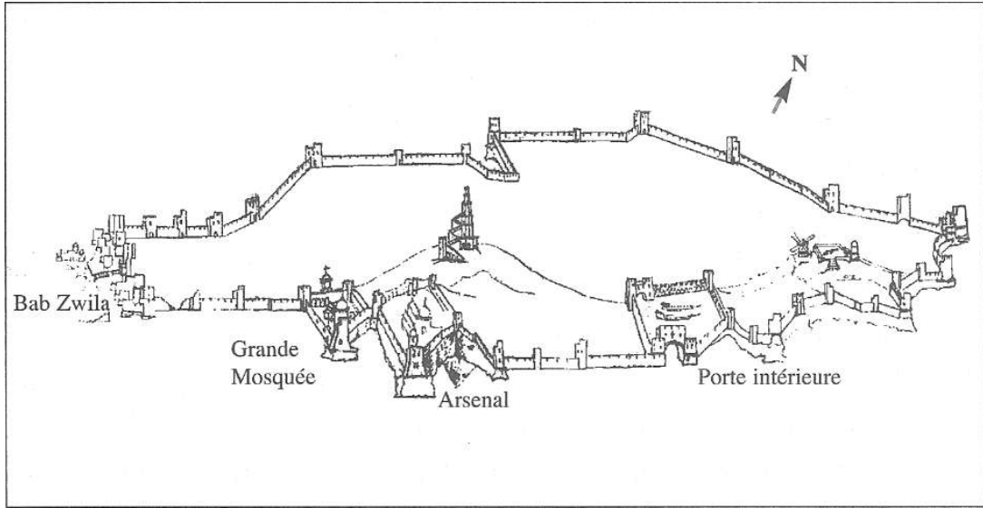
Harita 1.2: Mehdiye Şehir Planı. Farhat Dachroui, “L’Epoque Fatimide” Historie Generale de La Tunisie Le Moyen-Age (27-982/ 647-1574) , Nisan 2008, Tunus, s. 217.
