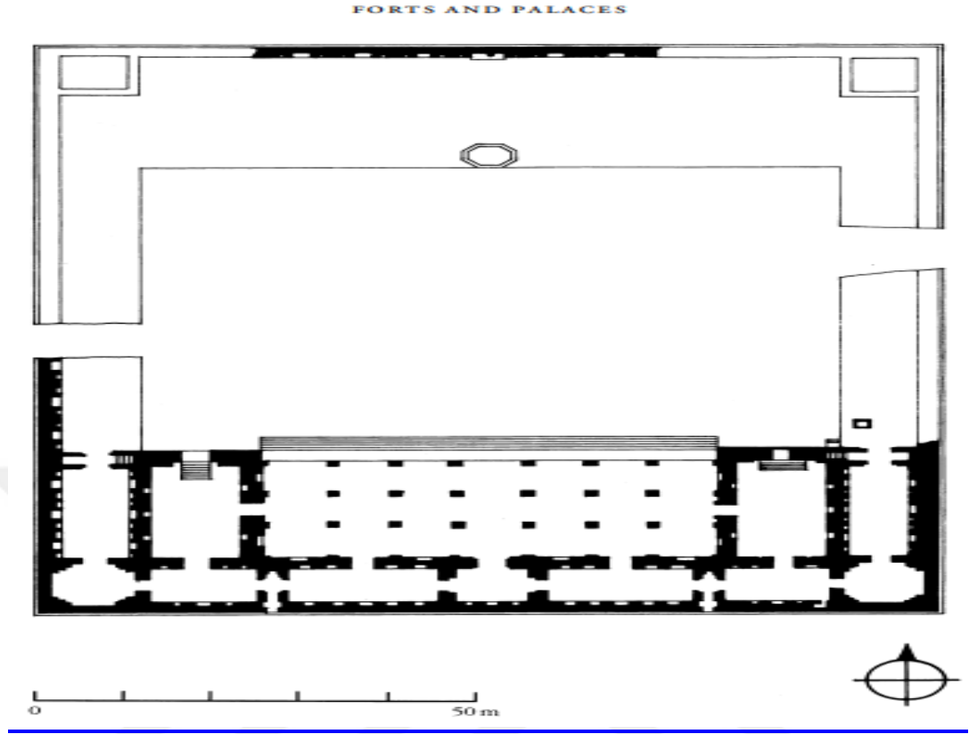
Plan 3. Durbar Planı (Michell-Zebrowski, 33.)
