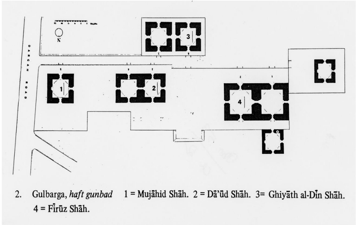
Plan 2. Gülberge'de Bulunan Haft Kumbet Planı ( https://www.archnet.org/sites/8475?media_content_id=90656 )
