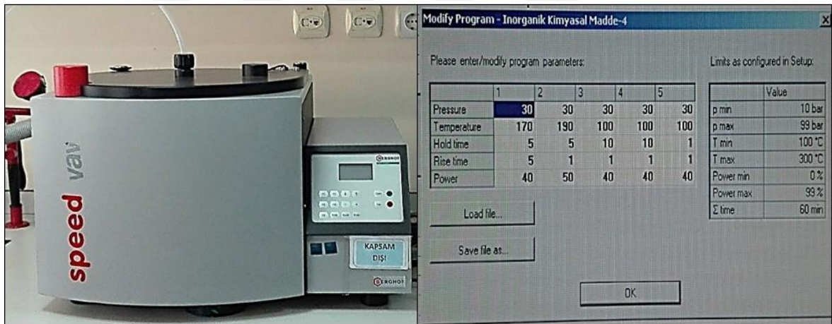
Şekil 2.10 Mikrodalga cihazı
