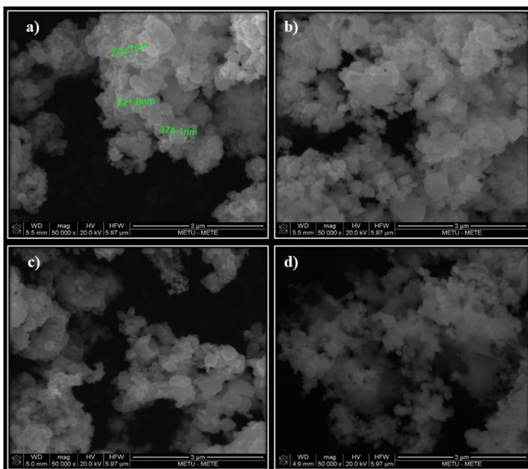
Figure 28. SEM micrographs of (a) Ni 2 P, (b) Ni 0.75 Co 0.25 P, (c) NiCoP, (d) Ni 0.25 Co 0.75 P.
