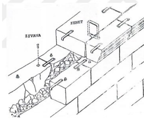
Şekil 3.29. Kesme taş ve keşet kullanılarak üretilen duvar detayı [99].
