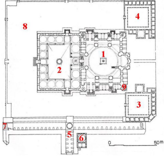
Şekil 2.21. Selimiye Camii ve Külliyesi vaziyet planı (1. Selimiye Camii, 2. Şadırvanlı avlu, 3. Selimiye Vakıf Müzesi, 4. Türk İslâm Eserleri Müzesi, 5. Kapalı çarşı, 6. Sıbyan mektebi, 7. Muvakkithane, 8. Cami dış avlu, 9. Kütüphane) [54].
