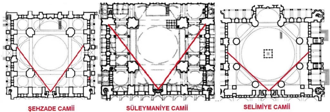
Şekil 3.6. Şehzade Camii, Süleymaniye Camii ve Selimiye Camilerinin girişlerinden yapı içlerine bakışta iç mekânın ne kadarına hâkim olduğunu anlatan karşılaştırmalı görsel [57].
