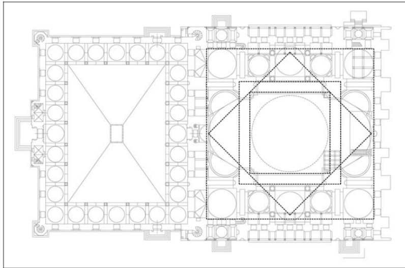
Şekil 2.17. Süleymaniye Camii planında oranlar [32].
