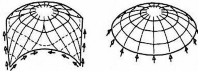
Şekil 3.24. Kubbe Tiplerinin Yük Aktarımı Grafiği [107].
