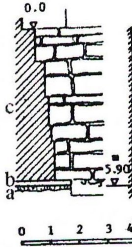
Şekil 3.9. Süleymaniye Camisi temel kesiti. Kible duvarlarının kuzey ucunda açılan sondaj çukurunda: a) Kum katmanı, b) Ahşap ızgara, c) Ampatmanlı temel [96].
