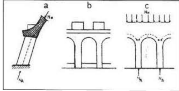
Şekil 3.27. Kubbe Mesnetleri- 2 [8].
