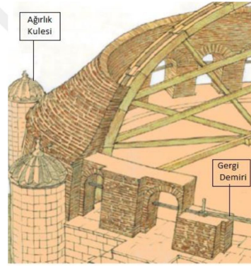
Şekil 3.23. Kubbe ve kasnak imalat şeması [100].
