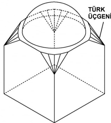
Şekil 3.17. Türk Üçgeni [57].
