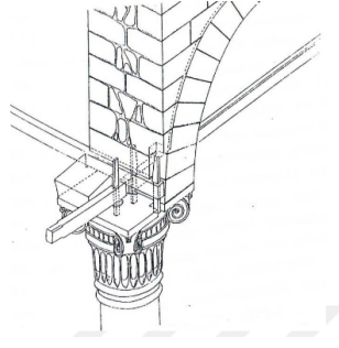
Şekil 3.21. Demir gergilerle ayakların birleşimi çizimi [99].
