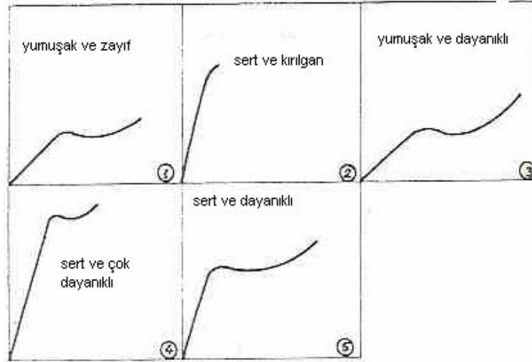
Şekil 4.2: Değişik mekanik özelliklerdeki plastik levhaların gerilme-uzama grafiği [1]
