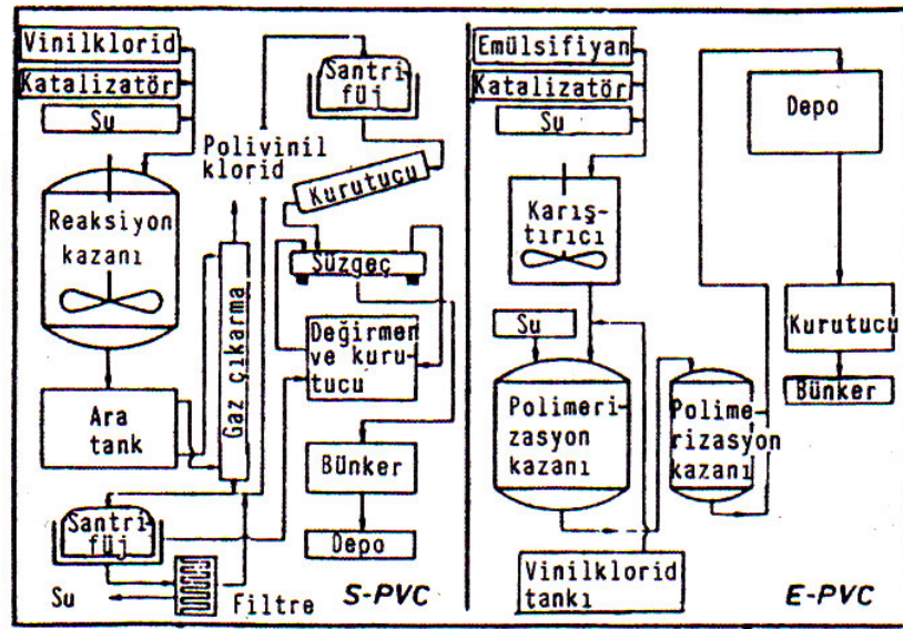
Şekil 3.52: Polivinilklorürün üretim şeması(S-PVC ve E-PVC) [3]
