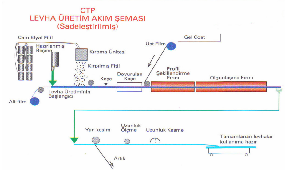
Şekil 3.24: CTP levha üretim akım şeması [30]
