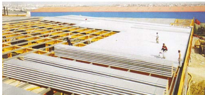
Şekil 3.45: Poliüretan dolgulu sandviç çatı paneli [42]
