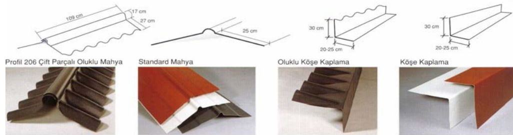
Şekil 3.26: Polyester levhadan üretilmiş mahya ve köşe kaplamaları [29]
