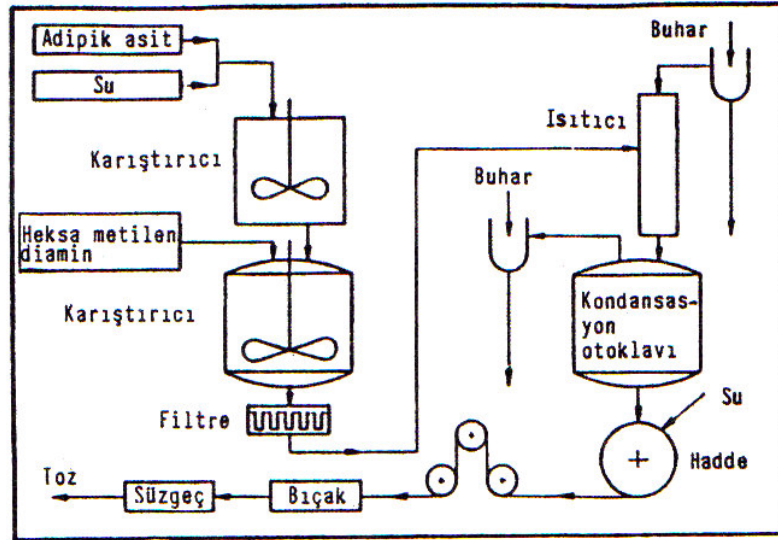
Şekil 3.19: Poliamidin(naylon) üretim şeması [1]
