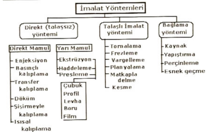
Şekil 2.2: Plastiklere uygulanan üretim yöntemleri [3]
