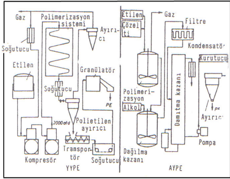
Şekil 3.32: AYPE ve YYPE' nin elde edilmesi
