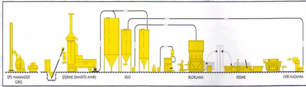
Şekil 3.43: EPS' nin üretim şekli [39]
