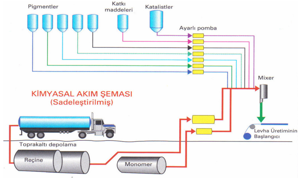
Şekil 3.23: Polyesterin kimyasal akım şeması [30]
