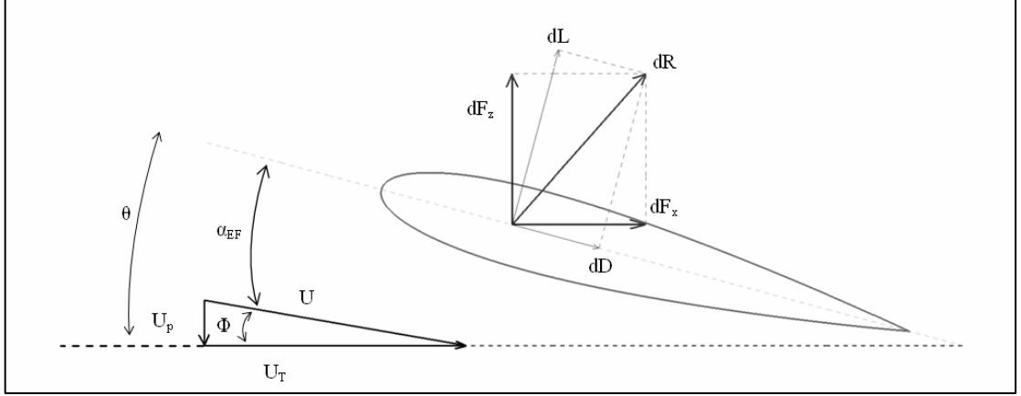
Şekil 7.2: Yerel hızlar ve yükler
