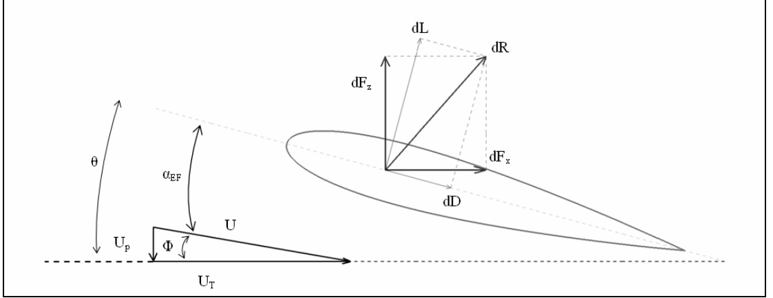
Şekil 7.8: Pala Elemanı üzerindeki hız ve yük bileşenleri
