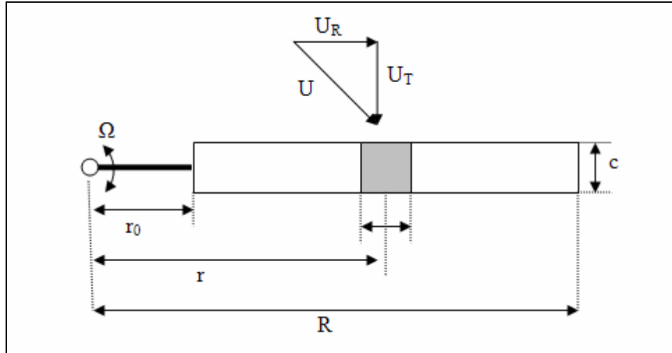
Şekil 7.1: Pala elemanı kuramı
