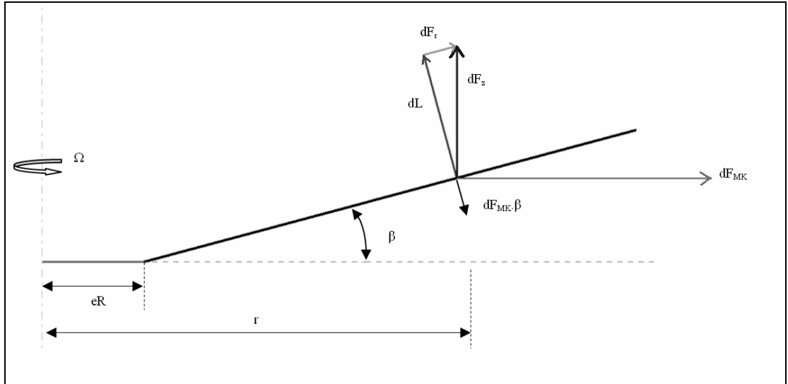
Şekil 7.6: Pala çırpınma açısı
