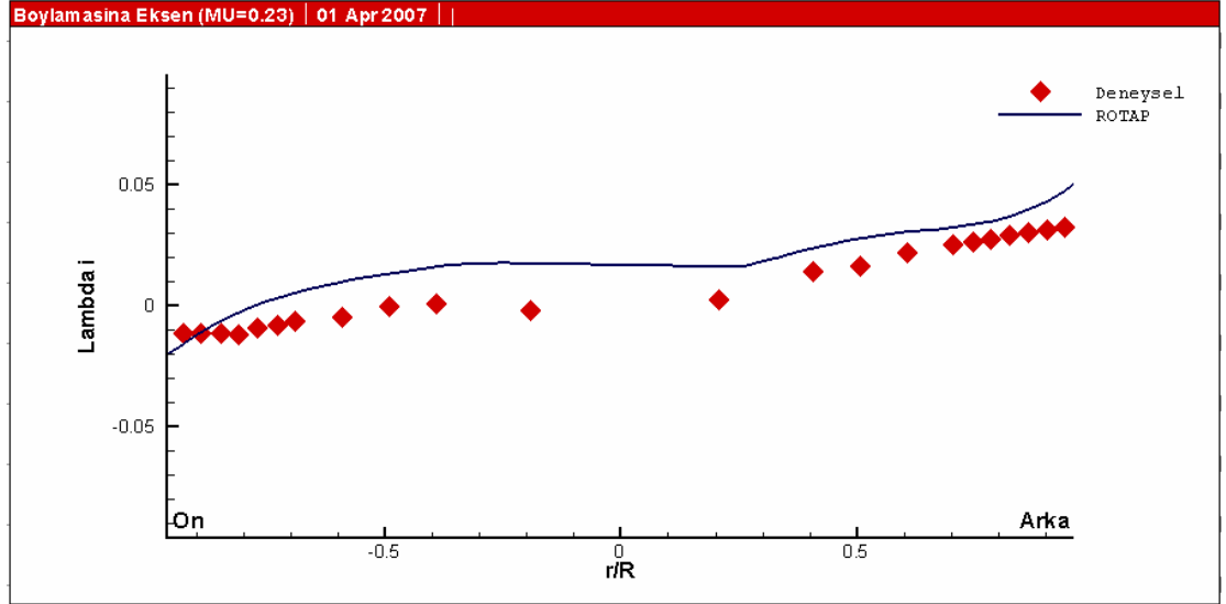
Şekil 7.14 b: \mu=0.23 için boylamasına eksen
