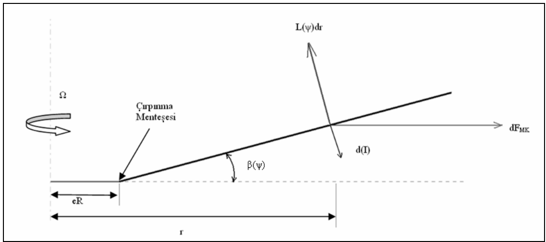
Şekil 7.11: Pala çırpınma hareketi
