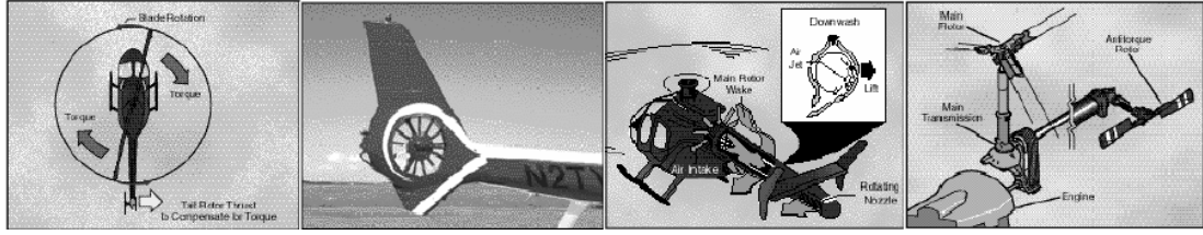
Şekil 2.2: TAR karşı tork Sistemleri [57]
