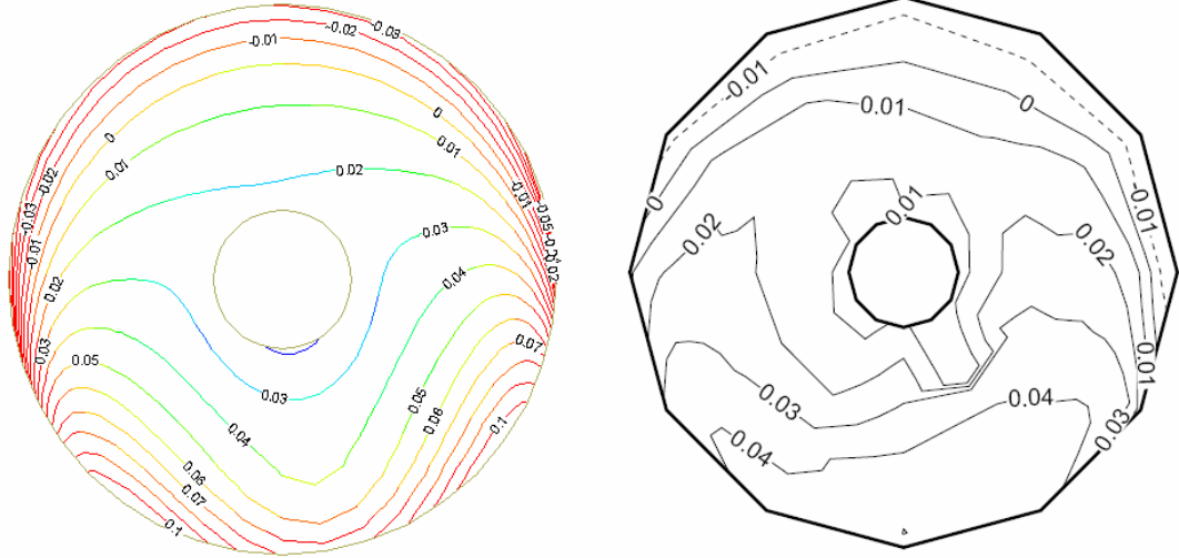
Şekil 7.15 a: \mu=0.15 İçe akış oranı disk dağılımı (ROTAP sol, deneysel sağ)
