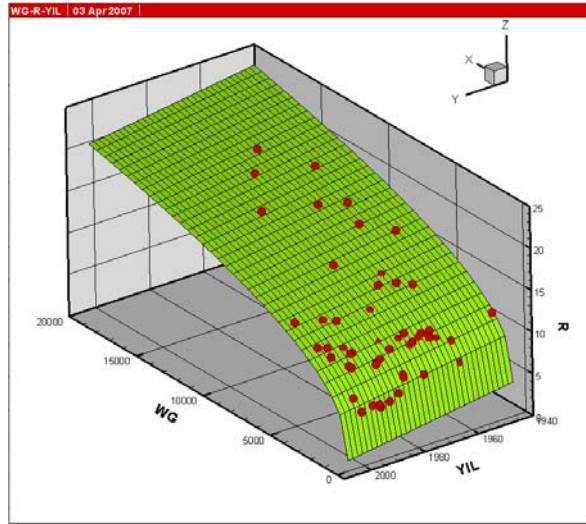
Şekil 5.5: Üstel fonksiyon kullanılarak elde edilen yüzey fonksiyonu
