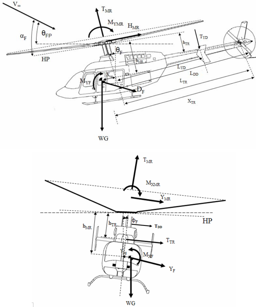
Şekil 7.16: Helikopter üzerindeki toplam yük ve momentler
