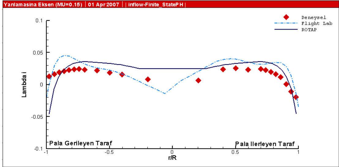
Şekil 7.13 a: \mu=0.15 için yanlamasına eksen
