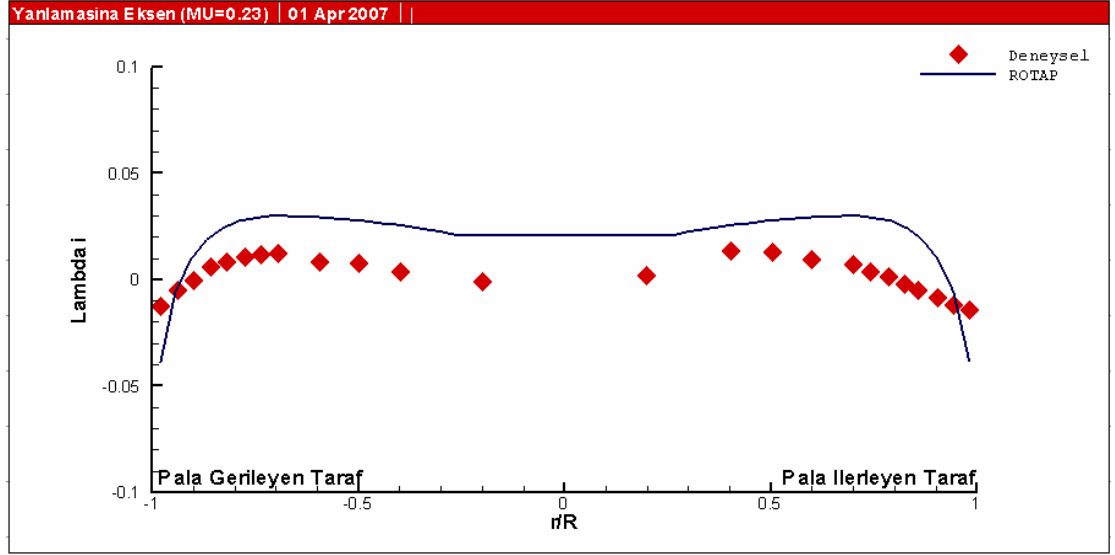
Şekil 7.14 a: \mu=0.23 için yanlamasına eksen
