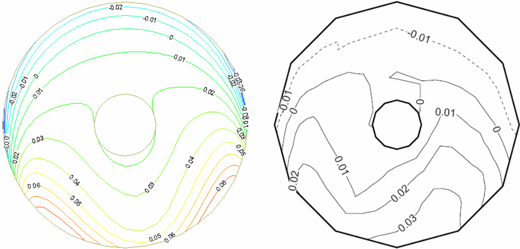
Şekil 7.15 b: \mu=0.23 İçe akış oranı disk dağılımı (ROTAP sol, deneysel sağ)
