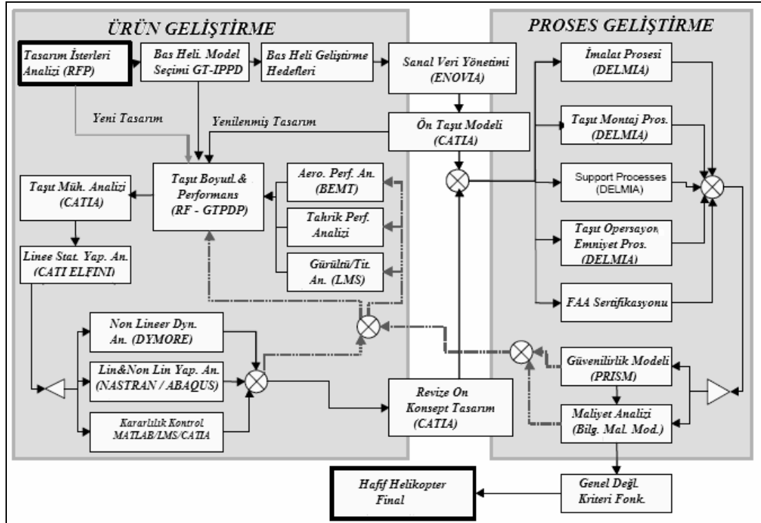
Şekil 1.1: Georgia Institute of Technology ürün ve süreç geliştirme yöntemi
