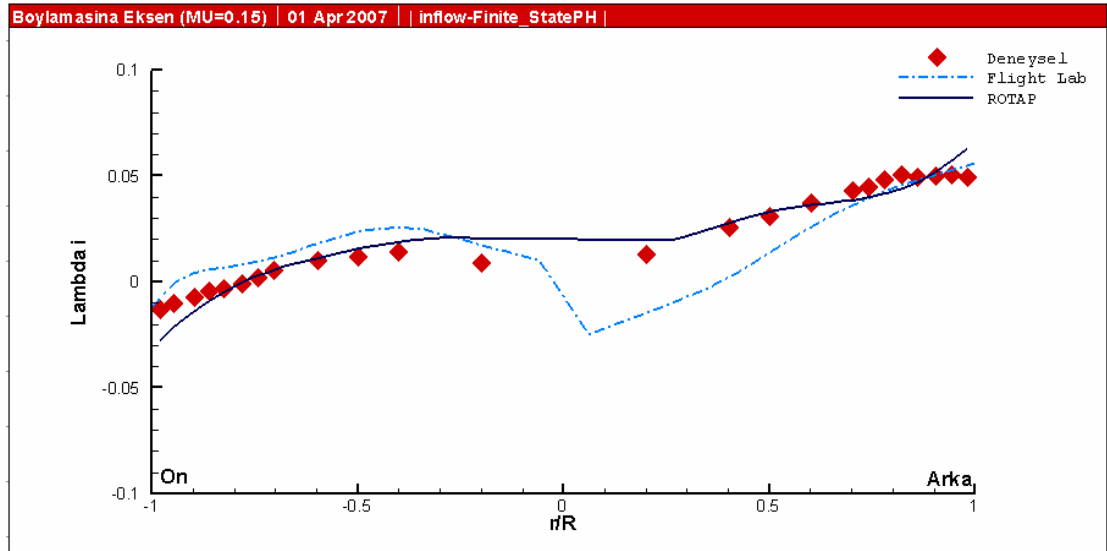
Şekil 7.13 b: \mu=0.15 için boylamasına eksen
