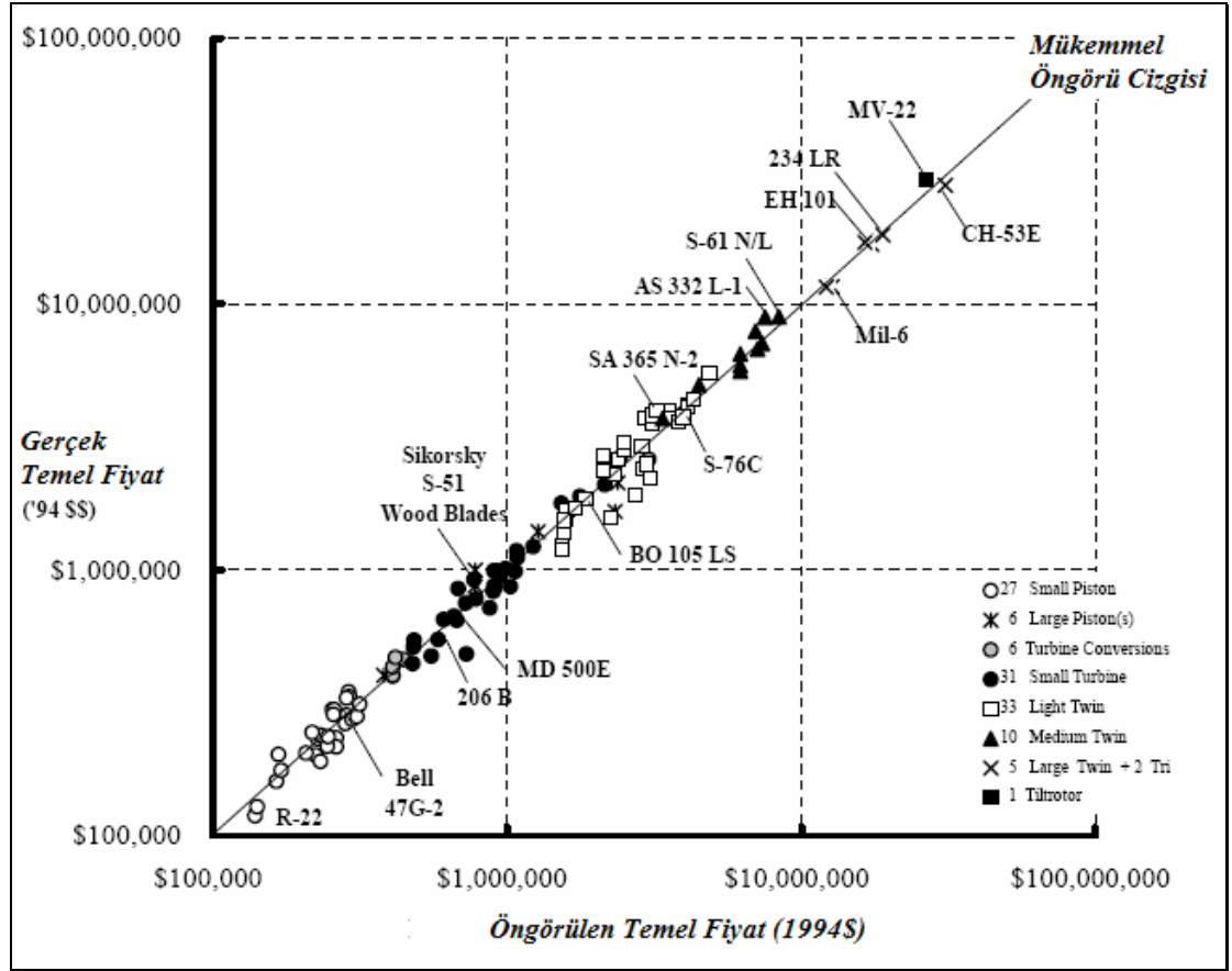
Şekil 9.3: Öngörülen ve gerçek helikopter temel fiyatları
