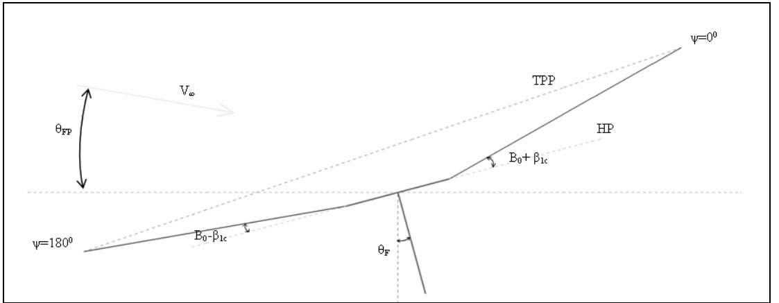
Şekil 7.9: Boylamasına doğrultuda rotor ileri uçuşu
