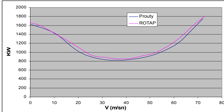
Şekil 11.1: Prouty örnek helikopter başarımları karşılaştırması
