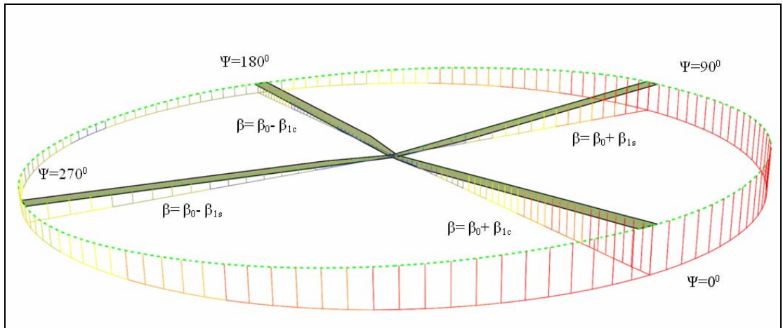
Şekil 7.7: Azimut boyunca çırpınma açısı değişimi
