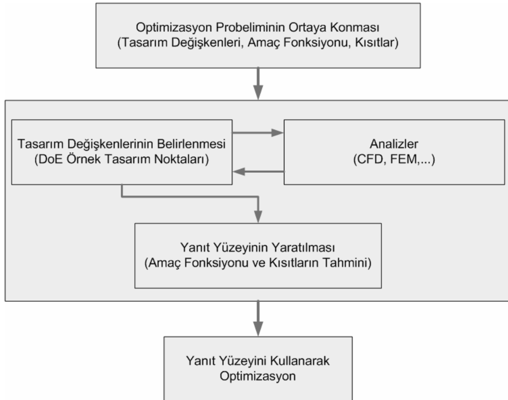
Şekil 6.1: RSM genel akış şeması
