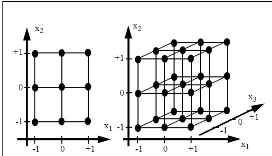
Şekil 6.4: Tam çarpanlı üçüncü seviye örnek tasarım noktaları
