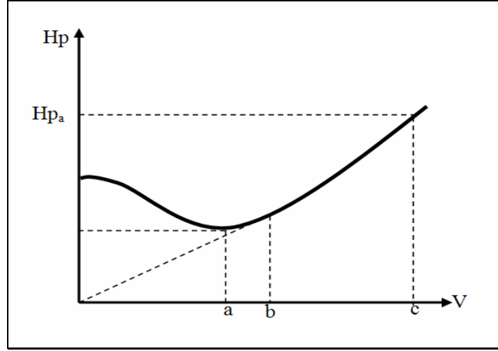
Şekil 7.19: Güç gereksinimi – Hız grafiği
