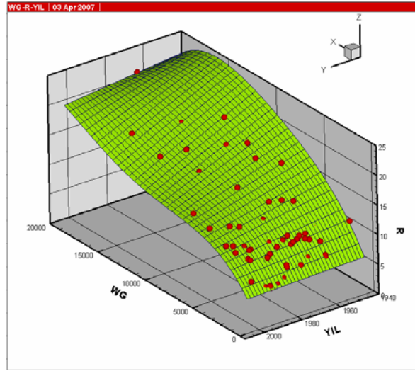
Şekil 5.6: Polinom fonksiyonu kullanılarak elde edilmiş yüzey fonksiyonu
