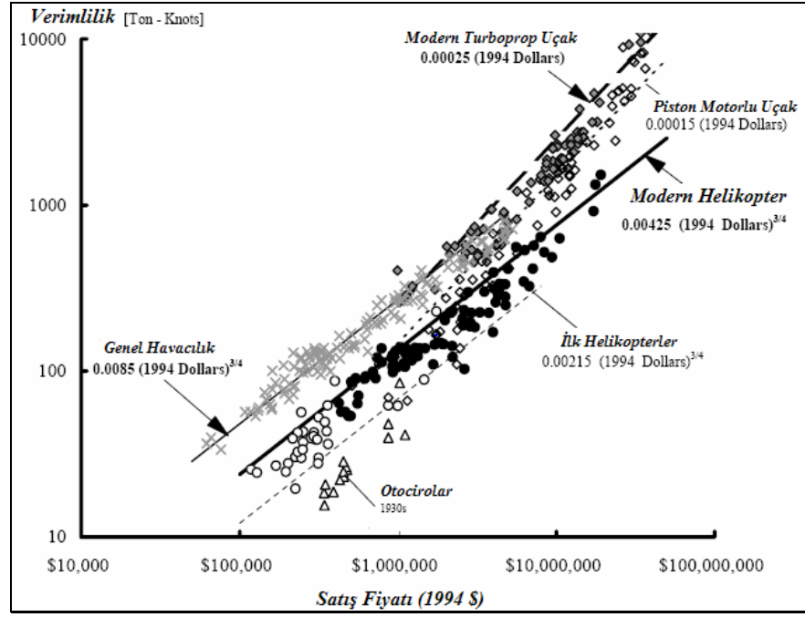
Şekil 9.1: Havacılık ürünleri verimlilik - satış fiyatı değişimleri
