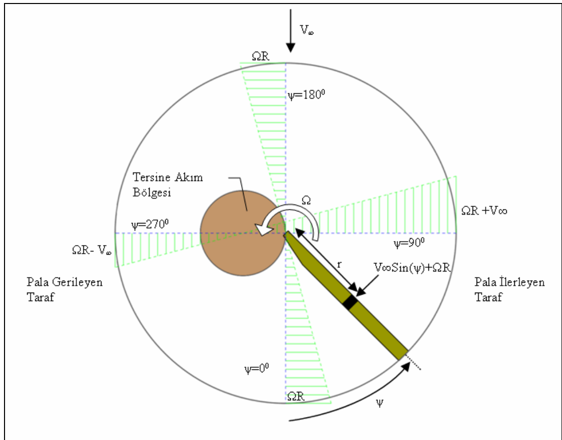
Şekil 7.5: İleri uçuşta disk boyunca hız değişimleri
