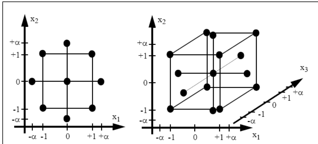
Şekil 6.5: CCD üçüncü seviye örnek tasarım noktaları
