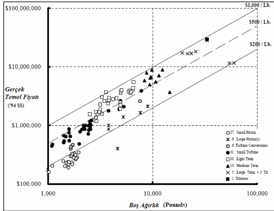
Şekil 9.2: Temel fiyat boş ağırlık değişimi
