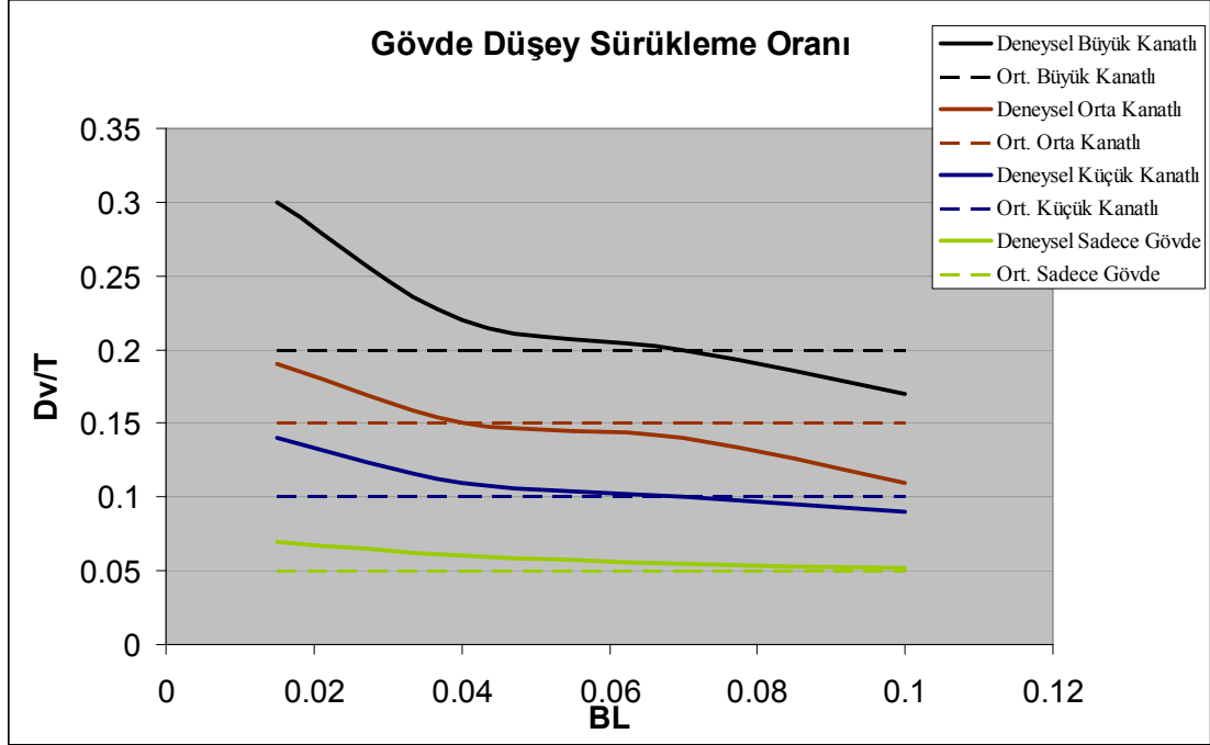
Şekil 7.4: Gövde düşey sürüklenme oranı
