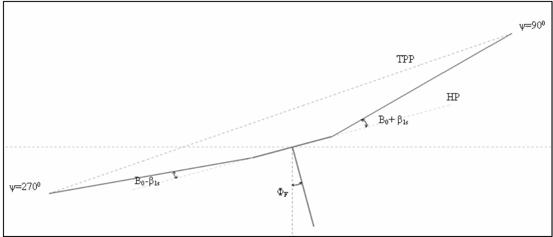
Şekil 7.10: Yanlamasına doğrultuda rotor ileri uçuşu
