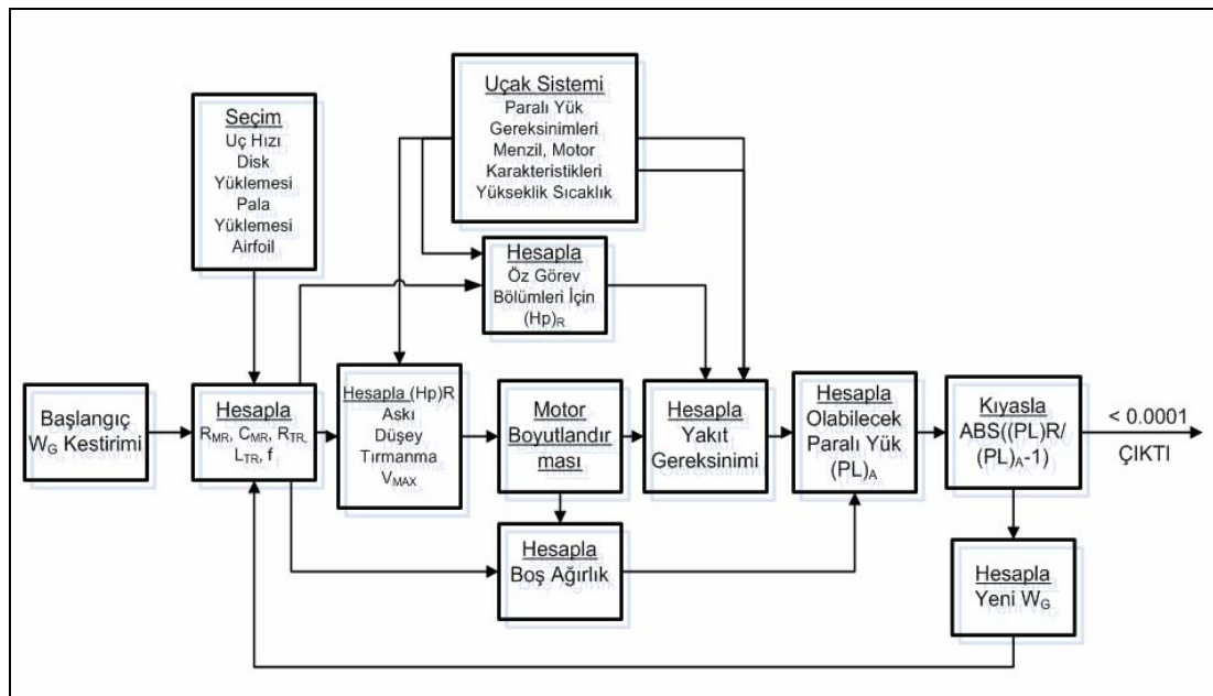
Şekil 3.3: GTPDP genel akış şeması
