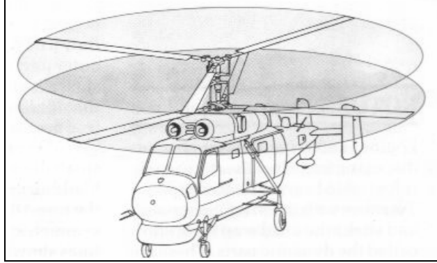
Şekil 2.4: Eş eksenli rotorlu helikopterler [56]
