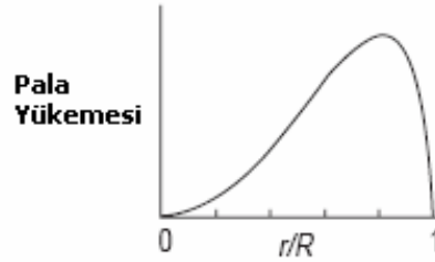
Şekil 6.12: Mangler Tarafından Kabul Edilen TİP3 Rotor Yükleme
