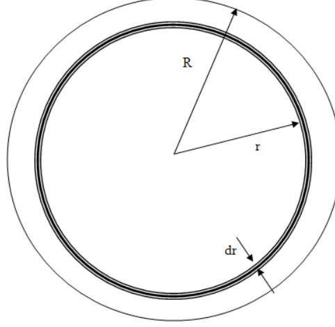
Şekil 7.3: Pala elemanı momentum kuramı içe akış modeli
