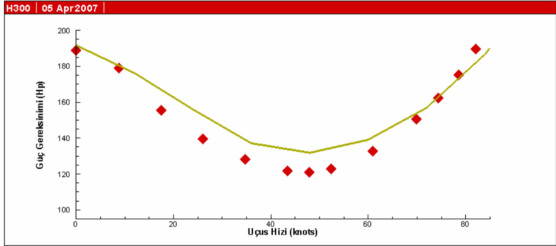
Şekil 7.18: H300 İleri Uçuş deneysel ve ROTAP analiz sonuçları
