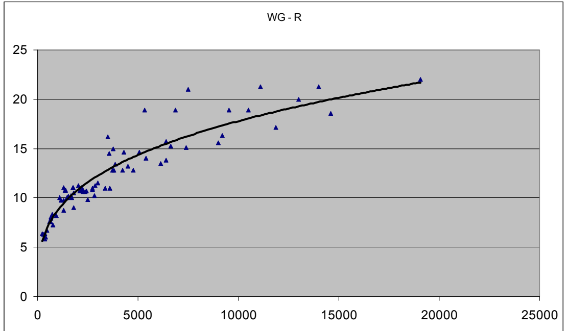
Şekil 5.1: İstatiksel rotor yarıçapı toplam kalkış ağırlığı değişimi
