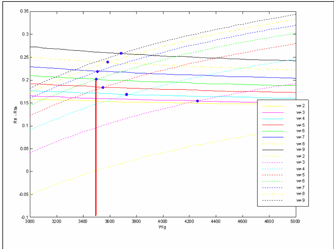
Şekil 3.2: Örnek R_F Metot yakıt ağırlık oranları ve kesişimleri
