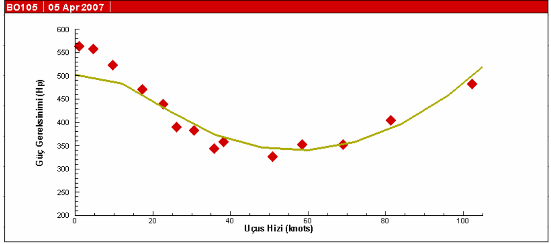
Şekil 7.17: BO105 İleri uçuş deneysel ve ROTAP analiz sonuçları
