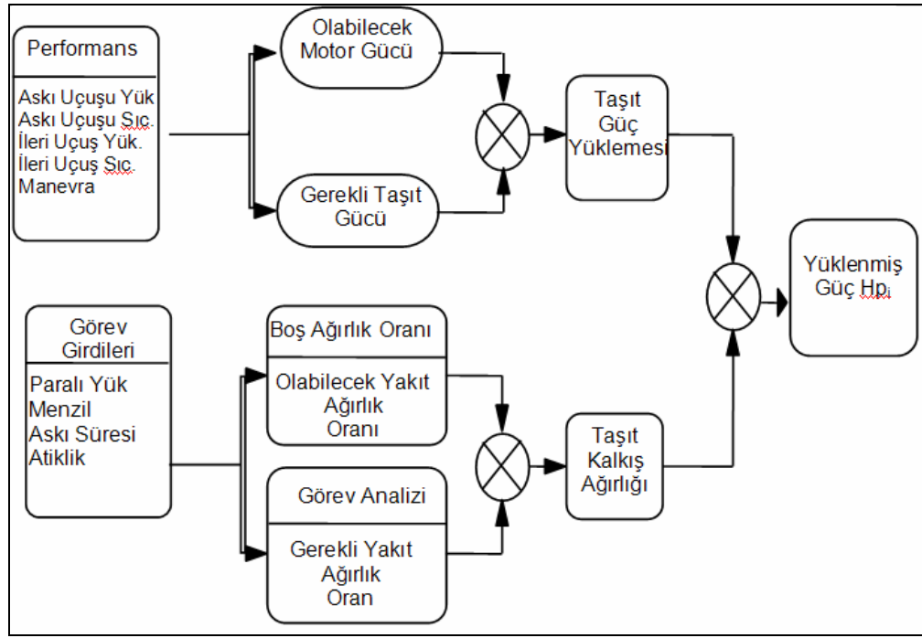
Şekil 3.1: R_F metodu genel akış şeması
