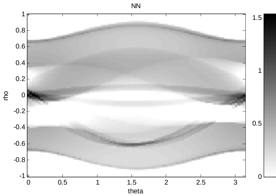
Şekil 6.9. 81x81 Shepp-Logan fontomunun sinogramı. sinogram 16,56 dak da oluşturulmuştur
