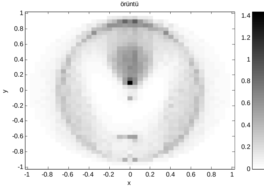
Şekil 6.7. 41x41 EM1 5 öteleme ile oluşturulmuştur. Laplace düzenlemesi (regularizasyon) ile gerçekleştirilmiştir. EM1 5 öteleme için 12,5dk da gerçekleştirilmiştir..
