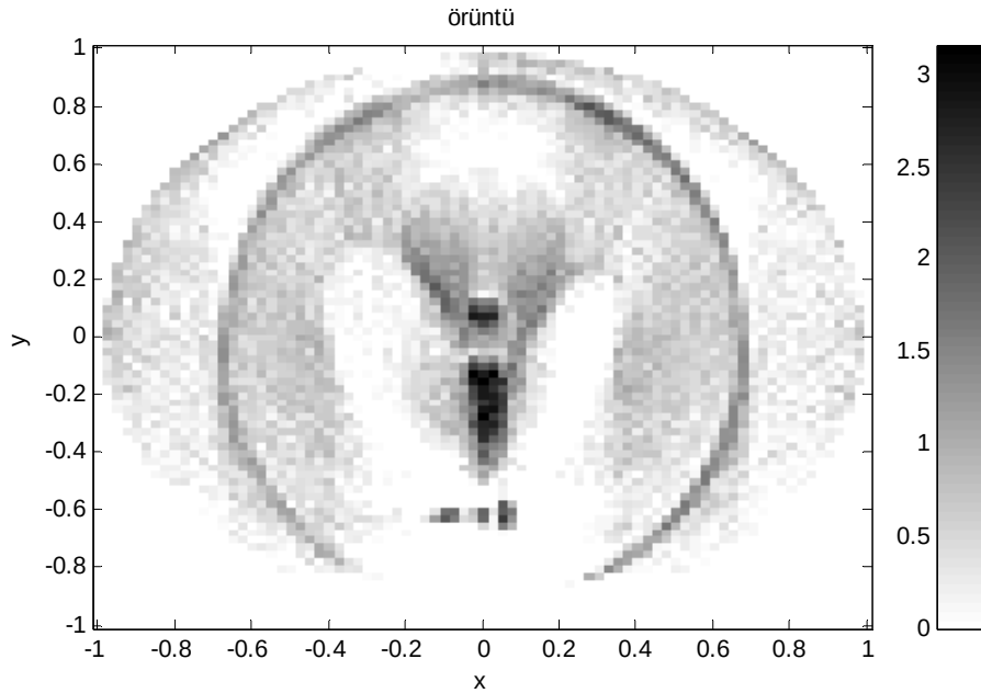
Şekil 6.39. Buradaki 81x81 görüntü ART yöntemi kullanılarak, 1 öteleme ile oluşturulmuştur. ART 1 öteleme için 36,63 dak. da gerçekleşmiştir..
