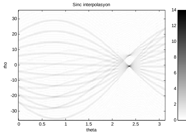
Şekil. Ek-A. 4. 51x51 piksel zayıflayan noktalar doğrusunun değişik interpolasyon stratejisi ile Radon dönüşümü (Sinc interpolasyon yöntemi ile).
