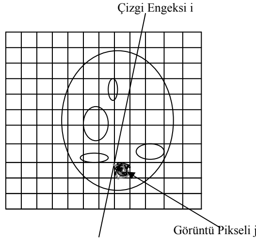
Şekil 5.1: Matris elemanı a_{ij} , i endeksli sinogram değeri ile j endeksli görüntü pikseli arasındaki ağırlık faktörü olarak değerlendirilebilir.
