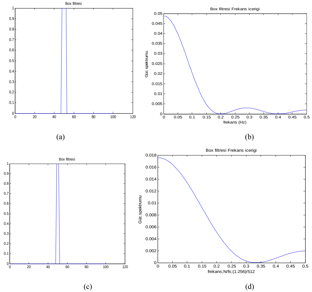
ekil 4.5: Kare(a)(48-52 arası 1) ve spektrumu(b) yanına izilmitir. Frekansı 0'dan rneklemeye frekansının yarısına kadardır. Yine kare(c)(49-51 arası 1) ve spektrumu(d) yanına izilmitir. ikinci spektrum olduka dz gzkmektedir.
