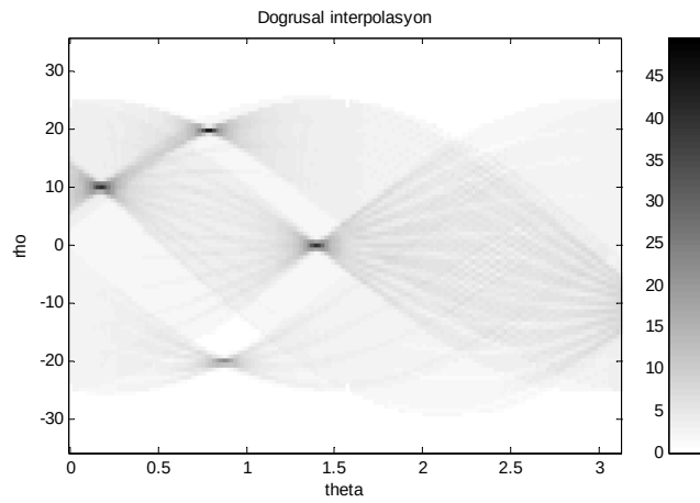
Şekil. Ek-A. 31. 51x51 piksel değişik eğimli dört çizgi doğrusunun, değişik interpolasyon stratejisi ile Radon dönüşümü (doğrusal interpolasyon yöntemi ile).
