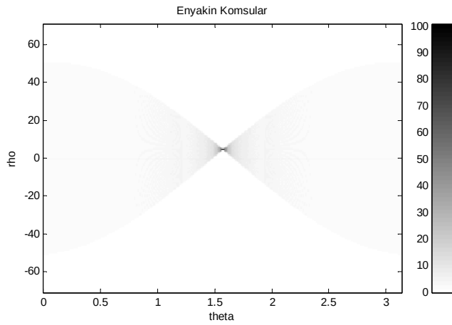
Şekil. Ek-A.42. 51x51 piksel bir nokta ile eğimi sıfır olan bir çizginin değişik interpolasyon stratejisi ile Radon dönüşümü (en yakın komşular yöntemi ile ).
