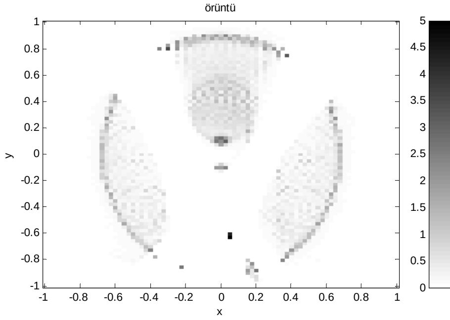
Şekil 6.21. Buradaki 81x81 görüntü EM1 kullanılarak, 40 öteleme ile oluşturulmuştur. EM1 40 öteleme için 134dk da gerçekleştirilmiştir..
