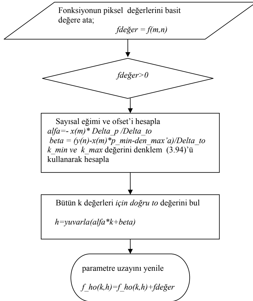
Algoritma 3.4 Optimum Hough dönüşümü
