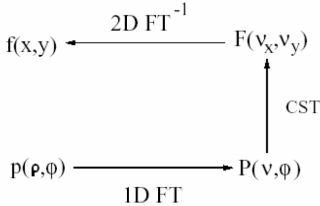
Şekil 4.3. Direkt Fourier Geri oluşturma algoritmasının şematik gösterimi
