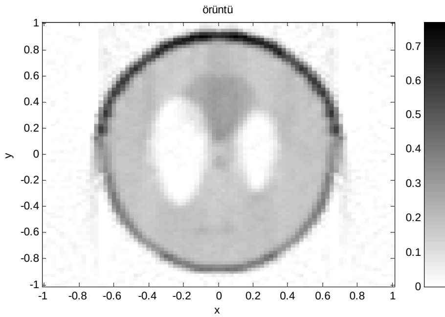
Şekil 6.57 81x81 Shepp-Logan fontomunun FBP ile geri oluşturulması. Piksel değer kestiriminde “en yakın komşular”, filtreleme için ise Hann filtresi kullanılmıştır.
