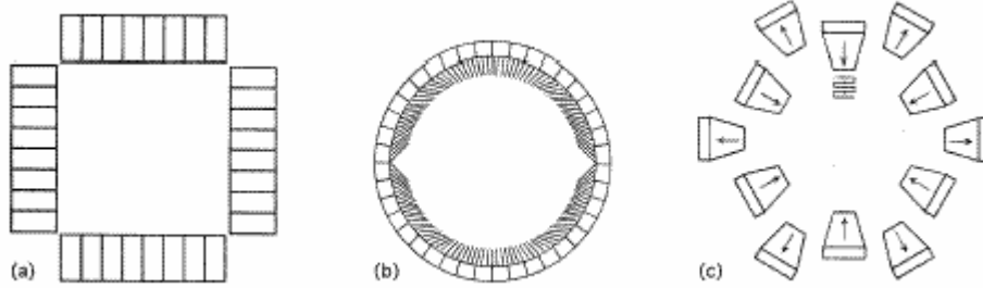
Şekil 2.17. Çok detektör tabanlı SPECT sistemleri. (a) Mark IV sistemi, sekiz bağımsız NaI(Tl)'den oluşan dört dizinli ve kare şeklindedir. (b) Headtome II dairesel detektörlerden oluşmaktadır. Detektörden projeksiyon verileri alabilmek için kolimatörleri değişik yönlere hareket ettirebilecek kanatlar konmuştur. (c) Oniki detektörden oluşan, radyal ve eğimli tarama yapabilen Cleon beyin SPECT sistemi.
