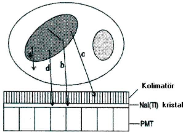
Şekil 2.16. Geleneksel nükleer tıp görüntüleme sistemi. İçeride dağılmış radyo aktif maddelerin salıverdiği gama ışınları ya fotoelektrik veya kırınım olayına karışır. Kolimatörün kabul açısından farklı açılarda gelen fotonlar kurşun kolimatörler tarafından emilirler. Kolimatörlerin kabul açısında gelen veya kolmatörlere çarpmayan fotonlar algılanırlar.
