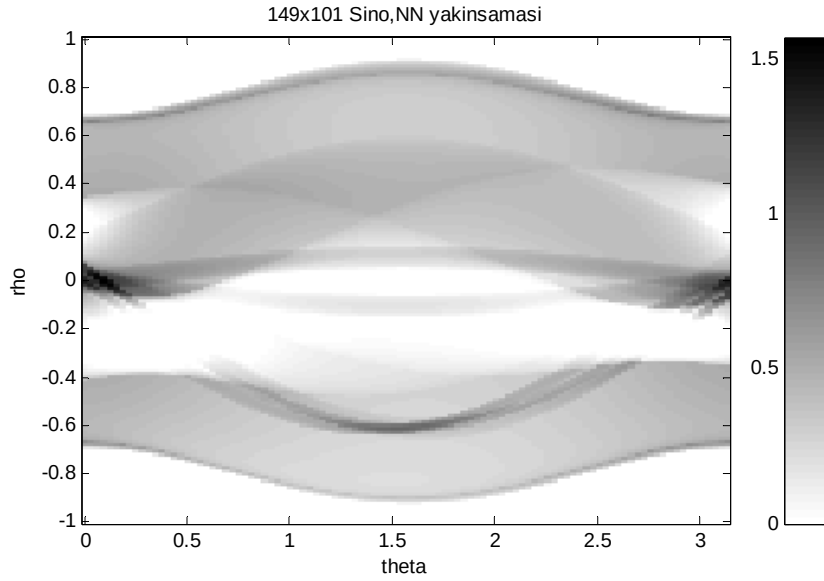
Şekil 6.58. 101x101 Shepp-Logan fontomunun sinogramı. Sinogram AMD Athlon2000 ile 160 dak da oluşturulmuştur
