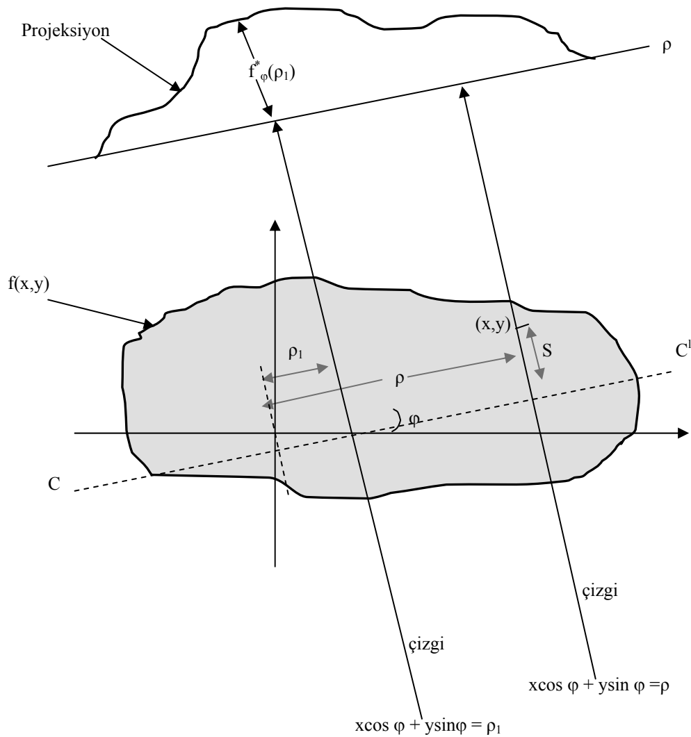
Şekil 3.2. f(x,y) nesnesi ve onun \phi açısı için Radon Dönüşümü f^*_{\phi}(\rho_1) ' in gösterimi
