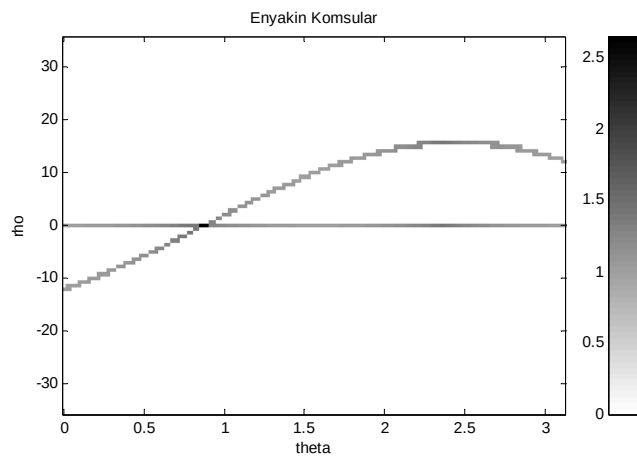
Şekil. Ek-A. 22. 51x51 piksel biri merkezde diğeri merkezden uzak olan iki noktanın, değişik interpolasyon stratejisi ile Radon dönüşümü (en yakın komşular yöntemi ile).
