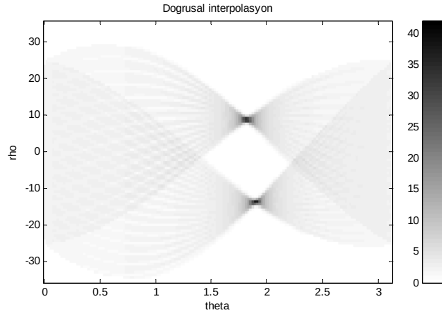
Şekil. Ek-A. 15. 51x51 piksel faklı eğimli iki çizgi doğrusunun değişik interpolasyon stratejisi ile Radon dönüşümü (dogrusal interpolasyon yöntemi ile).
