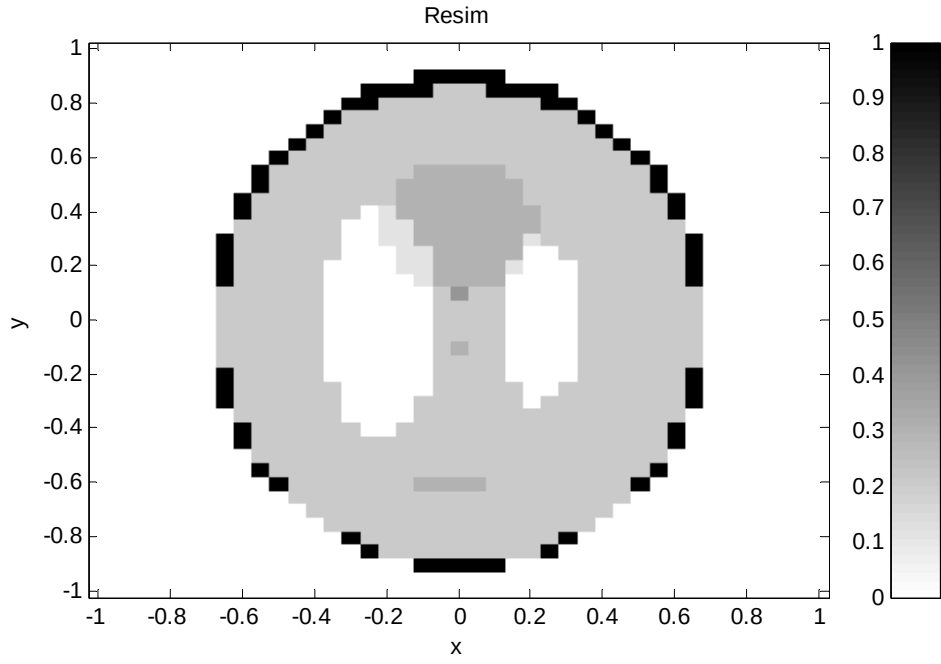
Şekil 6.3. 41x41 Shepp-Logan fontomu
