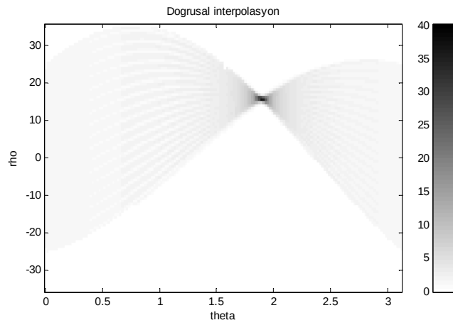
Şekil. Ek-A. 7. 51x51 piksel bir çizgi doğrusunun değişik interpolasyon stratejisi ile Radon dönüşümü (doğrusal interpolasyon yöntemi ile).
