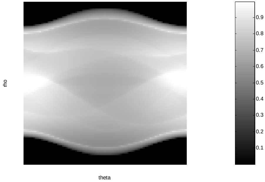
Şekil 6.2. Shepp-Logan fontomunun Radon dönüşümü.
