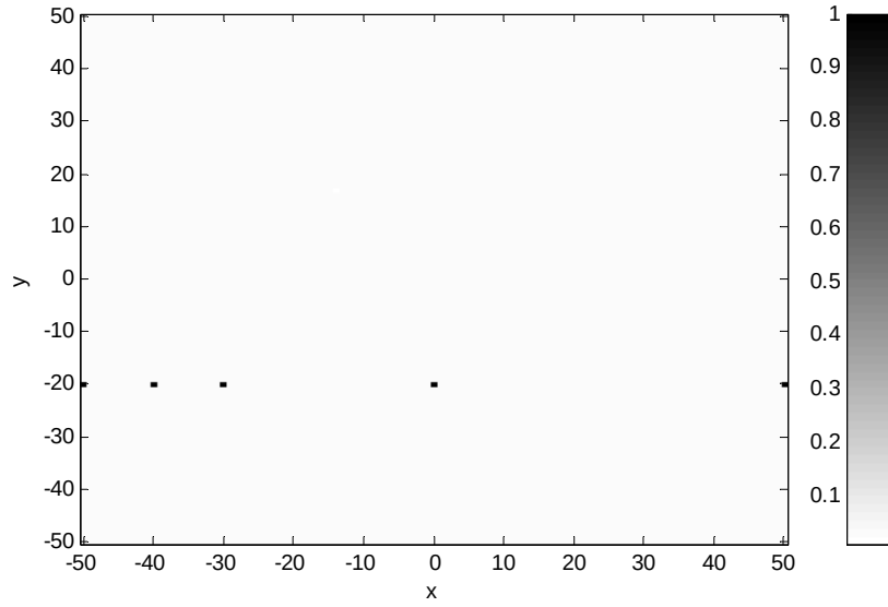
Şekil. Ek-B. 24. 101x101 piksel boyutlu, beş yatay nokta şekli
