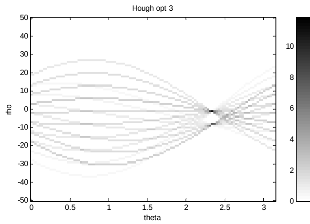
Şekil. Ek-B. 14. 101x101 piksel zayıflayan noktalar doğrusu şekli
