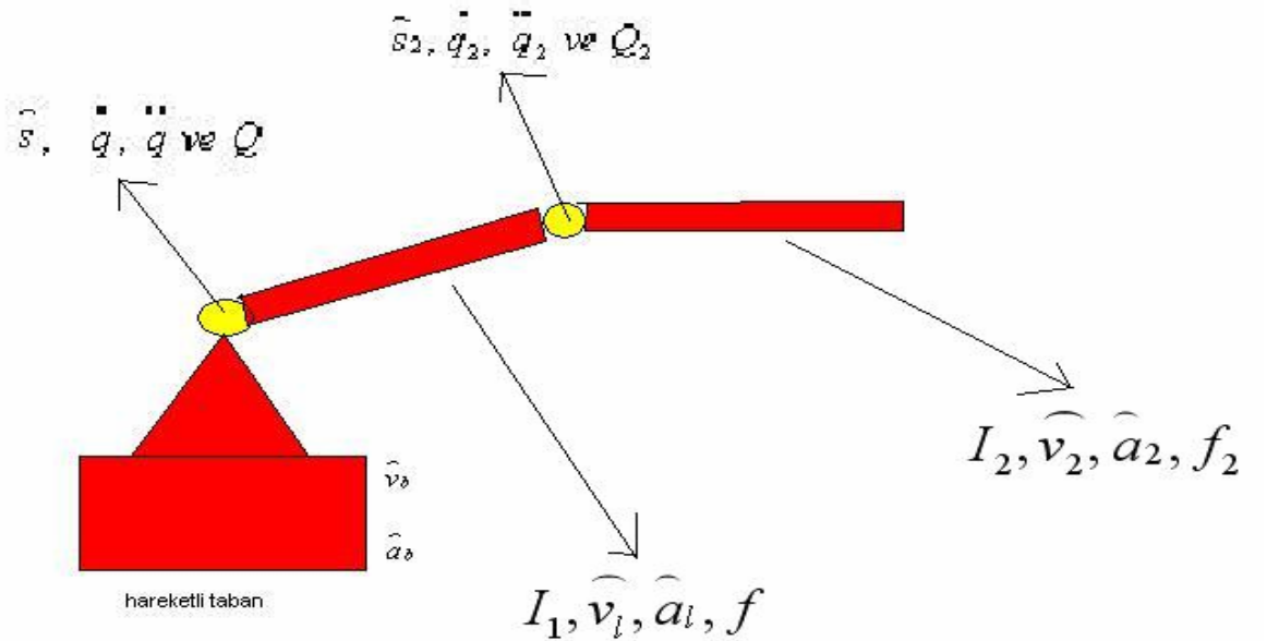
Şekil 4.2: Hareketli Tabana Sahip İki-Eklemli Robot
