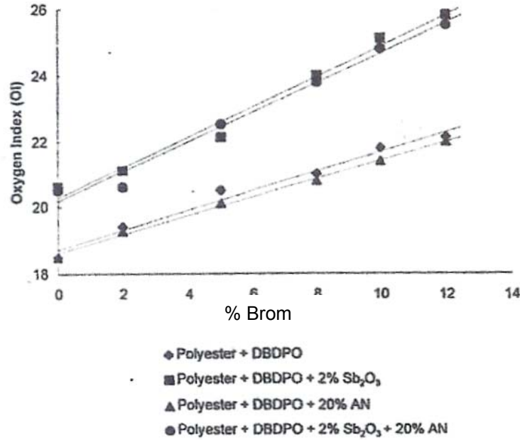
Şekil 2.7. LOI Test Sonuçları (Galip, 1999)
