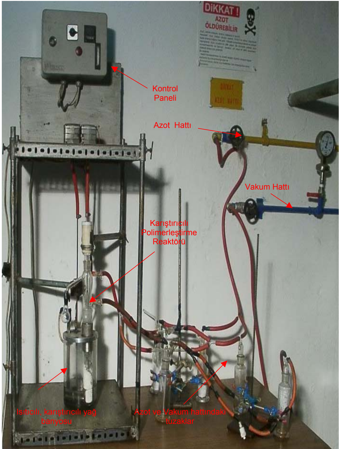
Şekil 3.1. Çalışmaların Yapıldığı Pilot tesis
