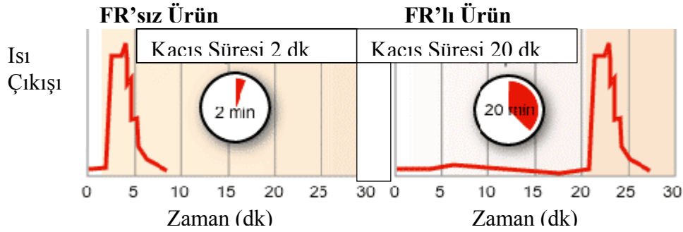
Şekil 1.3. FR'lı ve FR'sız Ürünlerin Isı çıkışı – Zaman İlişkisi
