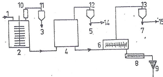
Poliester Üretiminde Polimerizasyon İşlem Dizisi
