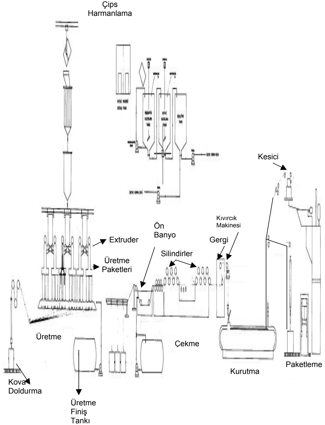
Şekil 3.4. Endüstriyel Denemelerde kullanılan Polyester Elyaf Üretim Prosesi
