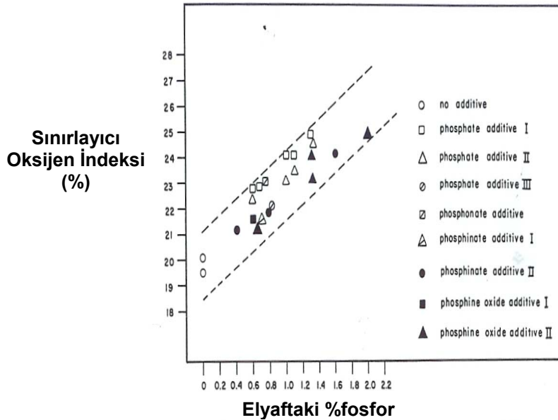
Şekil 1.18. Elyaf İçerisindeki Fosforun LOI Değerine Etkisi (Lawton, 1975)
