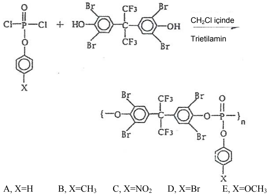
Şekil 2.1. Flor İçerikli Polifosfatların Sentezi (Liaw, 1996a)
