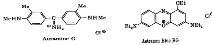
Şekil 1.19. Bazı Katyonik Boyalar
