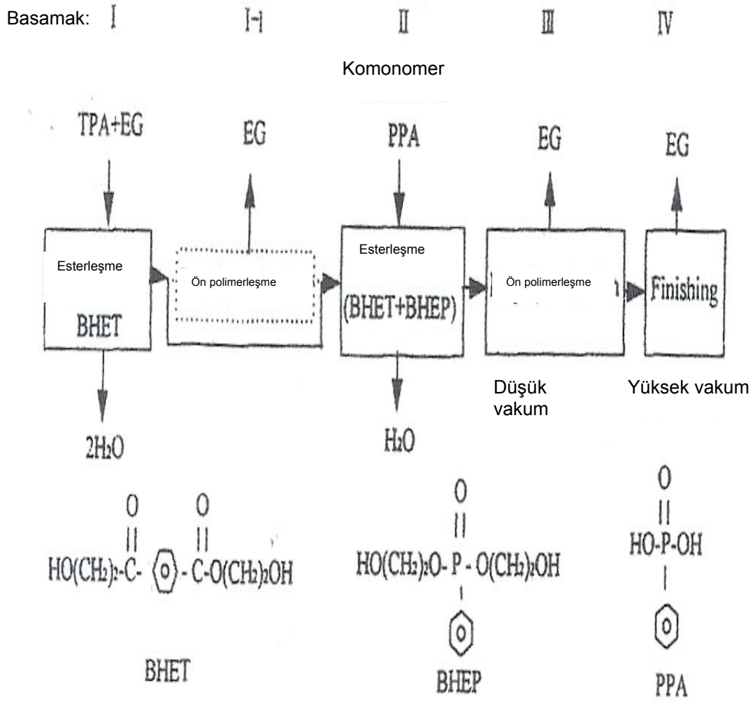
Şekil 2.4. FR polyesterin Oluşumu (Tang, 1996)
