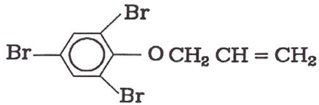
Tribromofenilalil eter
