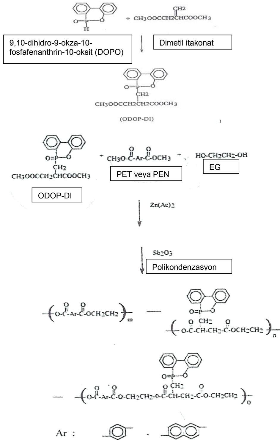
Şekil 2.5. Elde Edilen FR PET ve PEN Kopolyesterlerinin Şematik Diyagramı (Weng, 1997)
