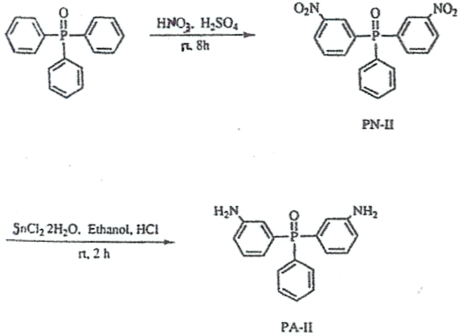
Şekil 2.3. Fosfor İçerikli Diaminin Sentezi (PAII) (Liu, 1996)
