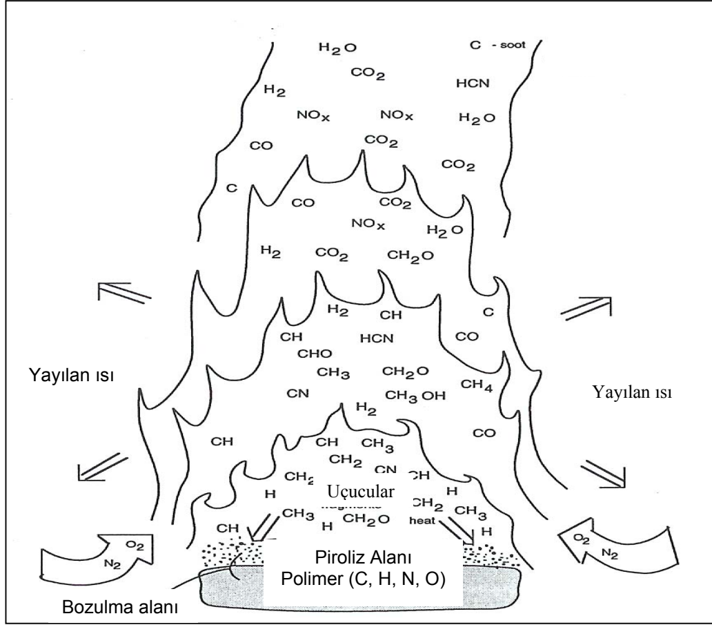
Şekil 1.6. Yanmadan Önce Bozulan Uçuşmuş Yakıtın Olduğu Yerde, Bozulma Alanını Gösteren, Organik Yakıt İçeren Alev (Nelson, 1995)
