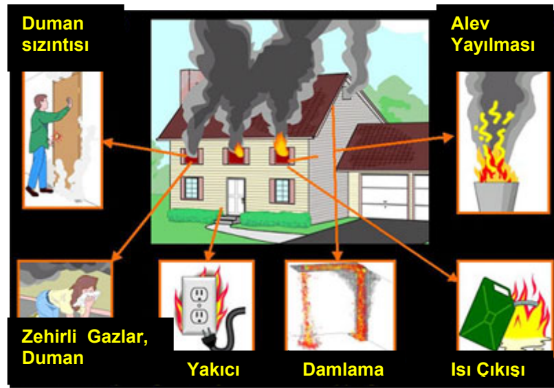
Şekil 1.1. Yangın ile İlgili Beş Anahtar
