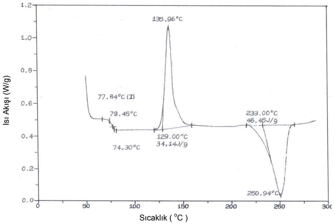
Şekil 4.2. Yanmaya Dirençli / Katyonik Boyanabilir Elyafın DSC grafiği
