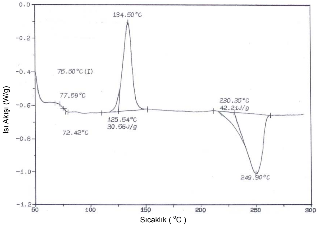
Şekil 4.1. Yanmaya Dirençli / Katyonik Boyanabilir Polimerin DSC grafiği
