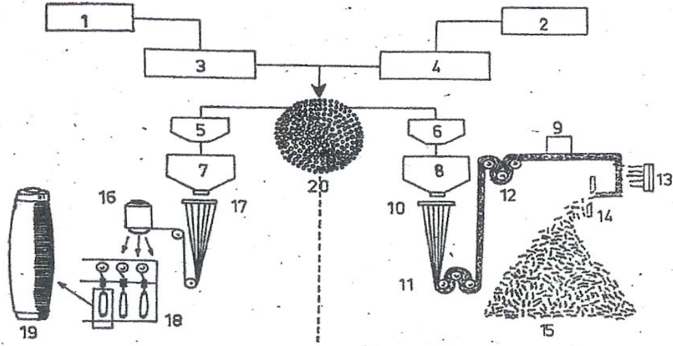
Şekil 78. Terilen Poliester Lif Üretimi
