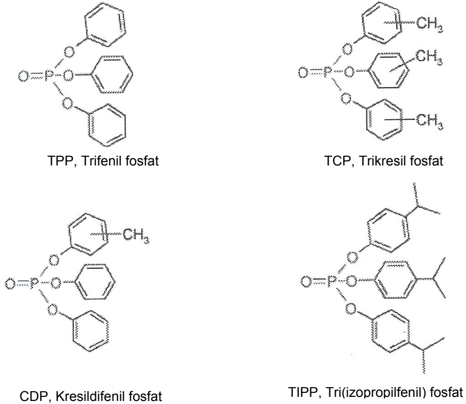
Şekil 1.10. Bazı Alkil-aril Fosfat Yanma Geciktiricileri
