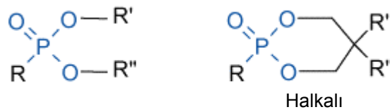
Şekil 1.11. Alkil Fosfanatların Genel Formülü
