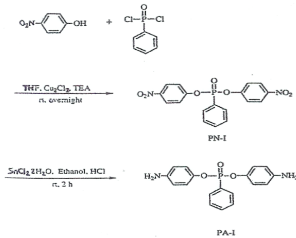
Şekil 2.2. Fosfor İçerikli Diamin'in Sentezi (PAI) (Liu,1996)
