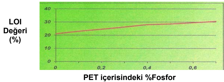
Şekil 1.17. PET İçerisinde Fosfor İçeriğine Karşılık LOI Değerinin Değişimi
