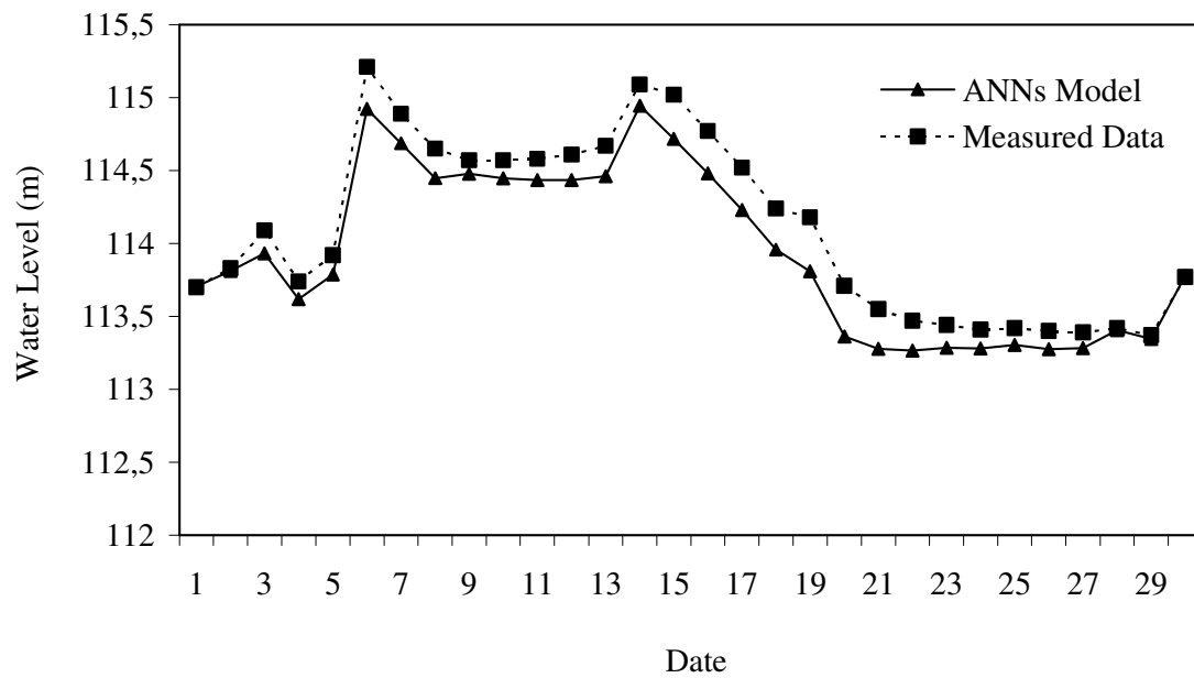
Piezometer #38
