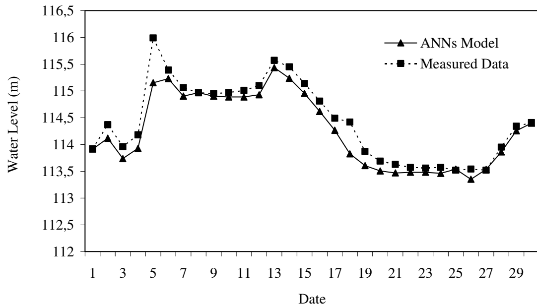
Piezometer #37
