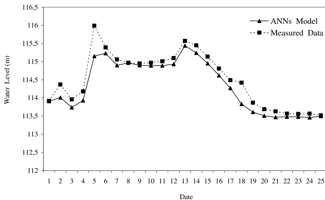
Piezometer #37
