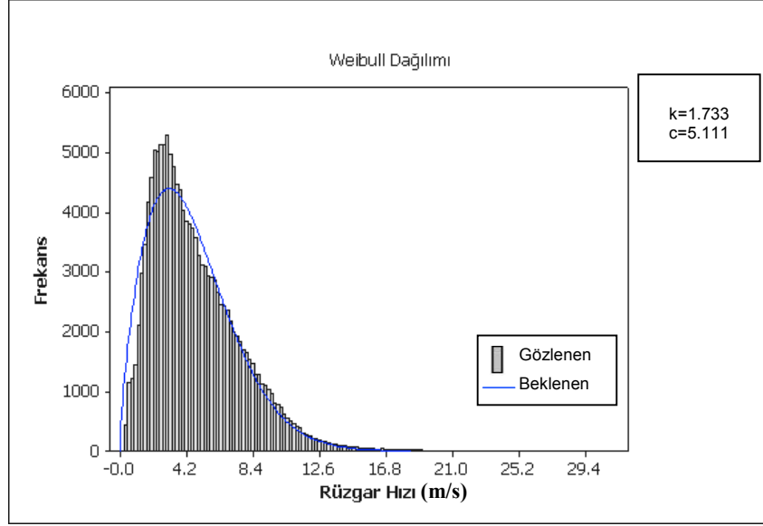
Şekil 5.3. Rüzgar Hız Verilerinin Frekans Dağılımı ile RADPE Tahmin Yöntemine Göre Teorik Weibull Dağılım Eğrisi
