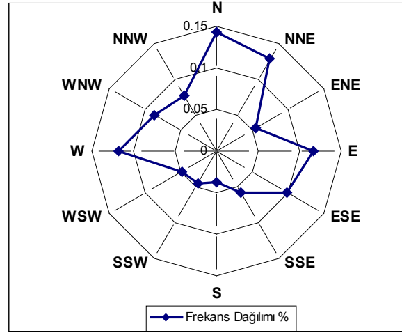
Şekil D.71. Haziran 2004 Rüzgar Yönü Frekans Dağılımı
