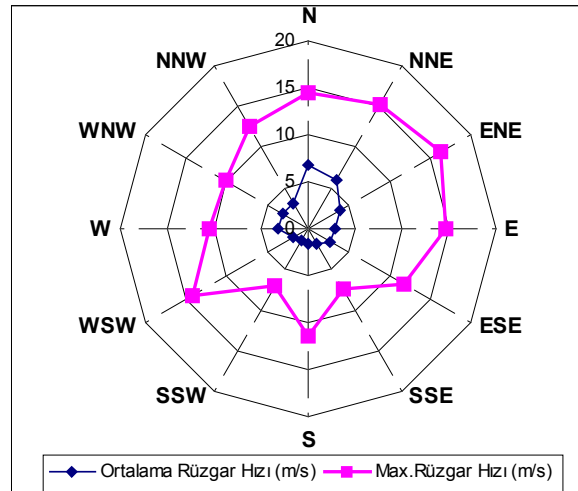
Şekil D.52. Ağustos 2003 Yönsel Rüzgar Hız Dağılımları
