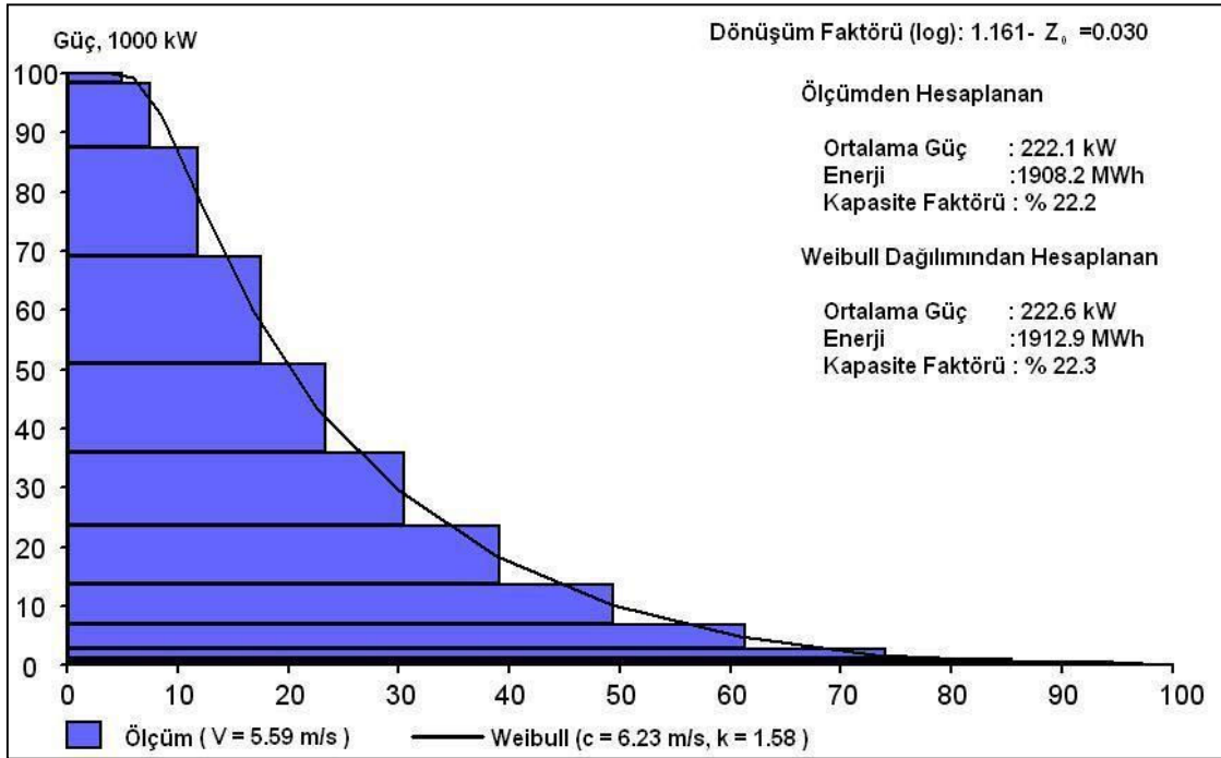
Şekil 5.49. DeWind D6 (1000) kW Rüzgar Türbini Zaman-Güç Yüzdesi Grafiği
