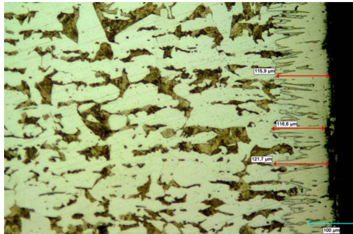
Şekil 6.6 : 1020 çeliği, 900 °C'de 4 saat borlanmış, borlu tabaka, matris ferrit ve perlit taneleri görülüyor, 200x, %2 Nital. Ortalama tabaka kalınlığı ~118.06 \mu\text{m} .
