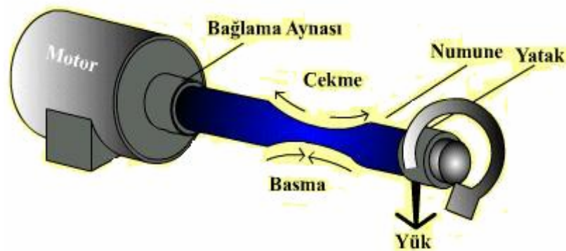
Şekil 3.1 : Dönen Destekli Kiriş Yorulma Test Düzeneği ( http://e-egitim.teknolojikarastirmalar.com/mekanik_deneyle/yorulma.htm )
