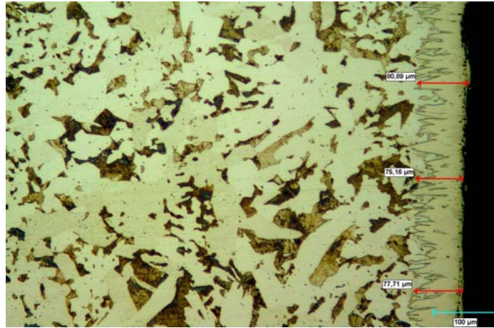
Şekil 6.5 : 1020 çeliği, 900 °C'de 2 saat borlanmış, borlu tabaka, matris ferrit ve perlit taneleri görülüyor, 200x, %2 Nital. Ortalama tabaka kalınlığı ~77.91 \mu\text{m} .
