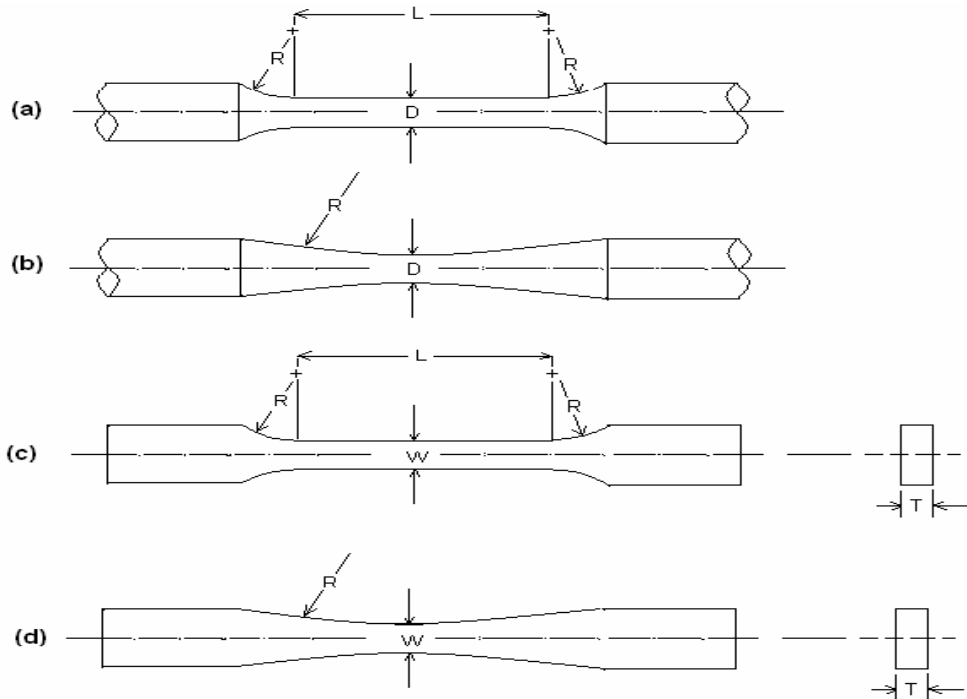
Şekil 3.8 : ASTM E – 466 ya göre aksel gerilmeli yorulma deneyi numuneleri (KAYALI, v.d., 1996)
