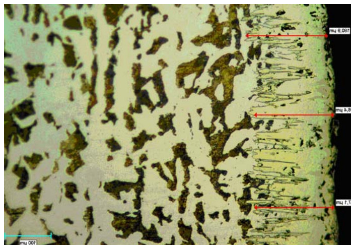
Şekil 6.7 : 1020 çeliği, 900 °C'de 6 saat borlanmış, borlu tabaka, matris ferrit ve perlit taneleri görülüyor, 200x, %2 Nital. Ortalama tabaka kalınlığı ~178.13 \mu\text{m} .
