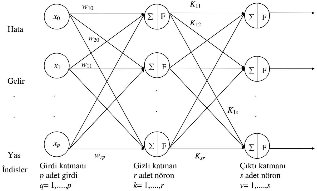
Şekil 3.5 Çok katmanlı algılayıcı (Thomas vd., 2002)
