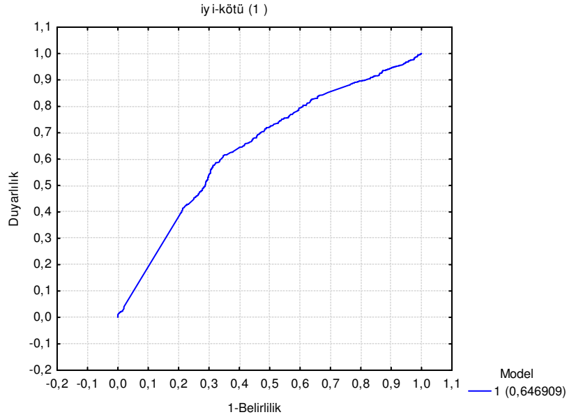
Şekil 4.2 ROC eğrisi
