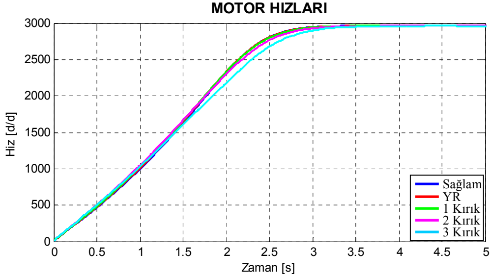
Şekil 7.82. Motor3 için benzetimle elde edilen arıza durumlarına göre çizilmiş yol alma hız grafikleri.
