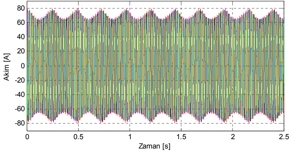
Şekil 8.12. Motor2 üç çubuğu kırık rotor için deneysel stator akımları.
