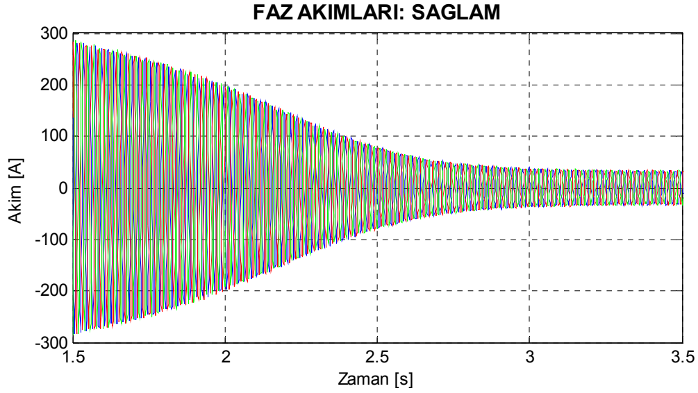
Şekil 7.50. Motor3 sağlam motor durumu için benzetimle elde edilen yol alma akımları.
