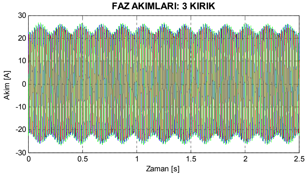
Şekil 8.24. Motor4 üç çubuğu kırık rotor için deneysel stator akımları.
