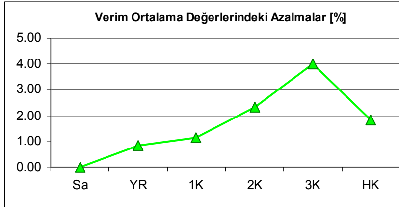
Şekil 9.11. Ortalama verim değerlerindeki azalmanın genelleştirilmiş oranlarının arızalara göre gösterimi.
