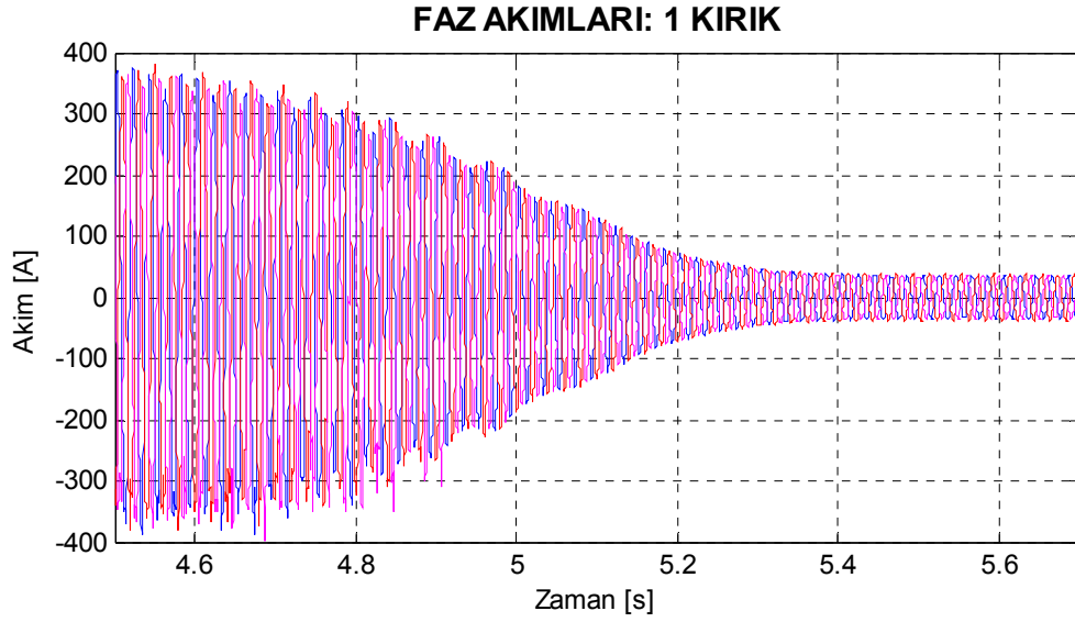
Şekil 8.49. Motor1 bir çubuğu kırık rotor için deneysel yol alma akımları.
