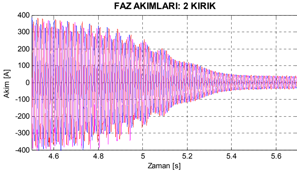
Şekil 8.50. Motor1 iki çubuğu kırık rotor için deneysel yol alma akımları.
