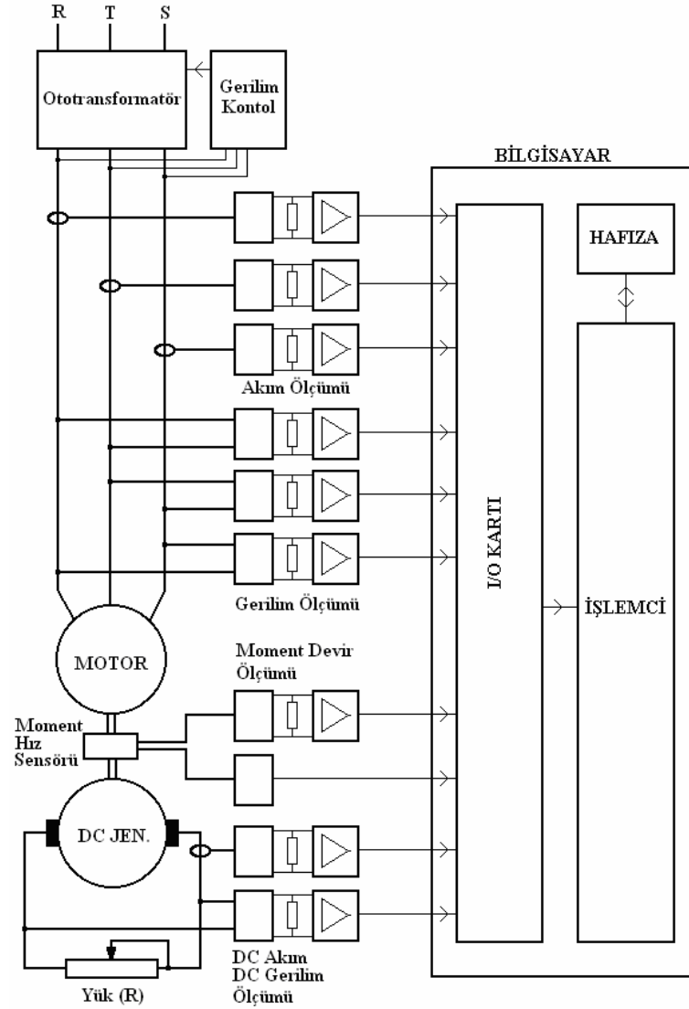
Şekil 6.1. Kullanılan deney düzeneğine ait blok şeması.
