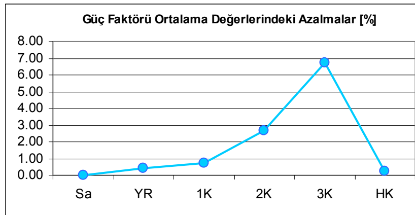
Şekil 9.7. Ortalama güç faktörü değerlerindeki azalmanın genelleştirilmiş oranlarının arızalara göre gösterimi.
