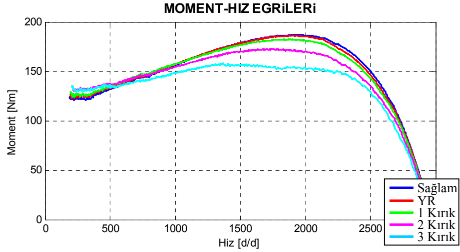
Şekil 7.86. Motor3 için benzetimle elde edilen arıza durumlarına göre çizilmiş hız-moment eğrileri.
