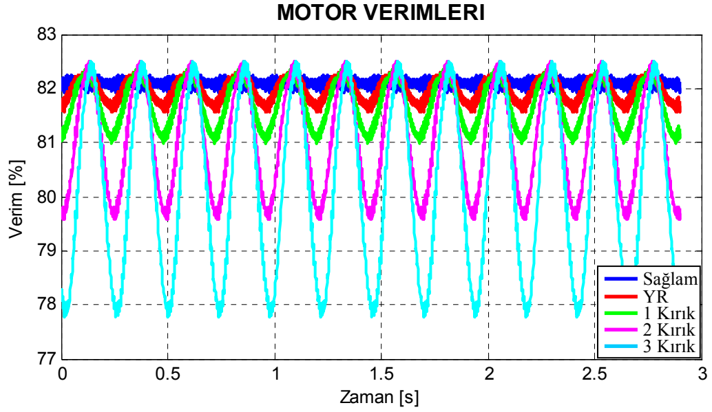
Şekil 7.37. Motor3 için benzetimle elde edilen arıza durumlarına göre çizilmiş verim grafikleri.
