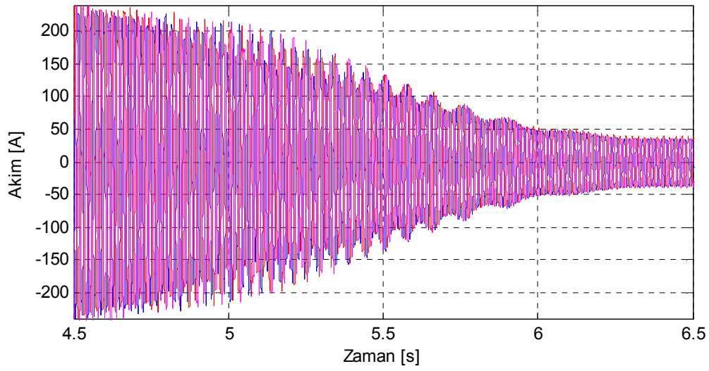
Şekil 8.63. Motor3 üç çubuğu kırık rotor için deneysel yol alma akımları.
