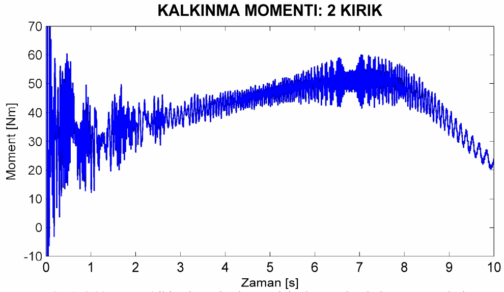
Şekil 8.92. Motor4 iki çubuğu kırık rotor için deneysel yol alma momentleri.
