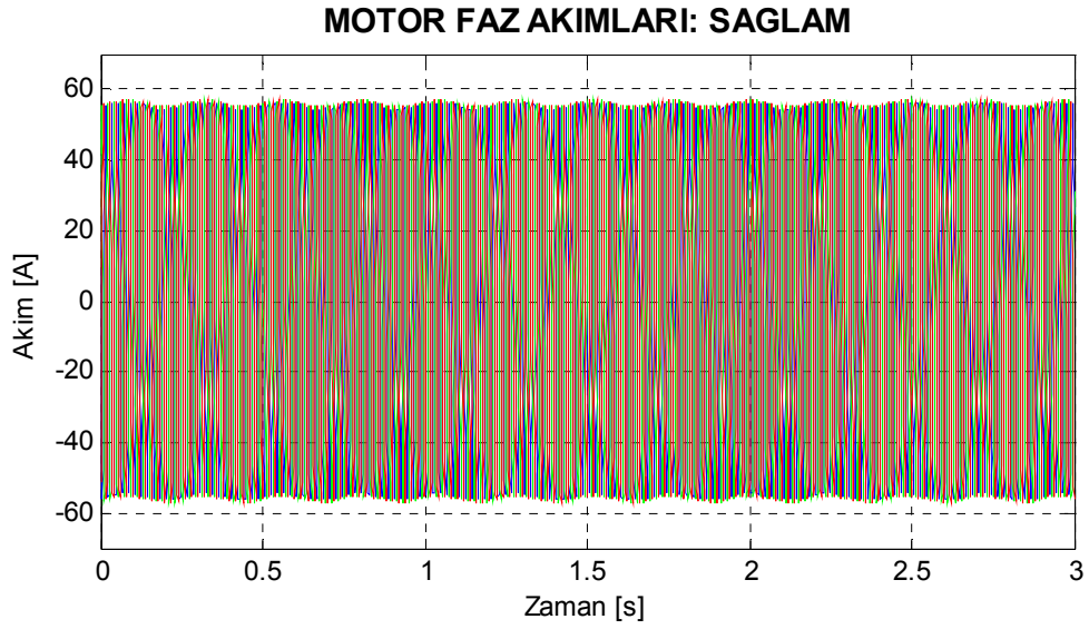
Şekil 7.12. Motor3 sağlam motor durumu için benzetimle elde edilen stator akımları.
