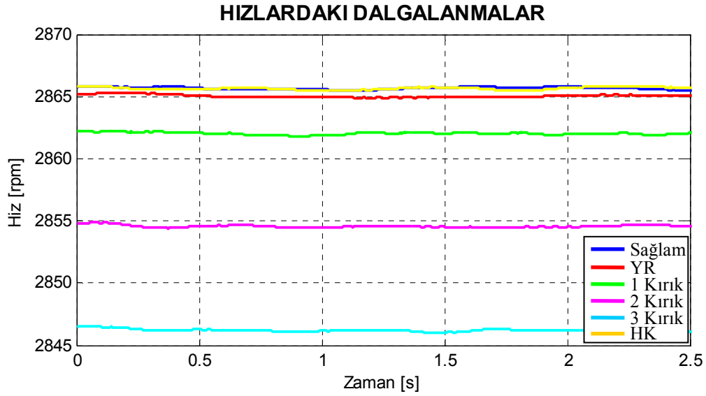
Şekil 8.33. Motor4 için deneysel arıza durumlarına göre çizilmiş hız-zaman grafikleri.
