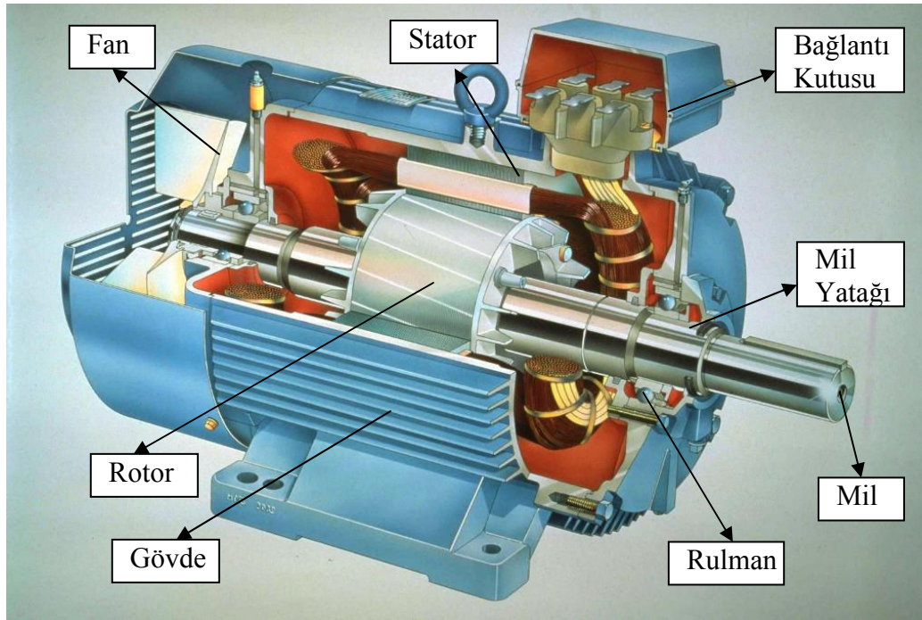
Şekil 3.2. Asenkron motor parçalarının gösterimi.
