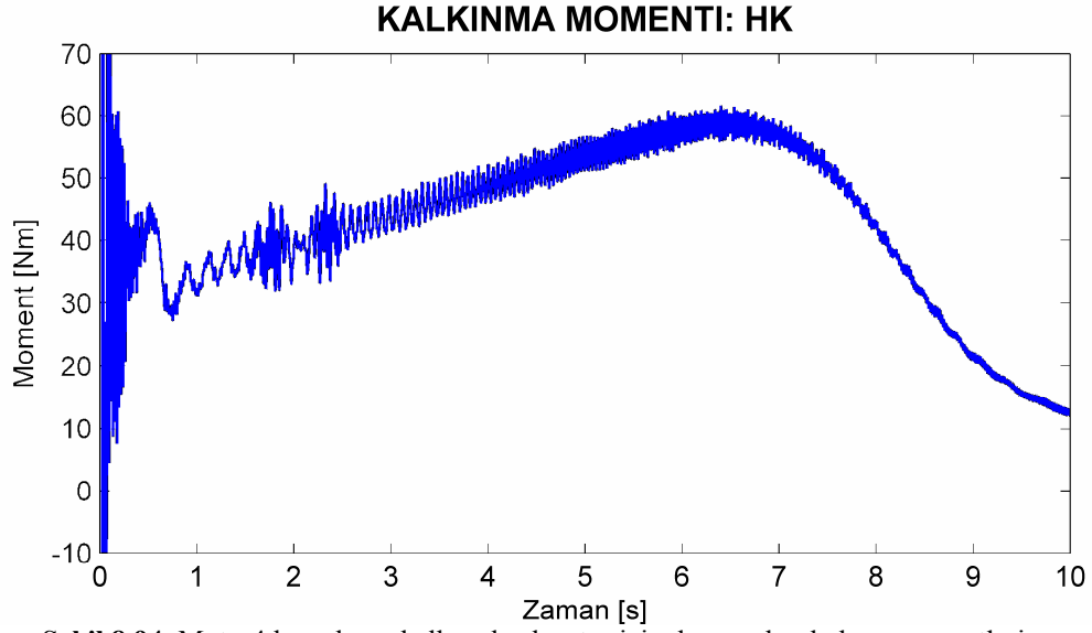
Şekil 8.94. Motor4 kısa devre halkası kırık rotor için deneysel yol alma momentleri.
