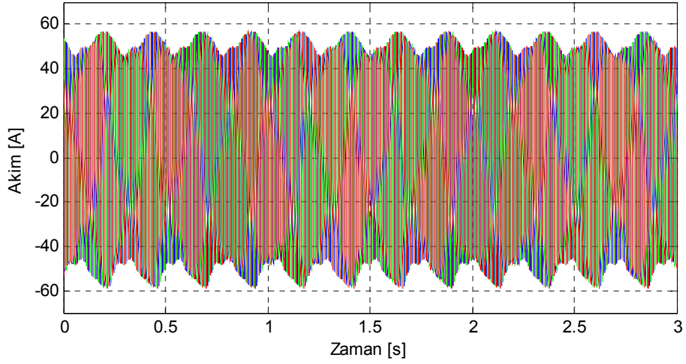
Şekil 7.16. Motor3 üç çubuğu kırık rotor için benzetimle elde edilen stator akımları.
