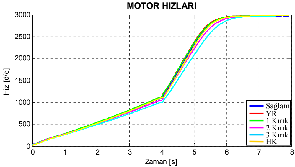
Şekil 8.97. Motor3 için arıza durumlarına göre çizilmiş deneysel yol alma hız grafikleri.
