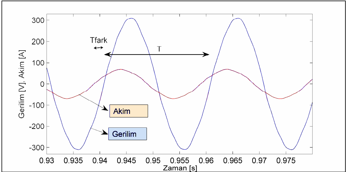
Şekil 4.3. Güç faktörünün hesaplamasında kullanılan ifadelerin gösterimi.
