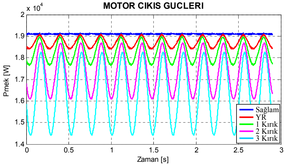
Şekil 7.33. Motor3 için benzetimle elde edilen arıza durumlarına göre çizilmiş mekanik güç grafikleri.
