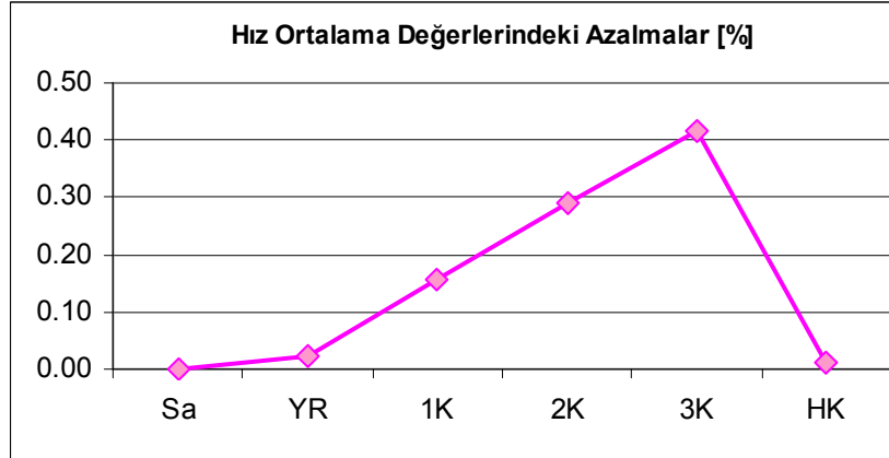
Şekil 9.5. Ortalama hız değerlerindeki azalmanın genelleştirilmiş oranlarının arızalara göre gösterimi.
