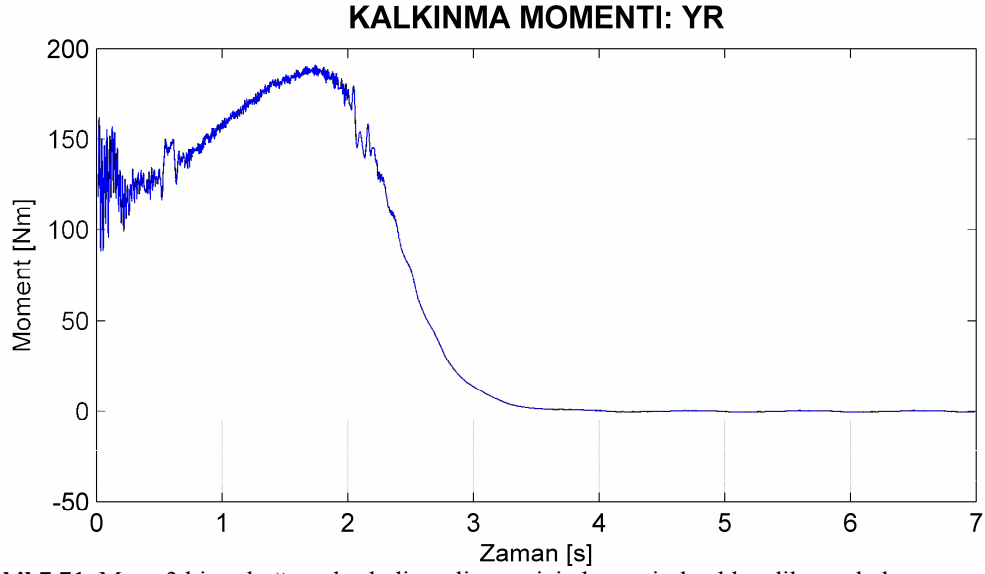
Şekil 7.71. Motor3 bir çubuğu yüksek dirençli rotor için benzetimle elde edilen yol alma momentleri.
