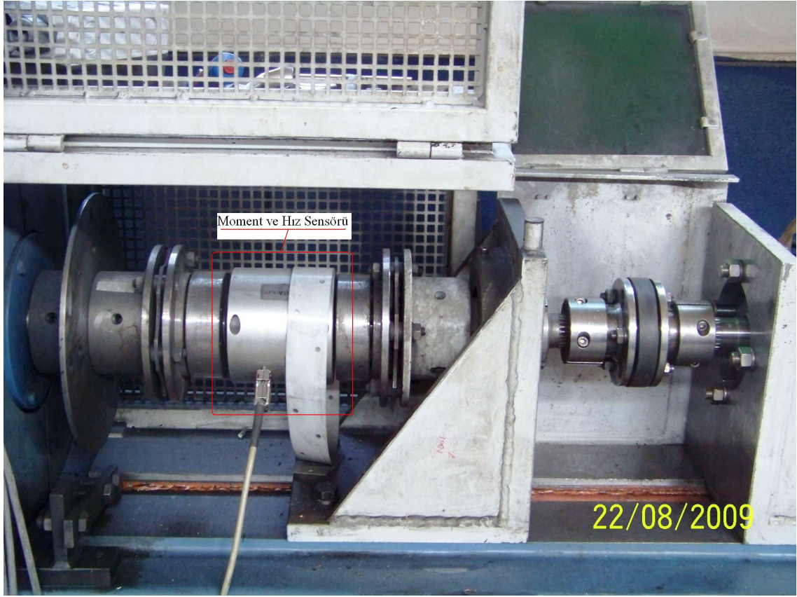
Şekil 6.6. Moment ve hız sensörü ve deney düzeneğine bağlanmış halinin fotoğrafı.
