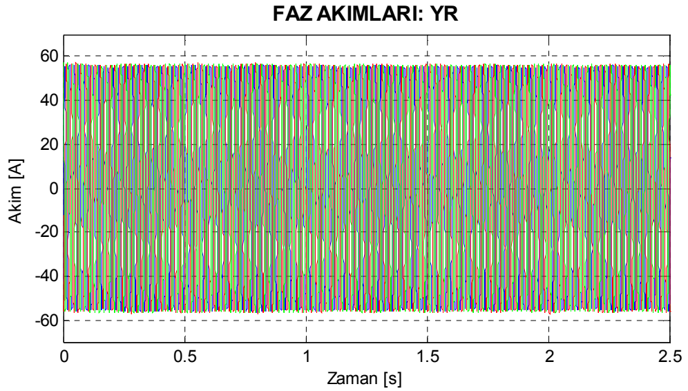
Şekil 8.15. Motor3 bir çubuğu yüksek dirençli rotor için deneysel stator akımları.
