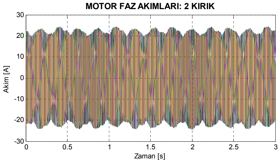
Şekil 7.20. Motor4 iki çubuğu kırık rotor için benzetimle elde edilen stator akımları.
