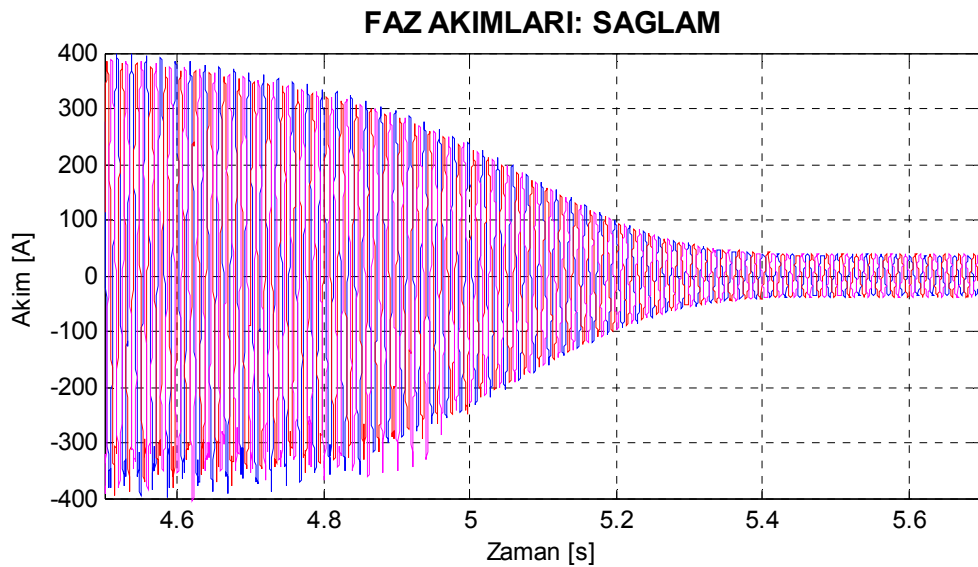
Şekil 8.47. Motor1 sağlam motor durumu için deneysel yol alma akımları.
