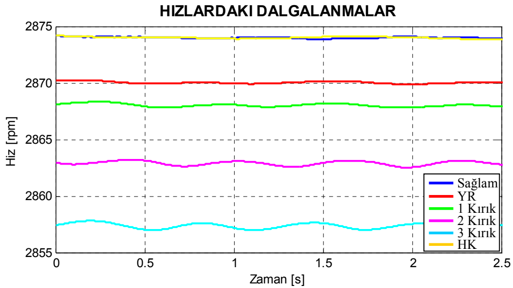
Şekil 8.32. Motor3 için deneysel arıza durumlarına göre çizilmiş hız-zaman grafikleri.
