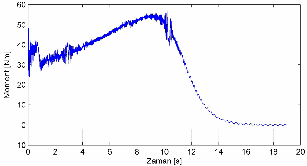
Şekil 7.76. Motor4 bir çubuğu yüksek dirençli rotor için benzetimle elde edilen yol alma momentleri.
