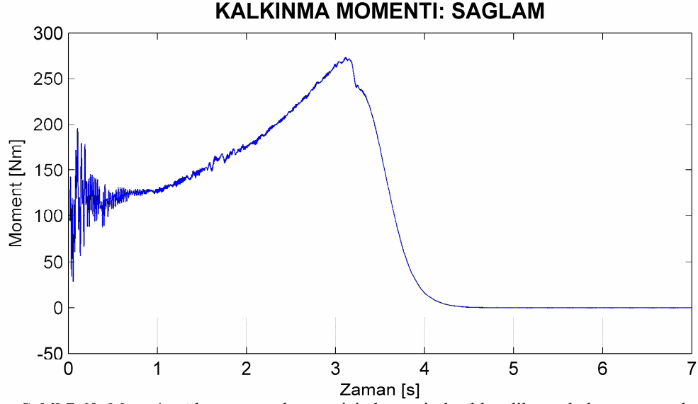
Şekil 7.60. Motor1 sağlam motor durumu için benzetimle elde edilen yol alma momentleri.
