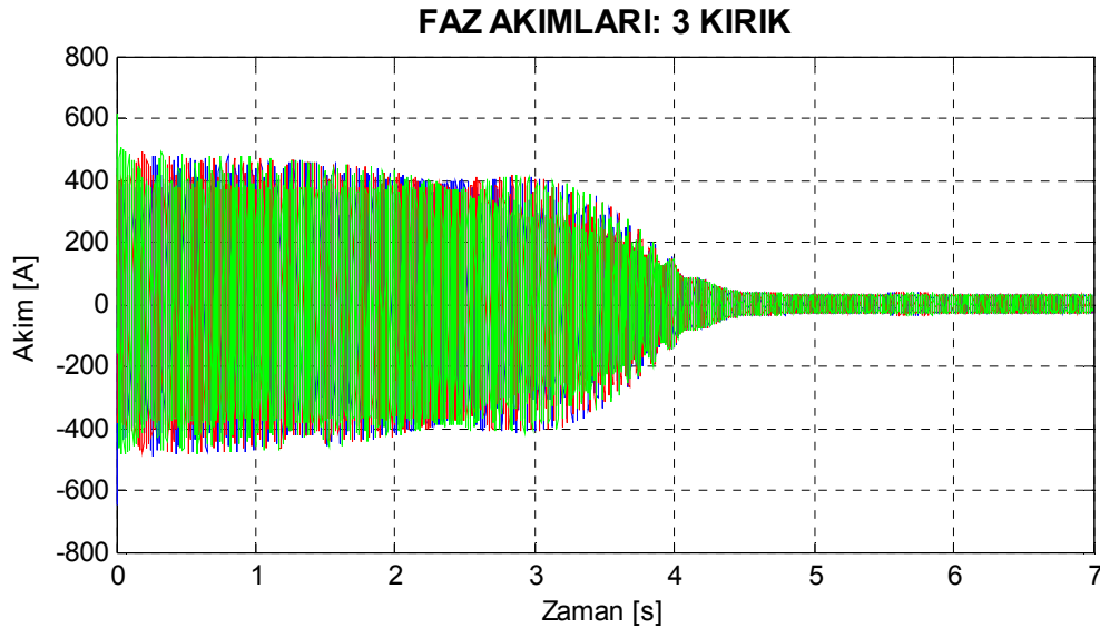
Şekil 7.39. Benzetimle elde edilen Motor1 üç kırık çubuklu rotor arızası için yol alma sürecinin tamamını içeren motor akım grafiği.
