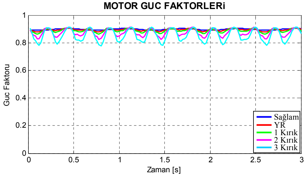
Şekil 7.30. Motor4 için benzetimle elde edilen arıza durumlarına göre çizilmiş güç faktörü grafikleri.
