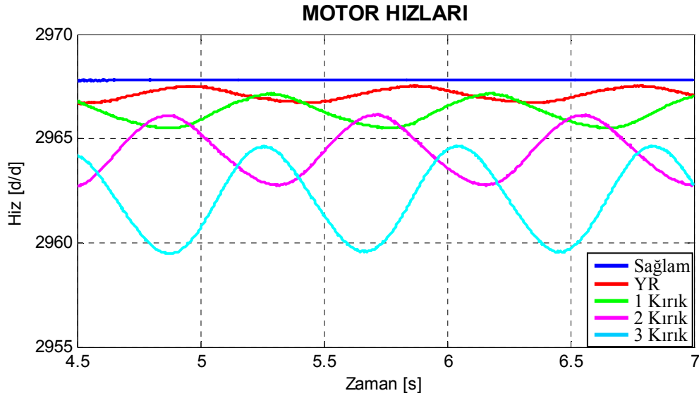
Şekil 7.25. Motor3 için benzetimle elde edilen arıza durumlarına göre çizilmiş hız-zaman grafikleri.
