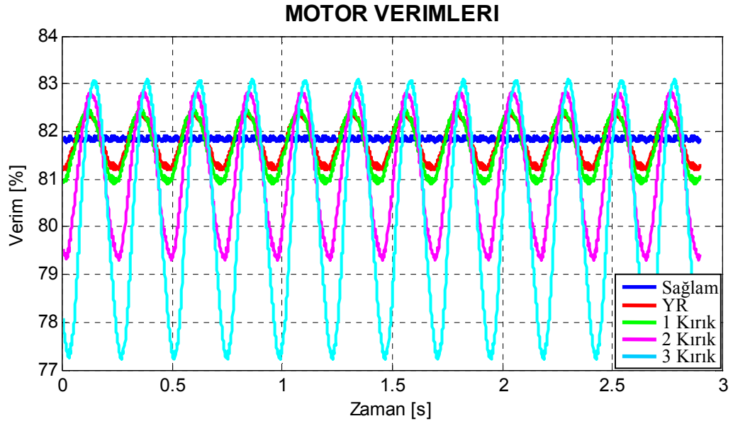
Şekil 7.36. Motor2 için benzetimle elde edilen arıza durumlarına göre çizilmiş verim grafikleri.
