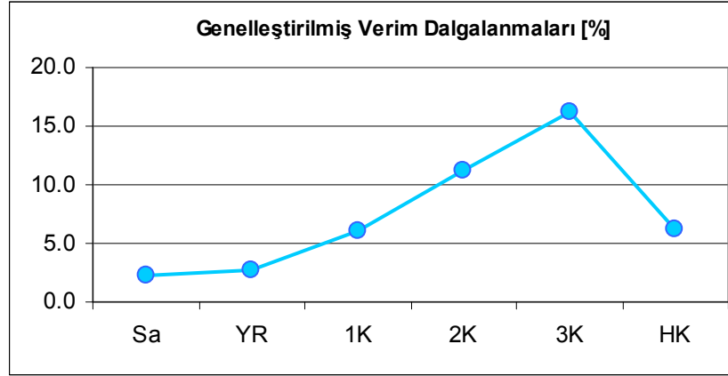
Şekil 9.10. Arızalara göre motor verimlerindeki genelleştirilmiş dalgalanma oranları.
