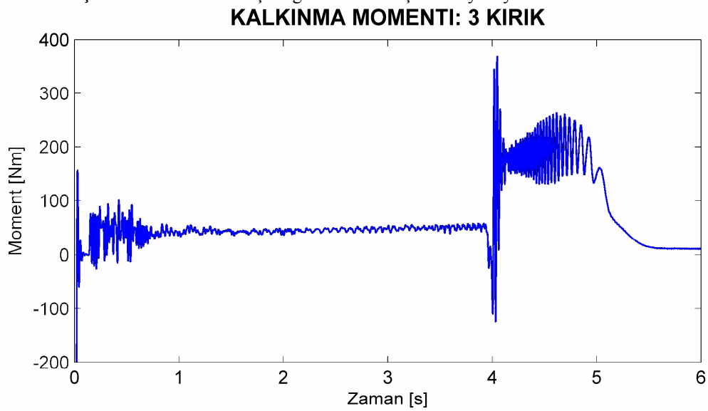
Şekil 8.75. Motor1 üç çubuğu kırık rotor için deneysel yol alma momentleri.
