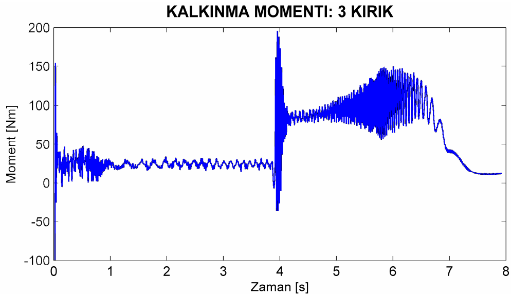
Şekil 8.81. Motor2 üç çubuğu kırık rotor için deneysel yol alma momentleri.
