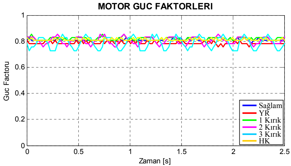
Şekil 8.37. Motor4 için deneysel arıza durumlarına göre çizilmiş güç faktörü grafikleri.
