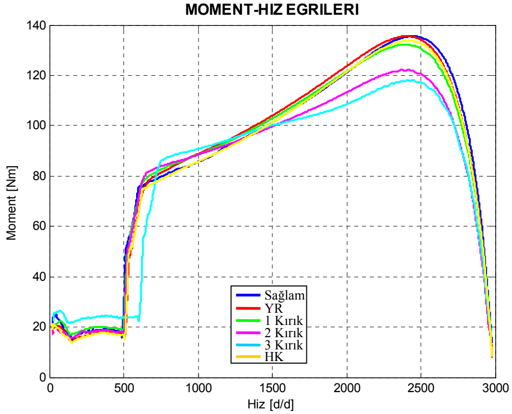
Şekil 8.100. Motor2 için arıza durumlarına göre çizilmiş deneysel hız-moment eğrileri.
