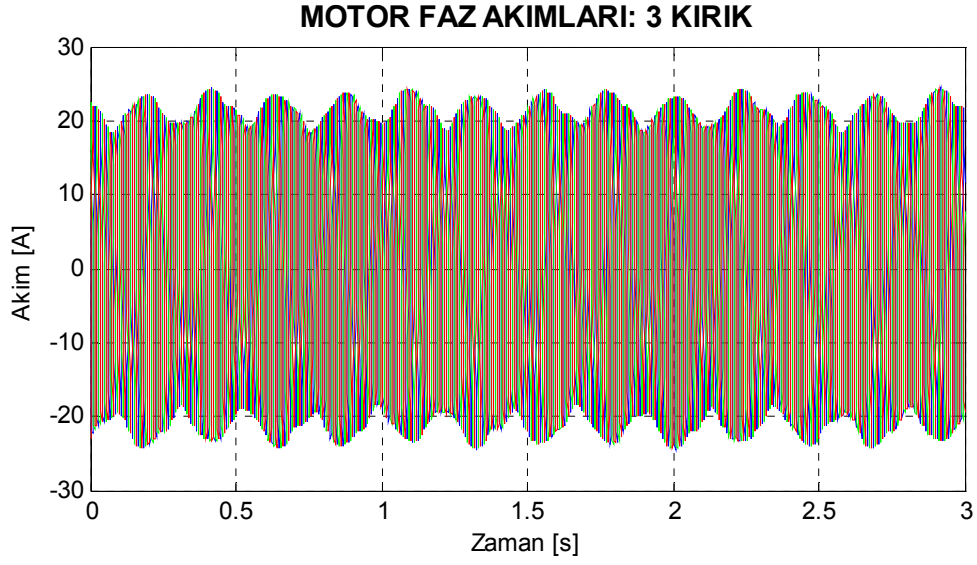
Şekil 7.21. Motor4 üç çubuğu kırık rotor için benzetimle elde edilen stator akımları.
