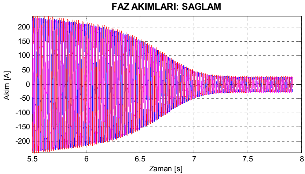
Şekil 8.53. Motor2 sağlam motor durumu için deneysel yol alma akımları.
