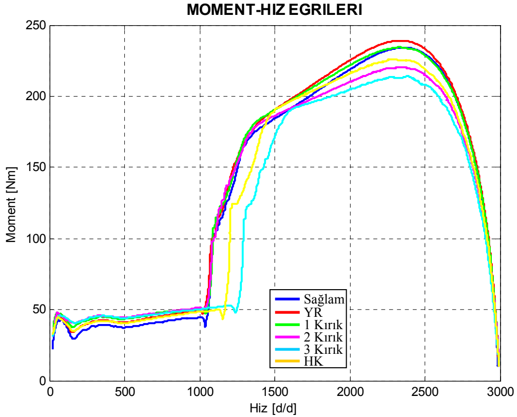
Şekil 8.99. Motor1 için arıza durumlarına göre çizilmiş deneysel hız-moment eğrileri.
