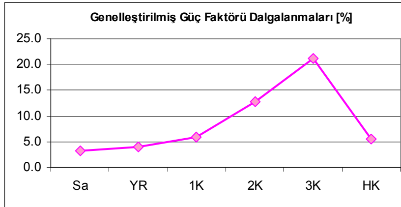
Şekil 9.6. Arızalara göre motor güç faktörlerindeki genelleştirilmiş dalgalanma oranları.
