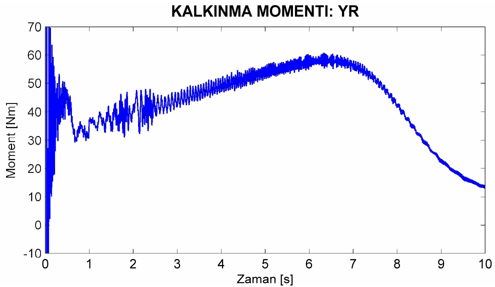
Şekil 8.90. Motor4 bir çubuğu yüksek dirençli rotor için deneysel yol alma momentleri.
