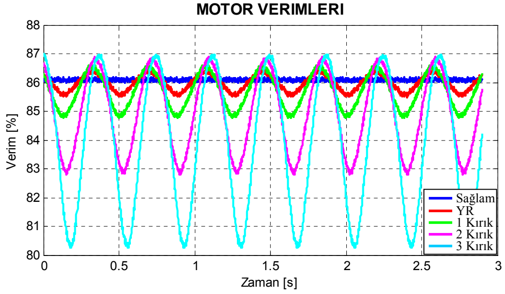
Şekil 7.35. Motor1 için benzetimle elde edilen arıza durumlarına göre çizilmiş verim grafikleri.
