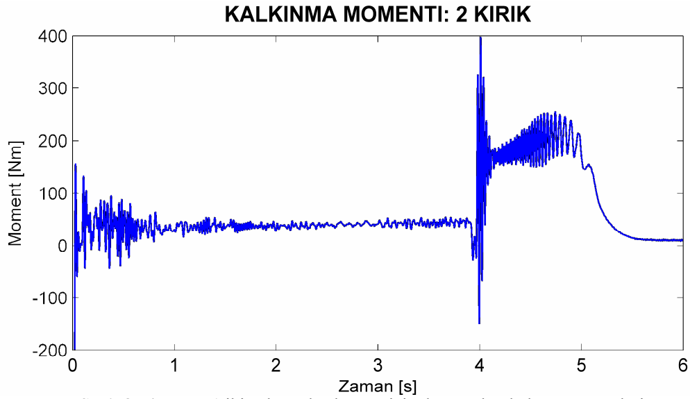
Şekil 8.74. Motor1 iki çubuğu kırık rotor için deneysel yol alma momentleri.
