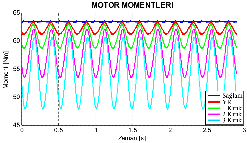
Şekil 7.25. Motor3 için benzetimle elde edilen arıza durumlarına göre çizilmiş moment grafikleri.
