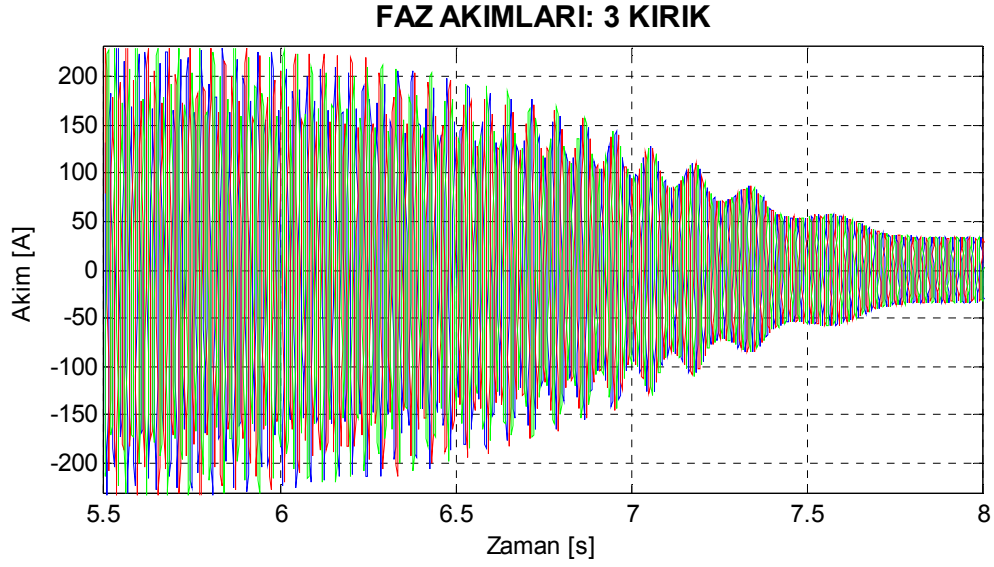
Şekil 7.49. Motor2 üç çubuğu kırık rotor için benzetimle elde edilen yol alma akımları.
