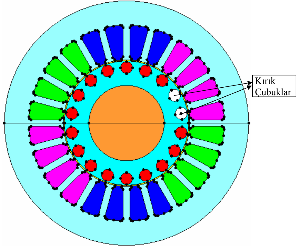
Şekil 5.6. Motor1’de iki kırık çubuk arızası benzetimi için seçilen rotor çubuklarının kesitte gösterimi.
