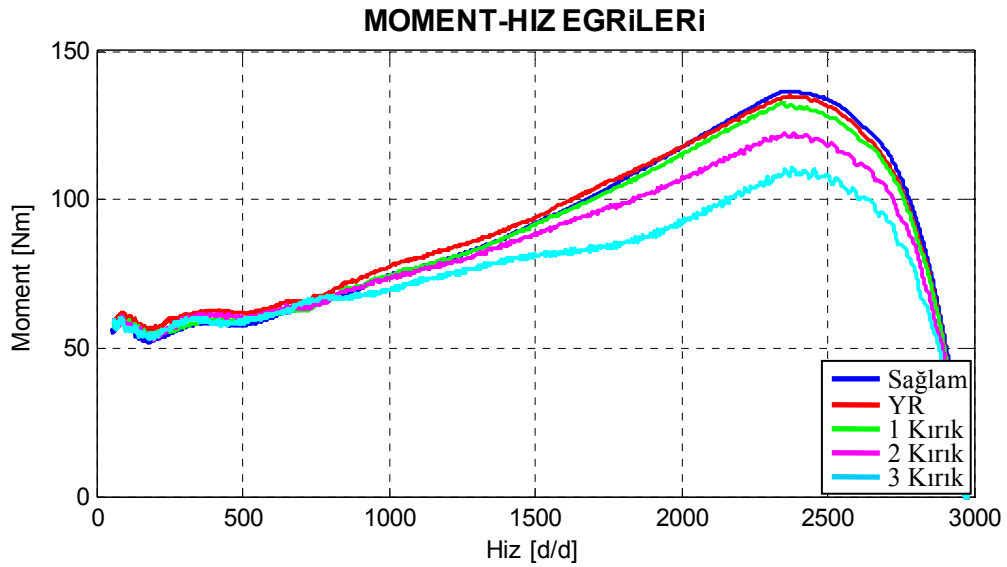
Şekil 7.85. Motor2 için benzetimle elde edilen arıza durumlarına göre çizilmiş hız-moment eğrileri.
