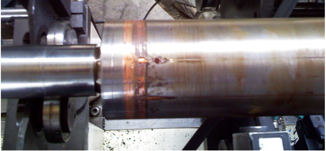
Şekil 6.11. Yüksek dirençli çubuk bulunan rotorun fotoğrafı.
