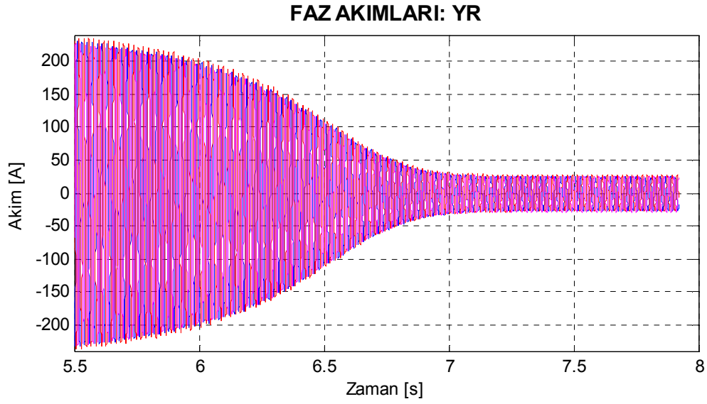
Şekil 8.54. Motor2 bir çubuğu yüksek dirençli rotor için deneysel yol alma akımları.
