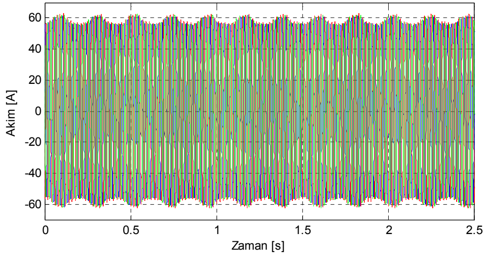
Şekil 8.17. Motor3 iki çubuğu kırık rotor için deneysel stator akımları.
