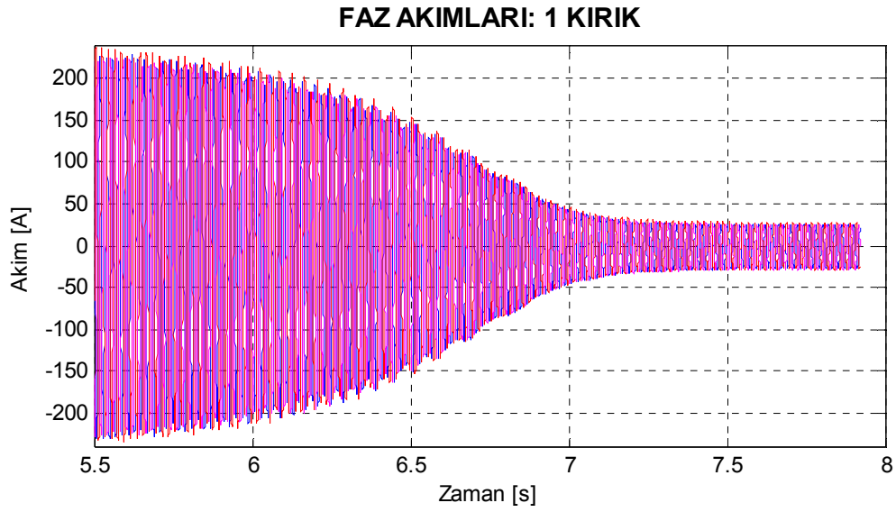
Şekil 8.55. Motor2 bir çubuğu kırık rotor için deneysel yol alma akımları.
