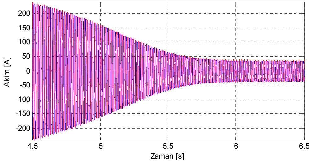
Şekil 8.64. Motor3 kısa devre halkası kırık rotor için deneysel yol alma akımları.
