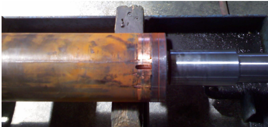
Şekil 6.14. Kısa devre halkası kırık rotorun fotoğrafı.
