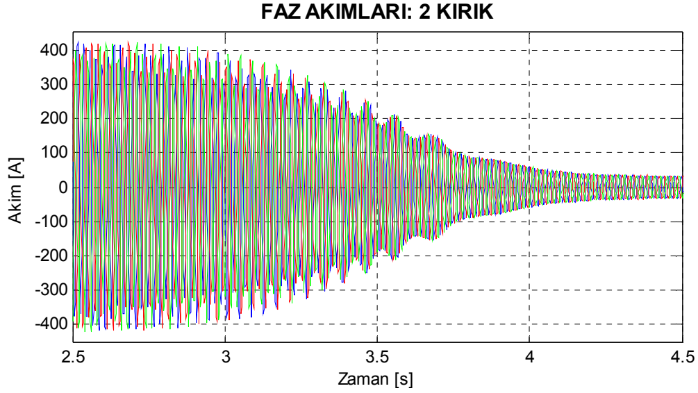
Şekil 7.43. Motor1 iki çubuğu kırık rotor için benzetimle elde edilen yol alma akımları.
