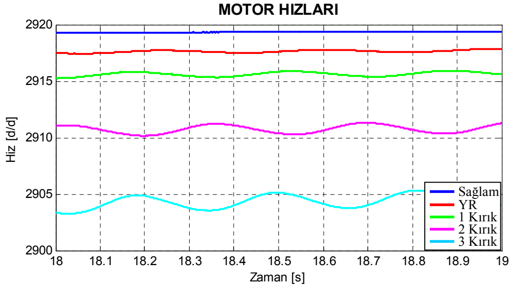
Şekil 7.26. Motor4 için benzetimle elde edilen arıza durumlarına göre çizilmiş hız-zaman grafikleri.
