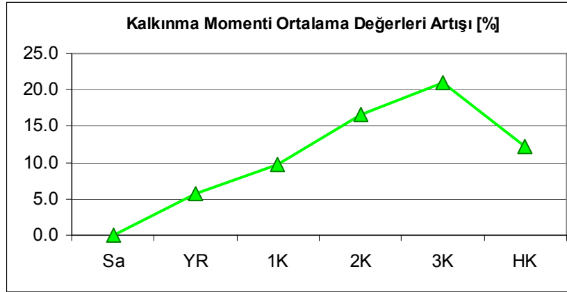
Şekil 9.16. Hız-moment eğrisindeki kalkınma momentlerinin arızalara göre yükselme oranları.
