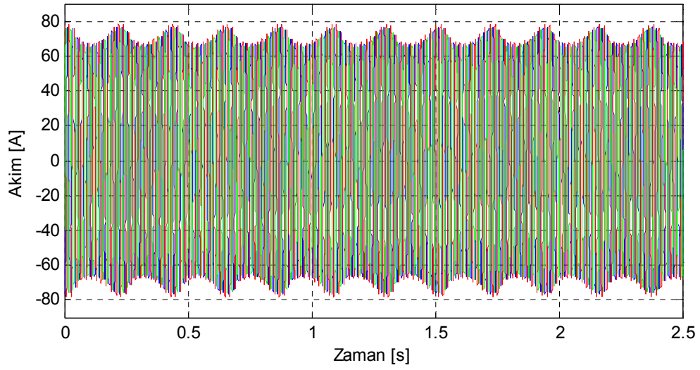
Şekil 8.11. Motor2 iki çubuğu kırık rotor için deneysel stator akımları.
