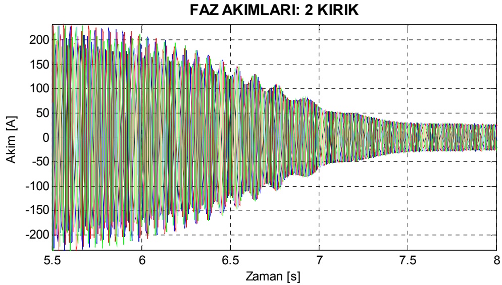
Şekil 7.48. Motor2 iki çubuğu kırık rotor için benzetimle elde edilen yol alma akımları.
