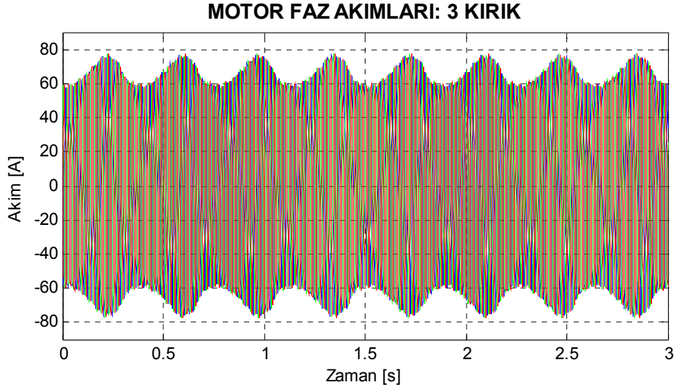
Şekil 7.6. Motor1 üç çubuğu kırık rotor için benzetimle elde edilen stator akımları.
