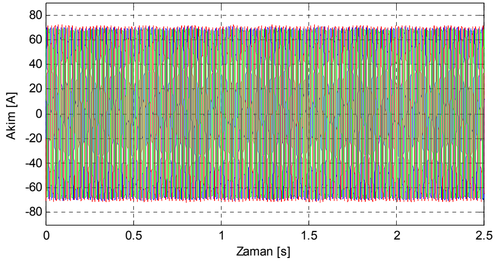
Şekil 8.8. Motor2 sağlam motor durumu için deneysel stator akımları.
