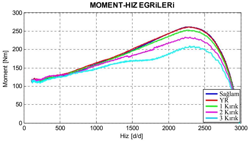
Şekil 7.84. Motor1 için benzetimle elde edilen arıza durumlarına göre çizilmiş hız-moment eğrileri.
