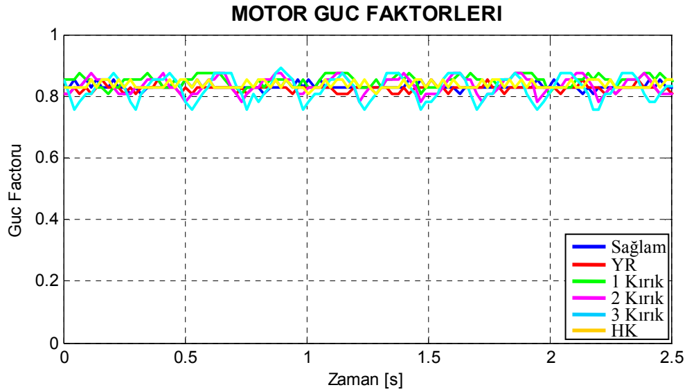
Şekil 8.36. Motor3 için deneysel arıza durumlarına göre çizilmiş güç faktörü grafikleri.
