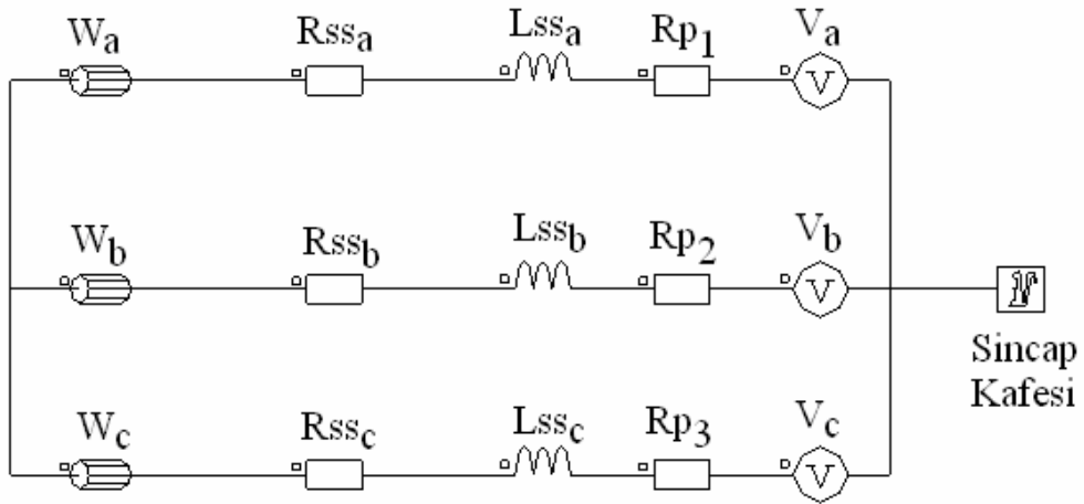
Şekil 5.4. Benzetimde kullanılan Motor4 için Flux programında çizilmiş elektriksel devresi.
