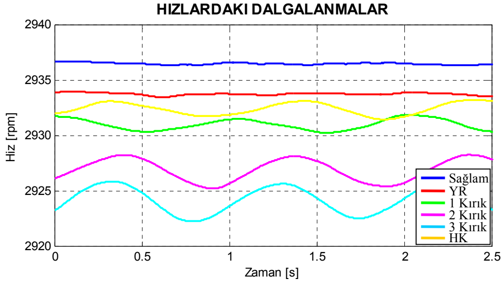
Şekil 8.30. Motor1 için deneysel arıza durumlarına göre çizilmiş hız-zaman grafikleri.
