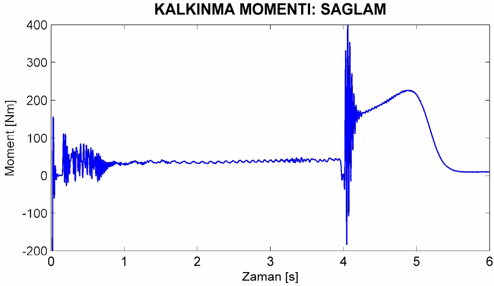
Şekil 8.71. Motor1 sağlam motor durumu için deneysel yol alma momentleri.
