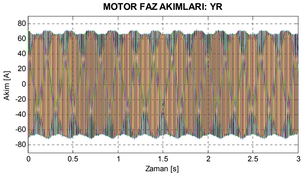
Şekil 7.8. Motor2 bir çubuğu yüksek dirençli rotor için benzetimle elde edilen stator akımları.
