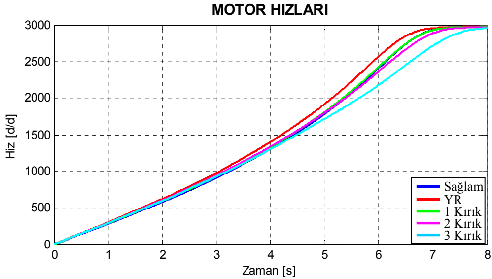
Şekil 7.81. Motor2 için benzetimle elde edilen arıza durumlarına göre çizilmiş yol alma hız grafikleri.
