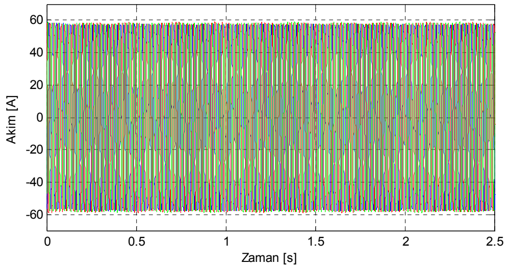
Şekil 8.19. Motor3 kısa devre halkası kırık rotor için deneysel stator akımları.
