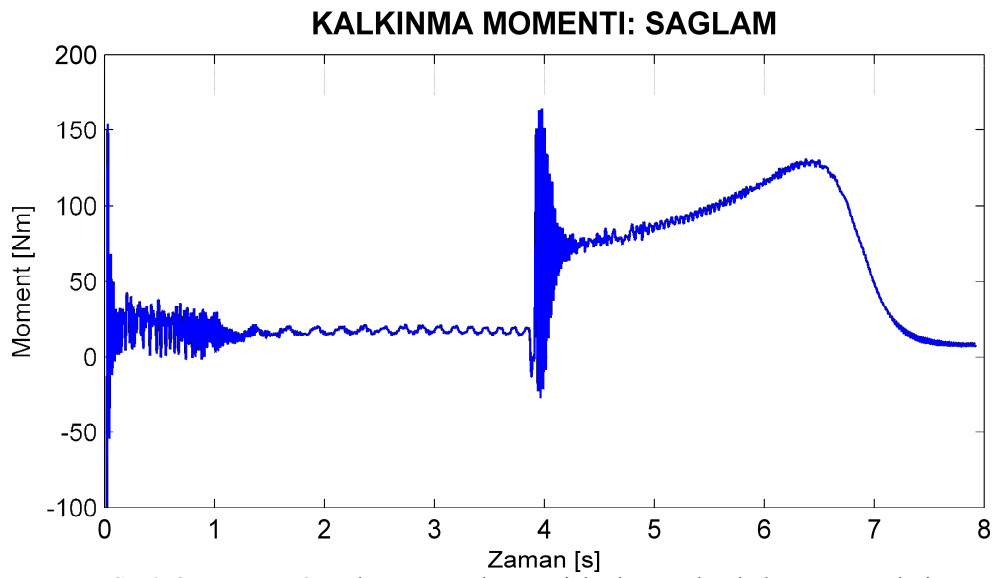
Şekil 8.77. Motor2 sağlam motor durumu için deneysel yol alma momentleri.
