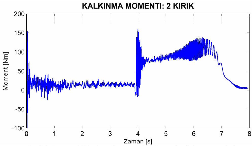
Şekil 8.80. Motor2 iki çubuğu kırık rotor için deneysel yol alma momentleri.
