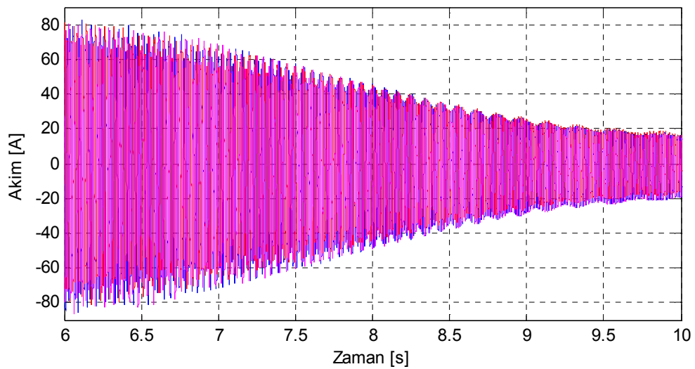
Şekil 8.68. Motor4 iki çubuğu kırık rotor için deneysel yol alma akımları.
