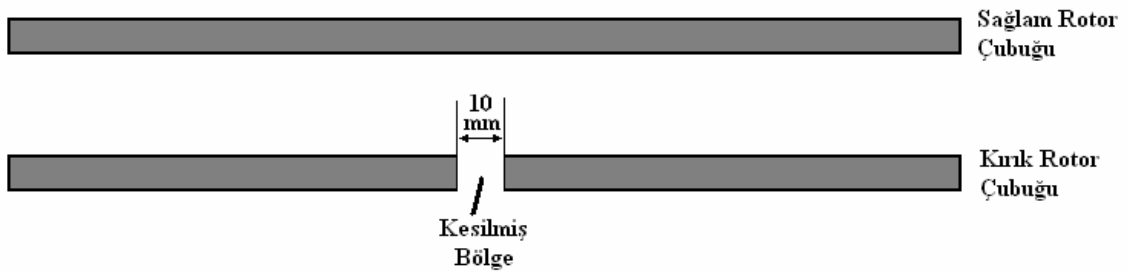
Şekil 6.12. Kırık çubuğun elde edilmesi.
