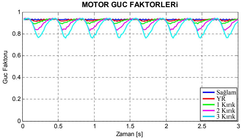
Şekil 7.27. Motor1 için benzetimle elde edilen arıza durumlarına göre çizilmiş güç faktörü grafikleri.
