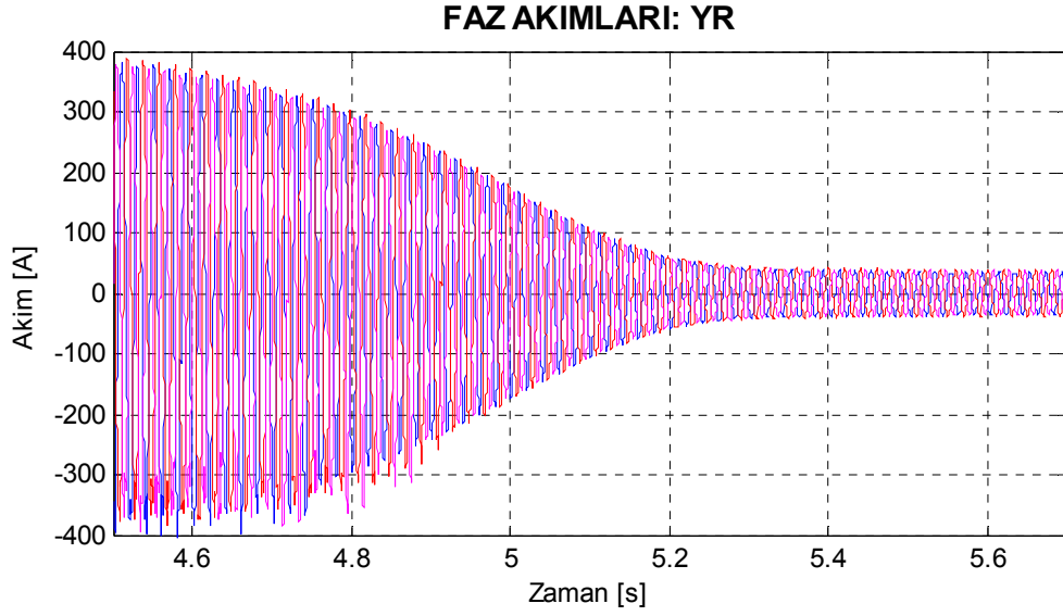
Şekil 8.48. Motor1 bir çubuğu yüksek dirençli rotor için deneysel yol alma akımları.
