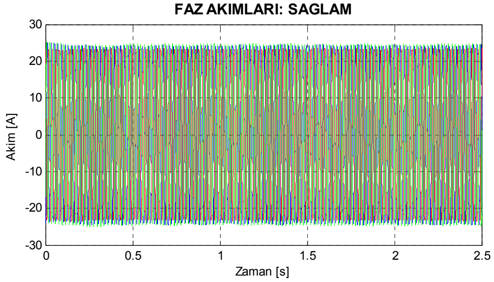
Şekil 8.20. Motor4 sağlam motor durumu için deneysel stator akımları.
