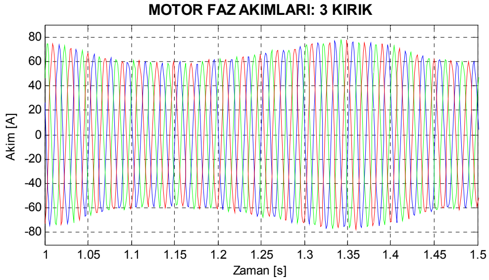
Şekil 8.1. Motor1 için deneysel üç kırık çubuklu rotor arızası için kısa veri aralığıyla çizilmiş motor akımları grafiği.
