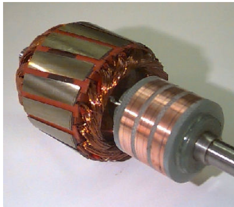
Şekil 3.3. Bilezikli rotor fotoğrafı.
