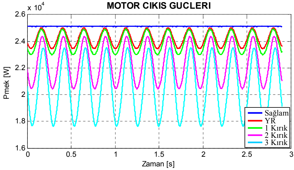
Şekil 7.32. Motor2 için benzetimle elde edilen arıza durumlarına göre çizilmiş mekanik güç grafikleri.
