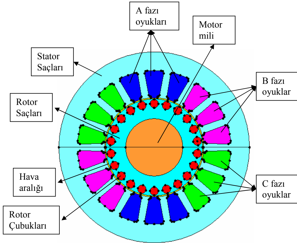
Şekil 5.2. Benzetim için Motor3 ve Motor4'nin Flux programında çizilmiş motor kesitleri.
