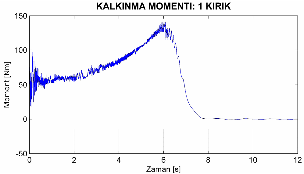
Şekil 7.67. Motor2 bir çubuğu kırık rotor için benzetimle elde edilen yol alma momentleri.
