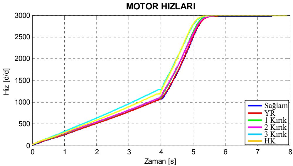
Şekil 8.95. Motor1 için arıza durumlarına göre çizilmiş deneysel yol alma hız grafikleri.
