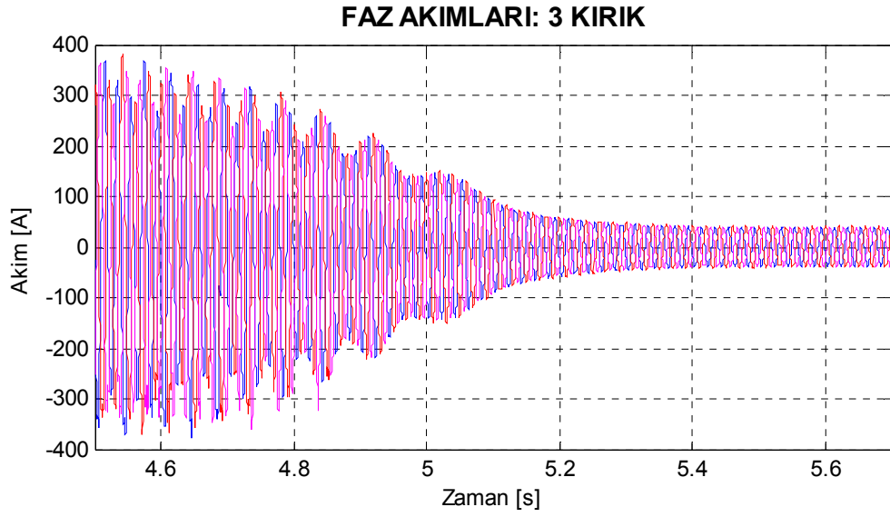
Şekil 8.51. Motor1 üç çubuğu kırık rotor için deneysel yol alma akımları.
