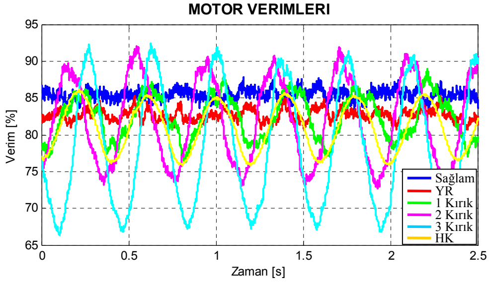
Şekil 8.42. Motor1 için deneysel arıza durumlarına göre çizilmiş verim grafikleri.
