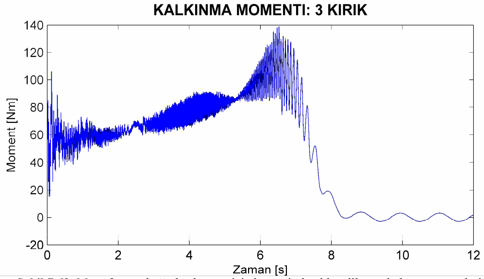
Şekil 7.69. Motor2 üç çubuğu kırık rotor için benzetimle elde edilen yol alma momentleri.
