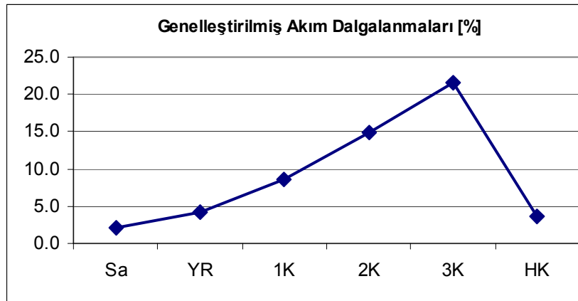
Şekil 9.1. Genelleştirilmiş arızalara göre motor akımı dalgalanması grafiği.
