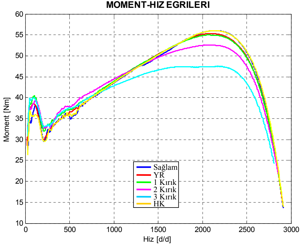
Şekil 8.102. Motor4 için arıza durumlarına göre çizilmiş deneysel hız-moment eğrileri.
