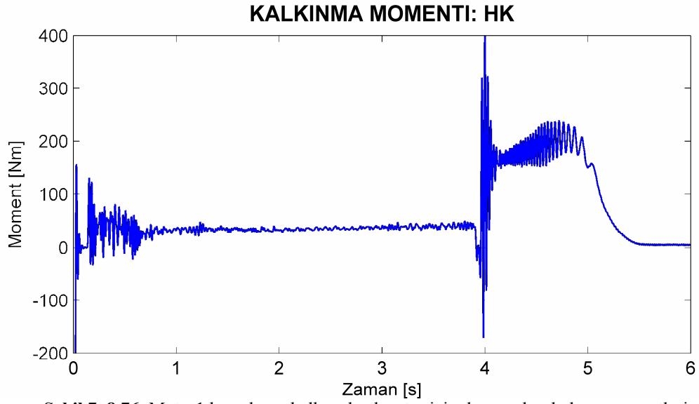
Şekil 7. 8.76. Motor1 kısa devre halkası kırık rotor için deneysel yol alma momentleri.
