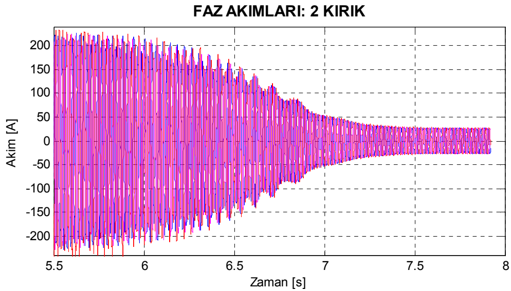
Şekil 8.56. Motor2 iki çubuğu kırık rotor için deneysel yol alma akımları.
