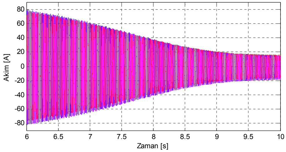
Şekil 8.66. Motor4 bir çubuğu yüksek dirençli rotor için deneysel yol alma akımları.
