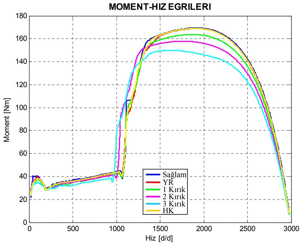
Şekil 8.101. Motor3 için arıza durumlarına göre çizilmiş deneysel hız-moment eğrileri.
