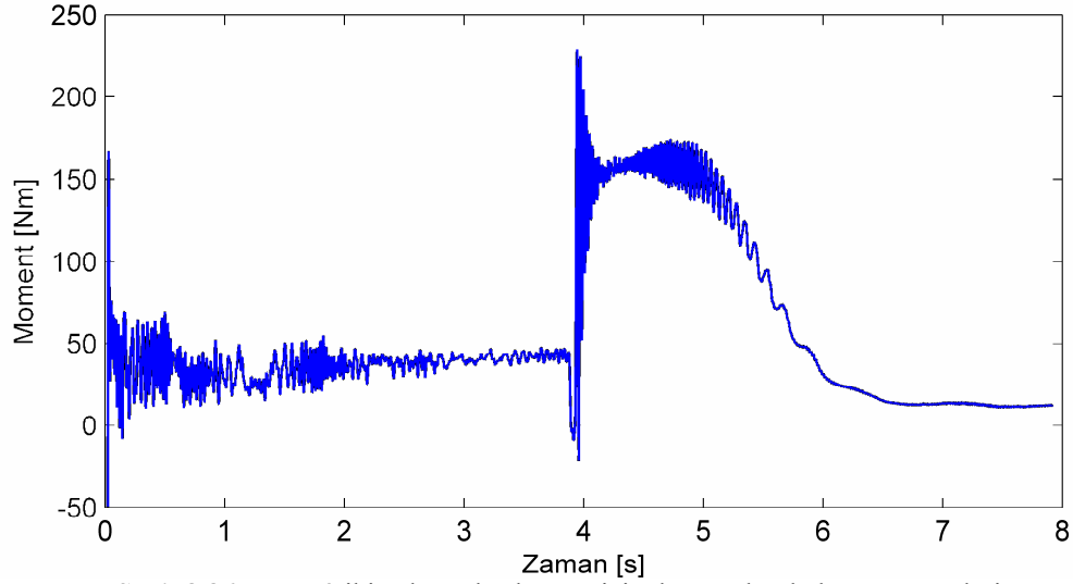
Şekil 8.86. Motor3 iki çubuğu kırık rotor için deneysel yol alma momentleri.
