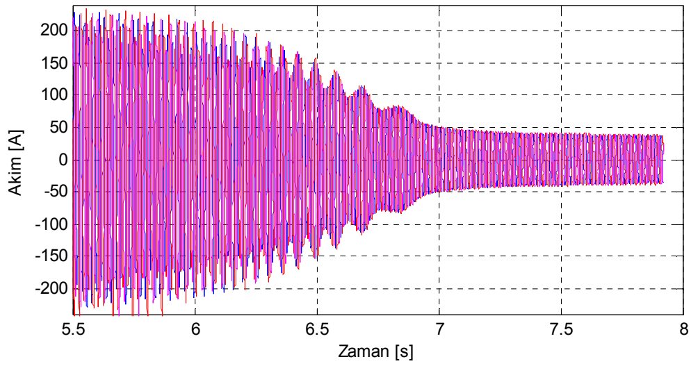
Şekil 8.57. Motor2 üç çubuğu kırık rotor için deneysel yol alma akımları.
