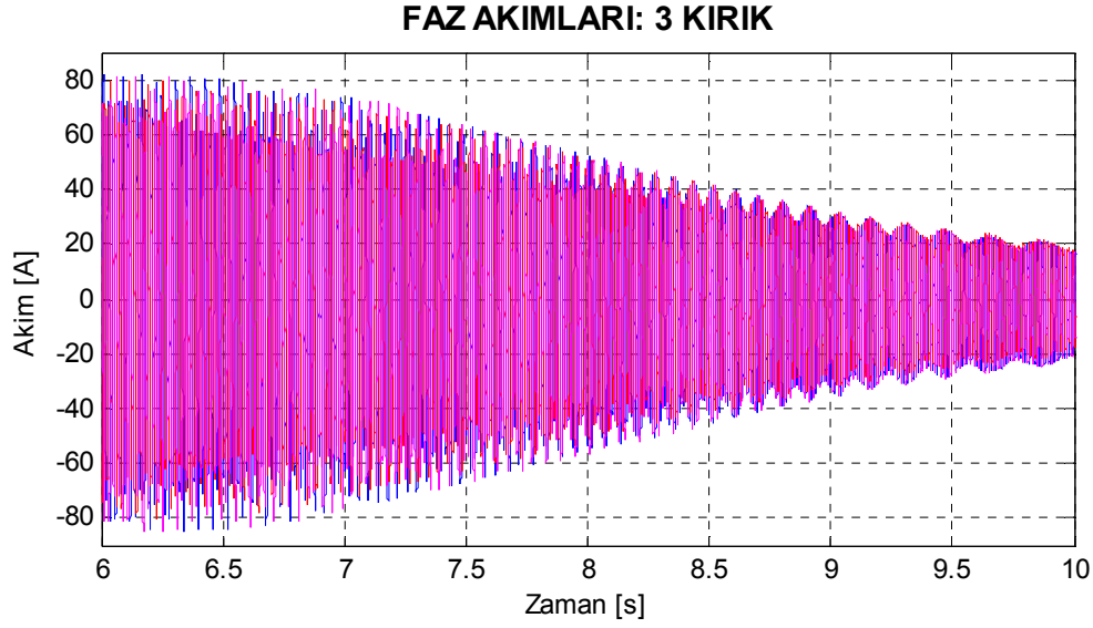
Şekil 8.69. Motor4 üç çubuğu kırık rotor için deneysel yol alma akımları.
