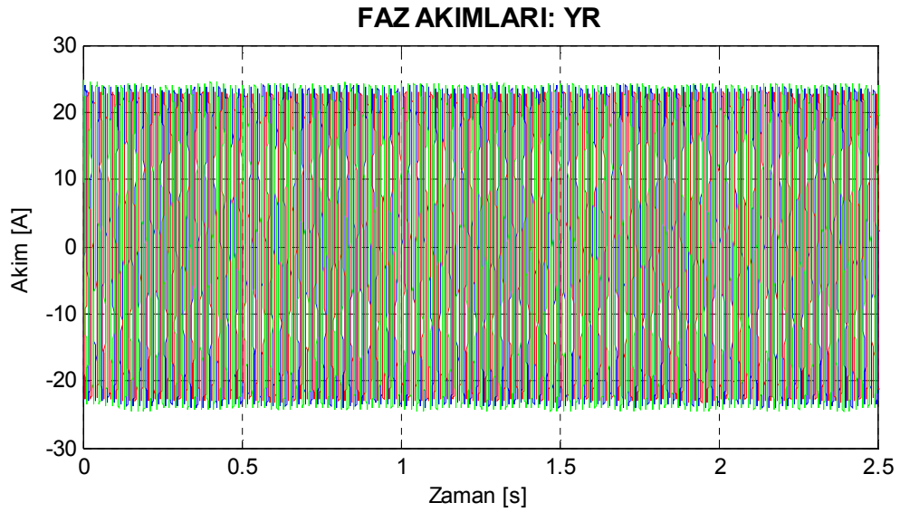
Şekil 8.21. Motor4 bir çubuğu yüksek dirençli rotor için deneysel stator akımları.
