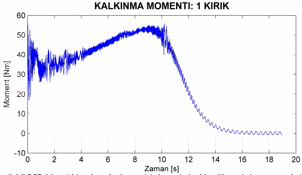
Şekil 7.77. Motor4 bir çubuğu kırık rotor için benzetimle elde edilen yol alma momentleri.
