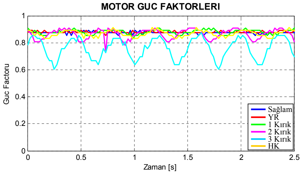
Şekil 8.34. Motor1 için deneysel arıza durumlarına göre çizilmiş güç faktörü grafikleri.
