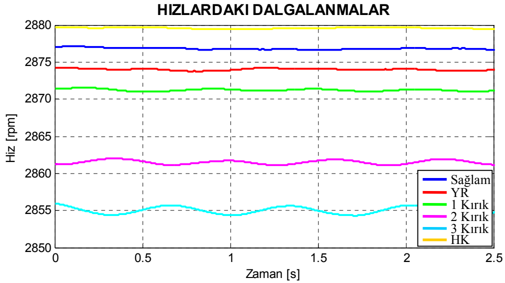
Şekil 8.31. Motor2 için deneysel arıza durumlarına göre çizilmiş hız-zaman grafikleri.
