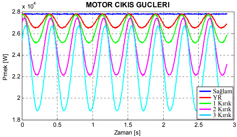
Şekil 7.31. Motor1 için benzetimle elde edilen arıza durumlarına göre çizilmiş mekaniki güç grafikleri.
