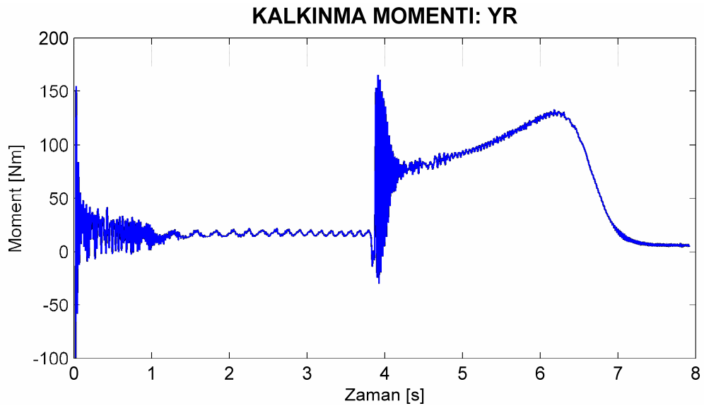
Şekil 8.78. Motor2 bir çubuğu yüksek dirençli rotor için deneysel yol alma momentleri.
