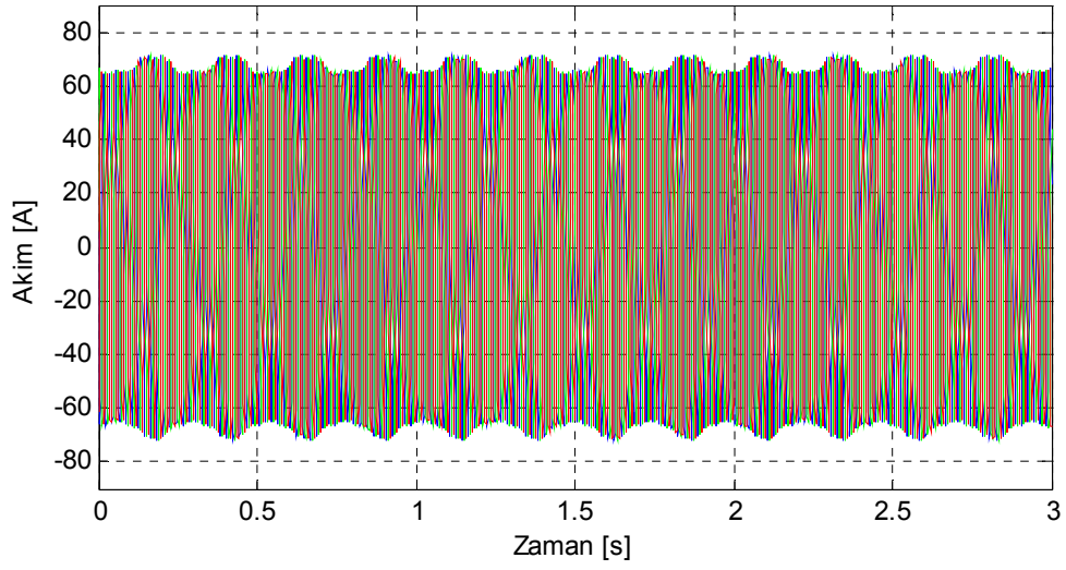
Şekil 7.9. Motor2 bir çubuğu kırık rotor için benzetimle elde edilen stator akımları.
