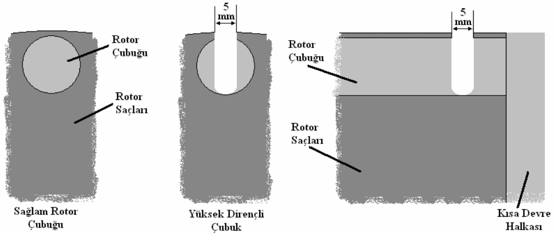
Şekil 6.10. Yüksek dirençli çubuğun elde edilmesi.
