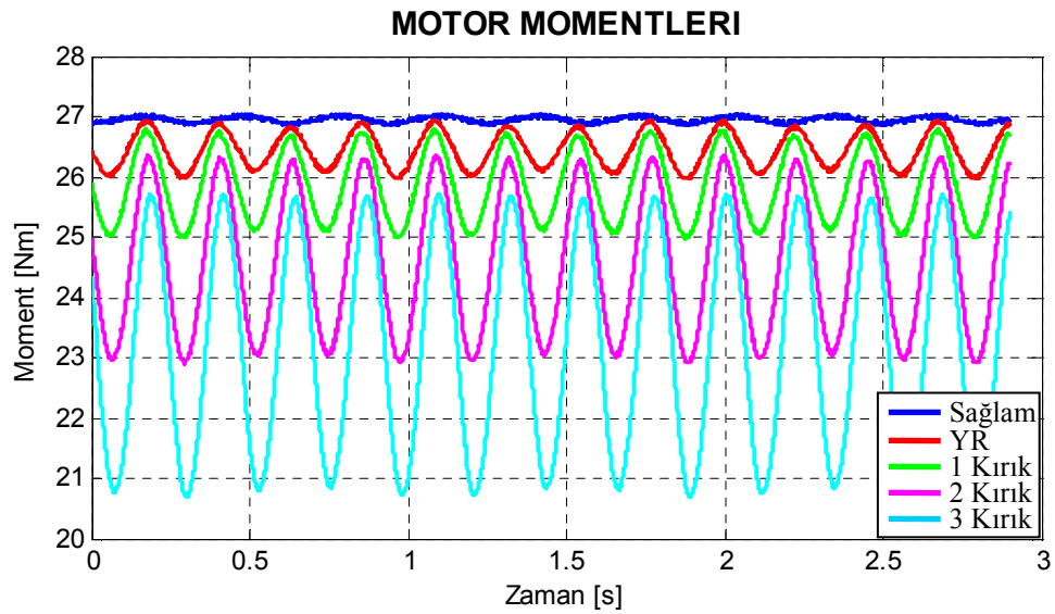
Şekil 7.26. Motor4 için benzetimle elde edilen arıza durumlarına göre çizilmiş moment grafikleri.
