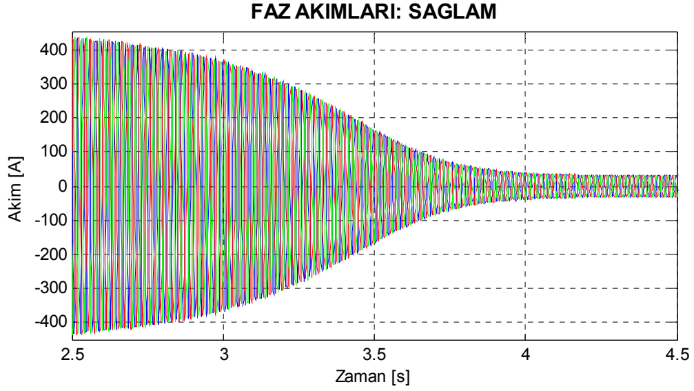
Şekil 7.40. Motor1 sağlam motor durumu için benzetimle elde edilen yol alma akımları.
