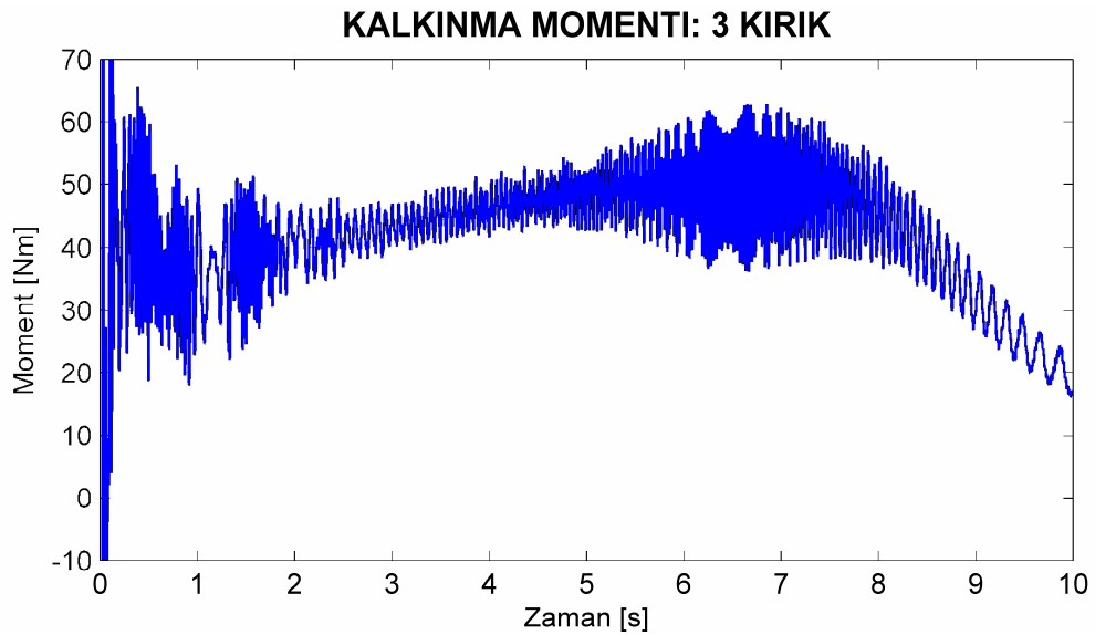
Şekil 8.93. Motor4 üç çubuğu kırık rotor için deneysel yol alma momentleri.
