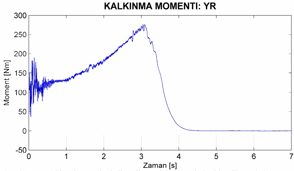
Şekil 7.61. Motor1 bir çubuğu yüksek dirençli rotor için benzetimle elde edilen yol alma momentleri.
