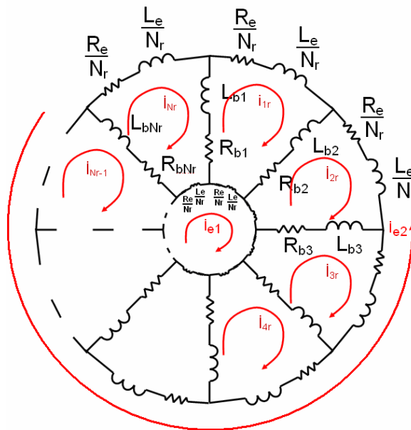
Şekil 5.1. Rotor çevre akımları ile rotor kafesi.
