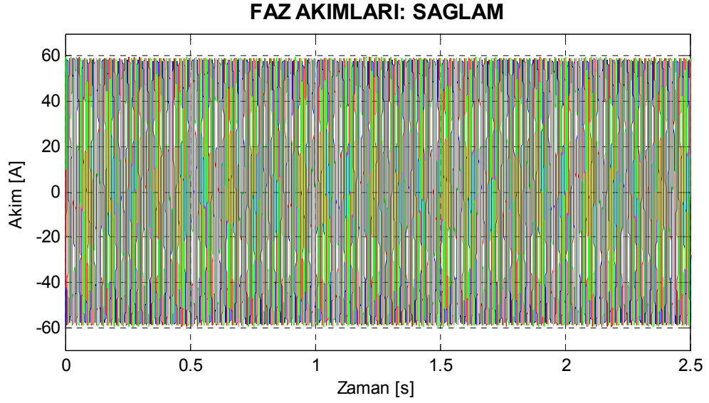
Şekil 8.14. Motor3 sağlam motor durumu için deneysel stator akımları.
