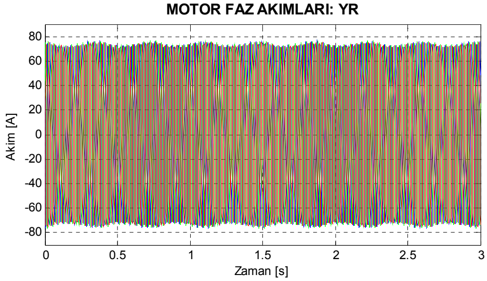
Şekil 7.3. Motor1 bir çubuğu yüksek dirençli rotor için benzetimle elde edilen stator akımları.
