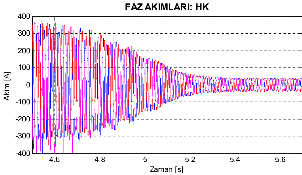
Şekil 8.52. Motor1 kısa devre halkası kırık rotor için deneysel yol alma akımları.
