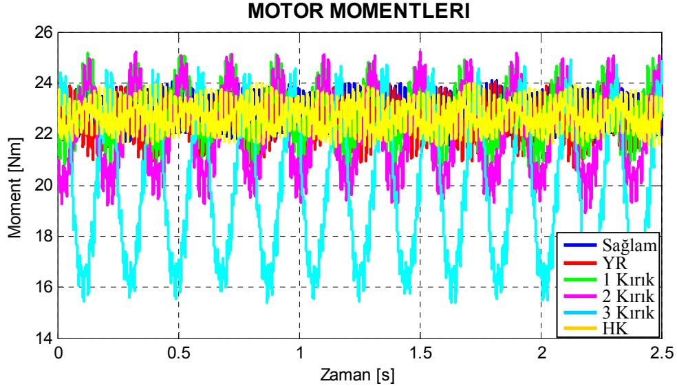
Şekil 8.29. Motor4 için deneysel arıza durumlarına göre çizilmiş moment grafikleri.
