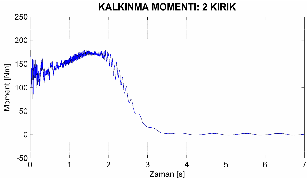
Şekil 7.73. Motor3 iki çubuğu kırık rotor için benzetimle elde edilen yol alma momentleri.
