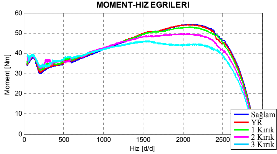
Şekil 7.87. Motor4 için benzetimle elde edilen arıza durumlarına göre çizilmiş hız-moment eğrileri.
