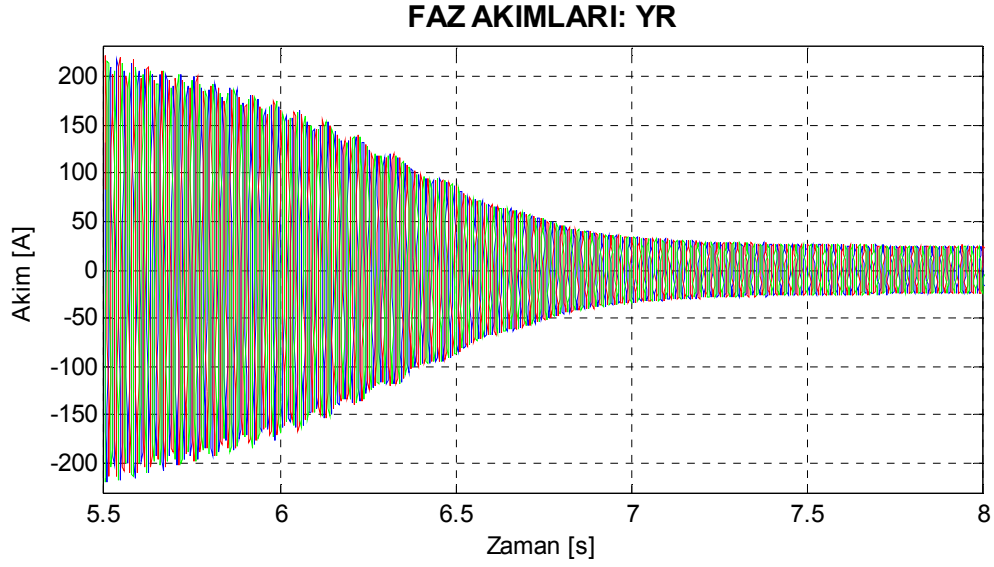
Şekil 7.46. Motor2 bir çubuğu yüksek dirençli rotor için benzetimle elde edilen yol alma akımları.
