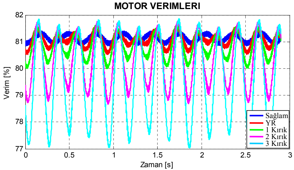
Şekil 7.38. Motor4 için benzetimle elde edilen arıza durumlarına göre çizilmiş verim grafikleri.
