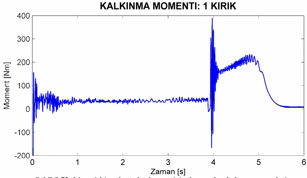
Şekil 8.73. Motor1 bir çubuğu kırık rotor için deneysel yol alma momentleri.
