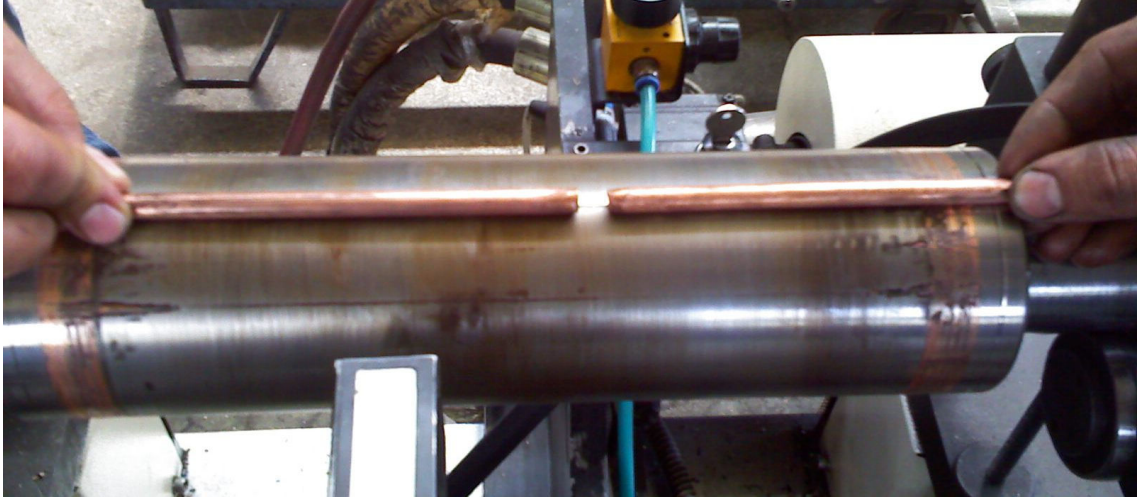
Şekil 6.13. Kırık çubuk arızasının rotor üzerinde gösterilmesi.
