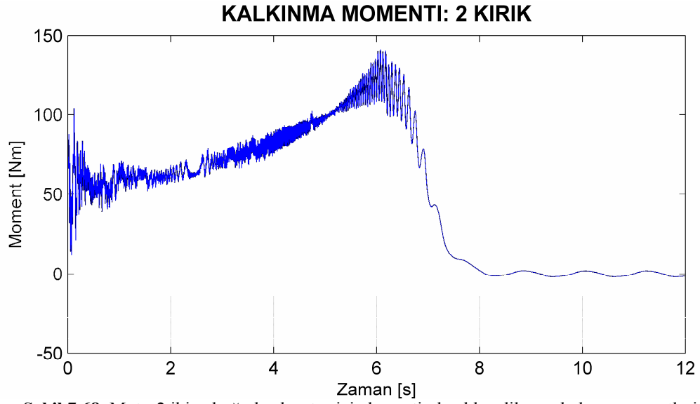
Şekil 7.68. Motor2 iki çubuğu kırık rotor için benzetimle elde edilen yol alma momentleri.
