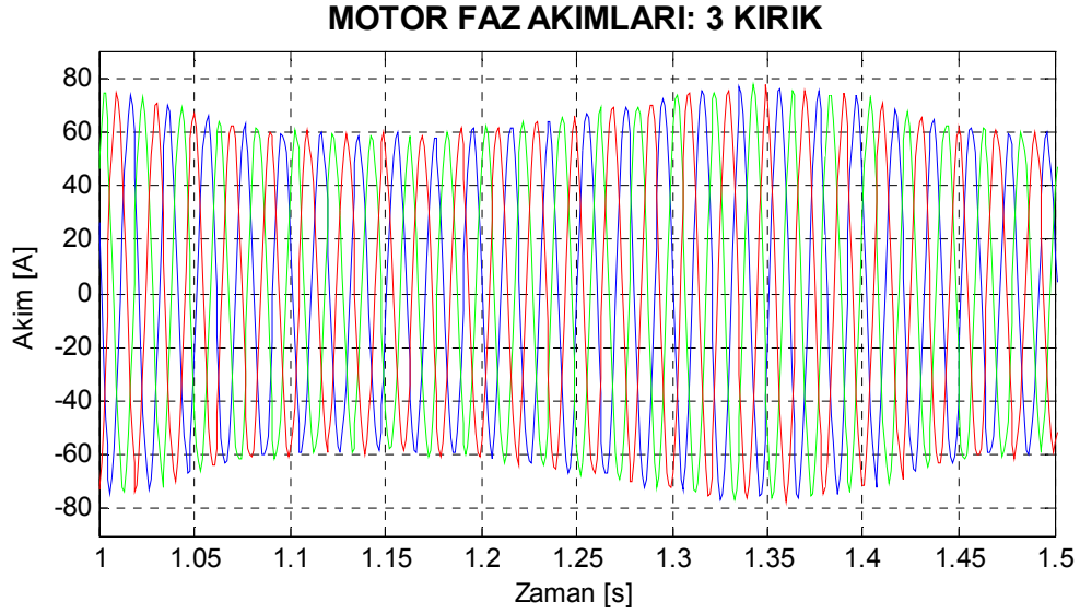
Şekil 7.1. Motor1 için benzetimle elde edilen üç kırık çubuklu rotor arızası için kısa veri aralığıyla çizilmiş motor akımı grafiği.
