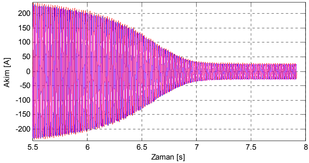
Şekil 8.58. Motor2 kısa devre halkası kırık rotor için deneysel yol alma akımları.
