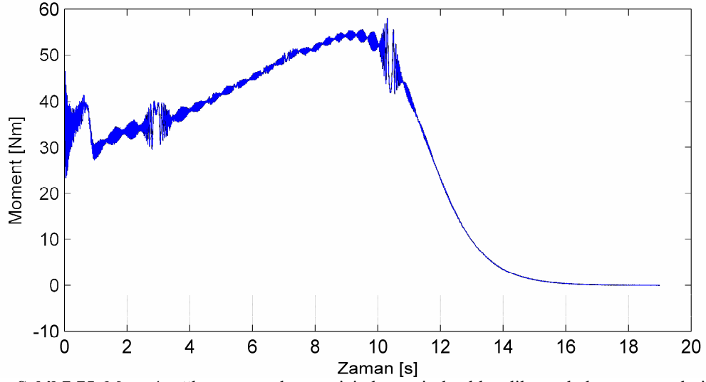
Şekil 7.75. Motor4 sağlam motor durumu için benzetimle elde edilen yol alma momentleri.
