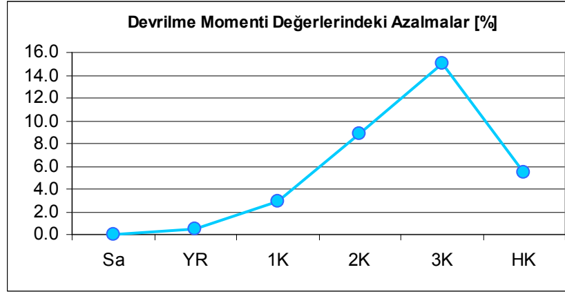
Şekil 9.15. Hız-moment eğrisindeki devrilme momentlerinin arızalara göre azalma oranları.
