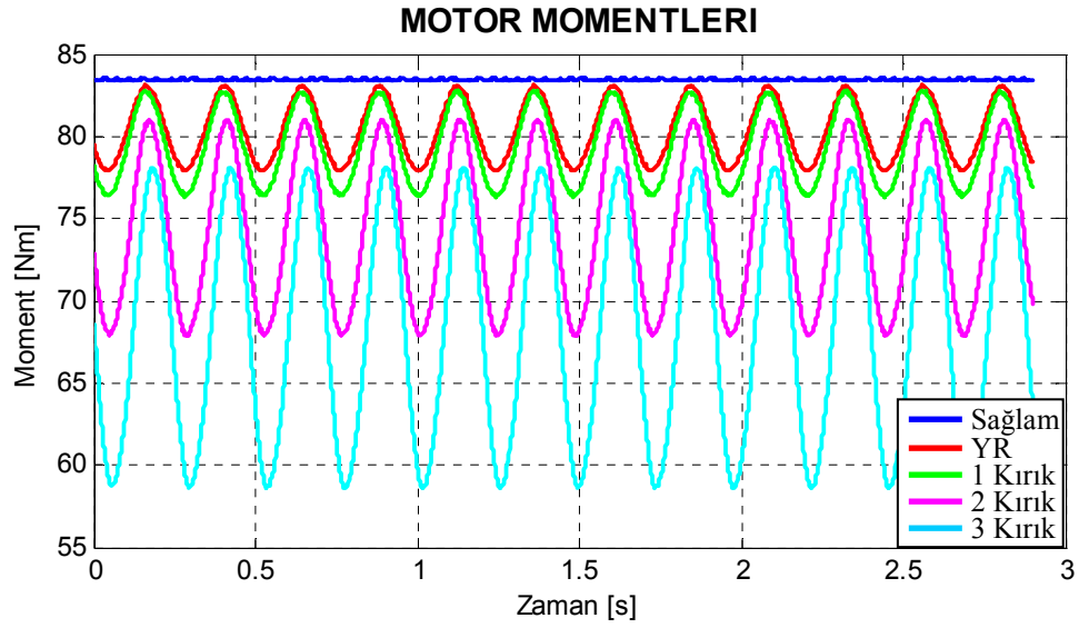
Şekil 7.24. Motor2 için benzetimle elde edilen arıza durumlarına göre çizilmiş moment grafikleri.
