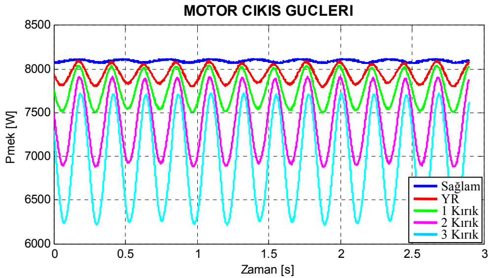
Şekil 7.34. Motor4 için benzetimle elde edilen arıza durumlarına göre çizilmiş mekanik güç grafikleri.
