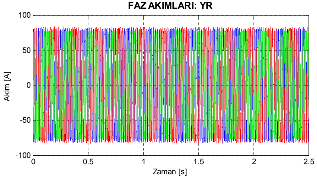
Şekil 8.3. Motor1 bir çubuğu yüksek dirençli rotor için deneysel stator akımları.
