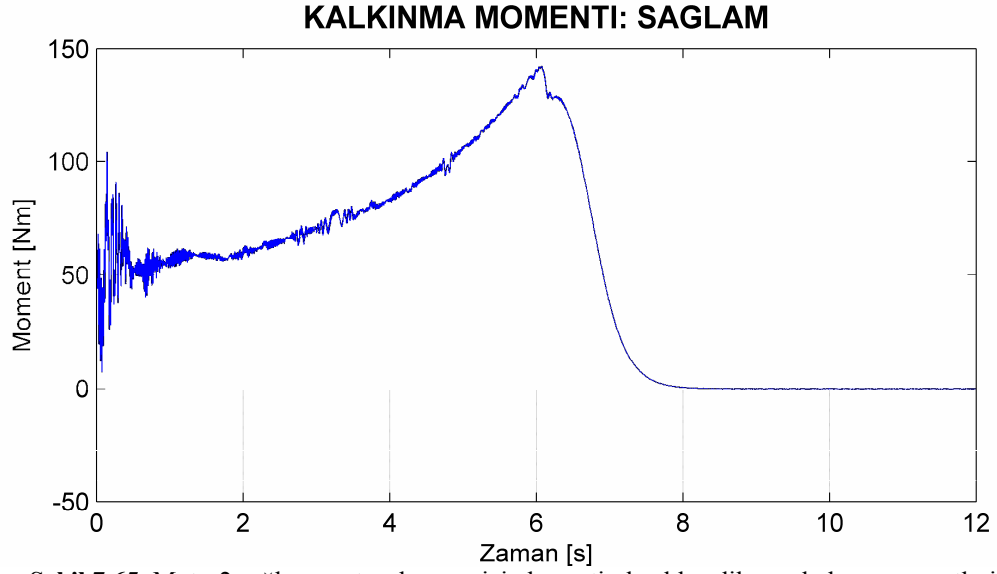
Şekil 7.65. Motor2 sağlam motor durumu için benzetimle elde edilen yol alma momentleri.
