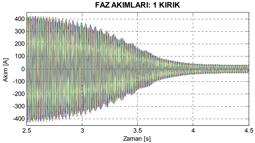
Şekil 7.42. Motor1 bir çubuğu kırık rotor için benzetimle elde edilen yol alma akımları.
