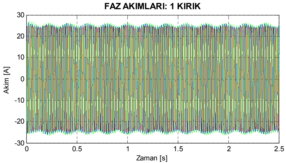
Şekil 8.22. Motor4 bir çubuğu kırık rotor için deneysel stator akımları.
