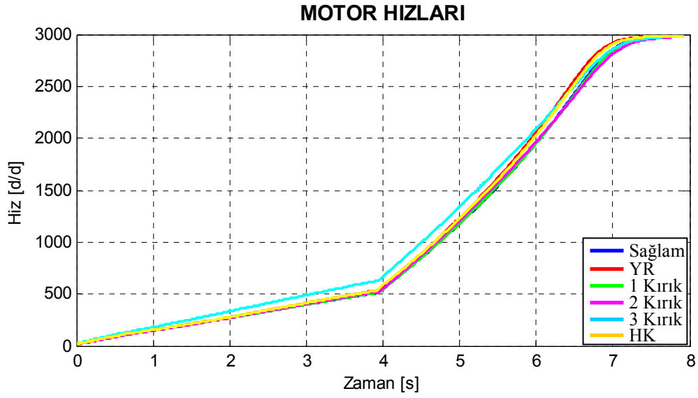
Şekil 8.96. Motor2 için arıza durumlarına göre çizilmiş deneysel yol alma hız grafikleri.
