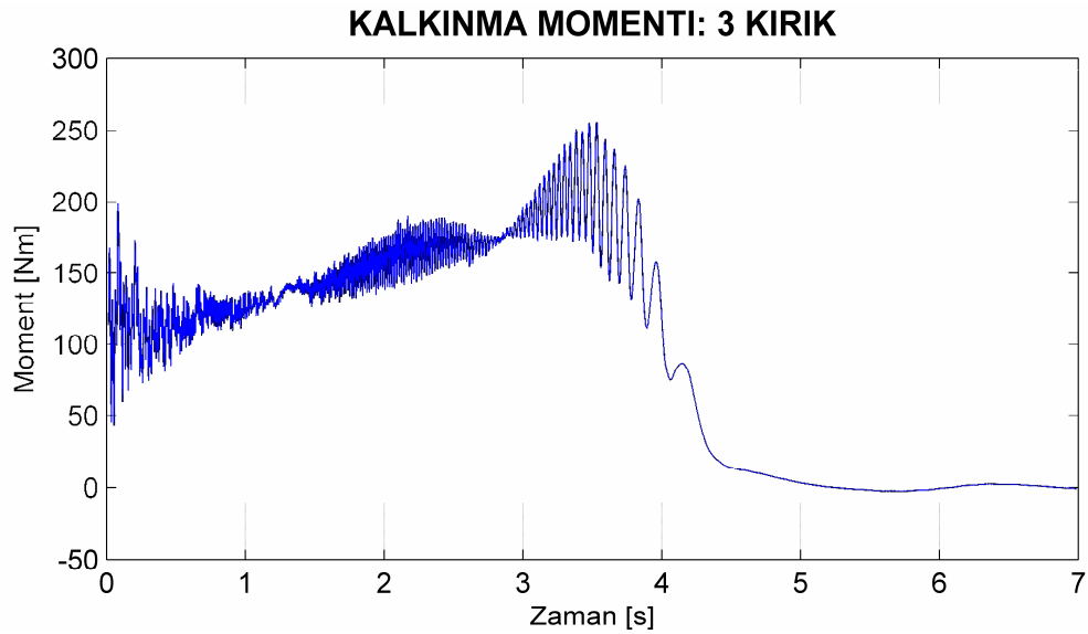
Şekil 7.64. Motor1 üç çubuğu kırık rotor için benzetimle elde edilen yol alma momentleri.
