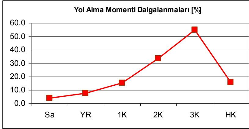
Şekil 9.14. Yol alma sürecinde arızalara göre motor momentlerindeki genelleştirilmiş dalgalanma oranları.
