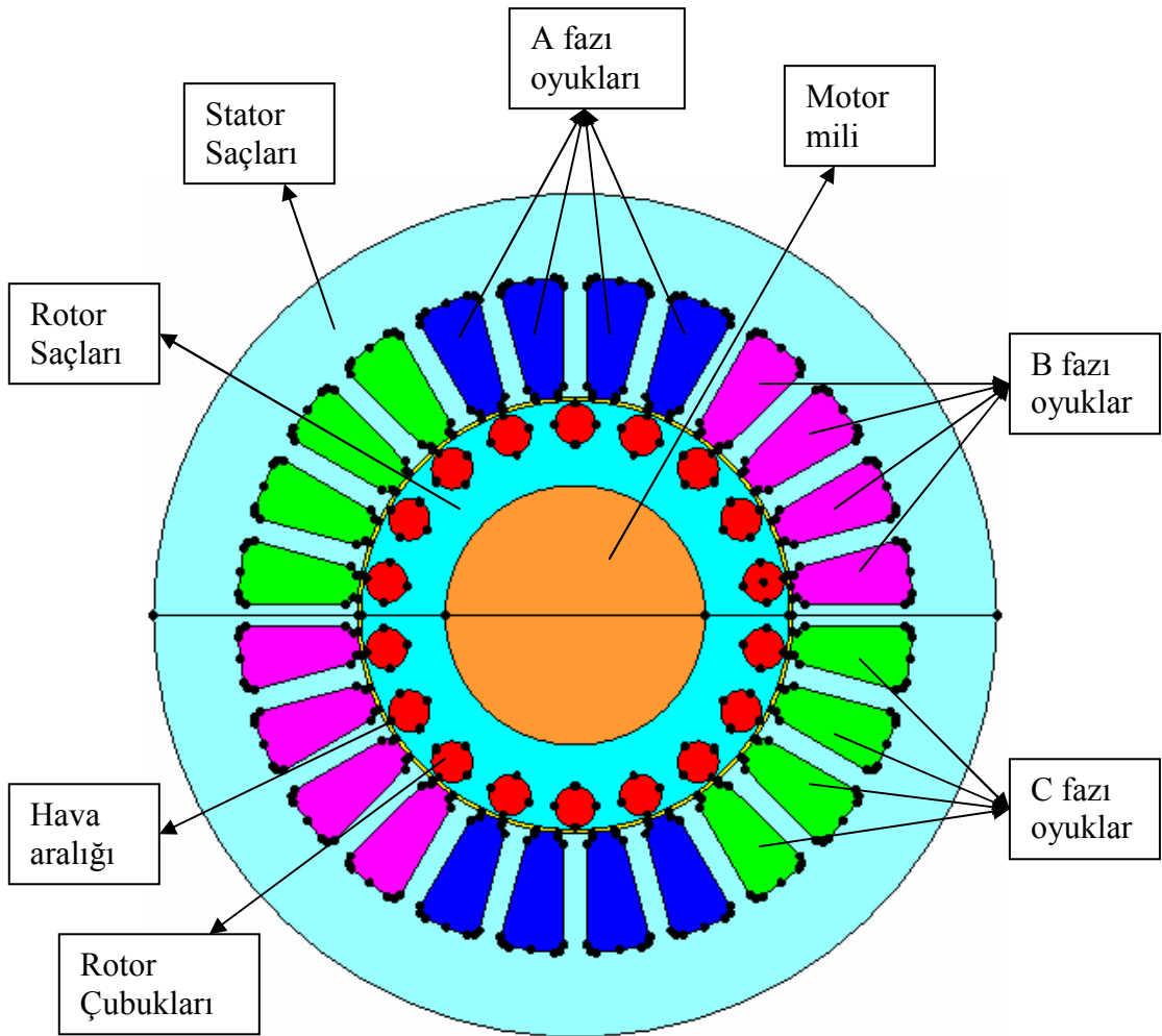
Şekil 5.1. Benzetim için Motor1 ve Motor2'nin Flux programında çizilmiş motor kesitleri.
