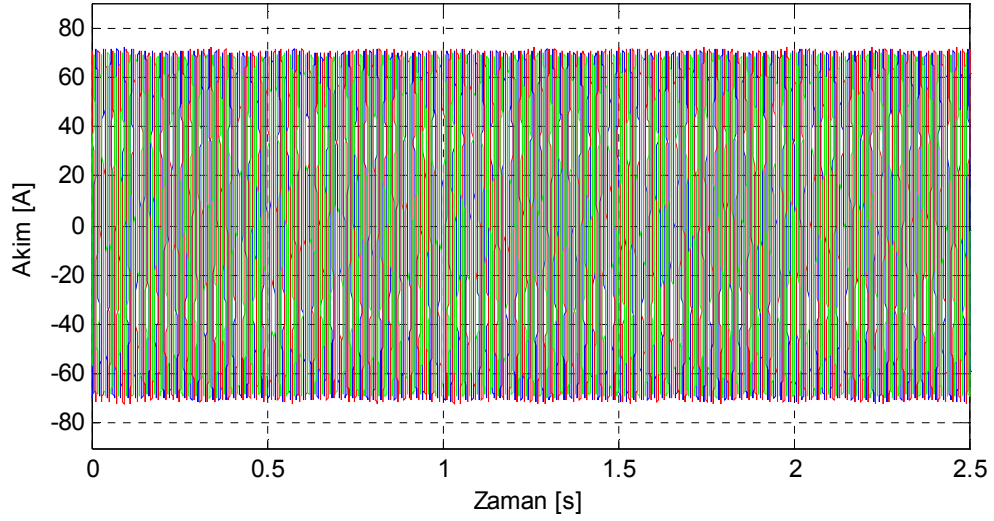
Şekil 8.9. Motor2 bir çubuğu yüksek dirençli rotor için deneysel stator akımları.
