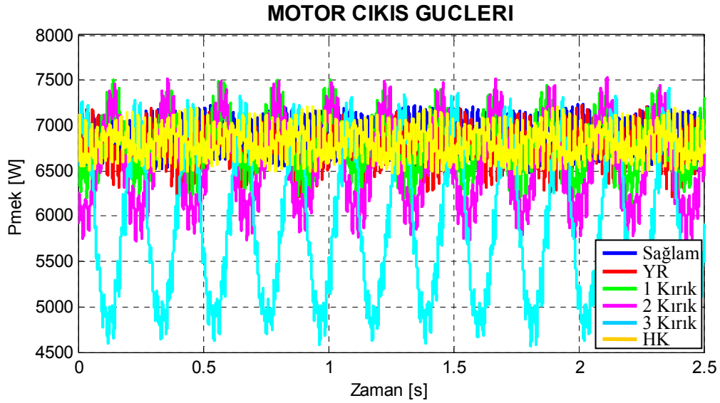
Şekil 8.41. Motor4 için deneysel arıza durumlarına göre çizilmiş mekanik güç grafikleri.
