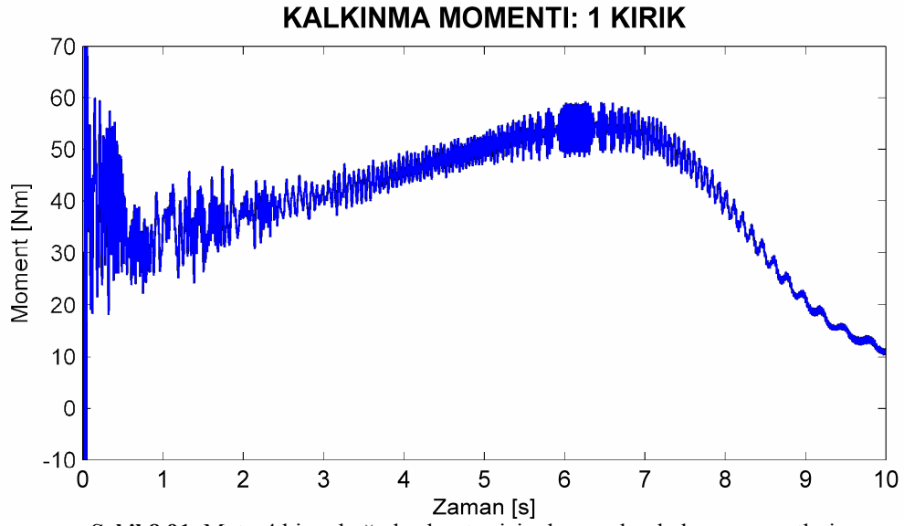
Şekil 8.91. Motor4 bir çubuğu kırık rotor için deneysel yol alma momentleri.
