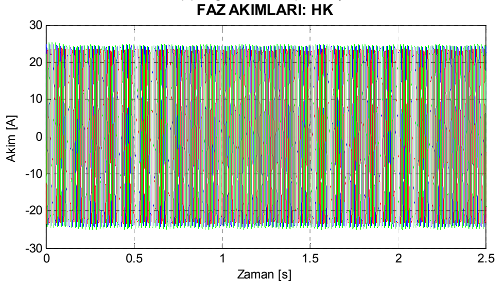
Şekil 8.25. Motor4 kısa devre halkası kırık rotor için deneysel stator akımları.
