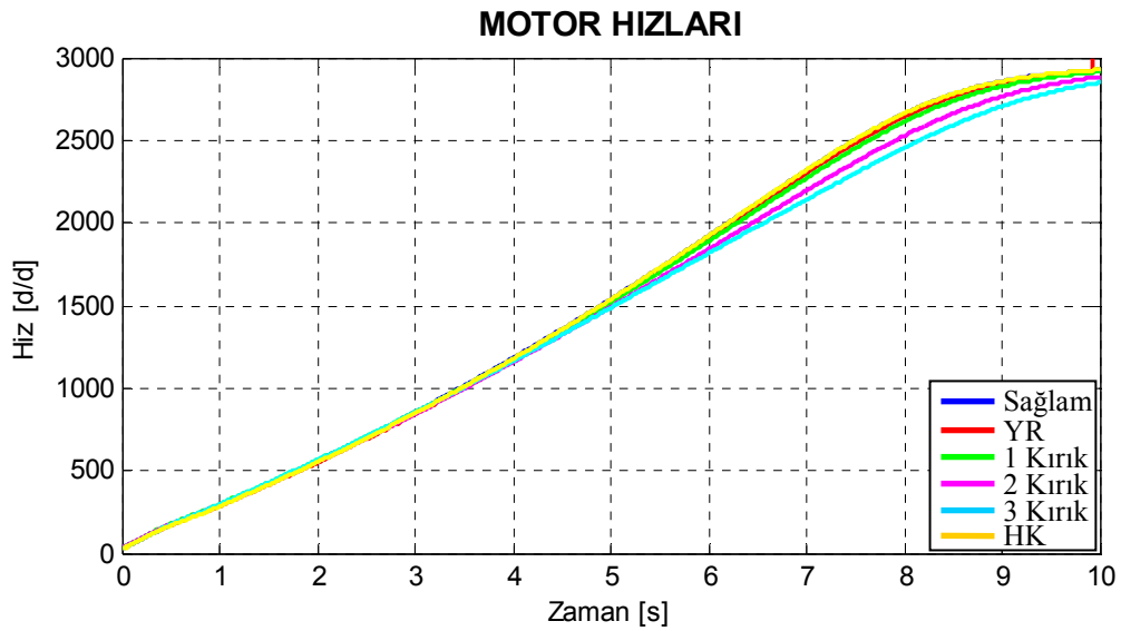
Şekil 8.98. Motor4 için arıza durumlarına göre çizilmiş deneysel yol alma hız grafikleri.
