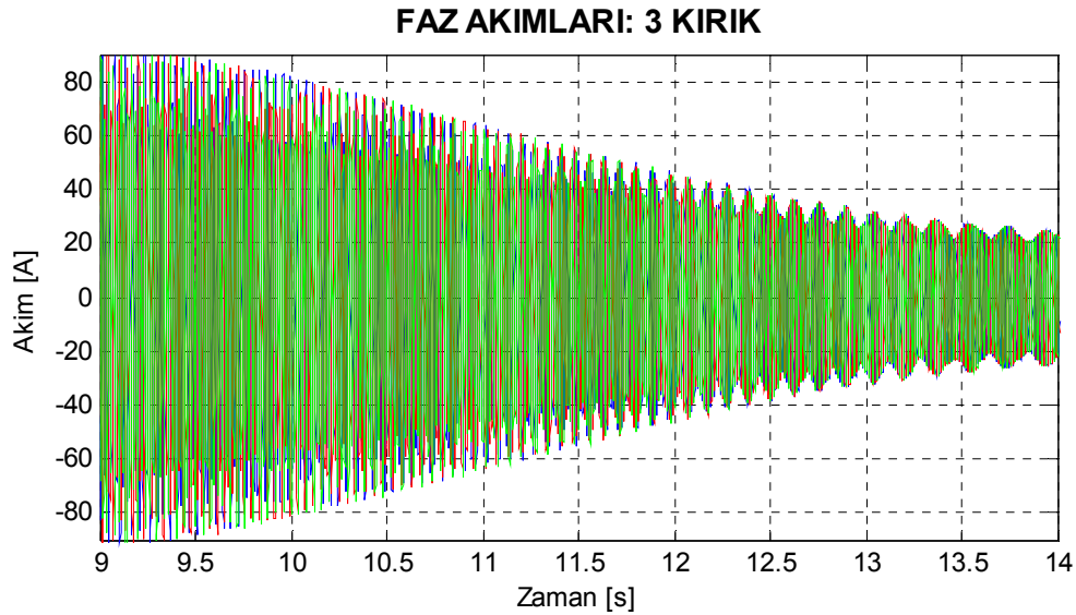
Şekil 7.59. Motor4 üç çubuğu kırık rotor için benzetimle elde edilen yol alma akımları.
