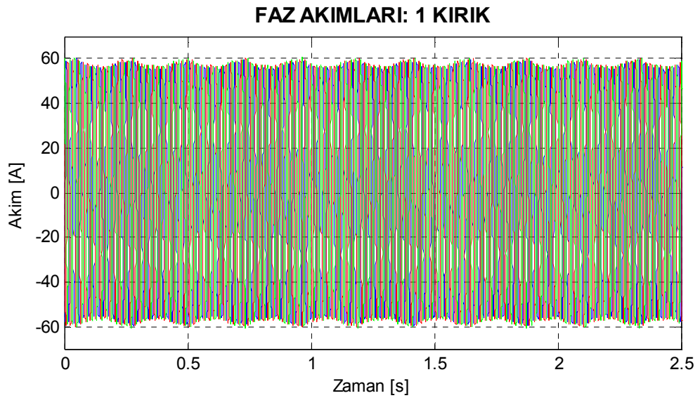
Şekil 8.16. Motor3 bir çubuğu kırık rotor için deneysel stator akımları.
