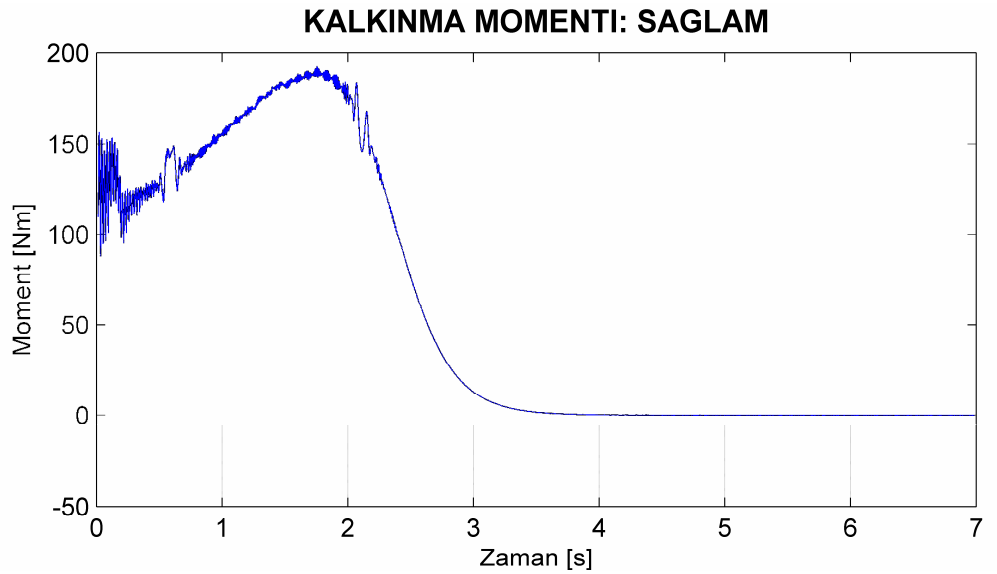
Şekil 7.70. Motor3 sağlam motor durumu için benzetimle elde edilen yol alma momentleri.
