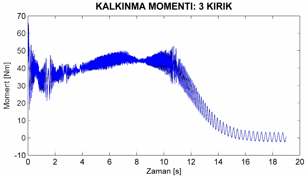
Şekil 7.79. Motor4 üç çubuğu kırık rotor için benzetimle elde edilen yol alma momentleri.
