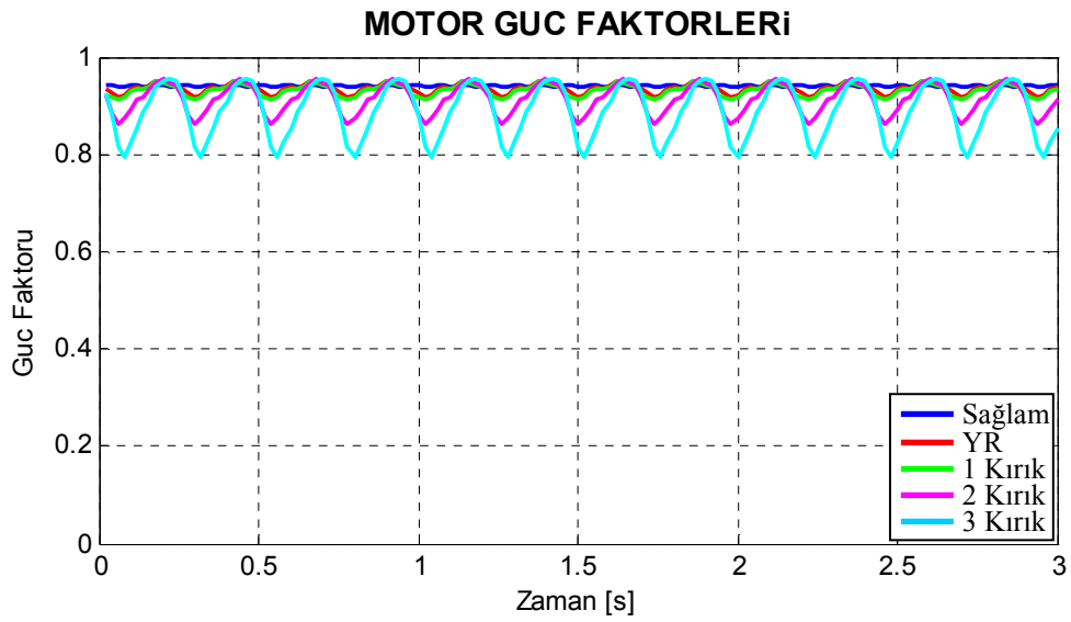
Şekil 7.28. Motor2 için benzetimle elde edilen arıza durumlarına göre çizilmiş güç faktörü grafikleri.
