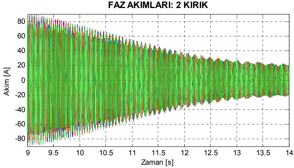
Şekil 7.58. Motor4 iki çubuğu kırık rotor için benzetimle elde edilen yol alma akımları.
