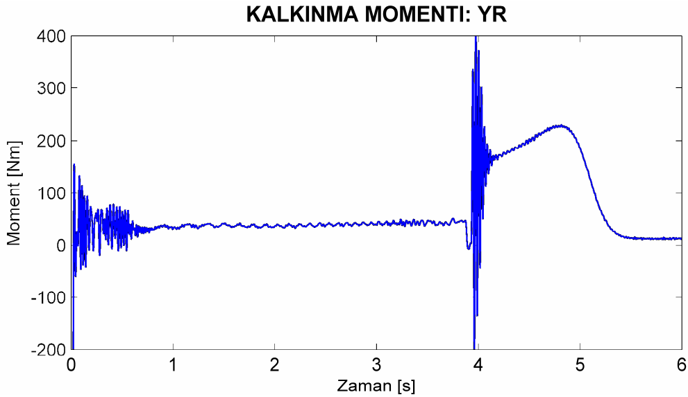
Şekil 8.72. Motor1 bir çubuğu yüksek dirençli rotor için deneysel yol alma momentleri.
