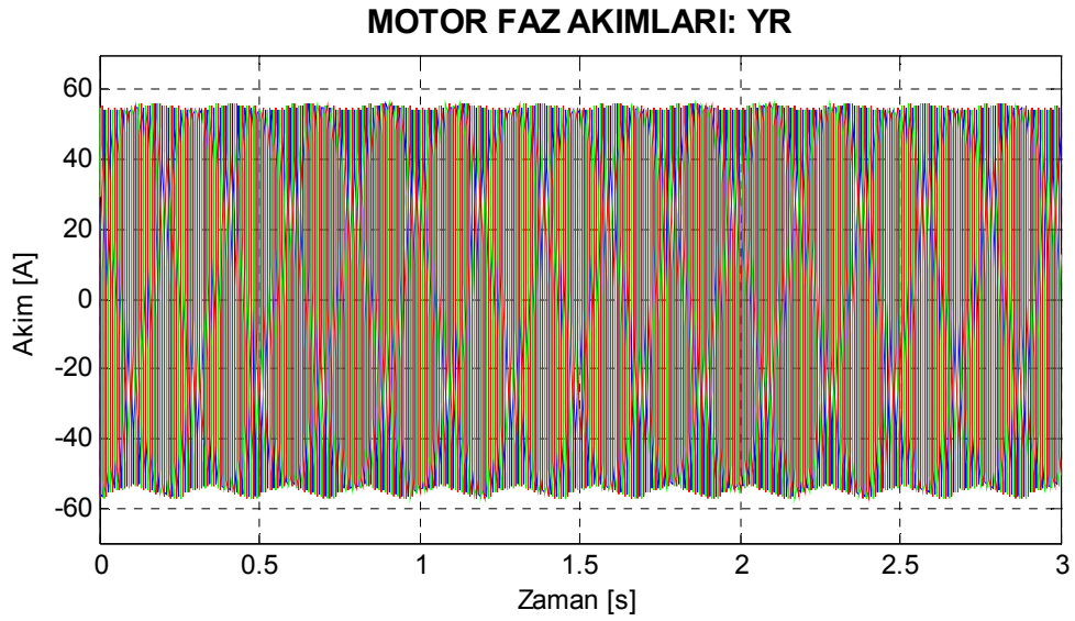
Şekil 7.13. Motor3 bir çubuğu yüksek dirençli rotor için benzetimle elde edilen stator akımları.
