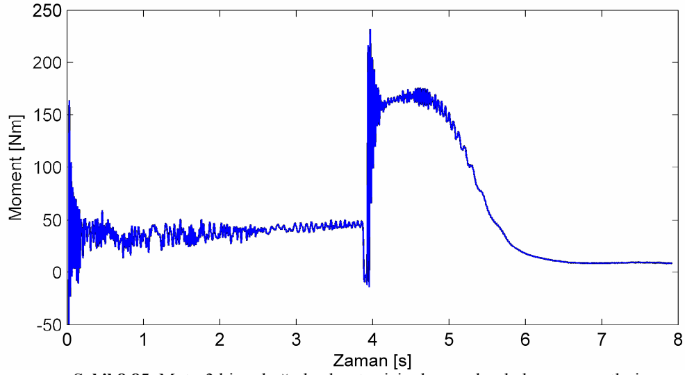
Şekil 8.85. Motor3 bir çubuğu kırık rotor için deneysel yol alma momentleri.
