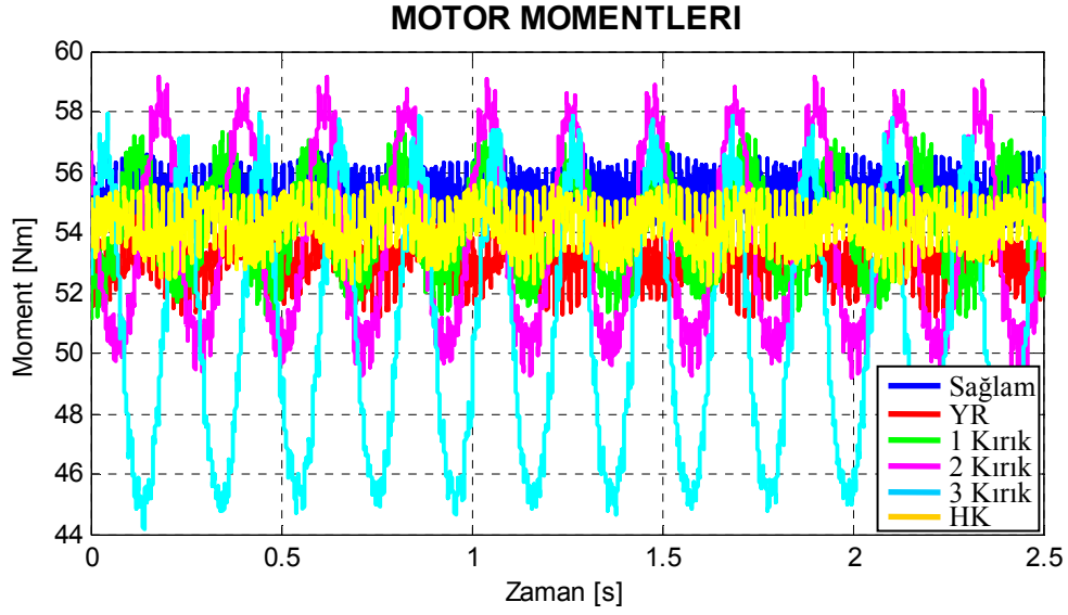
Şekil 8.28. Motor3 için deneysel arıza durumlarına göre çizilmiş moment grafikleri.
