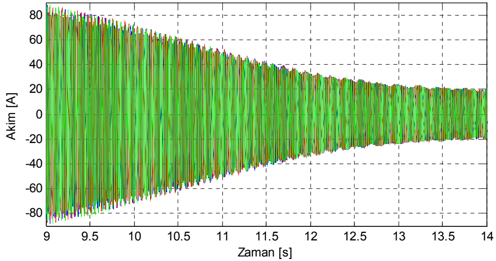
Şekil 7.57. Motor4 bir çubuğu kırık rotor için benzetimle elde edilen yol alma akımları.
