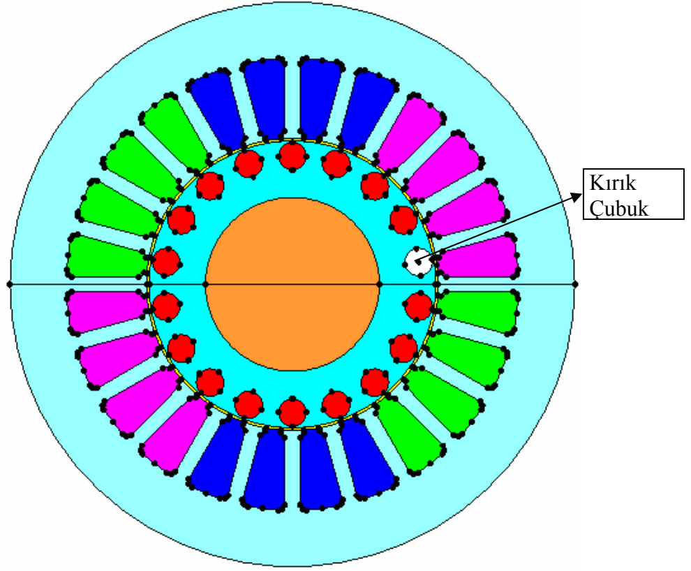
Şekil 5.5. Motor1’de bir kırık çubuk arızası benzetimi için seçilen rotor çubuğunun kesitte gösterimi.
