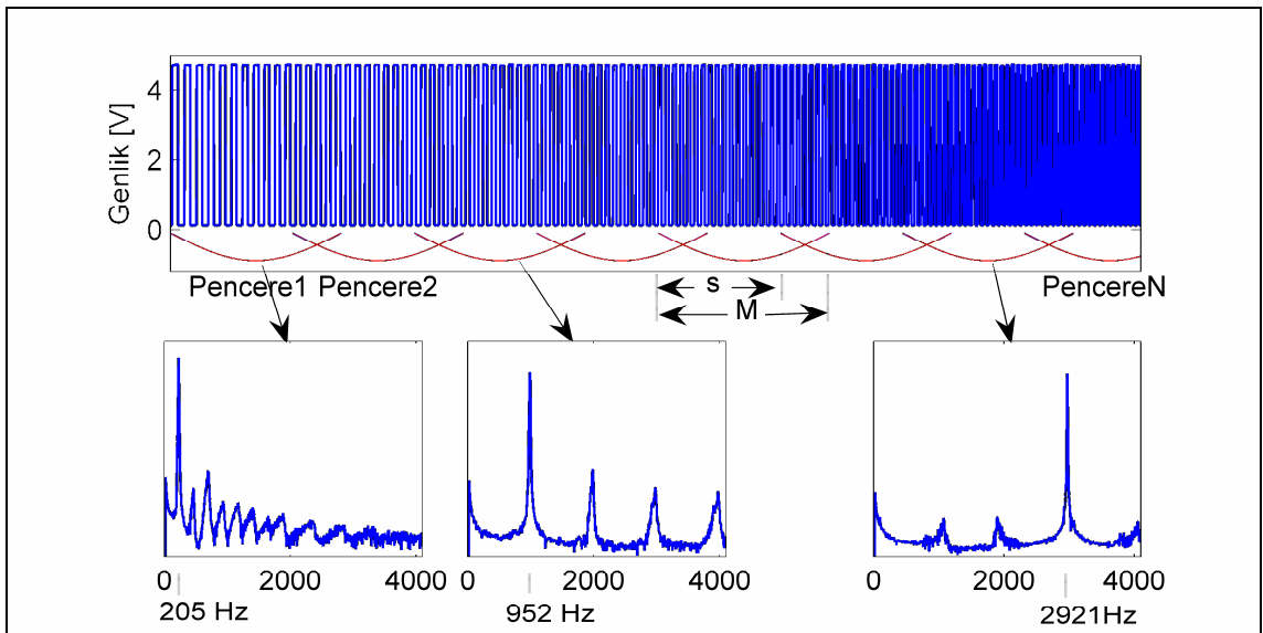
Şekil 4.2. Hız sensöründen örneklenen kare dalga hız sinyali ve HFD ile bulunan bazı pencerelerin frekans değişimleri.
