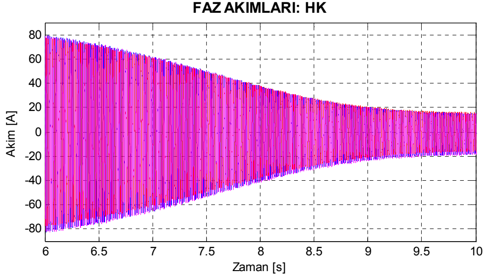
Şekil 8.70. Motor4 kısa devre halkası kırık rotor için deneysel yol alma akımları.
