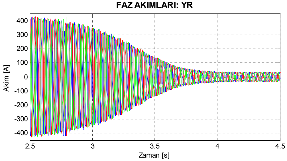
Şekil 7.41. Motor1 bir çubuğu yüksek dirençli rotor için benzetimle elde edilen yol alma akımları.
