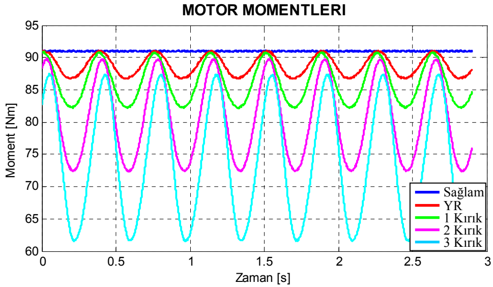
Şekil 7.23. Motor1 için benzetimle elde edilen arıza durumlarına göre çizilmiş moment grafikleri.
