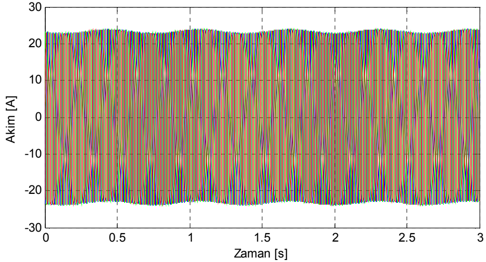
Şekil 7.17. Motor4 sağlam motor durumu için benzetimle elde edilen stator akımları.
