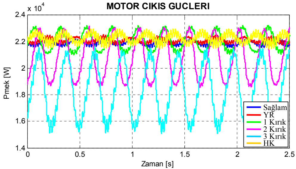
Şekil 8.39. Motor2 için deneysel arıza durumlarına göre çizilmiş mekaniki güç grafikleri.
