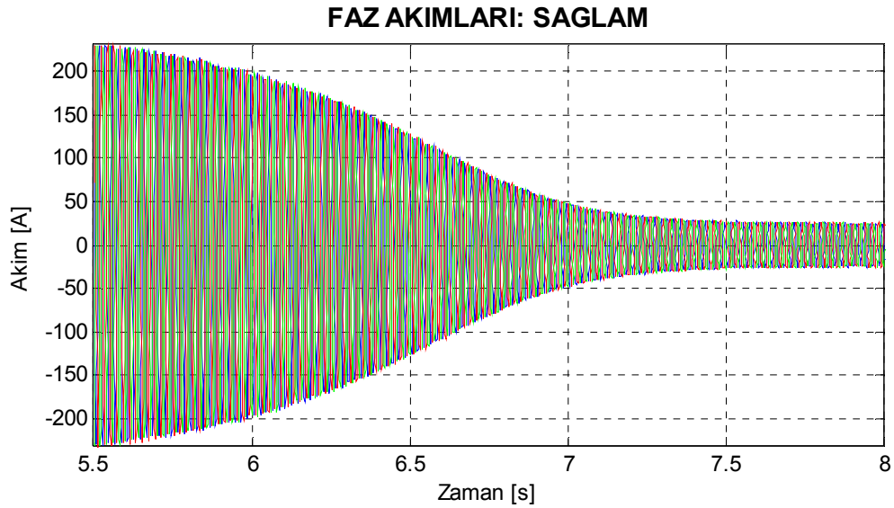
Şekil 7.45. Motor2 sağlam motor durumu için benzetimle elde edilen yol alma akımları.
