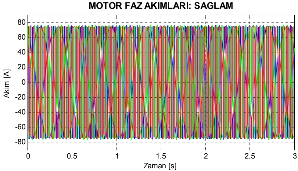
Şekil 7.2. Motor1 sağlam motor durumu için benzetimle elde edilen stator akımları.
