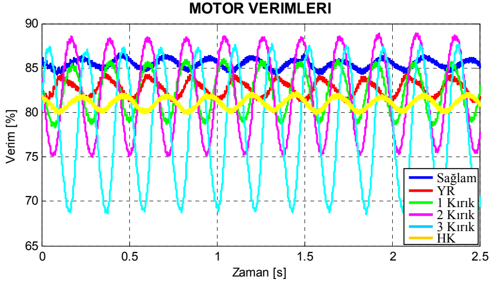
Şekil 8.45. Motor4 için deneysel arıza durumlarına göre çizilmiş verim grafikleri.
