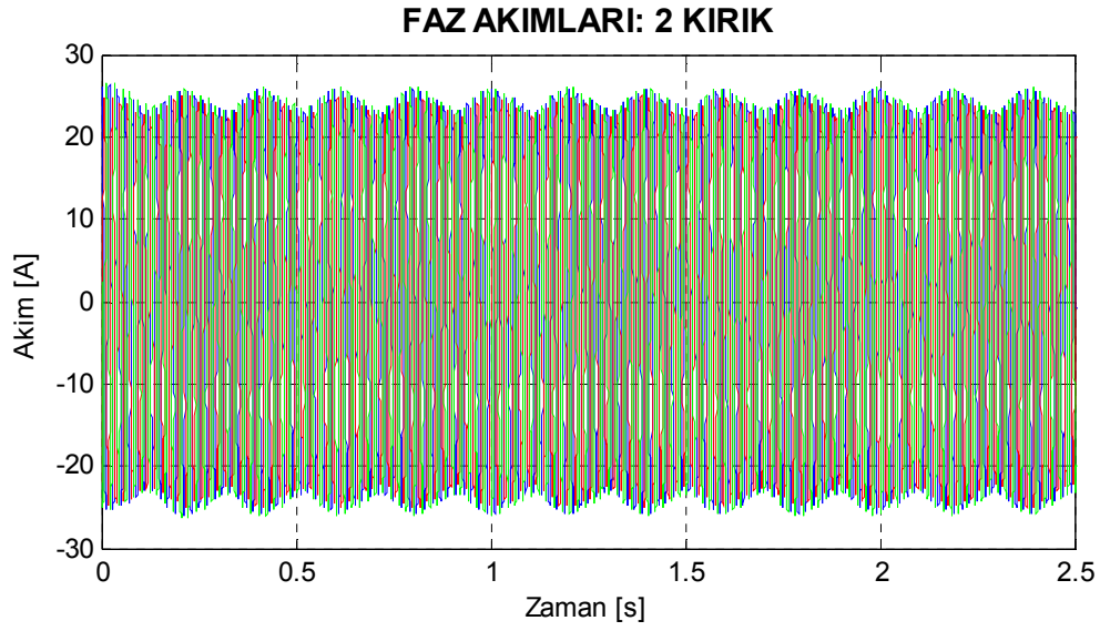
Şekil 8.23. Motor4 iki çubuğu kırık rotor için deneysel stator akımları.
