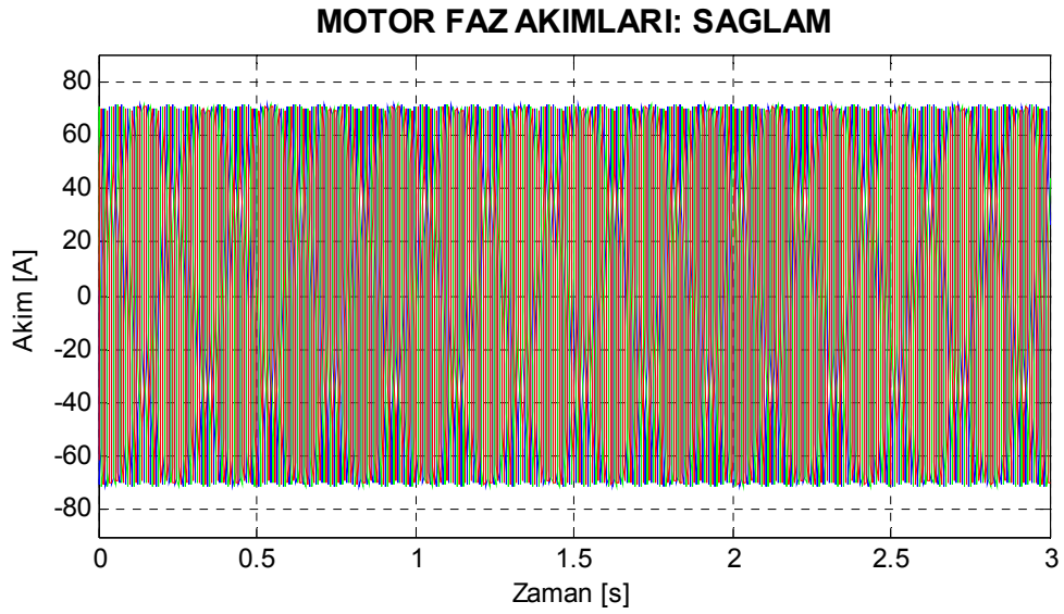
Şekil 7.7. Motor2 sağlam motor durumu için benzetimle elde edilen stator akımları.
