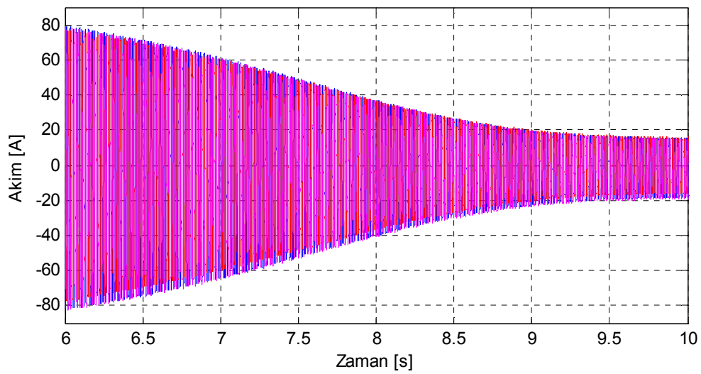
Şekil 8.65. Motor4 sağlam motor durumu için deneysel yol alma akımları.
