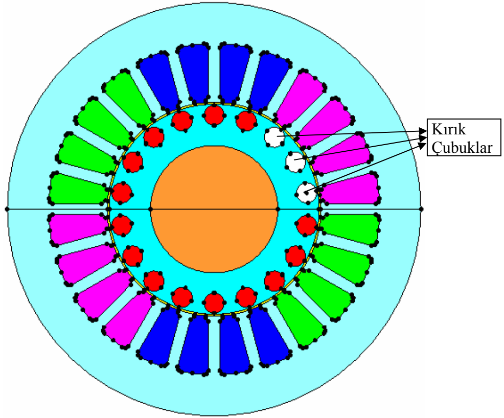
Şekil 5.7. Motor1’de üç kırık çubuk arızası benzetimi için seçilen rotor çubuklarının kesitte gösterimi.
