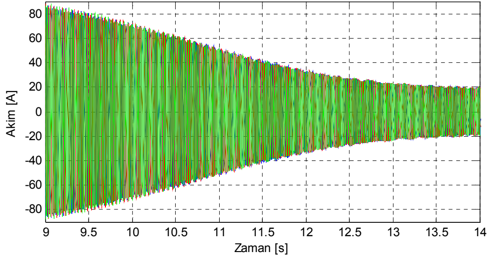
Şekil 7.56. Motor4 bir çubuğu yüksek dirençli rotor için benzetimle elde edilen yol alma akımları.
