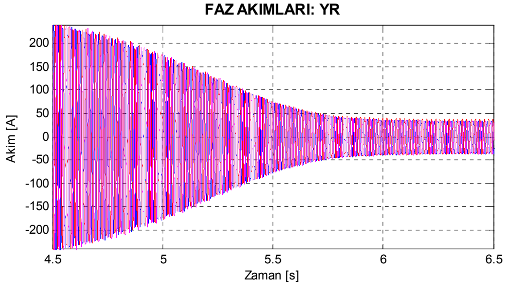
Şekil 8.60. Motor3 bir çubuğu yüksek dirençli rotor için deneysel yol alma akımları.
