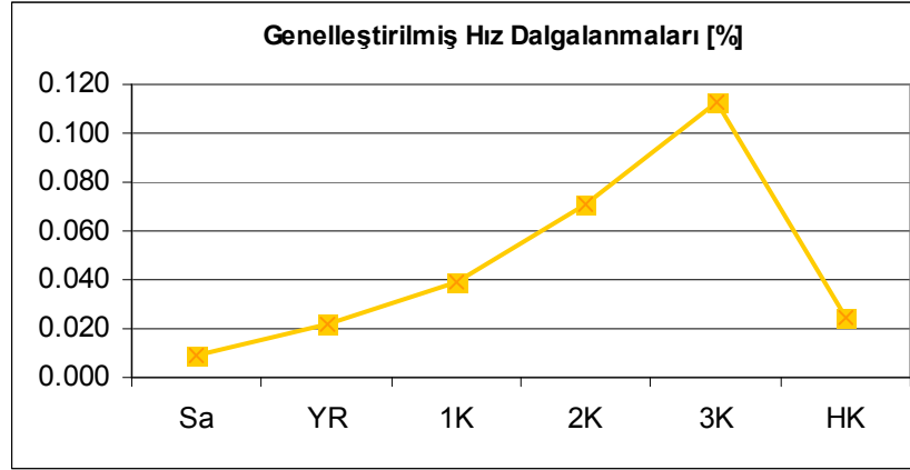
Şekil 9.4. Genelleştirilmiş arızalara göre motor hızlarındaki dalgalanma oranları.
