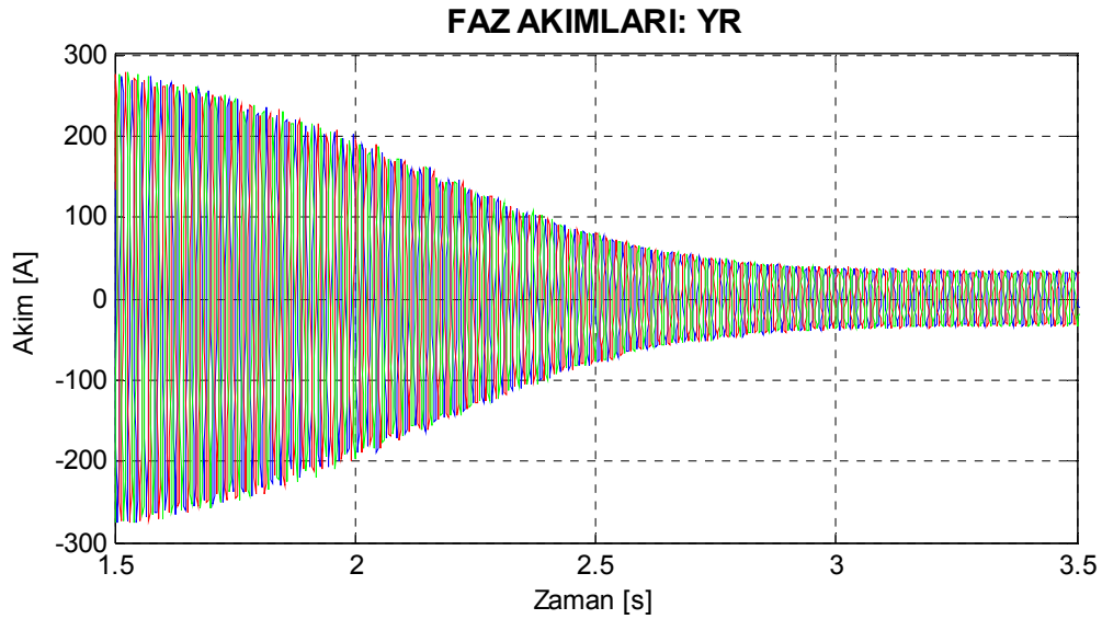
Şekil 7.51. Motor3 bir çubuğu yüksek dirençli rotor için benzetimle elde edilen yol alma akımları.
