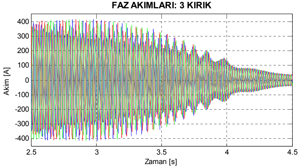
Şekil 7.44. Motor1 üç çubuğu kırık rotor için benzetimle elde edilen yol alma akımları.
