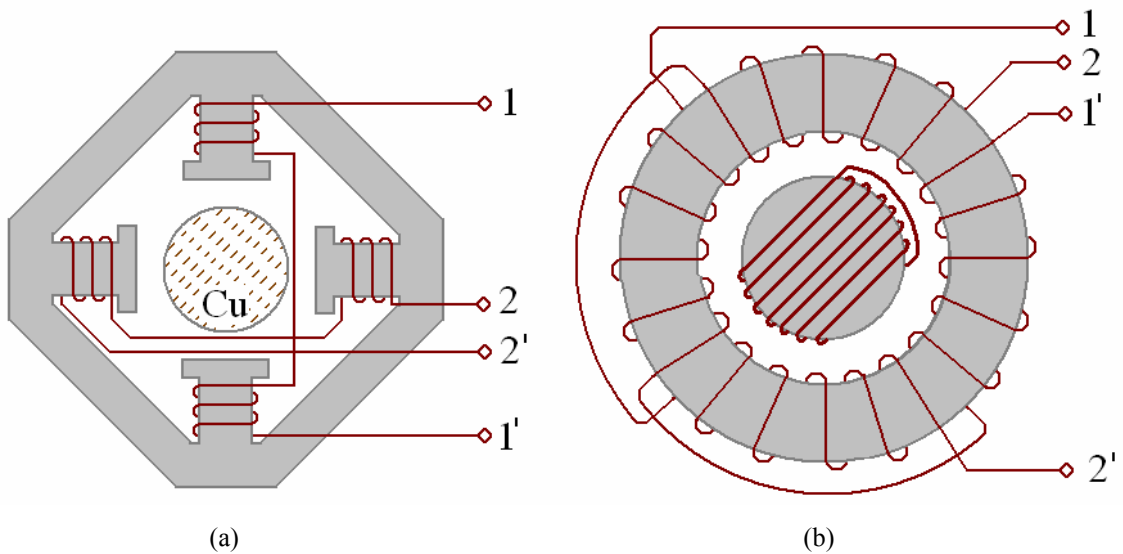
Şekil 3.1. (a) Ferrari'nin asenkron motorunun yapısı, (b) Tesla'nın asenkron motorunun yapısı
