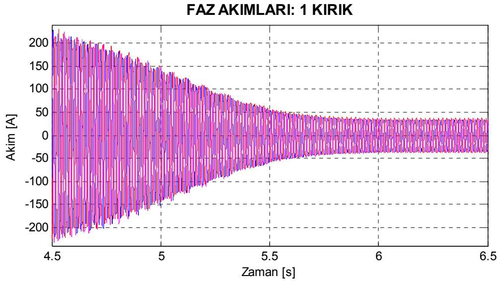
Şekil 8.61. Motor3 bir çubuğu kırık rotor için deneysel yol alma akımları.
