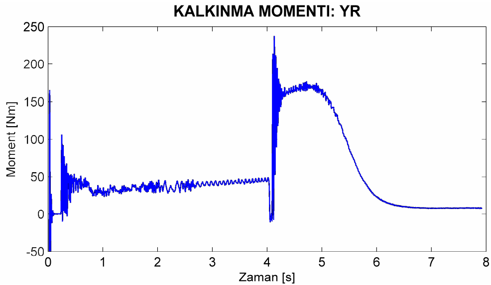
Şekil 8.84. Motor3 bir çubuğu yüksek dirençli rotor için deneysel yol alma momentleri.
