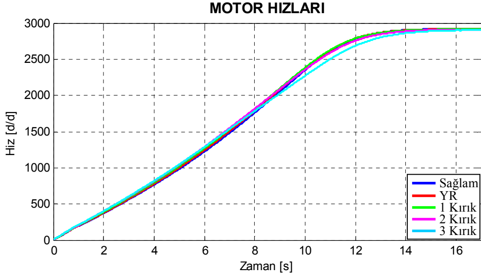
Şekil 7.83. Motor4 için benzetimle elde edilen arıza durumlarına göre çizilmiş yol alma hız grafikleri.
