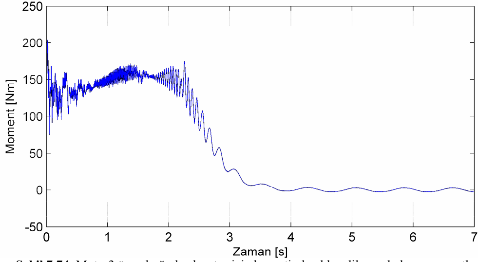
Şekil 7.74. Motor3 üç çubuğu kırık rotor için benzetimle elde edilen yol alma momentleri.
