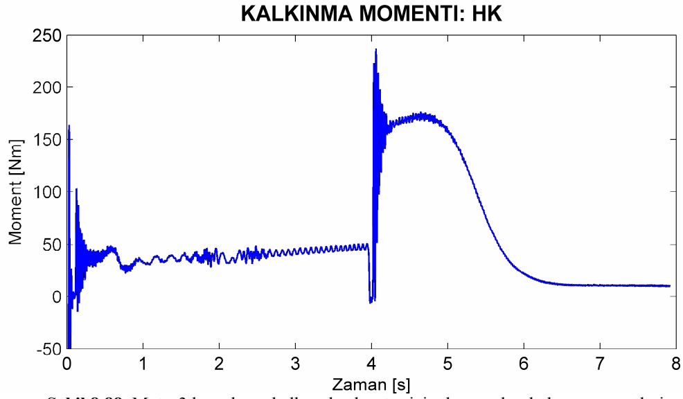
Şekil 8.88. Motor3 kısa devre halkası kırık rotor için deneysel yol alma momentleri.
