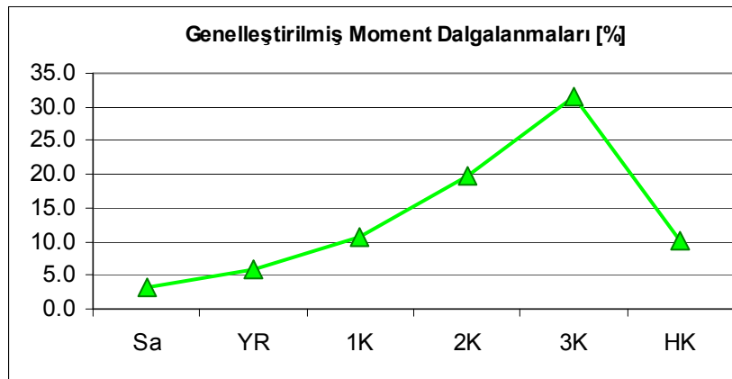
Şekil 9.2. Genelleştirilmiş arızalara göre motor momentlerindeki dalgalanma oranları.
