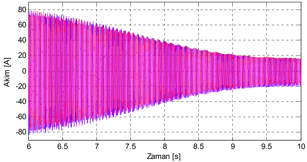
Şekil 8.67. Motor4 bir çubuğu kırık rotor için deneysel yol alma akımları.
