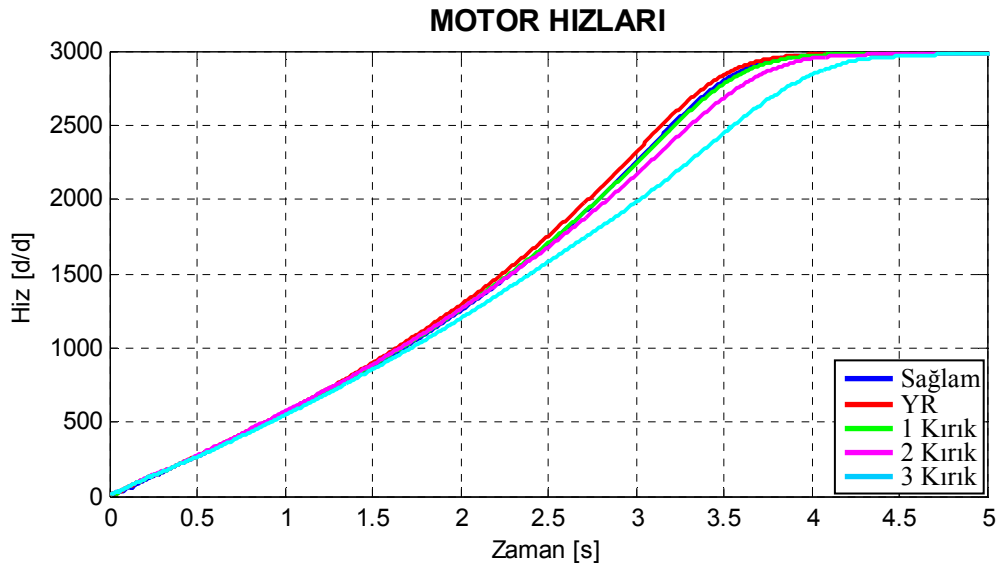
Şekil 7.80. Motor1 için benzetimle elde edilen arıza durumlarına göre çizilmiş yol alma hız grafikleri.
