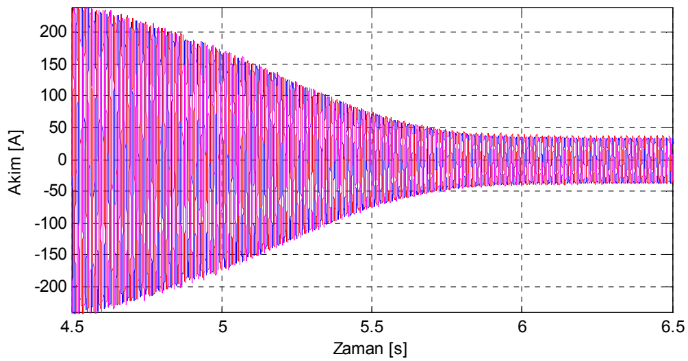
Şekil 8.59. Motor3 sağlam motor durumu için deneysel yol alma akımları.
