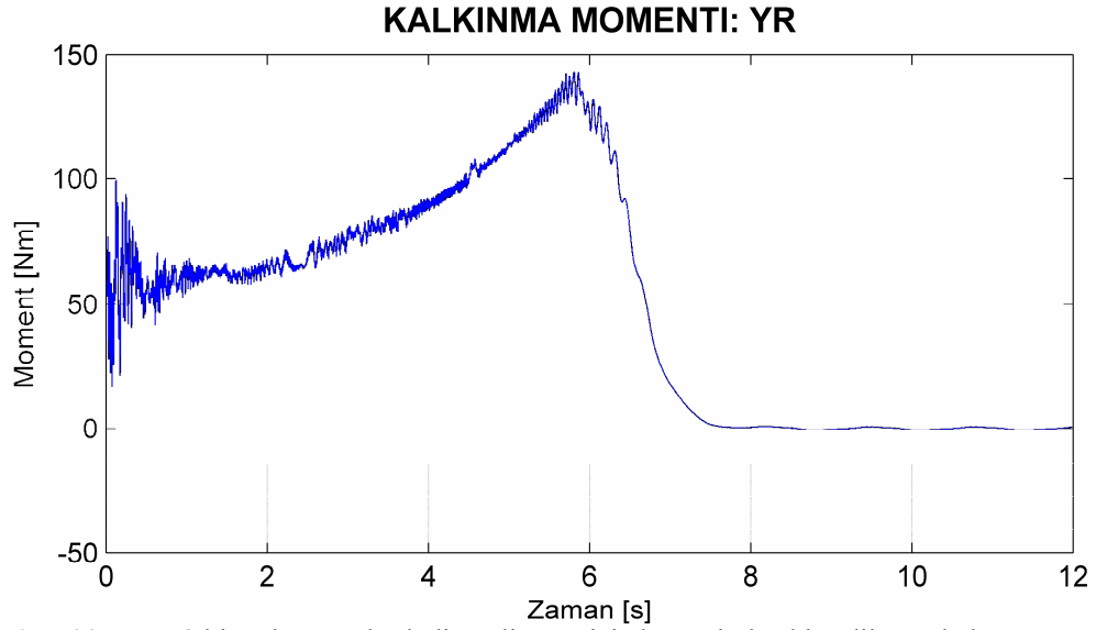
Şekil 7.66. Motor2 bir çubuğu yüksek dirençli rotor için benzetimle elde edilen yol alma momentleri.
