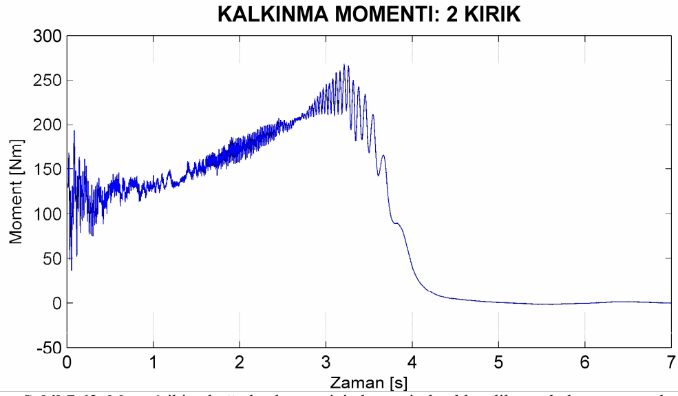
Şekil 7.63. Motor1 iki çubuğu kırık rotor için benzetimle elde edilen yol alma momentleri.
