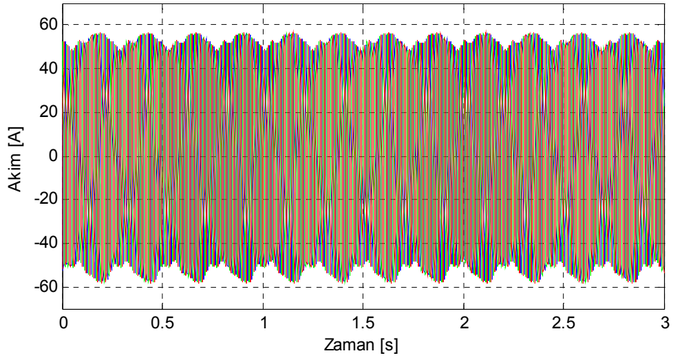
Şekil 7.15. Motor3 iki çubuğu kırık rotor için benzetimle elde edilen stator akımları.
