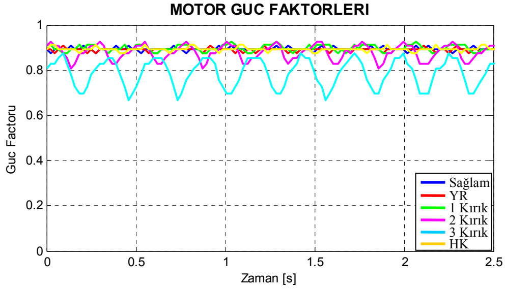
Şekil 8.35. Motor2 için deneysel arıza durumlarına göre çizilmiş güç faktörü grafikleri.
