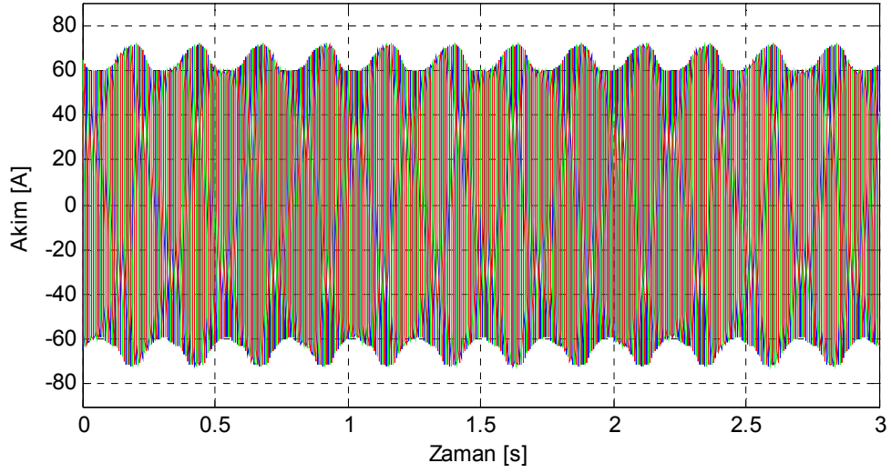
Şekil 7.10. Motor2 iki çubuğu kırık rotor için benzetimle elde edilen stator akımları.
