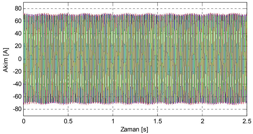
Şekil 8.13. Motor2 kısa devre halkası kırık rotor için deneysel stator akımları.
