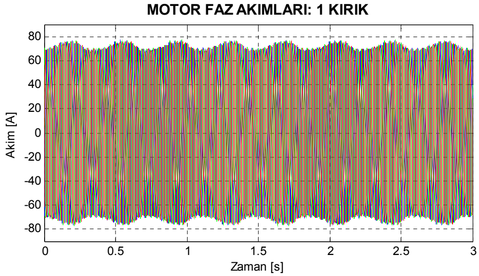
Şekil 7.4. Motor1 bir çubuğu kırık rotor için benzetimle elde edilen stator akımları.
