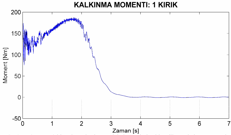
Şekil 7.72. Motor3 bir çubuğu kırık rotor için benzetimle elde edilen yol alma momentleri.
