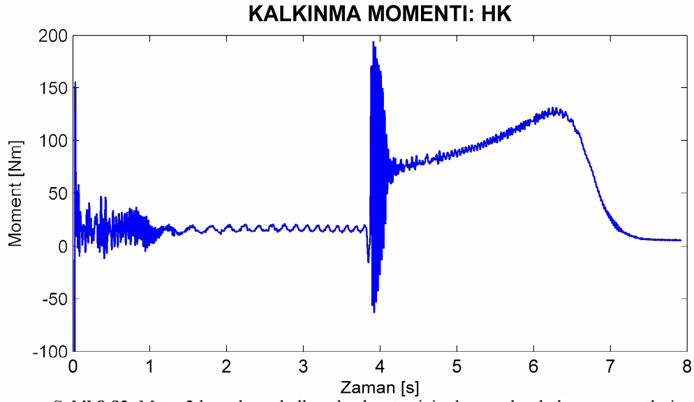
Şekil 8.82. Motor2 kısa devre halkası kırık rotor için deneysel yol alma momentleri.
