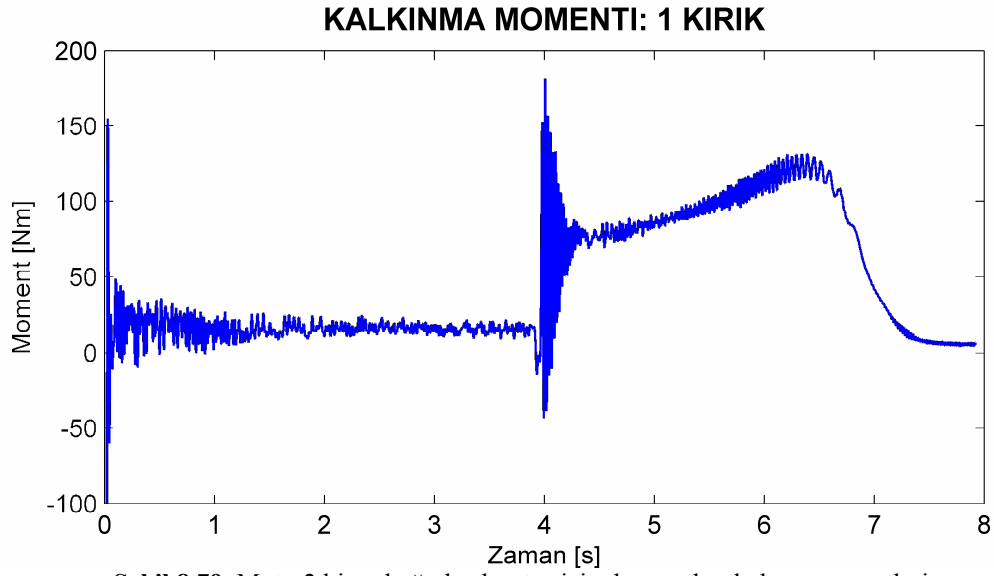
Şekil 8.79. Motor2 bir çubuğu kırık rotor için deneysel yol alma momentleri.
