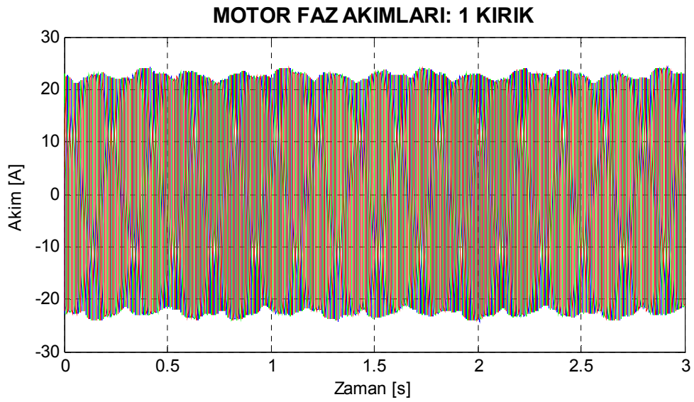
Şekil 7.19. Motor4 bir çubuğu kırık rotor için benzetimle elde edilen stator akımları.
