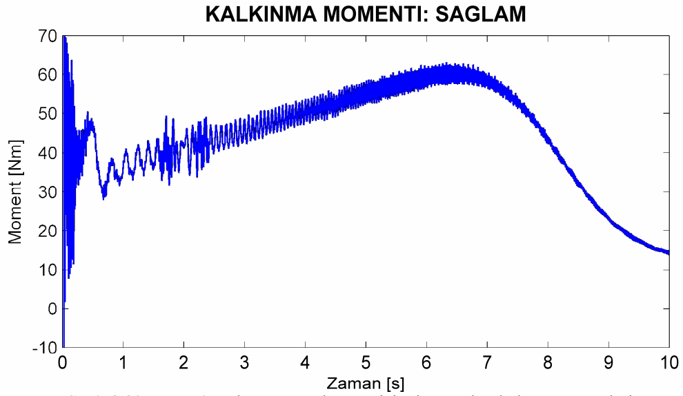
Şekil 8.89. Motor4 sağlam motor durumu için deneysel yol alma momentleri.
