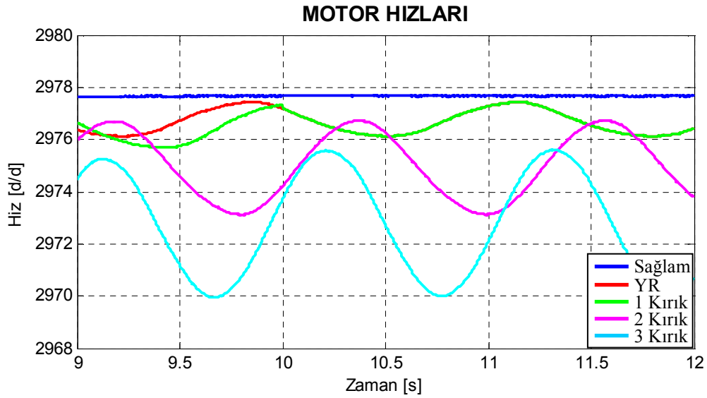
Şekil 7.24. Motor2 için benzetimle elde edilen arıza durumlarına göre çizilmiş hız-zaman grafikleri.
