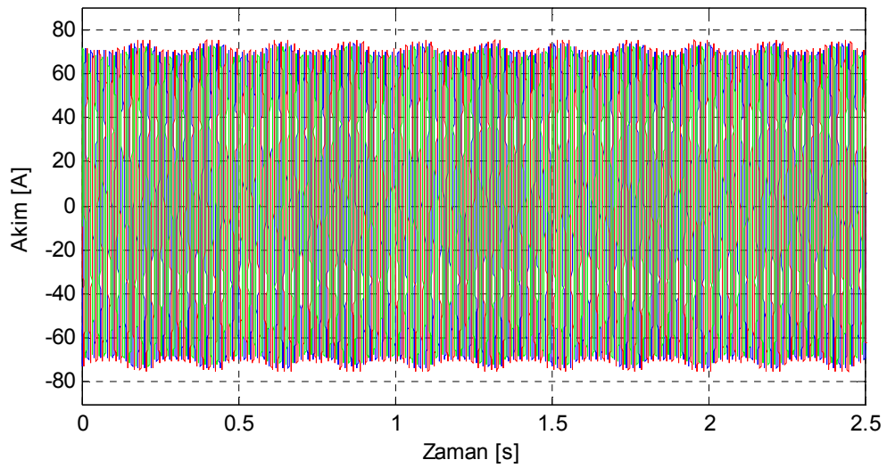
Şekil 8.10. Motor2 bir çubuğu kırık rotor için deneysel stator akımları.
