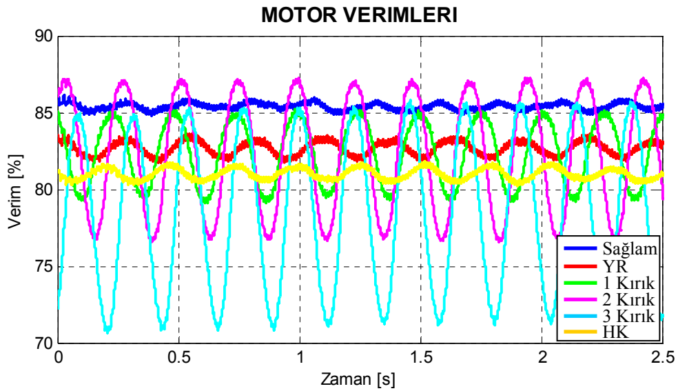
Şekil 8.44. Motor3 için deneysel arıza durumlarına göre çizilmiş verim grafikleri.
