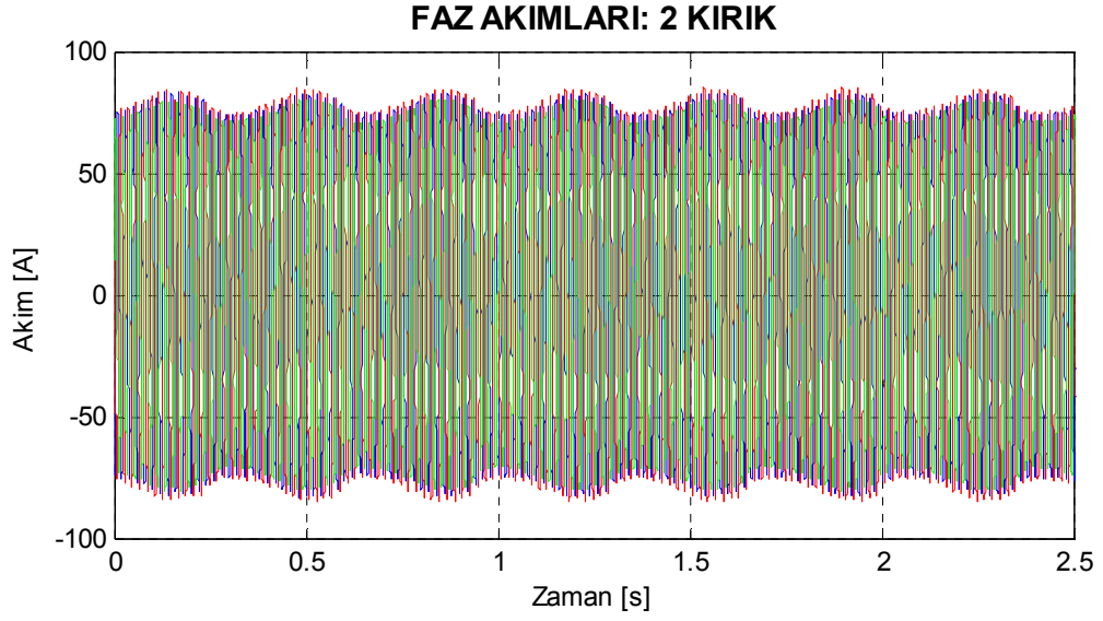
Şekil 8.5. Motor1 iki çubuğu kırık rotor için deneysel stator akımları.
