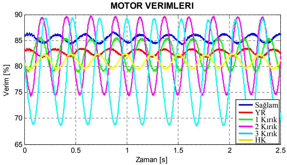
Şekil 8.43. Motor2 için deneysel arıza durumlarına göre çizilmiş verim grafikleri.
