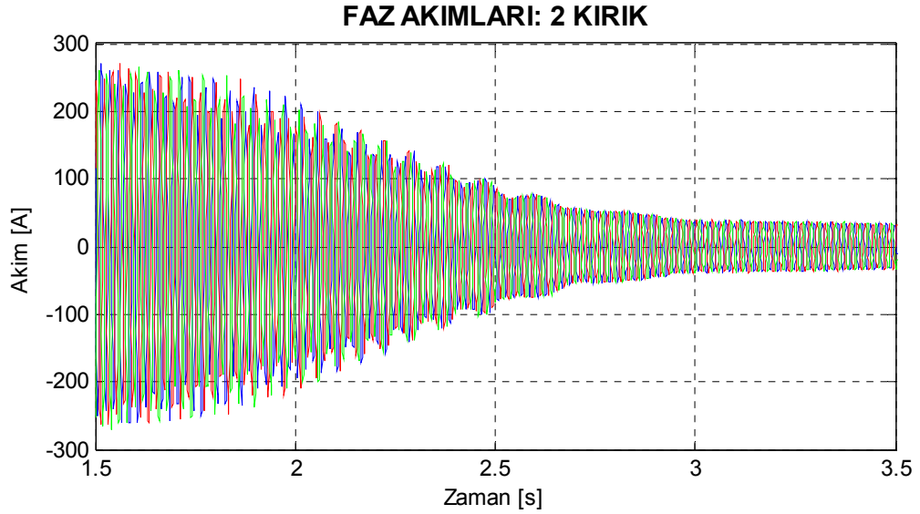
Şekil 7.53. Motor3 iki çubuğu kırık rotor için benzetimle elde edilen yol alma akımları.
