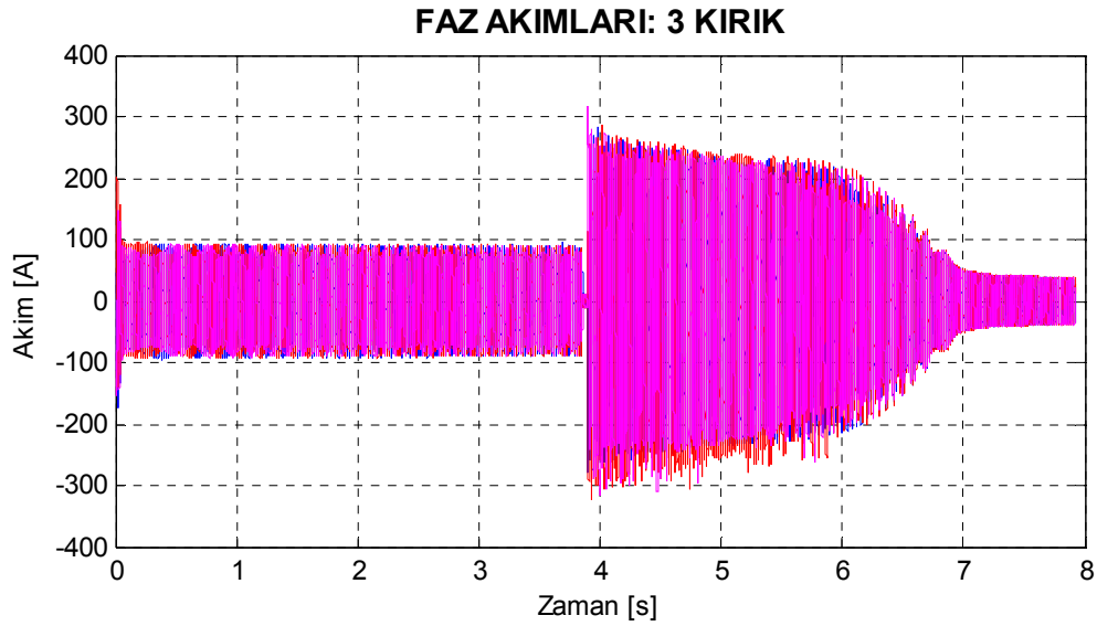
Şekil 8.46. Motor1 üç kırık çubuklu rotor arızası için yol alma sürecinin tamamı için çizilen deneysel motor akım grafiği.
