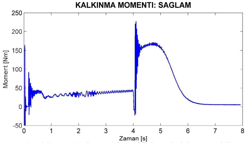
Şekil 8.83. Motor3 sağlam motor durumu için deneysel yol alma momentleri.
