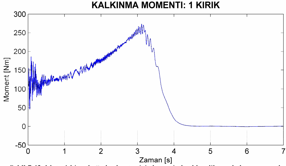
Şekil 7.62. Motor1 bir çubuğu kırık rotor için benzetimle elde edilen yol alma momentleri.
