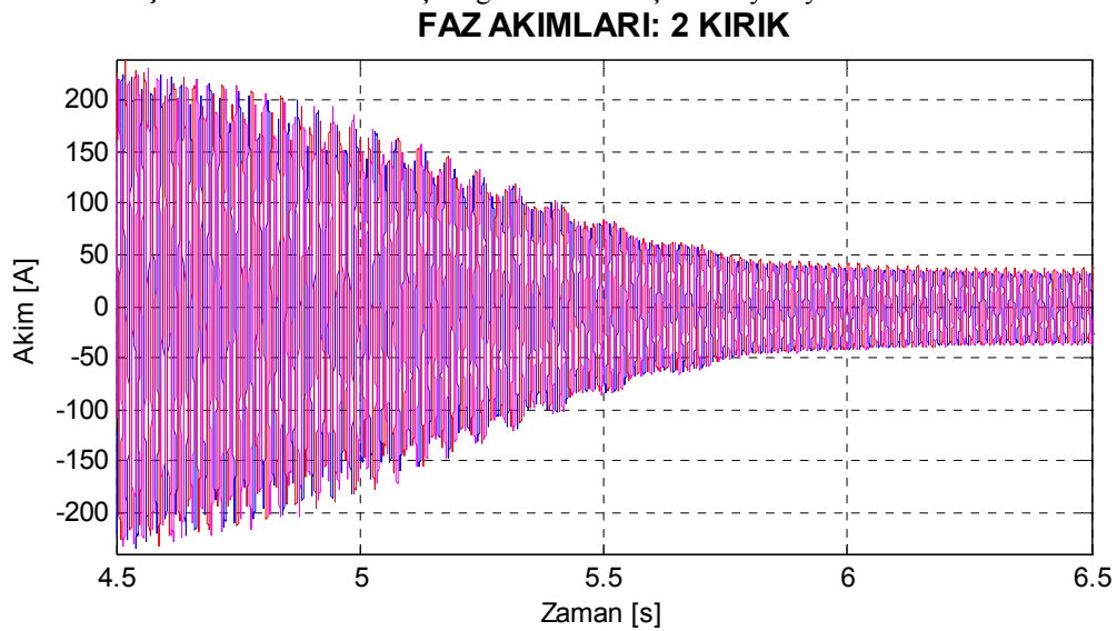
Şekil 8.62. Motor3 iki çubuğu kırık rotor için deneysel yol alma akımları.
