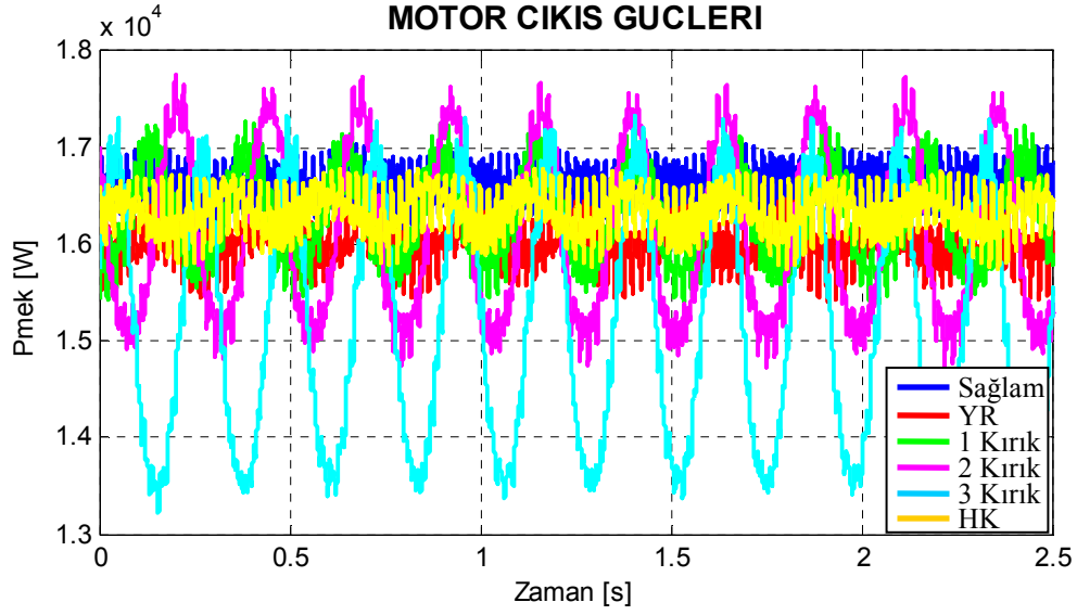
Şekil 8.40. Motor3 için deneysel arıza durumlarına göre çizilmiş mekanik güç grafikleri.
