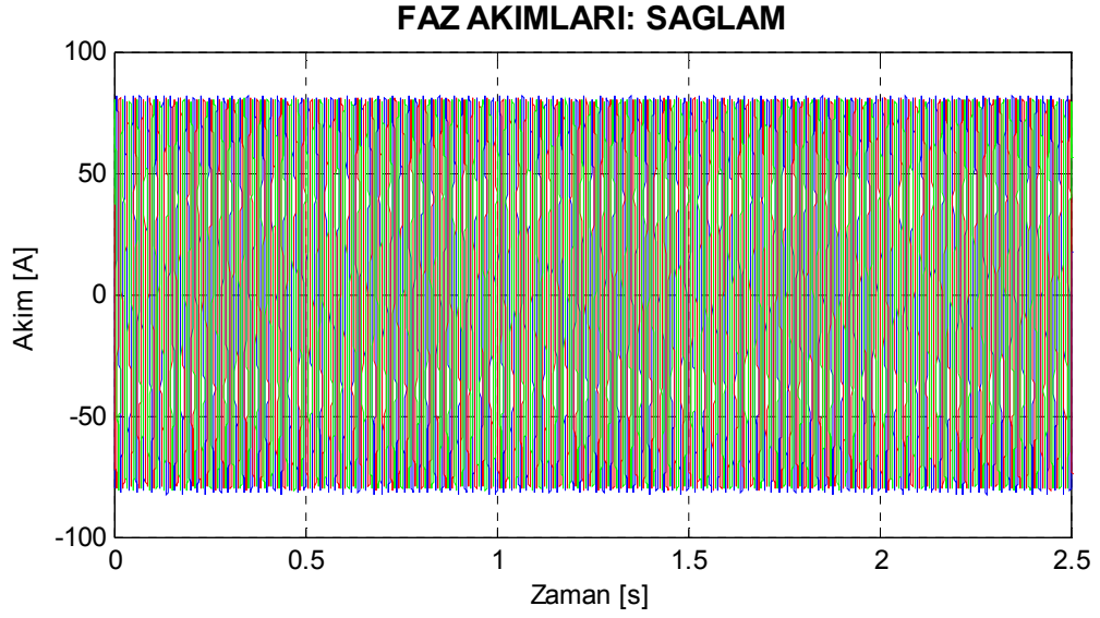
Şekil 8.2. Motor1 sağlam motor durumu için deneysel stator akımları.
