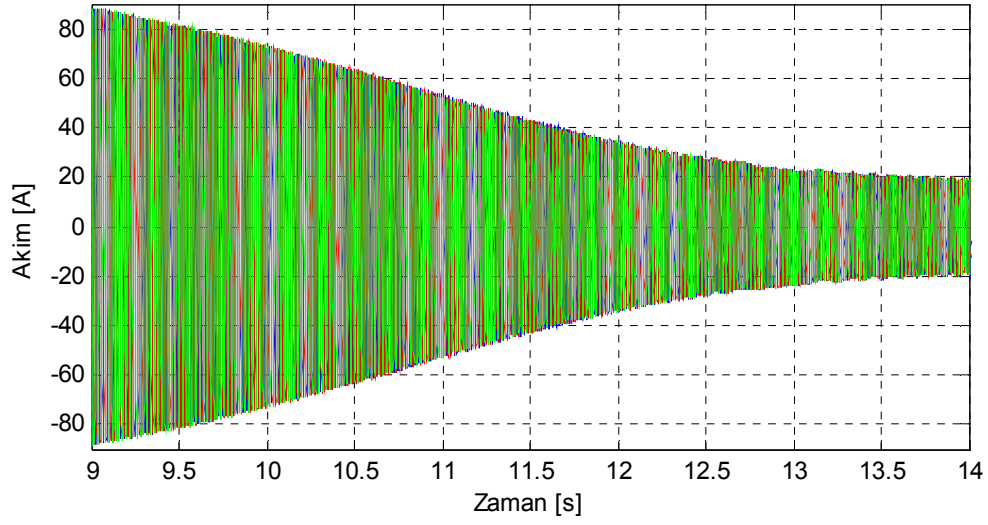
Şekil 7.55. Motor4 sağlam motor durumu için benzetimle elde edilen yol alma akımları.
