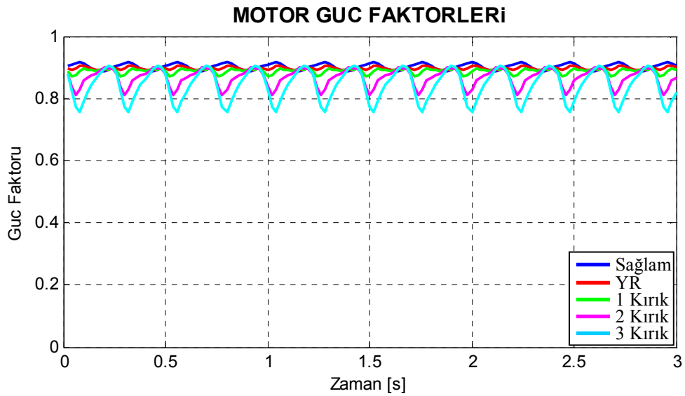
Şekil 7.29. Motor3 için benzetimle elde edilen arıza durumlarına göre çizilmiş güç faktörü grafikleri.
