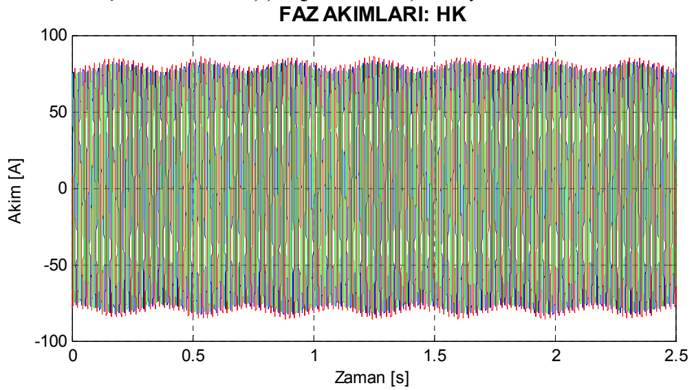
Şekil 8.7. Motor1 kısa devre halkası kırık rotor için deneysel stator akımları.
