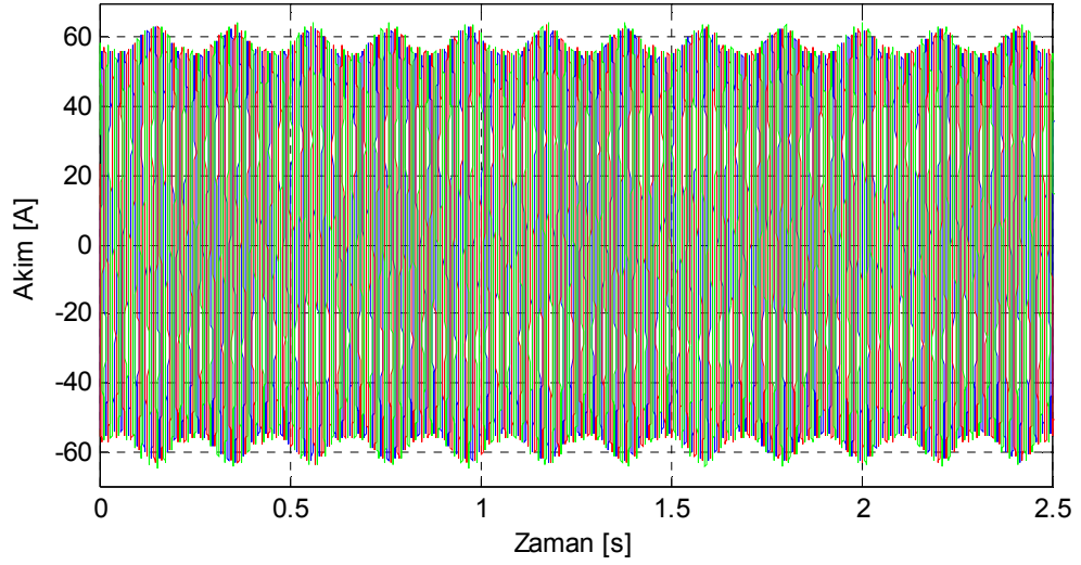
Şekil 8.18. Motor3 üç çubuğu kırık rotor için deneysel stator akımları.
