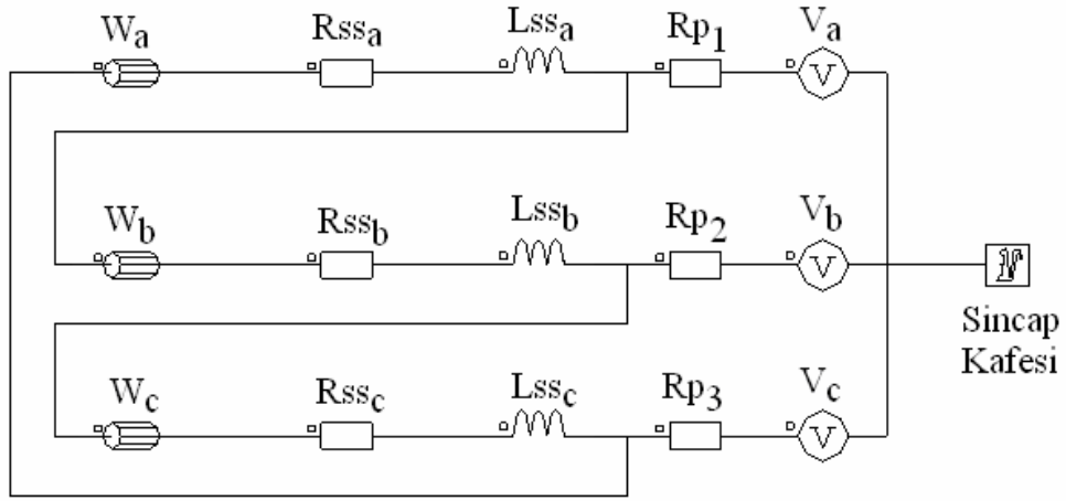
Şekil 5.3. Benzetimde kullanılan Motor1, Motor2 ve Motor3 için Flux programında çizilmiş elektriksel devresi.
