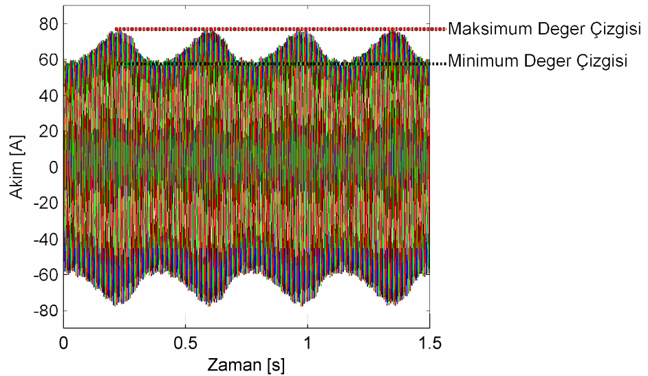
Şekil 4.1. Motor akımının dalgalanma hesabında kullanılan değerlerin gösterimi.
