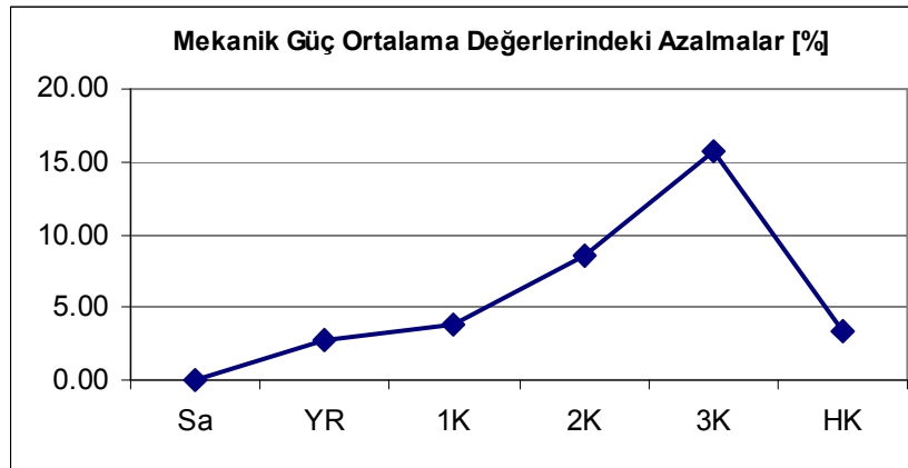
Şekil 9.9. Ortalama mekanik güç değerlerindeki azalmanın genelleştirilmiş oranlarının arızalara göre gösterimi.
