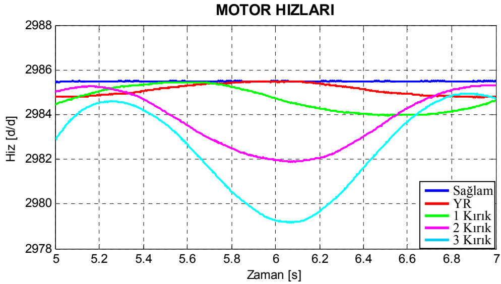
Şekil 7.23. Motor1 için benzetimle elde edilen arıza durumlarına göre çizilmiş hız-zaman grafikleri.
