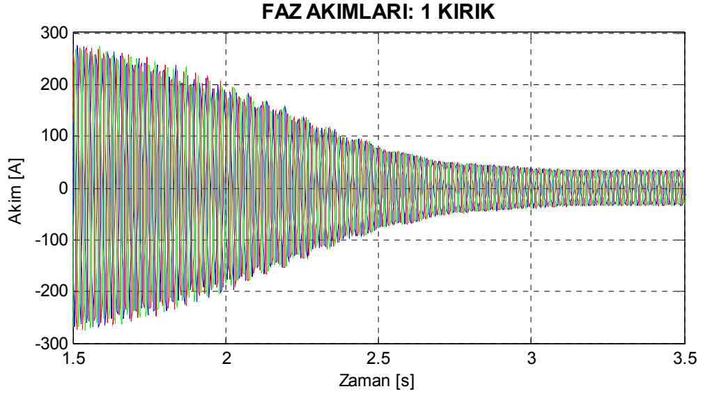
Şekil 7.52. Motor3 bir çubuğu kırık rotor için benzetimle elde edilen yol alma akımları.
