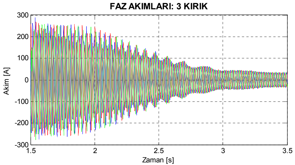
Şekil 7.54. Motor3 üç çubuğu kırık rotor için benzetimle elde edilen yol alma akımları.
