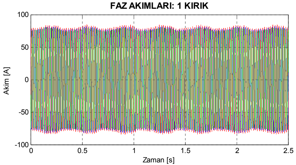
Şekil 8.4. Motor1 bir çubuğu kırık rotor için deneysel stator akımları.
