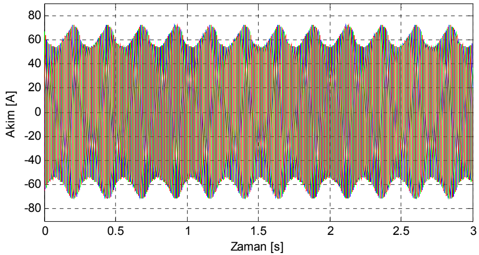
Şekil 7.11. Motor2 üç çubuğu kırık rotor için benzetimle elde edilen stator akımları.
