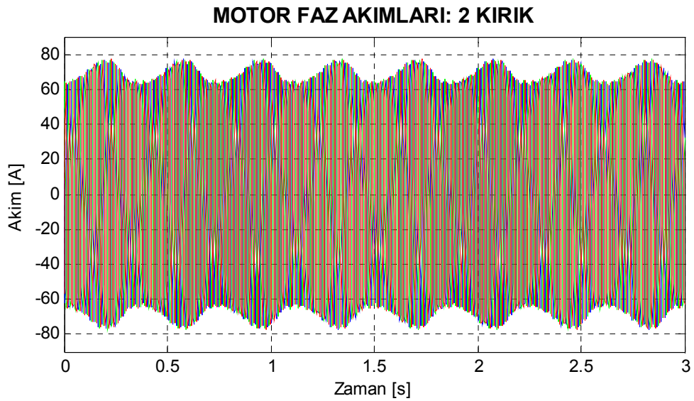
Şekil 7.5. Motor1 iki çubuğu kırık rotor için benzetimle elde edilen stator akımları.
