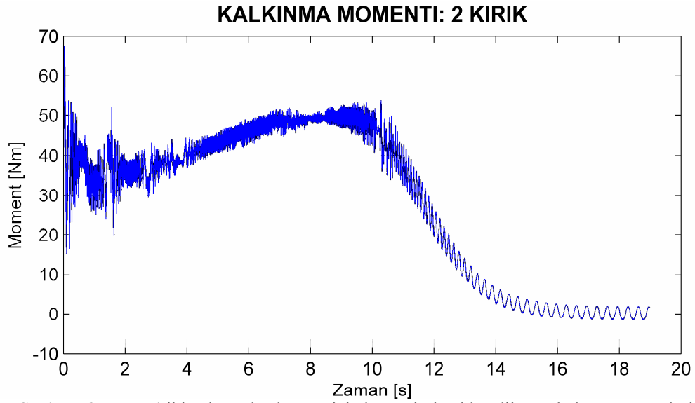
Şekil 7.78. Motor4 iki çubuğu kırık rotor için benzetimle elde edilen yol alma momentleri.
