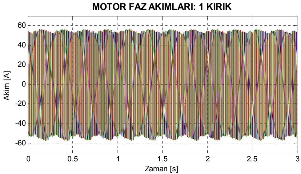
Şekil 7.14. Motor3 bir çubuğu kırık rotor için benzetimle elde edilen stator akımları.
