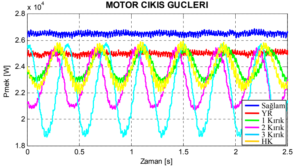
Şekil 8.38. Motor1 için deneysel arıza durumlarına göre çizilmiş mekaniki güç grafikleri.
