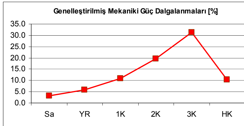
Şekil 9.8. Arızalara göre motor mekaniki güçlerindeki genelleştirilmiş dalgalanma oranları.
