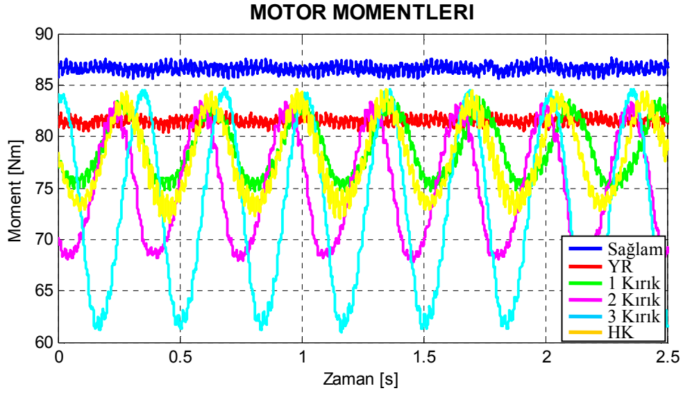
Şekil 8.26. Motor1 için deneysel arıza durumlarına göre çizilmiş moment grafikleri.
