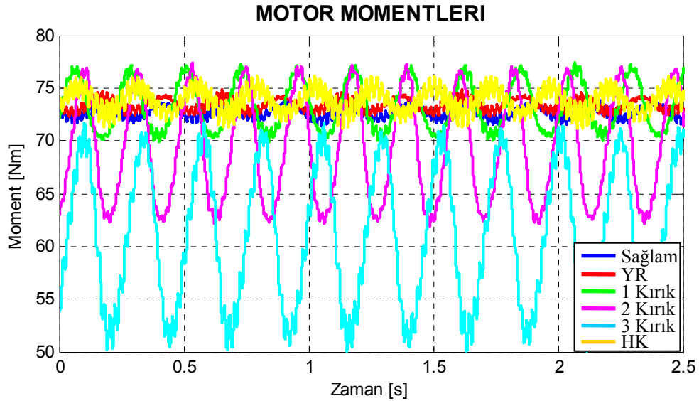
Şekil 8.27. Motor2 için deneysel arıza durumlarına göre çizilmiş moment grafikleri.
