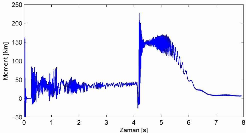
Şekil 8.87. Motor3 üç çubuğu kırık rotor için deneysel yol alma momentleri.
