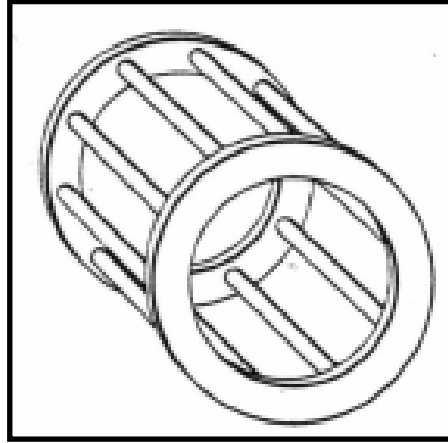
Şekil 3.4. Rotordaki sincap kafesinin yapısı.
