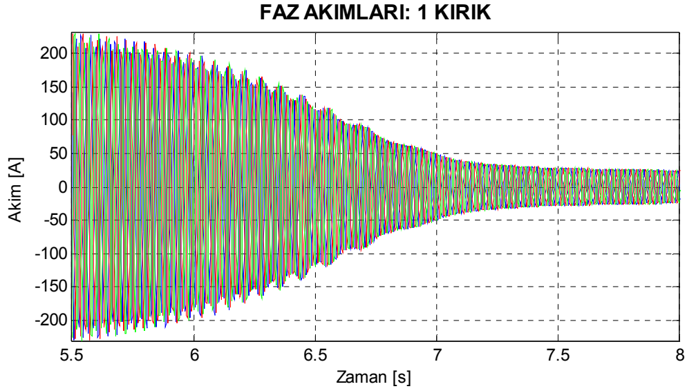
Şekil 7.47. Motor2 bir çubuğu kırık rotor için benzetimle elde edilen yol alma akımları.
