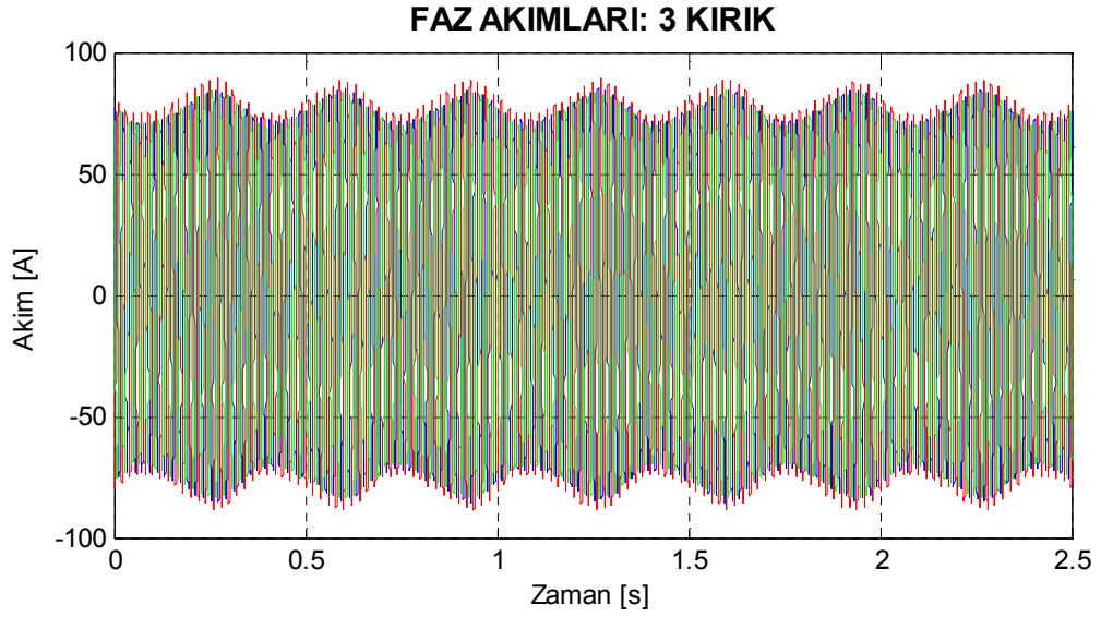
Şekil 8.6. Motor1 üç çubuğu kırık rotor için deneysel stator akımları.
